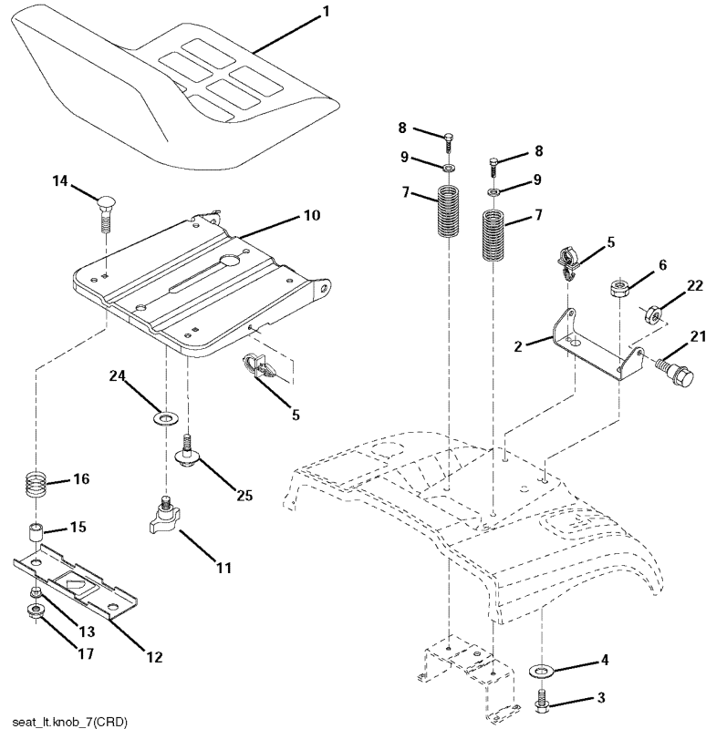
シート FIG.09 SEAT ASSEMBLY
