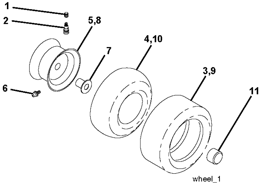
FIG.02 ホイル WHEELS&TIRES
