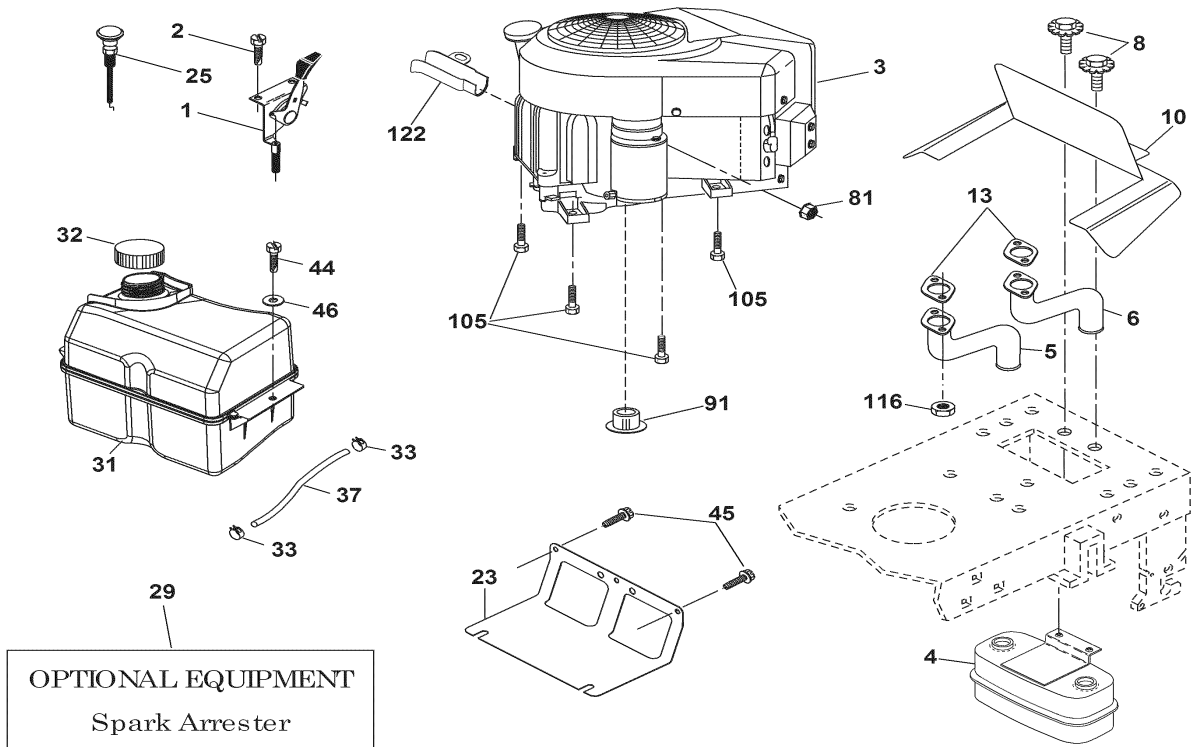
FIG. 08 エンジン ENGINE
