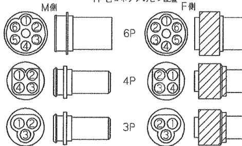
YPCコネクタのピン配置
