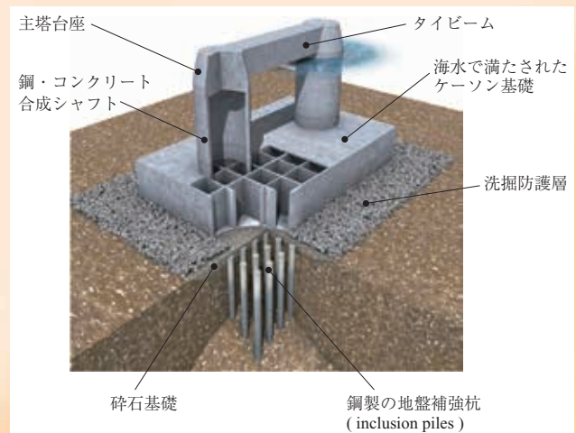
主塔基礎
