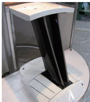
構造用ガイドベーン(SGV)
