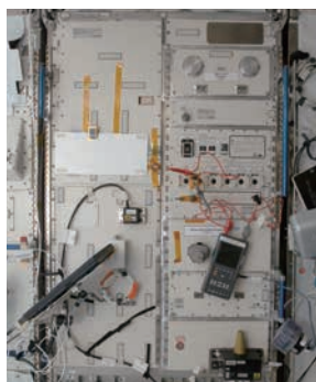
勾配炉ラック
