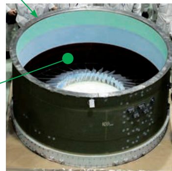
FAN-SGVモジュール
