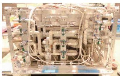
沸騰・二相流実験装置(TPF)
