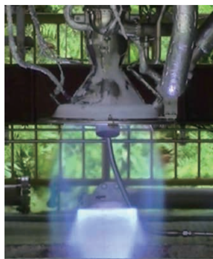
再生冷却LNGエンジン
