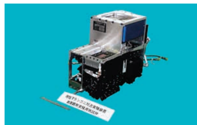
マランゴニ対流実験用供試体
