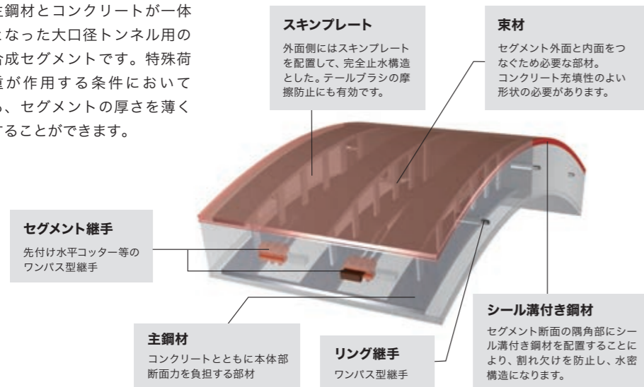
セグメント内面
