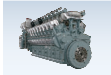
ガスエンジン 18V28AGS
