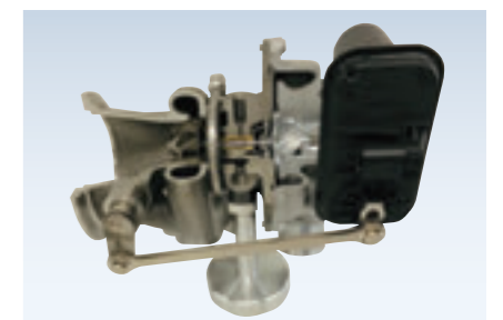
車両用ターボチャージャ
