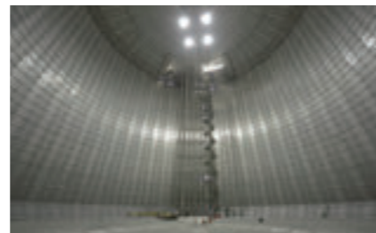
世界最大容量LNG地下タンク(メンブレン) 写真提供:東京ガス(株)
