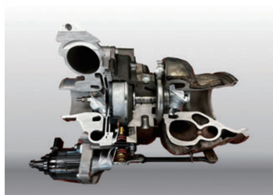
ハイブリッド自動車向け電動アシストターボ
