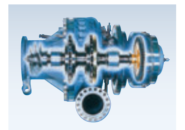
ロケットエンジン用液体水素ターボポンプ
