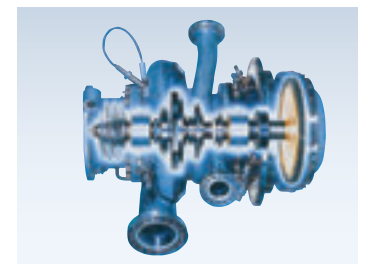
ロケットエンジン用液体酸素ターボポンプ
