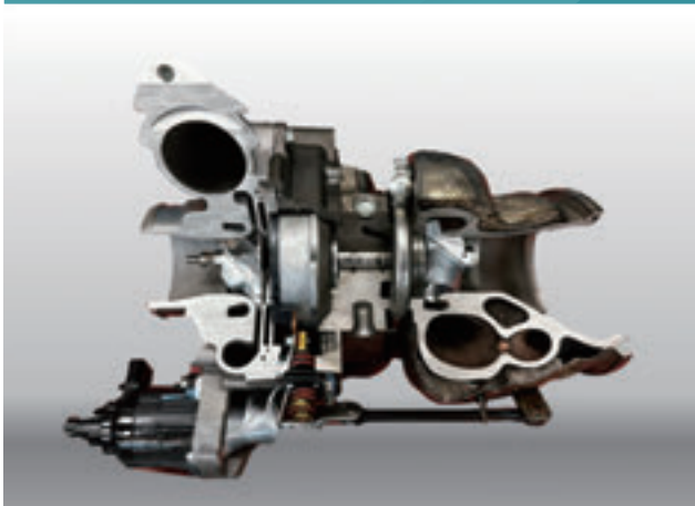
ハイブリッド自動車向け電動アシストターボ
