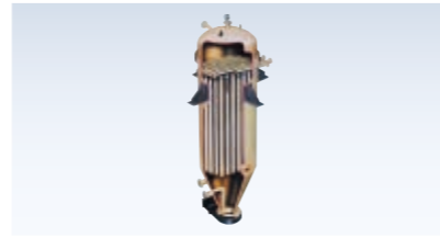
IHI - FUNDABAC 过滤器
