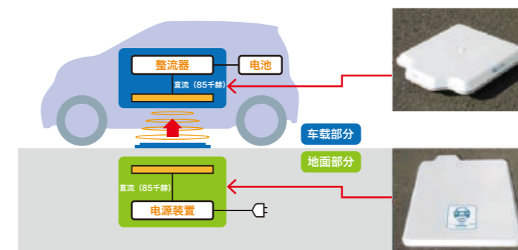
利用磁场，从地面向车载的线圈单元充电
