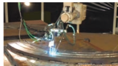
自律型焊接技术的开发 (全自动焊接)
