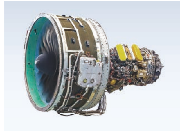
PW1100G-JM型 涡轮扇引擎
