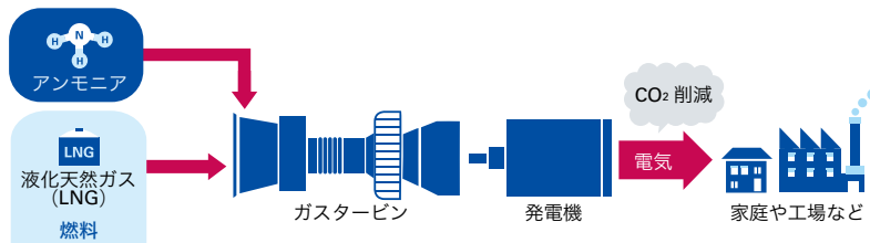
アンモニア混焼ガスタービン試験設備 (IHI 横浜事業所内)
