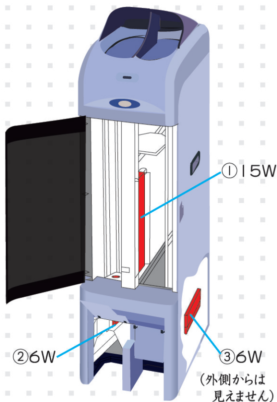
■紫外線ランプの位置
