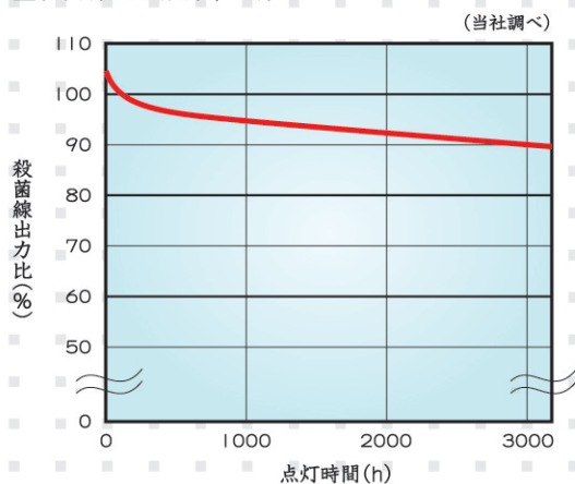
■殺菌線出力維持率曲線
