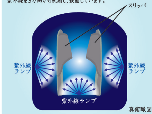
■スリッパ殺菌のしくみ
