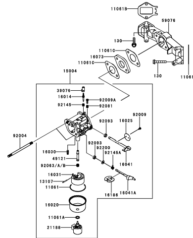
B-10 CARBURETOR
