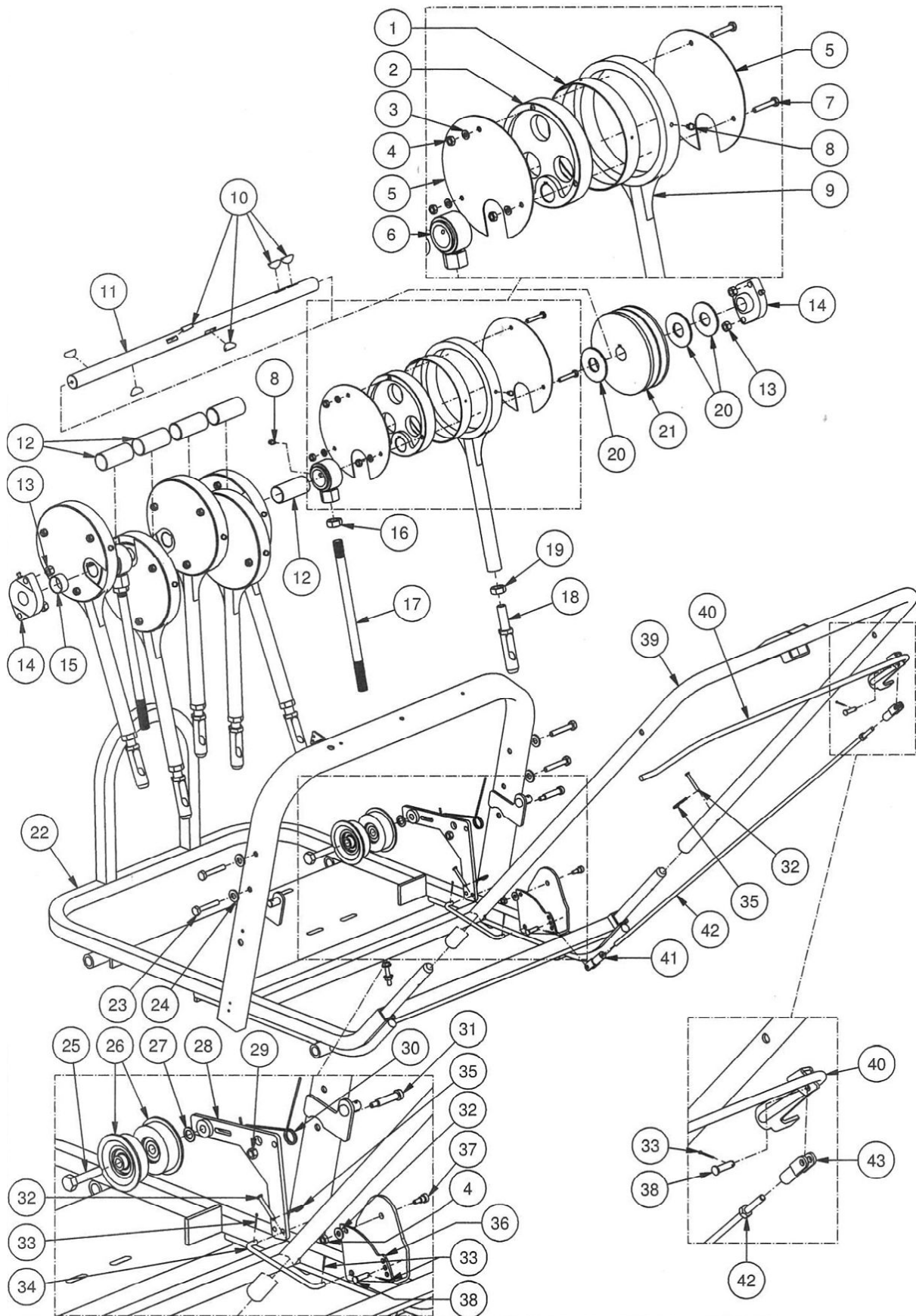
FIG. 102 クランク、タイン、フレーム CRANK, TINE, FRAME
