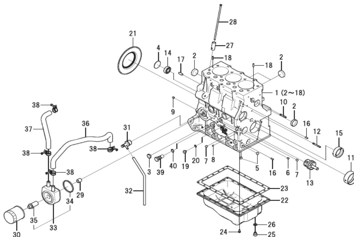
シリンダ ブロック CYLINDER BLOCK
