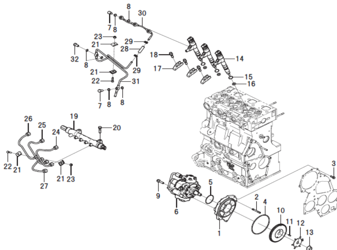
FIG. 109 インジェクタ・HP ポンプ & フュエル フィルタ INJECTOR・HP PUMP & FUEL FILTER
