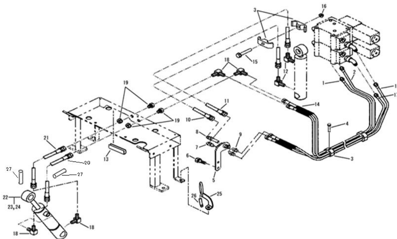
FIG. 220 ユアツ ハイカン ; バルブ ~ シリンダ HYDRAULIC PIPING ; VALVE ~ CYLINDER
