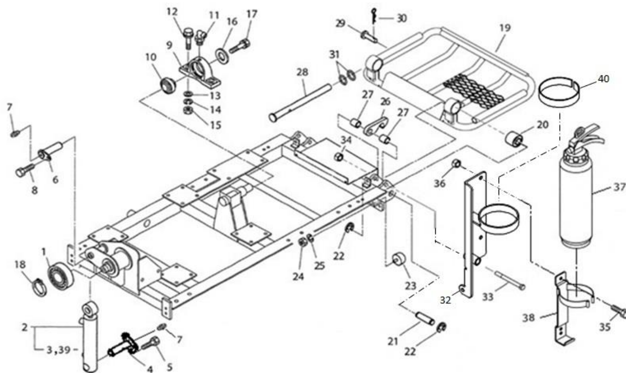
シリンダ & ステップ CYLINDER & STEP
