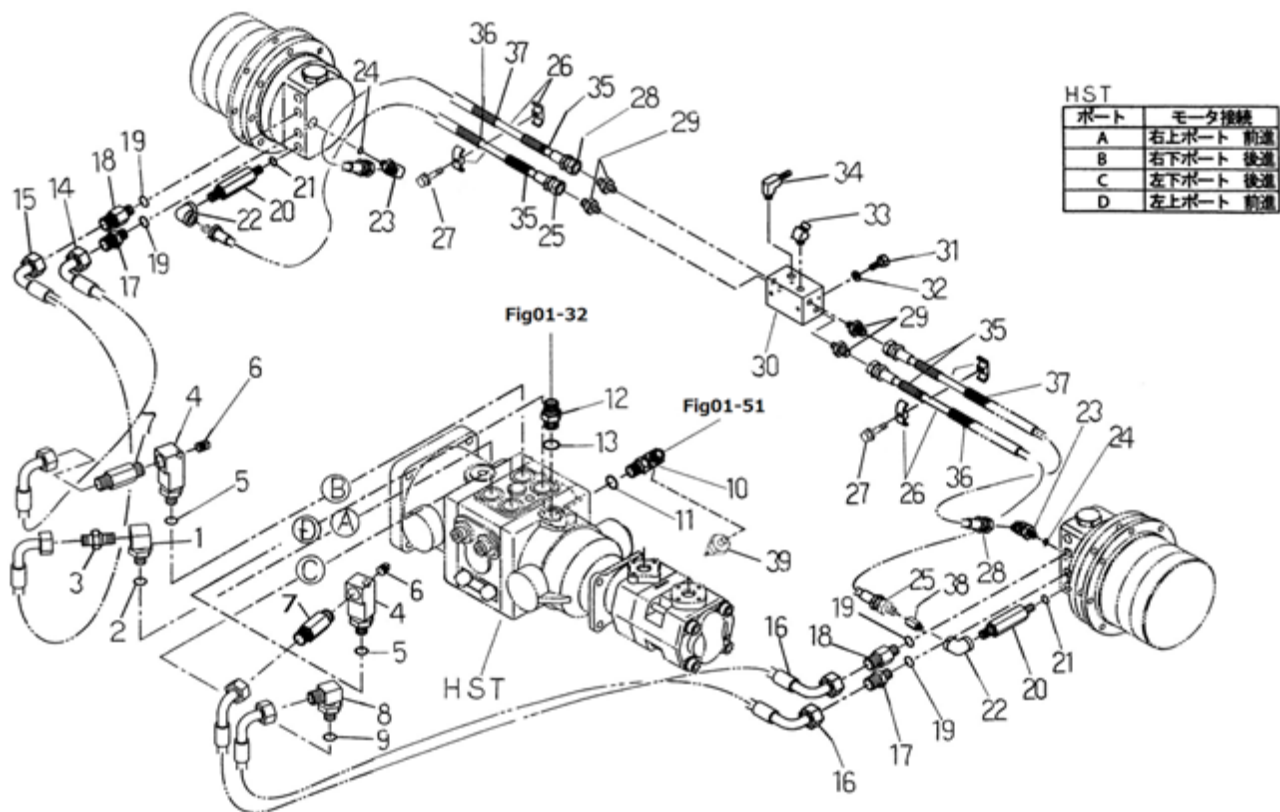
FIG. 217 ユアツ ハイカン ; HST HYDRAULIC PIPING ; HST
