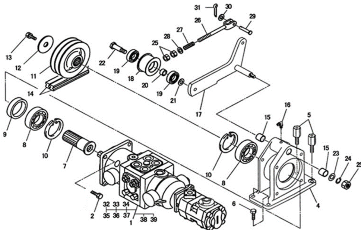
HST ポンプ & テンション HST PUMP & TENSION
