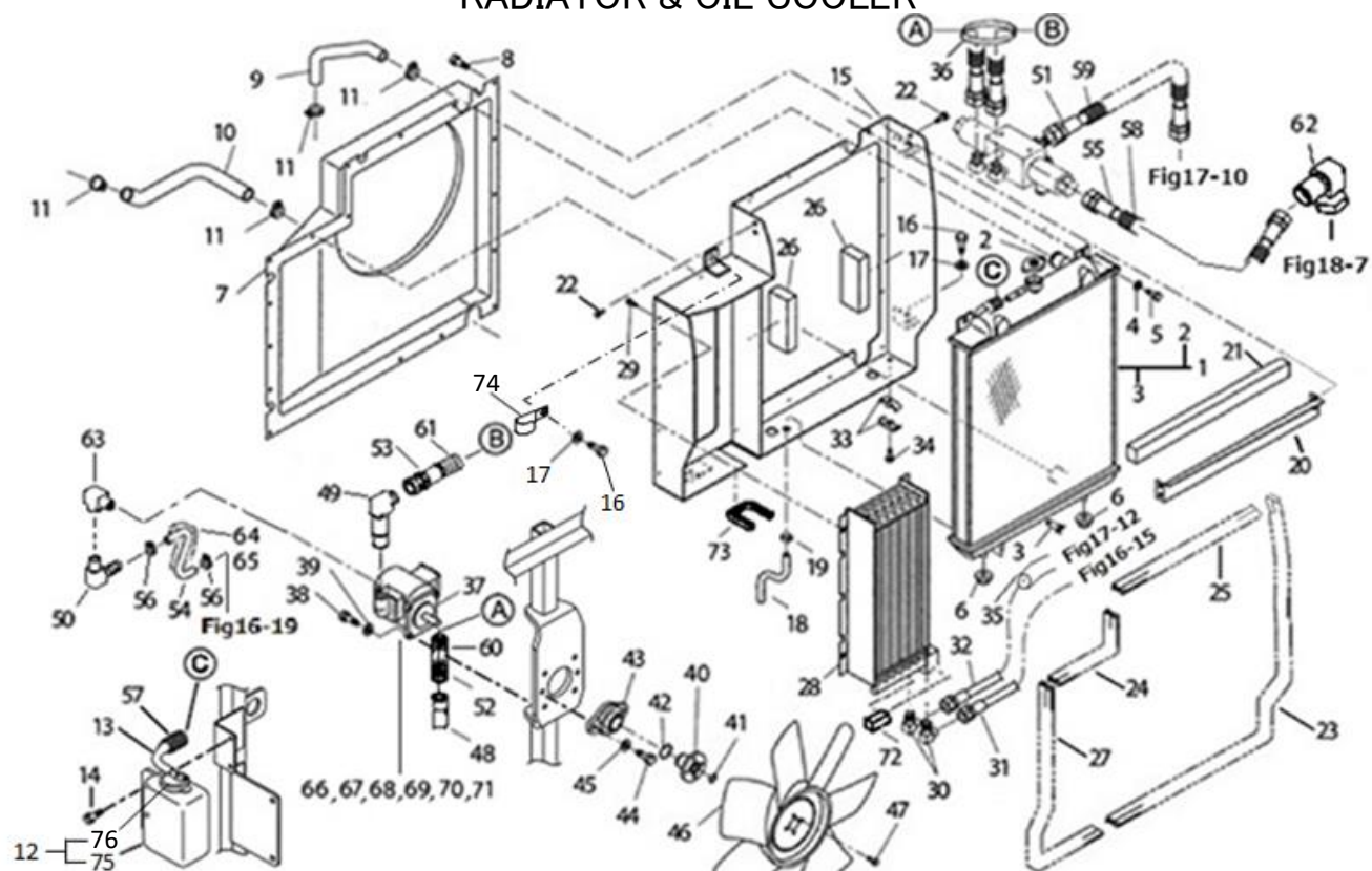
ラジエータ & オイルクーラ RADIATOR & OIL COOLER
