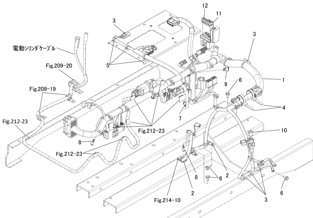
FIG.213 ワイヤハーネス WIRE HARNESS
