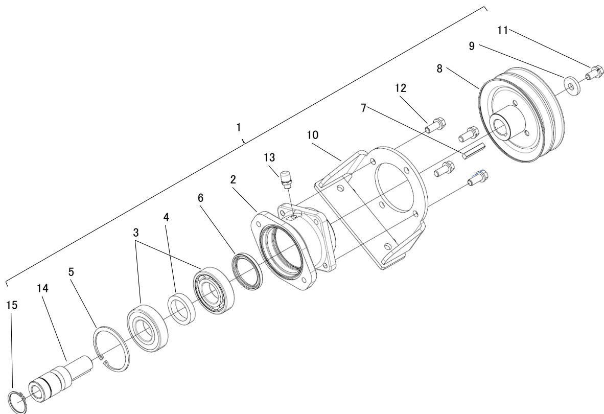
FIG.302 モア;モータベアリング MOWER;MOTOR BEARING
