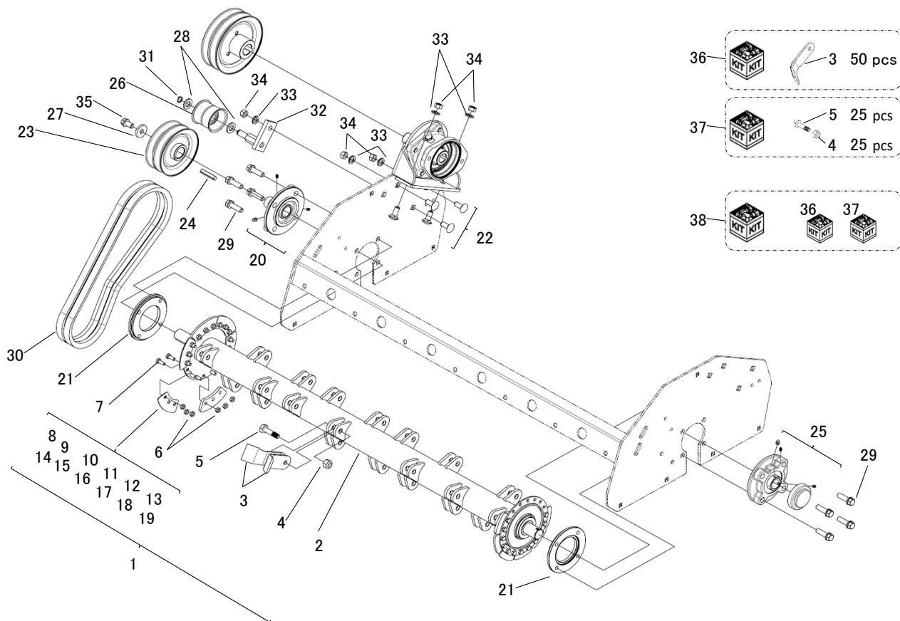
FIG.303 モア;伝動 MOWER;DRIVING
