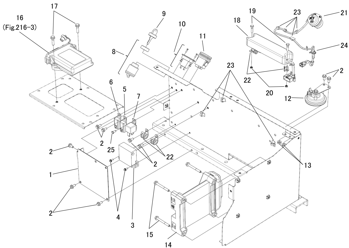
FIG.212 電装品 ELECTRIC PARTS
