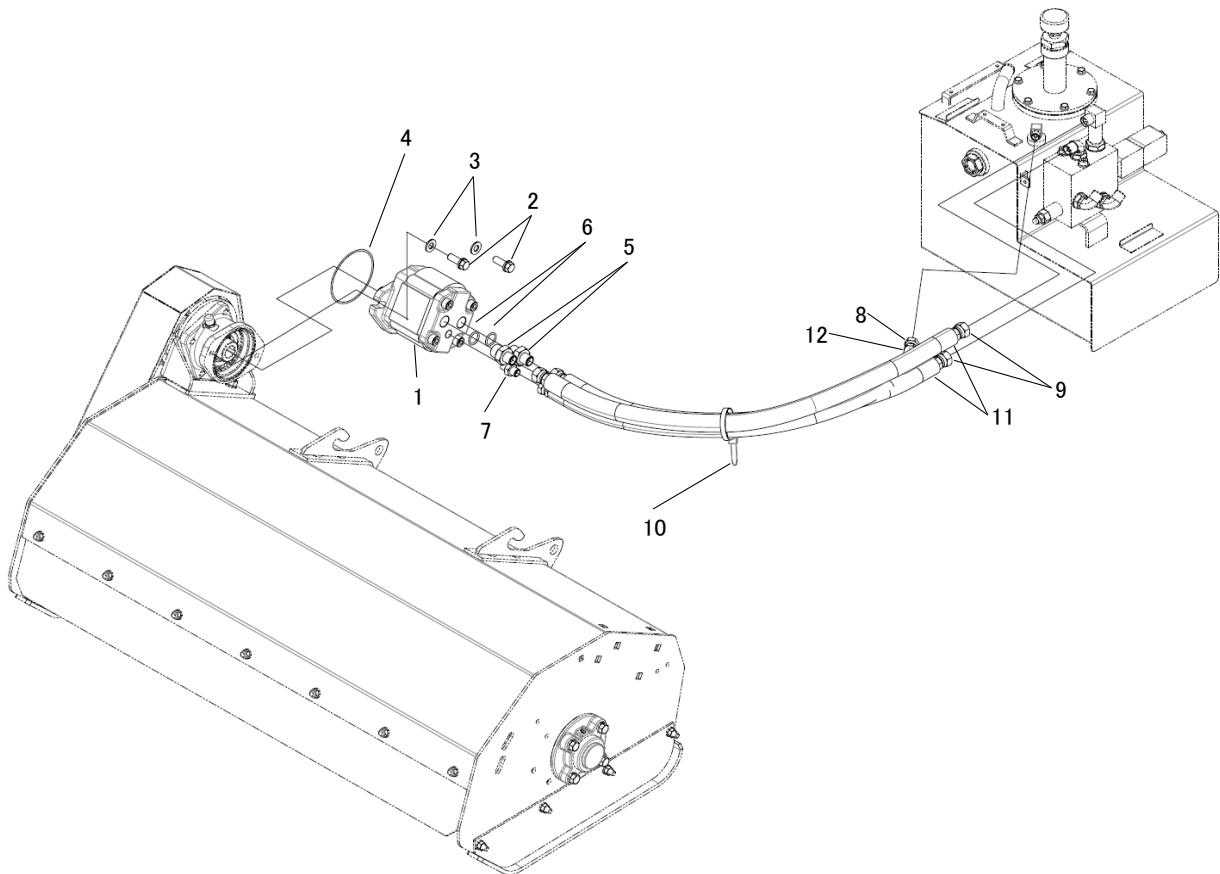
FIG.304 モア;油圧モーター MOWER;HYDRO MOTOR
