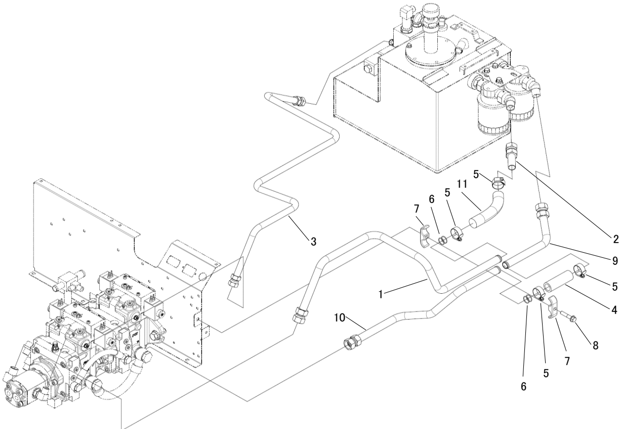
FIG.204 HSTポンプ配管
