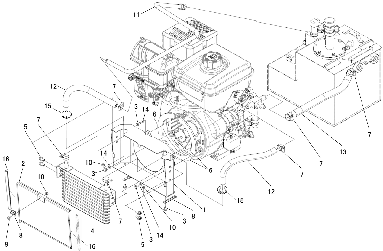
FIG.206 オイルクーラー OIL COOLER
