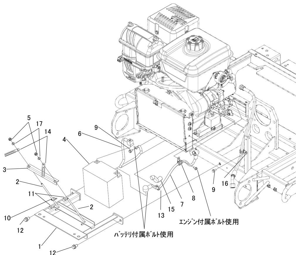
FIG.211 バッテリ台 & バッテリ BATTERY STAND & BATTERY
