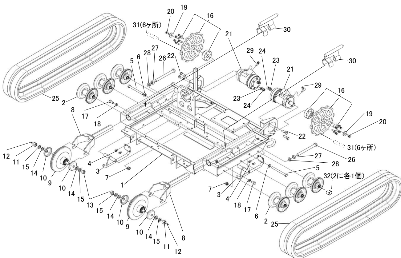
FIG.201 フレーム & モーター & クローラ LOWER FRAME & MOTOR & CRAWLER
