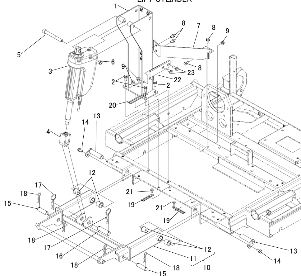
FIG.209 リフトシリンダ LIFT CYLINDER
