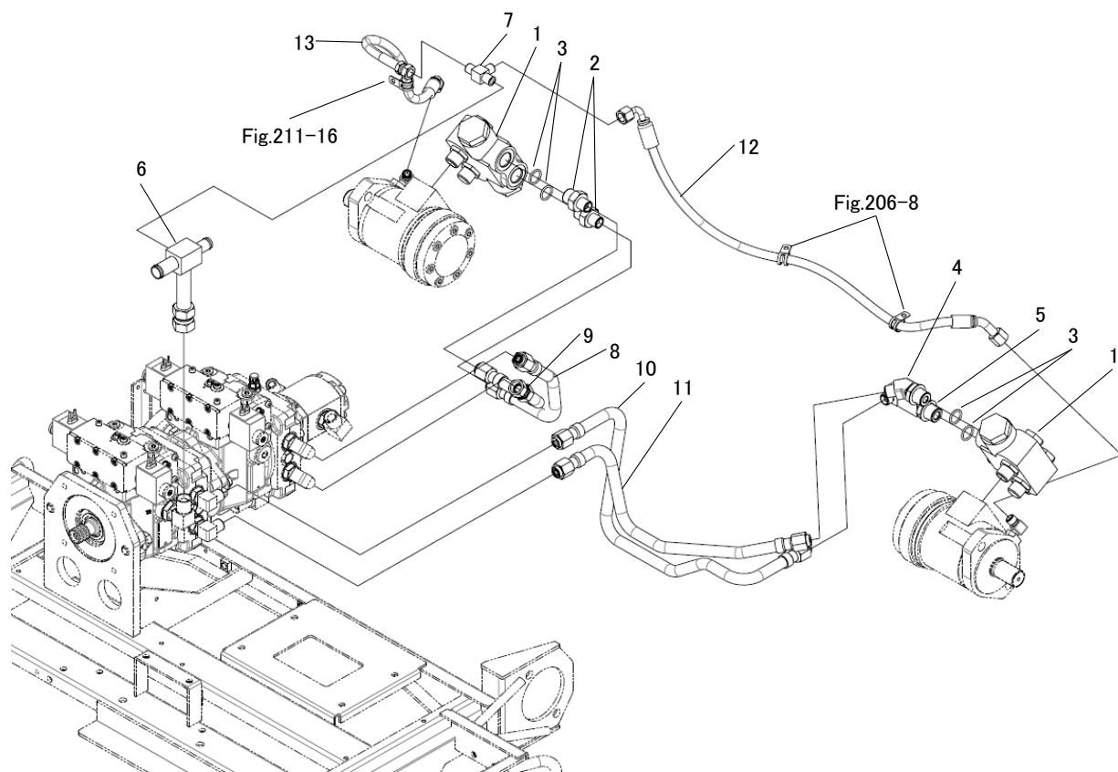
FIG.203 走行モータ配管 MOTOR OIL PIPE
