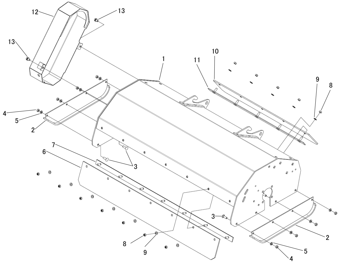
FIG.301 モア;カバー MOWER;COVER
