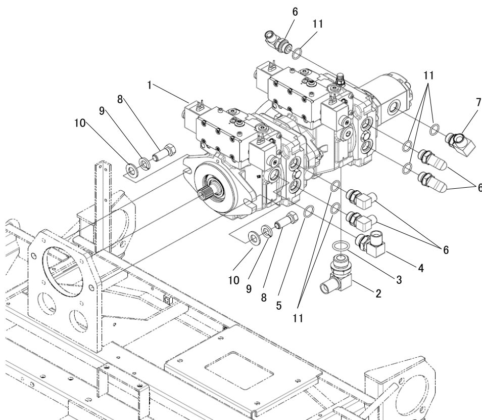
FIG.202 HST & アダプタ HST & ADAPTER
