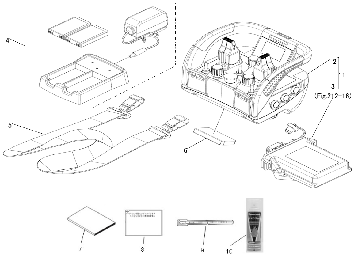
FIG.216 送受信機 & アクセサリー TRANSMITTER/RECEIVER & ACCESSARY
