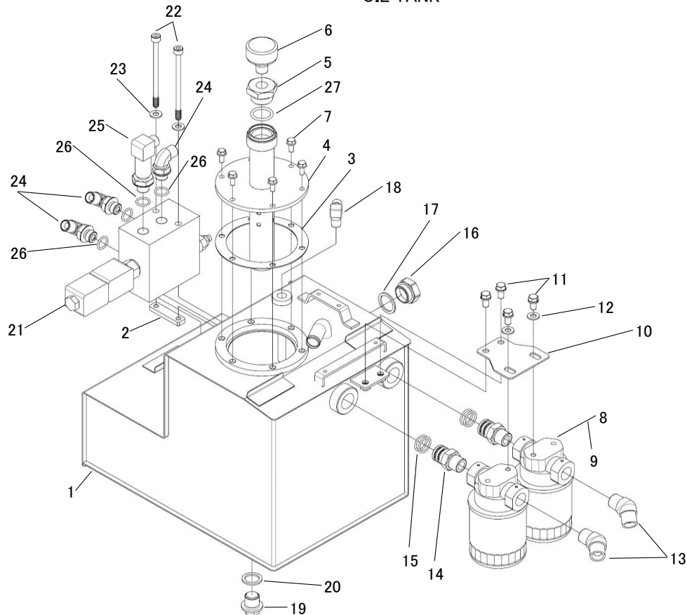
FIG.208 オイルタンク OIL TANK
