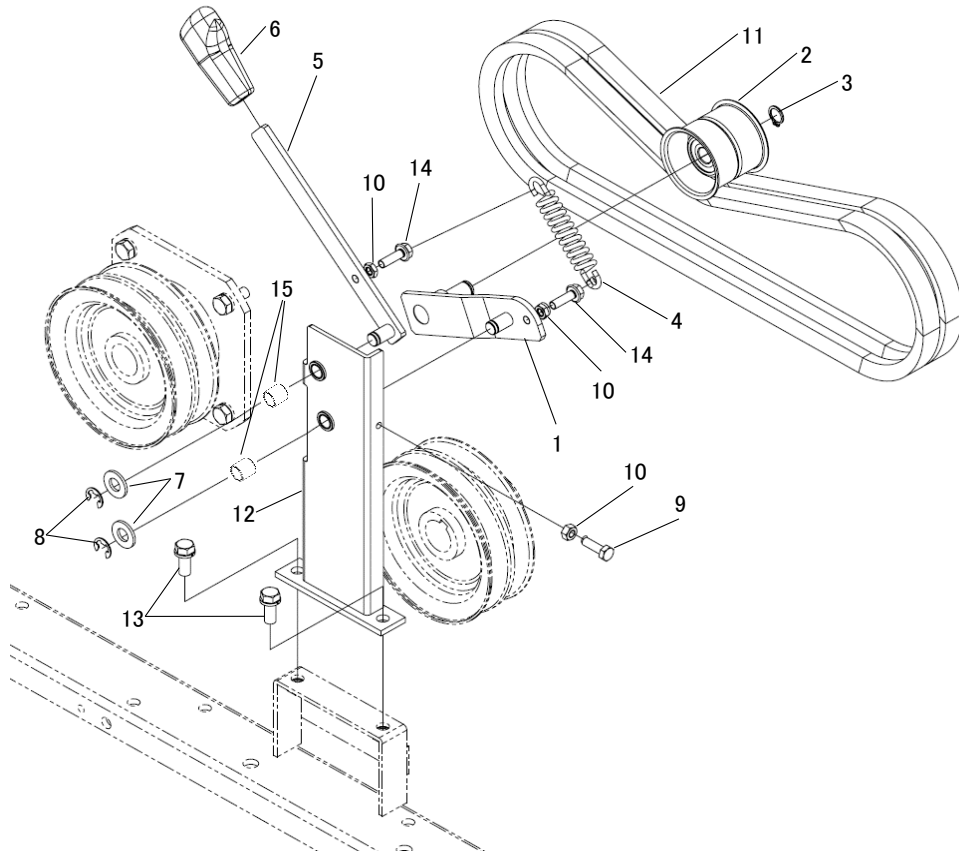
FIG.207 動力クラッチ CLUTCH
