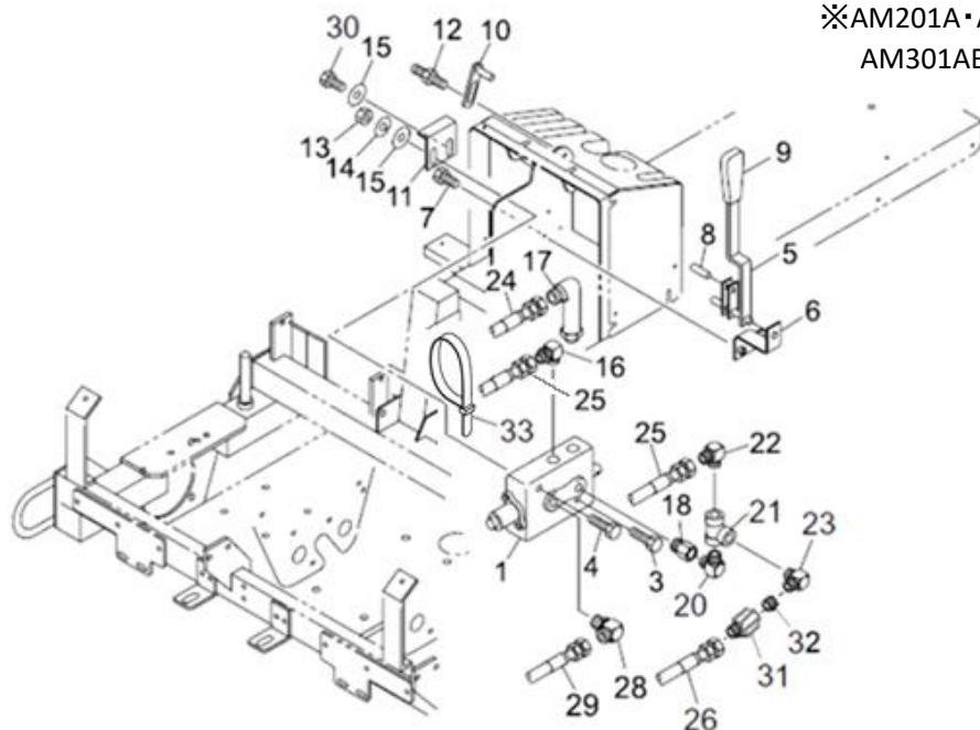
FIG.21(2) ショウコバルブ UP/DOWN VALVE
