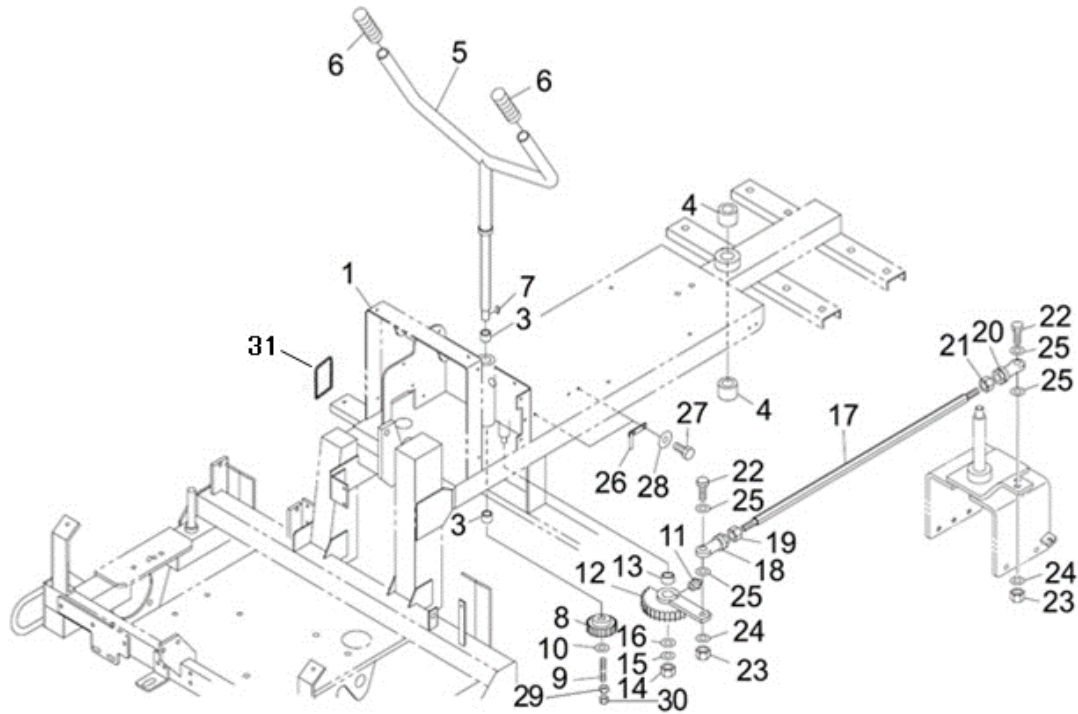
FIG.3 ステアリング STEERING
