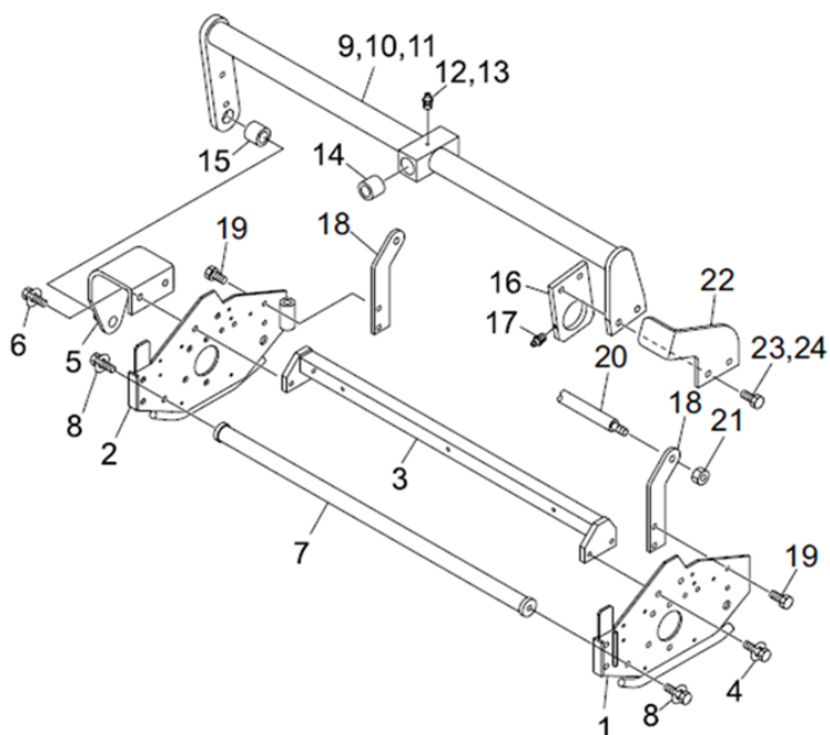
FIG.103 カッターフレーム CUTTER FRAME
