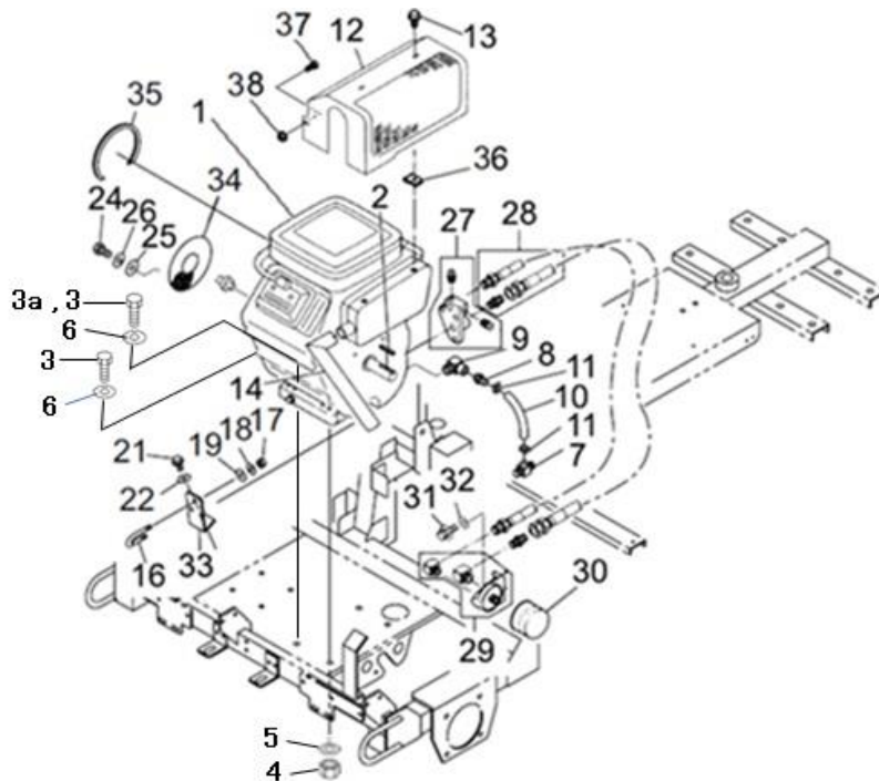
FIG.1 エンジン ENGINE
