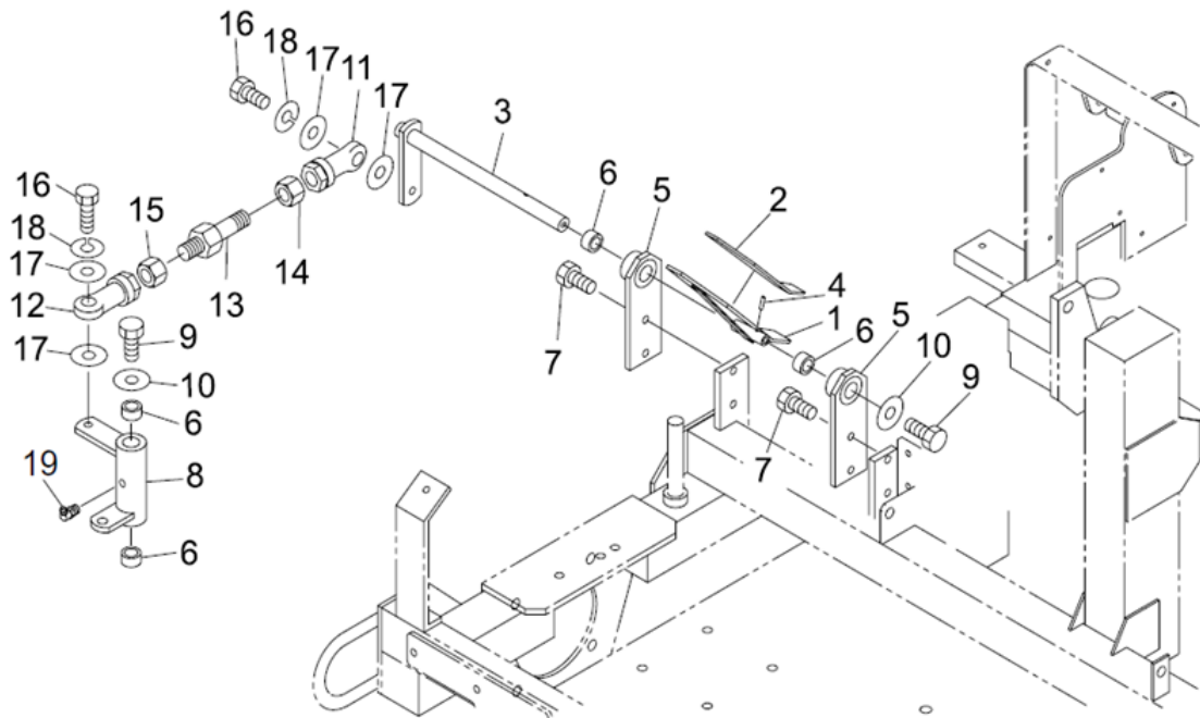
FIG.13 ペダル PEDAL
