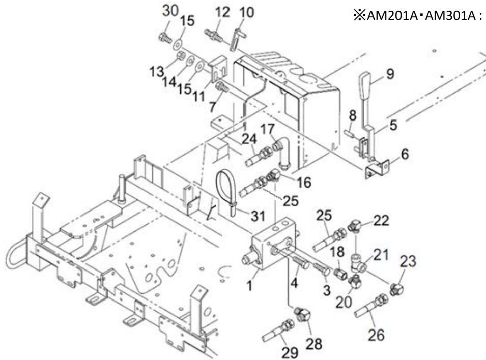
FIG.21(1) ショウコウバルブ UP/DOWN VALVE
