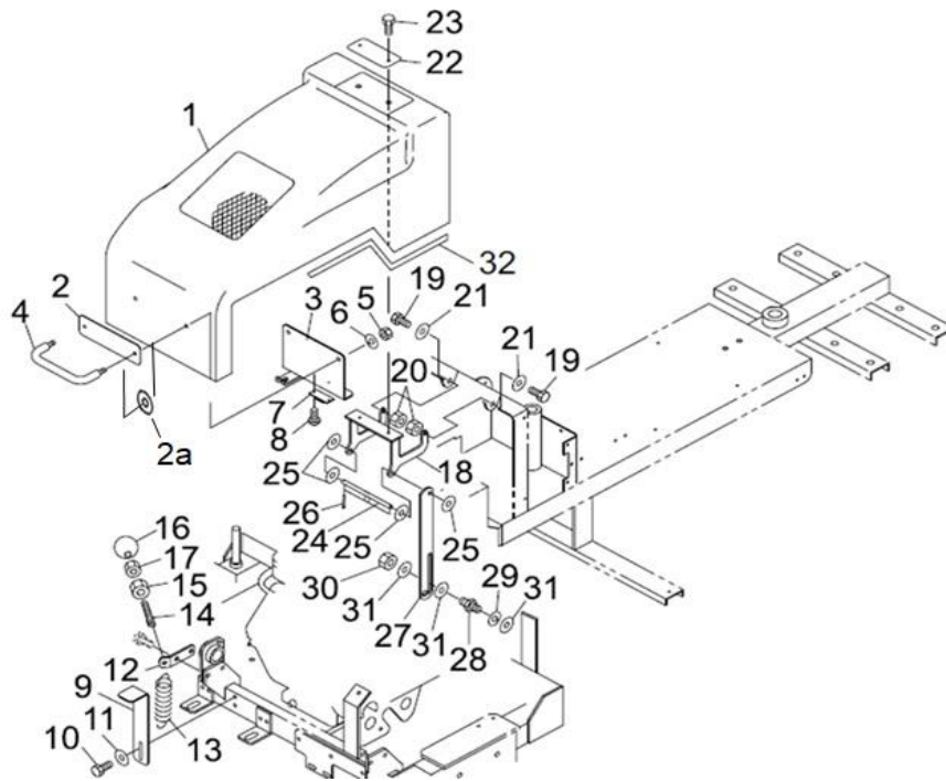
FIG.10 エンジンカバー ENGINE COVER
