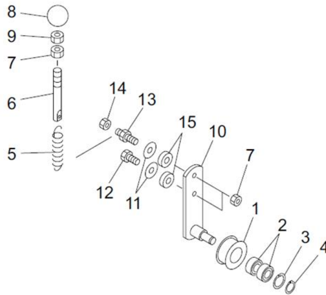
FIG.4(2) テンションアーム(2) TENSION ARM(2)
