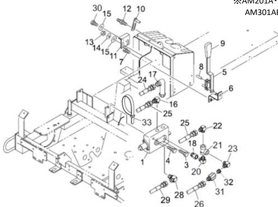
FIG.21(3) ショウコウバルブ UP/DOWN VALVE
