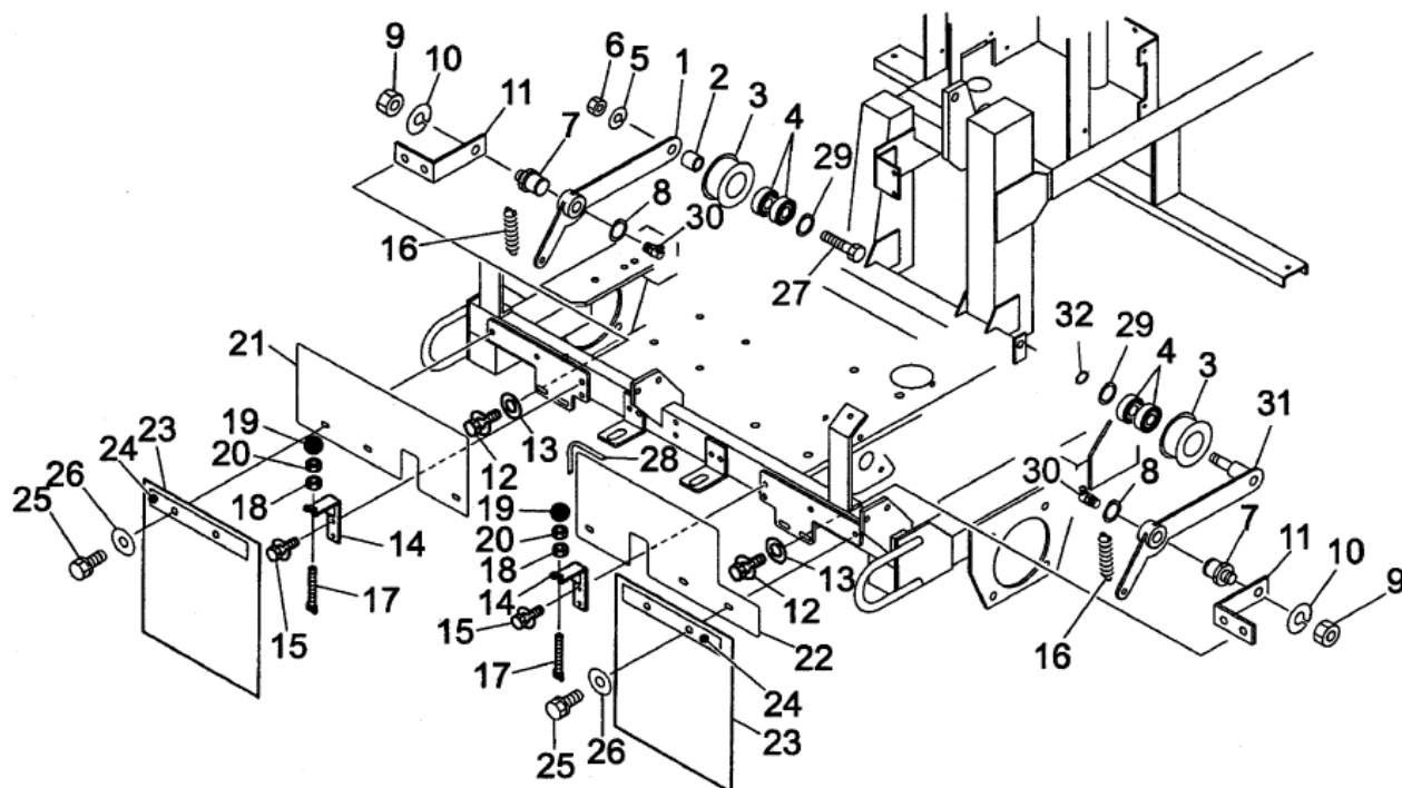
FIG.4(1) テンションアーム(1) TENSION ARM(1)
