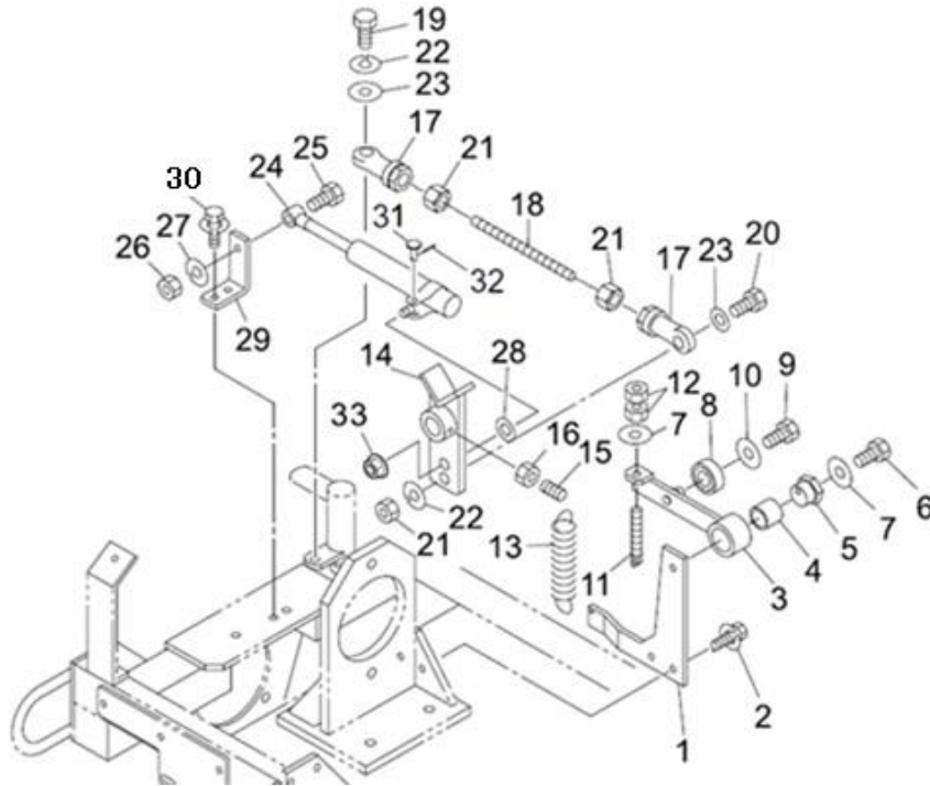
FIG.14 トラニオン TRANION
