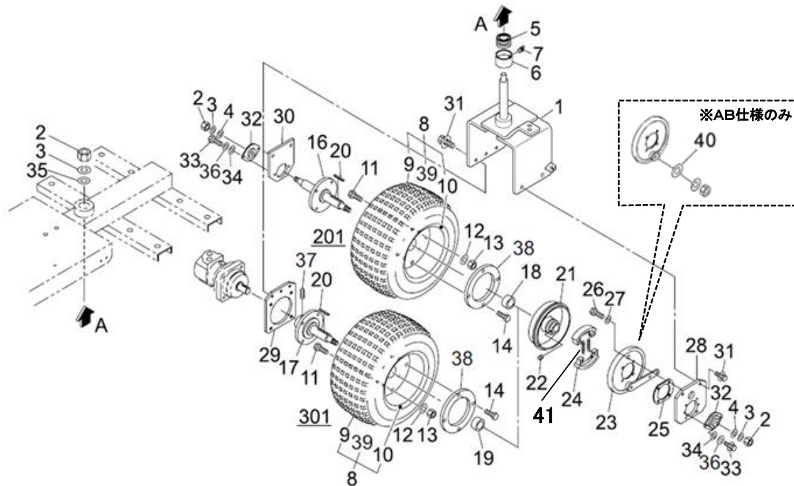
FIG.2 フォーク FORK
