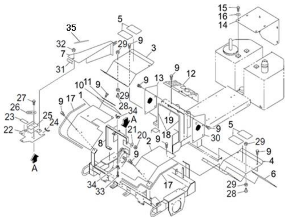
FIG.11 カバー COVER
