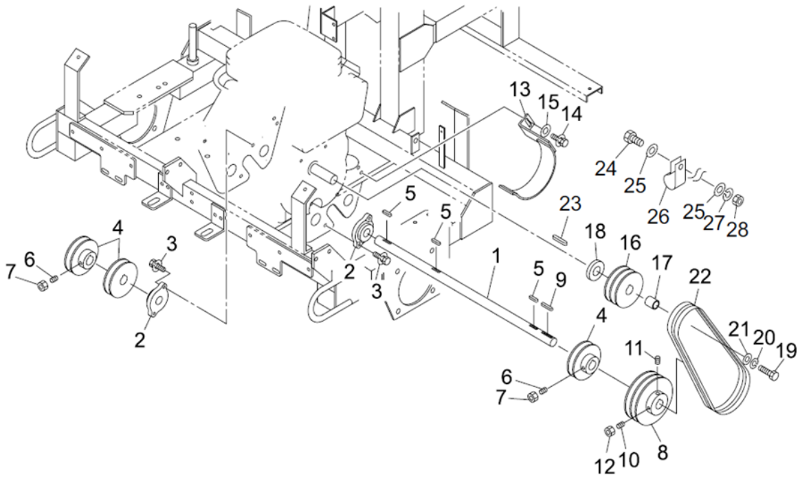
FIG.5 カッターシャフト CUTTER SHAFT
