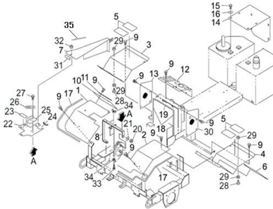
FIG.11 カバー COVER
