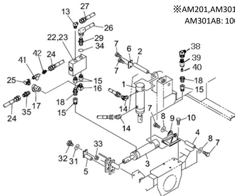
FIG.9(3) シリンダ CYLINDER
