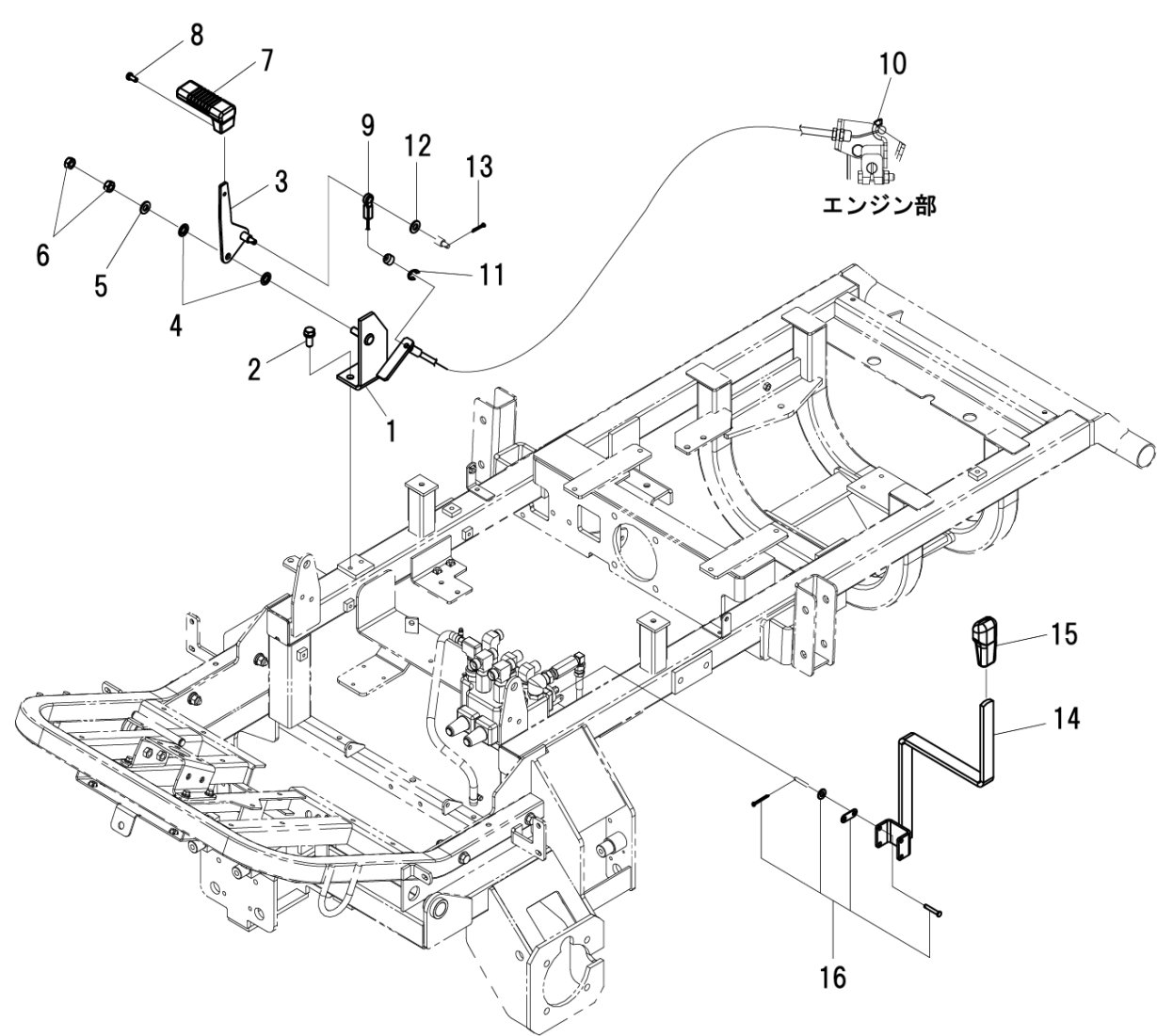
FIG.209 アクセル、2/4WD レバー ACCEL、2/4WD LEVER
