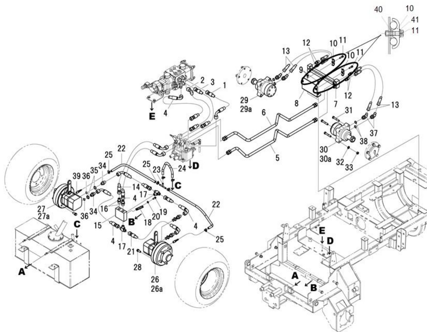
FIG.221 ユアツ ; ソウコウ HYDRAULIC ; DRIVE
