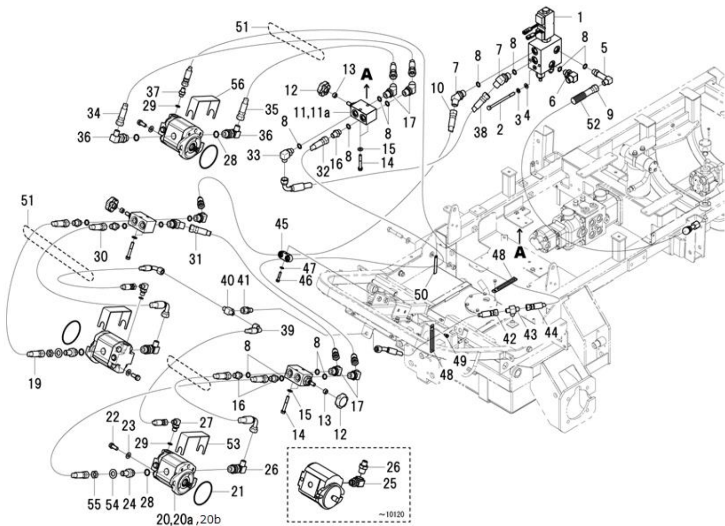
FIG.224 ユアツ ; リール HYDRAULIC ; REEL
