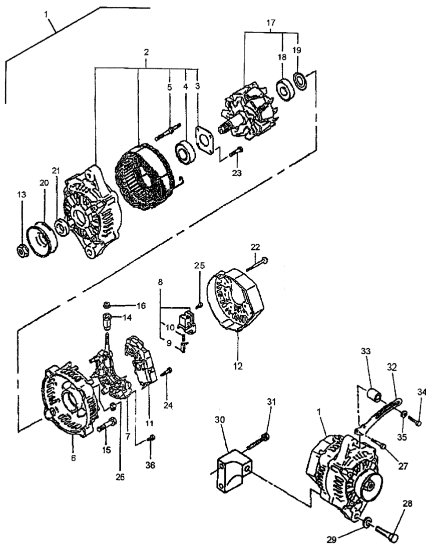
オルタネータ ALTERNATOR
