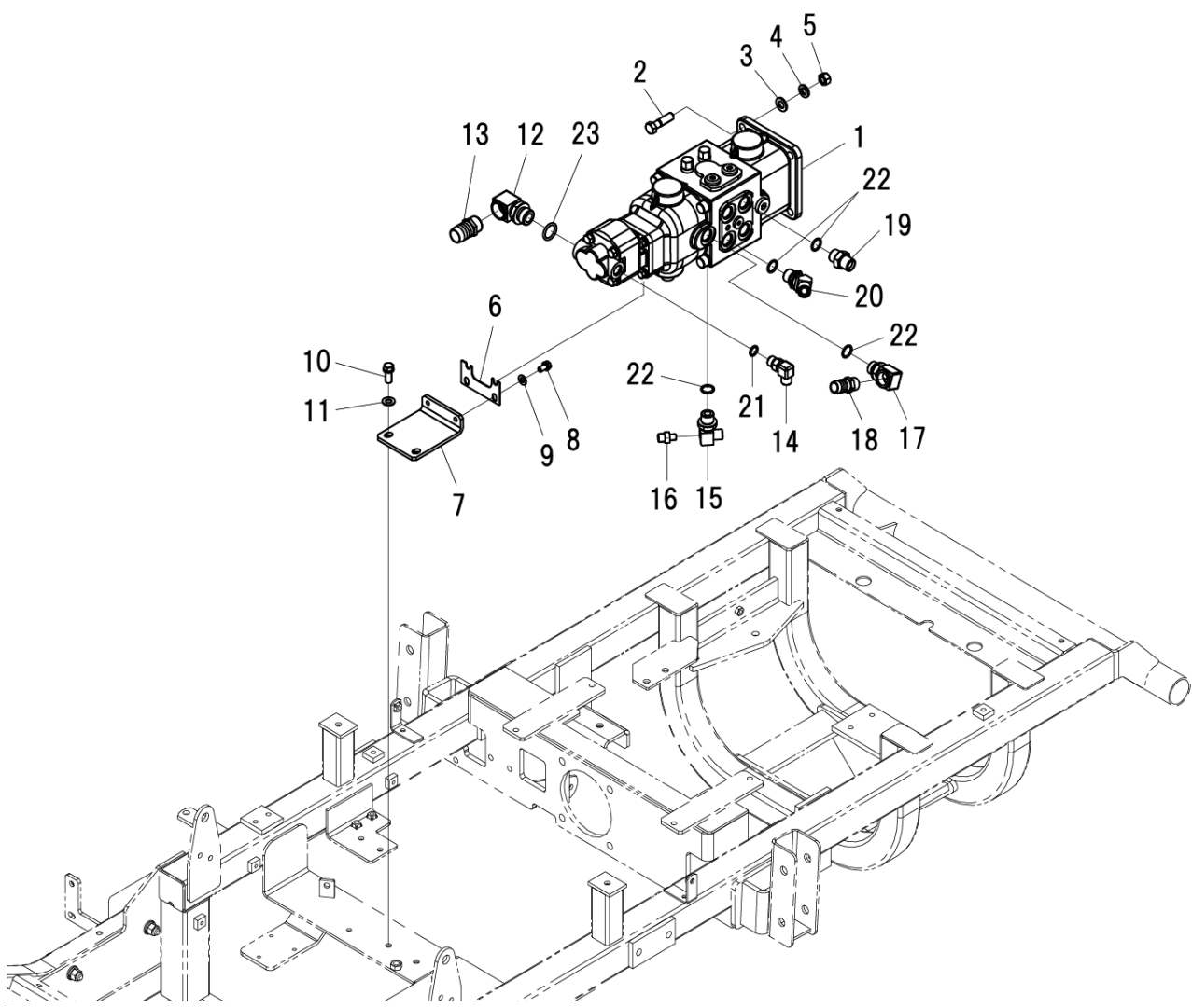
FIG.218 ユアツ ; HST HYDRAULIC ; HST
