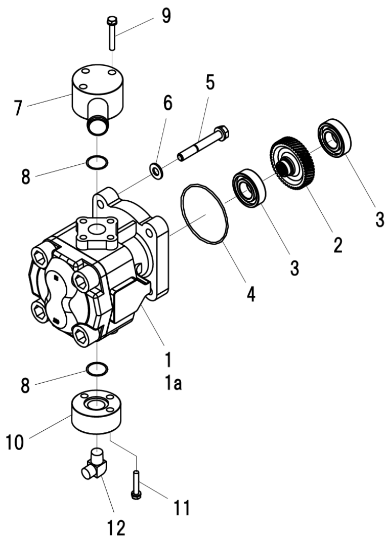
ポンプ PUMP
