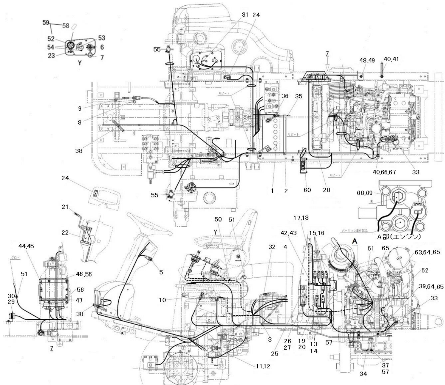
ワイヤーハーネス
