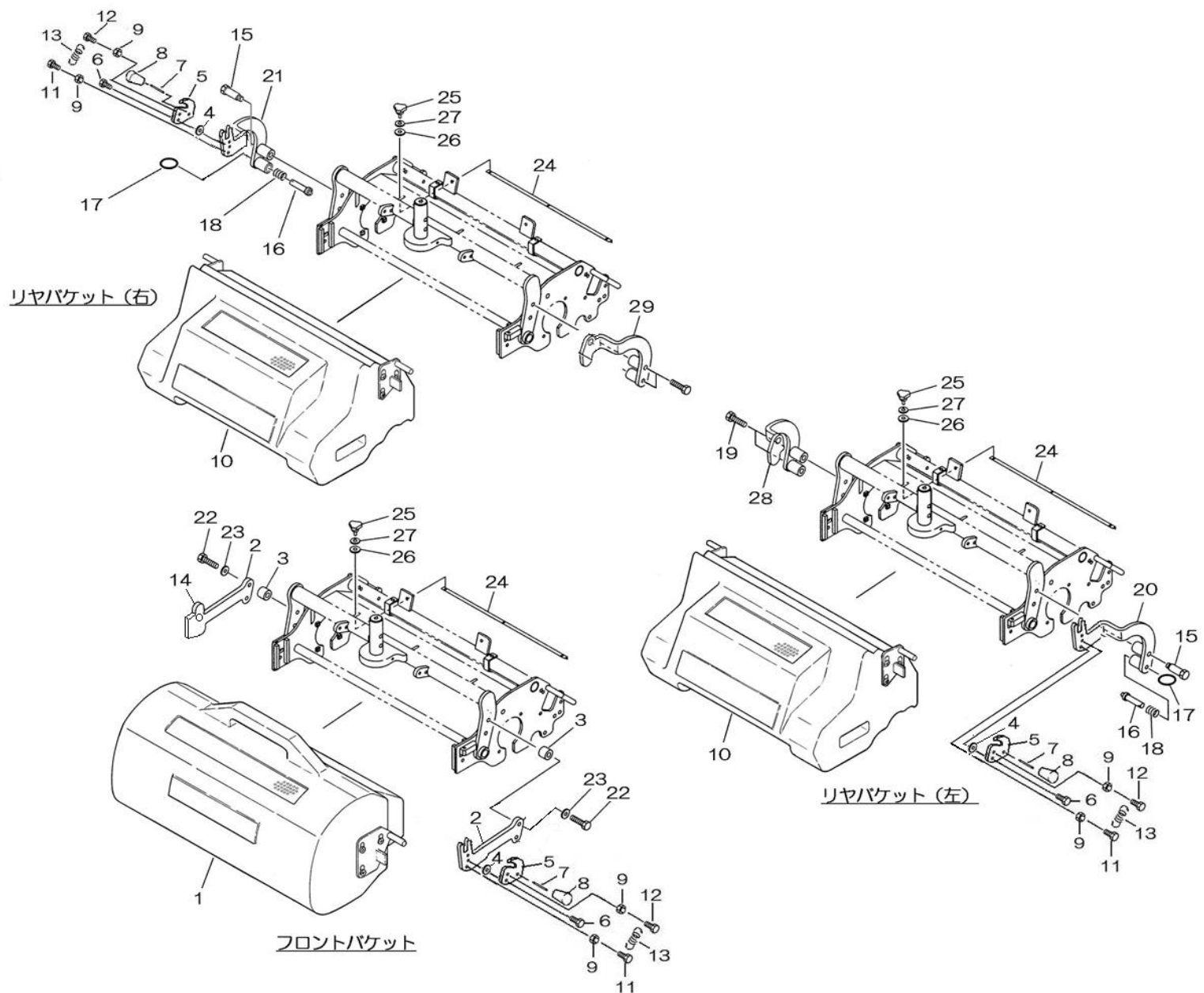
FIG.306 BUCKET ASSY 22INCH バケットASSY 22インチ
