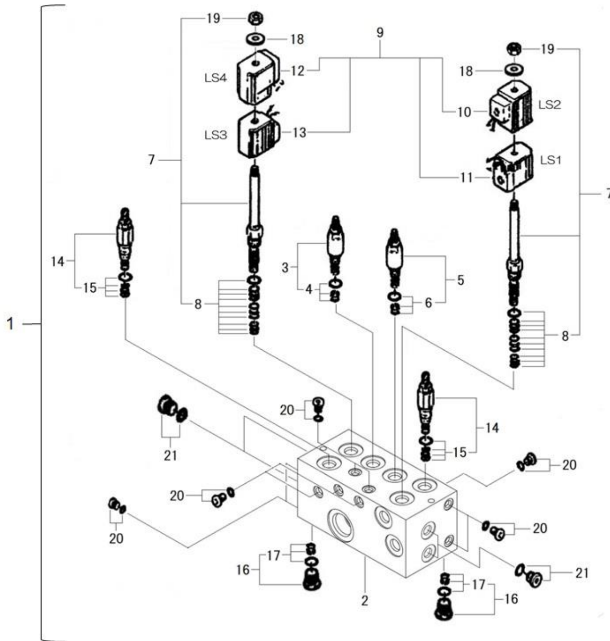
FIG.234 CONTROL VALVE (IMPLEMENT) コントロールバルブ（作業機）
