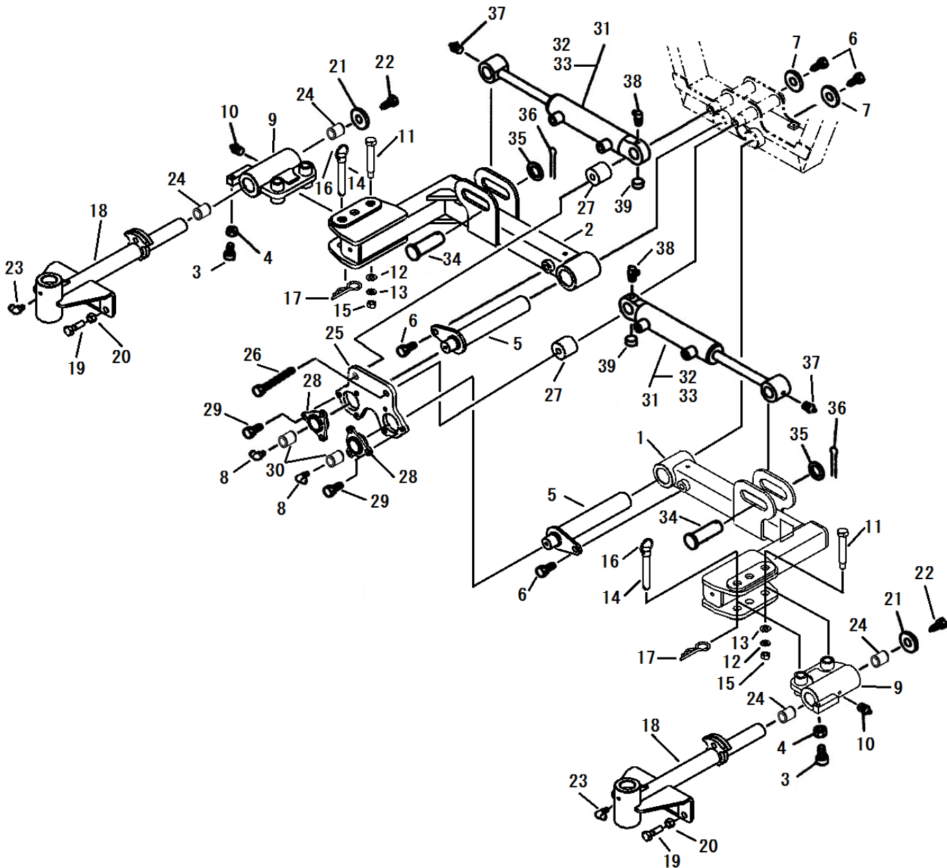
カッターアーム(リヤ) 26インチ
