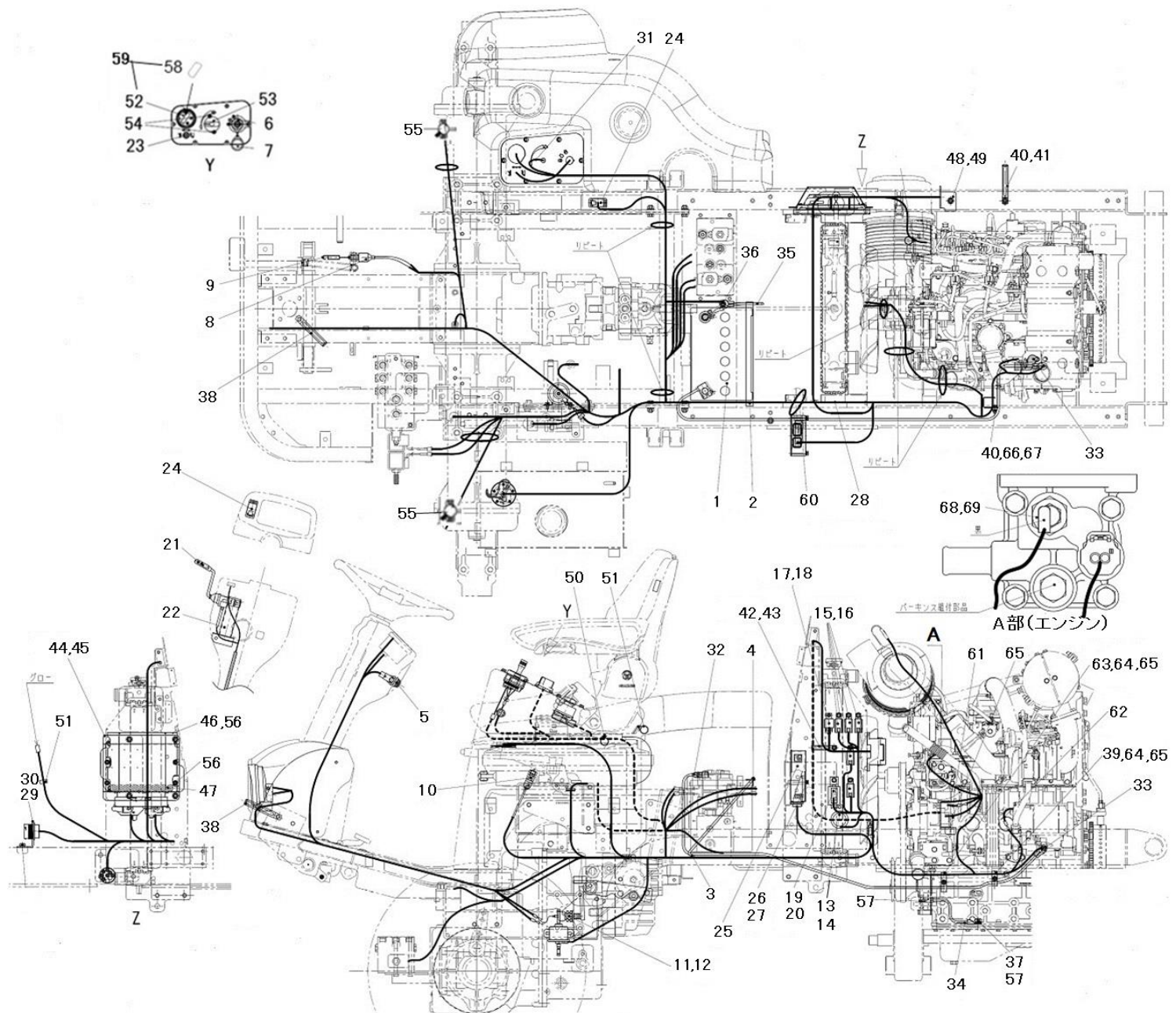
FIG.242 WIRE HARNESS ワイヤーハーネス
