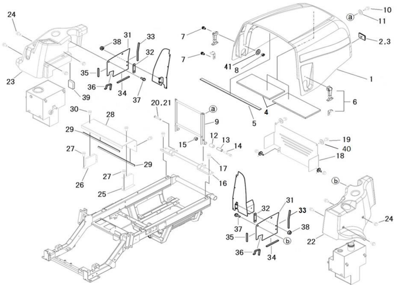
ボンネット, フェンダ
