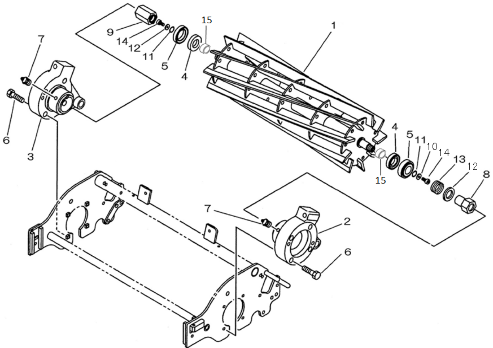
FIG.302 REEL BLADE 22INCH カイテンバ 22インチ
