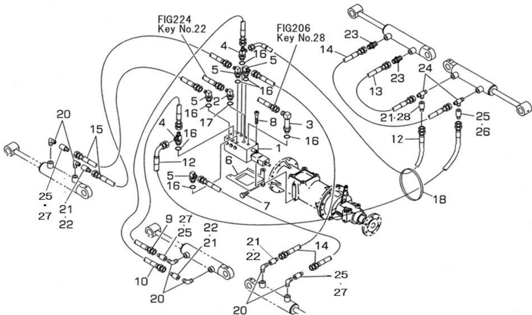
FIG.240 HYDRAULIC PIPING (LIFT) 22インチ ユアツハイカン(リフト) 22インチ
