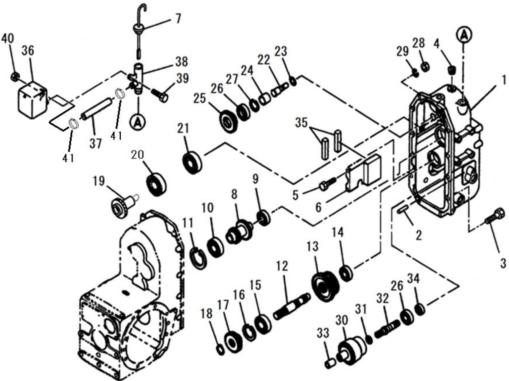
FIG.204 TRANSMISSION,DRIVE トランスミッション;走行
