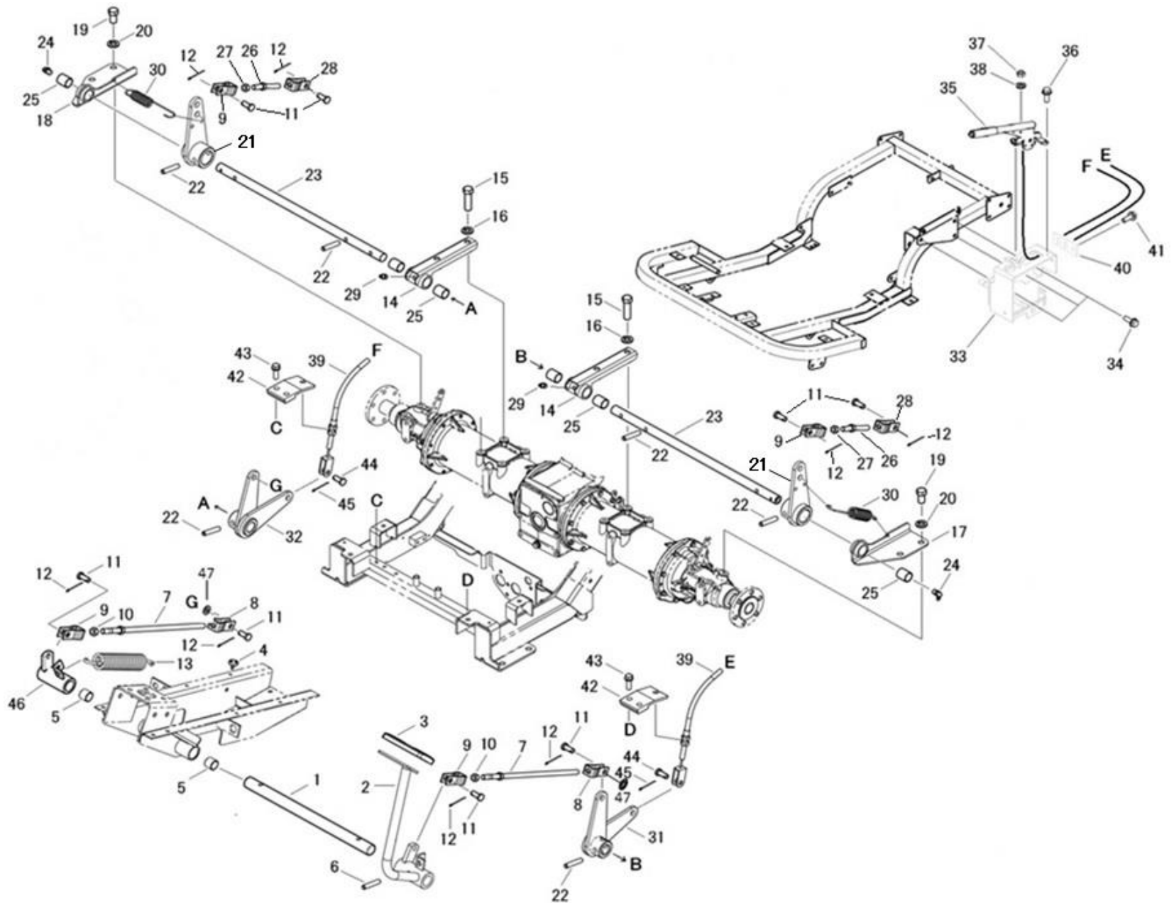
FIG.230 BRAKE PEDALS ブレーキペダル
