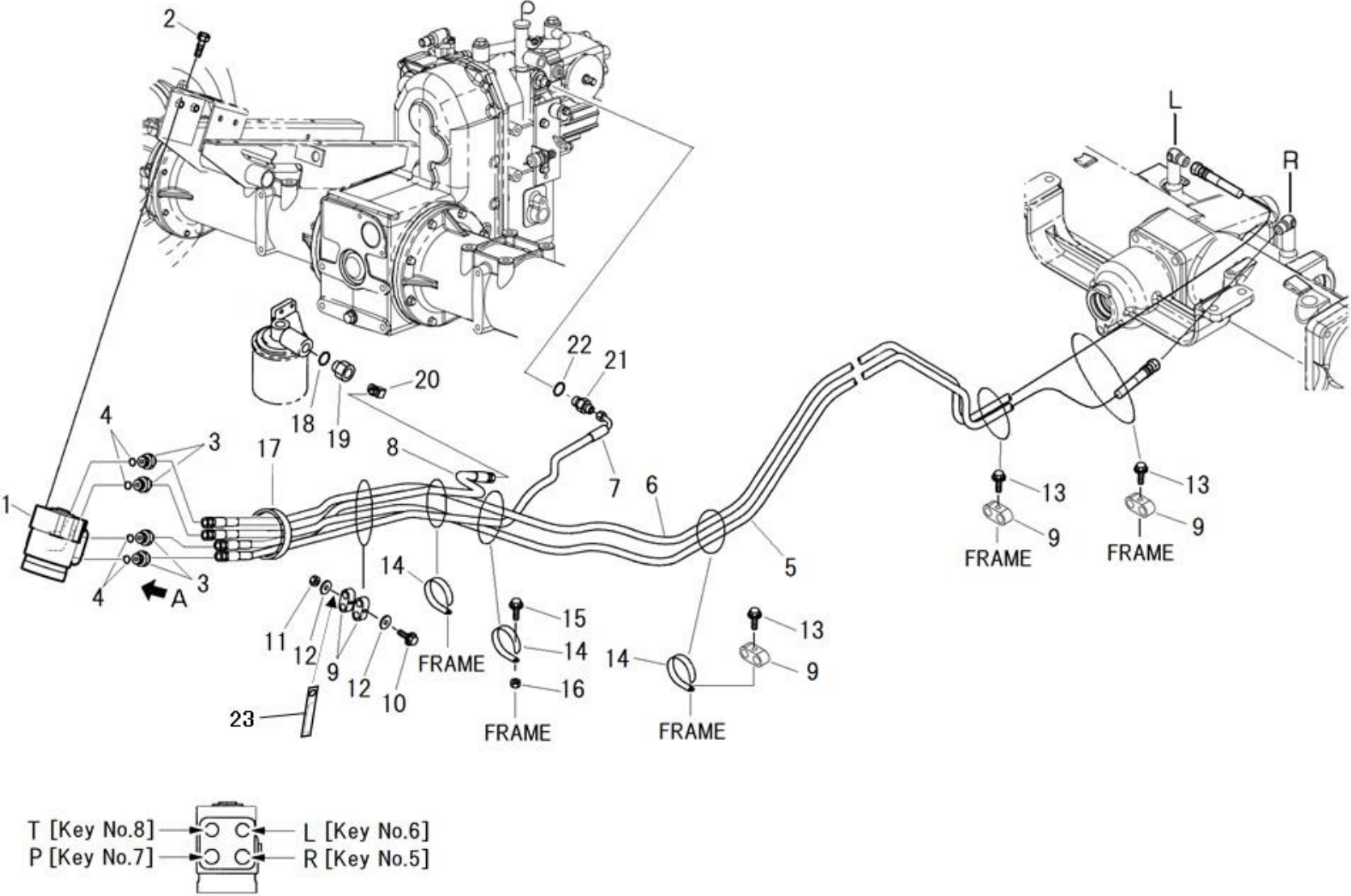
FIG.222 STEERING CASE, HYDRAULICS ステアリングケース
