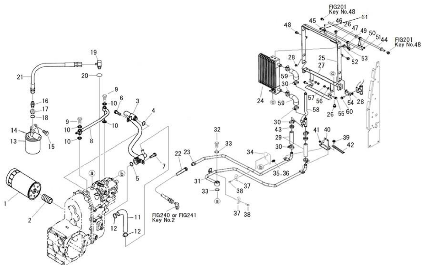
FIG.224 FILTER, HYDRAULICS フィルター
