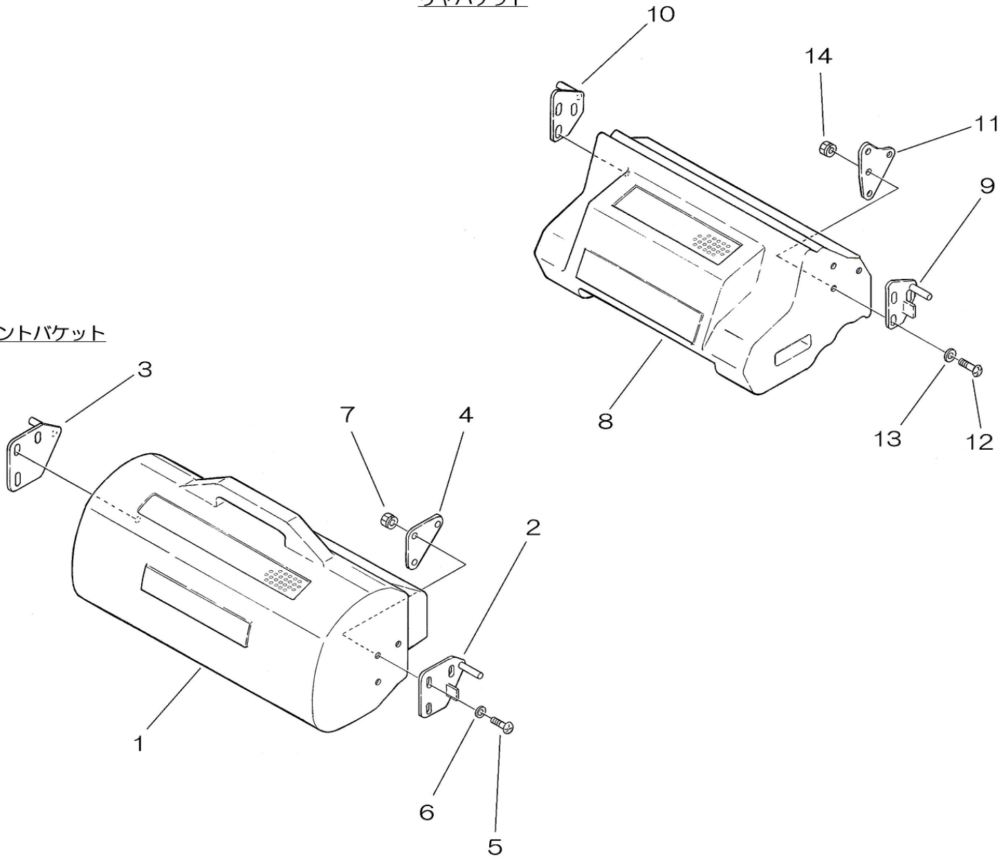
FIG.307 BUCKET 22INCH バケット 22インチ
