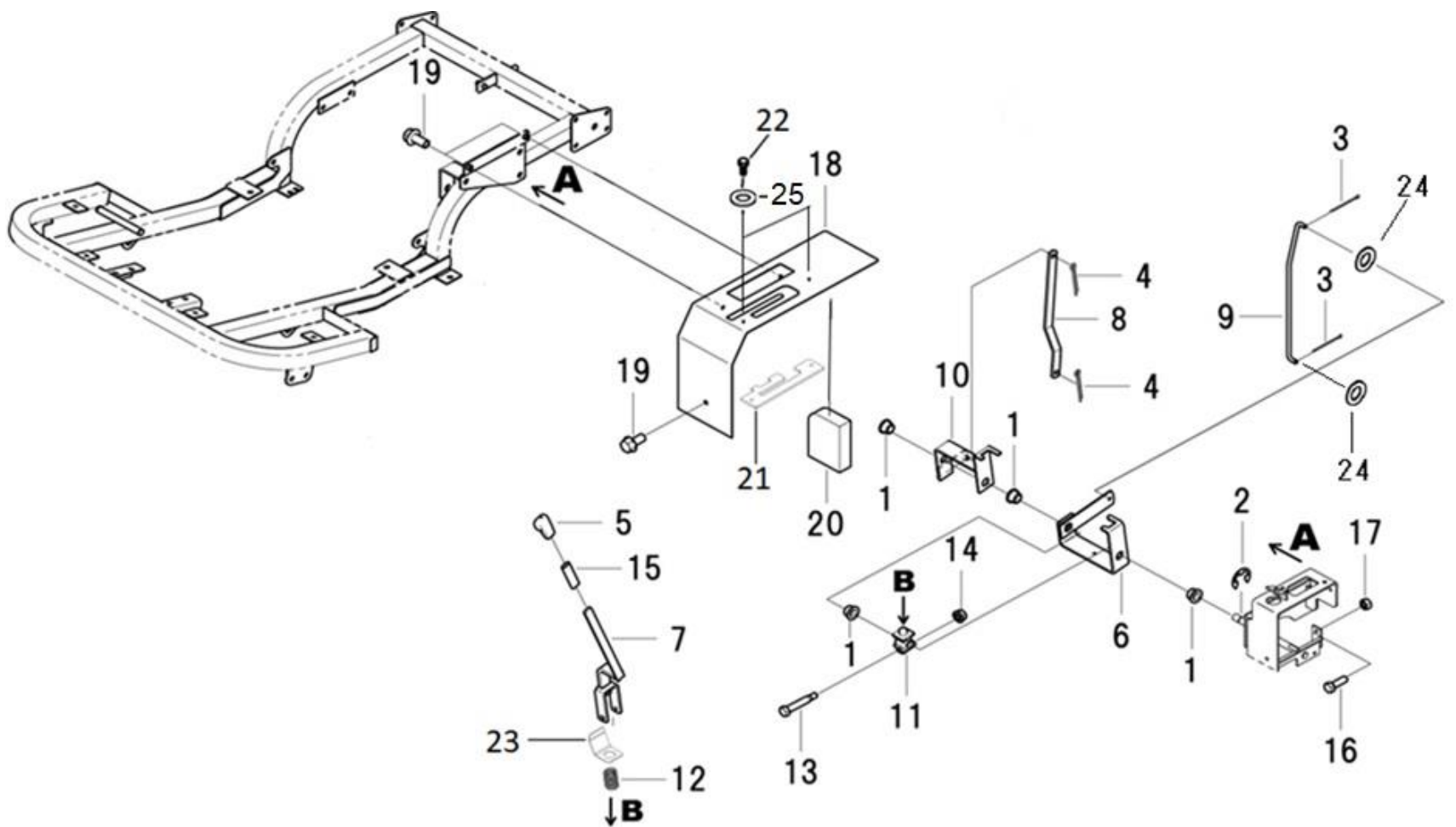
FIG.214 CHANGE LEVER シフター
