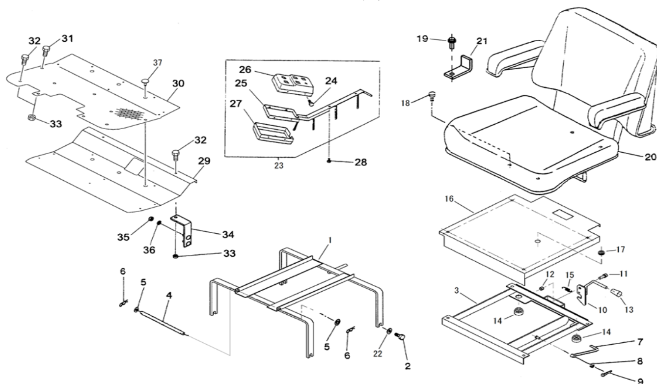
SEAT & STEP シート & ステップ
