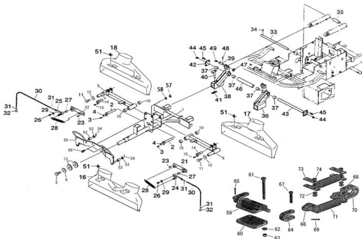
REEL MOUNT リール マウント
