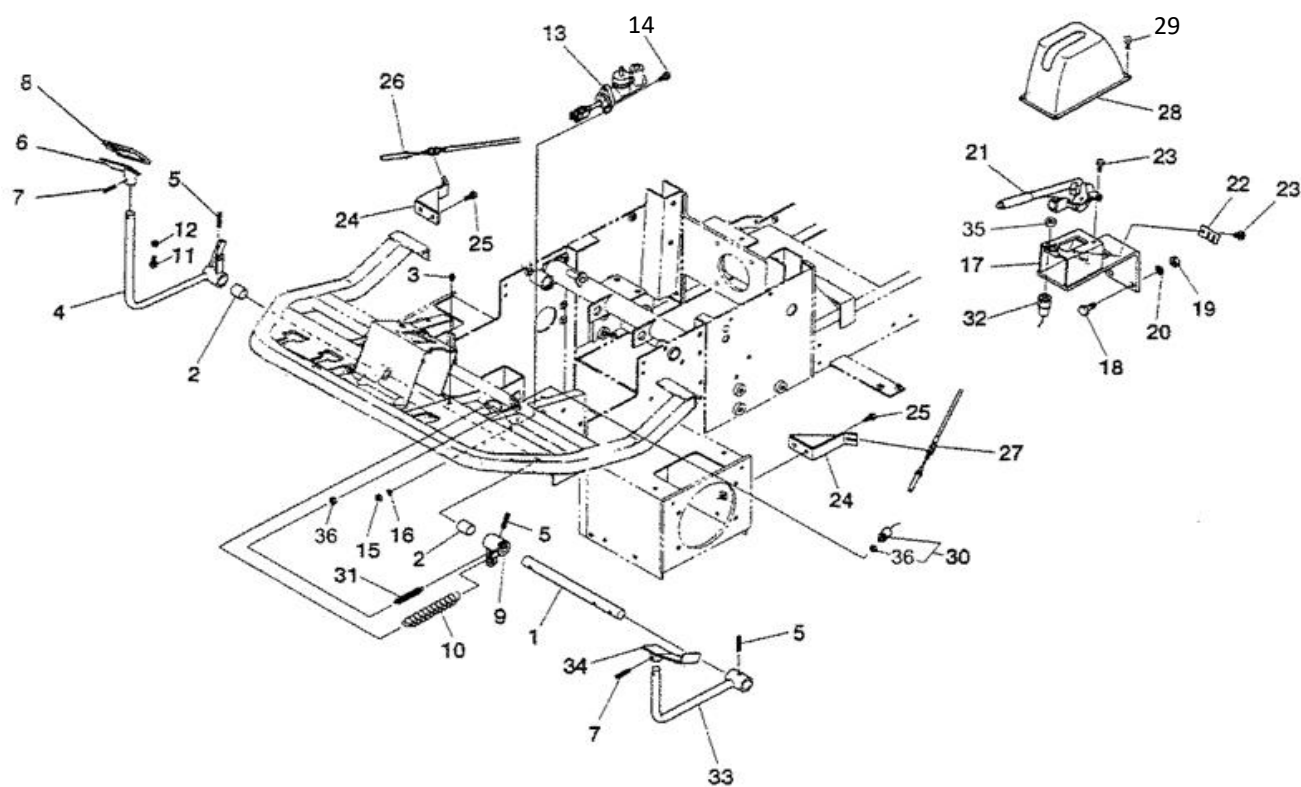
BRAKE ブレーキ
