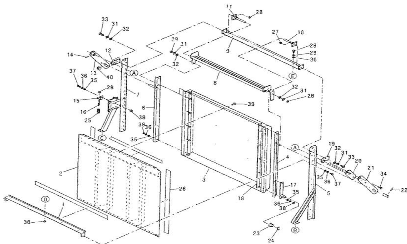
HOPPER : - 2 ホッパー : - 2
