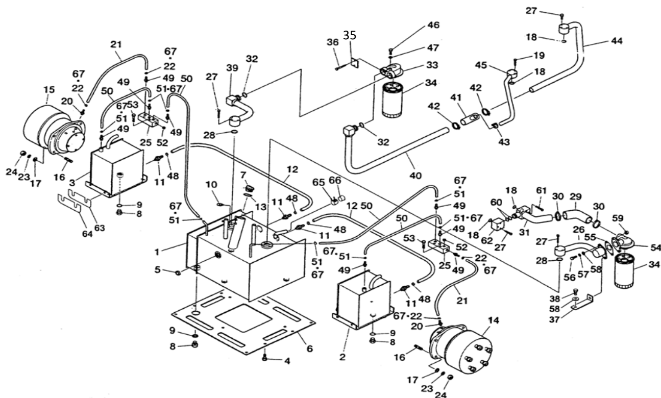
OIL TANK オイル タンク
