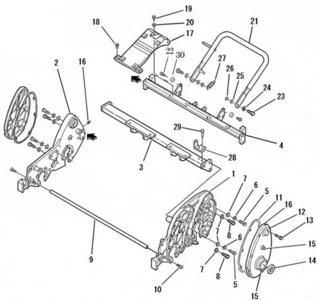
FIG. 201 フレーム関係 FRAME
