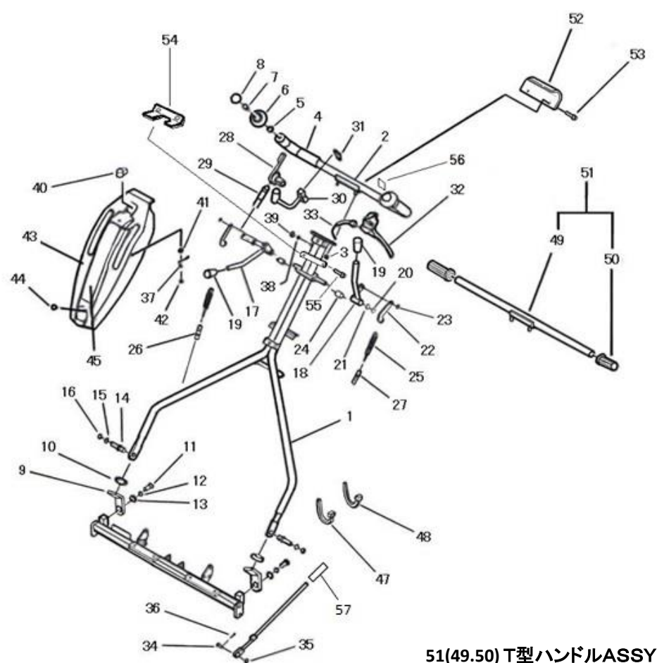
FIG. 212 ハンドル関係 HANDLE
