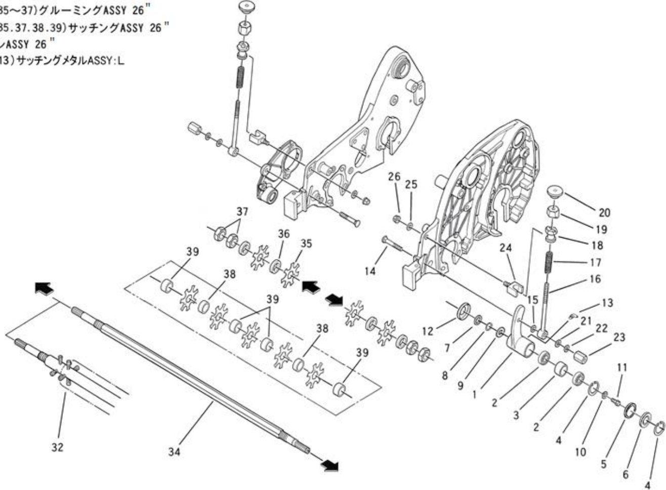
FIG. 209 グルーミングカッター関係 GROOMING CUTTER
