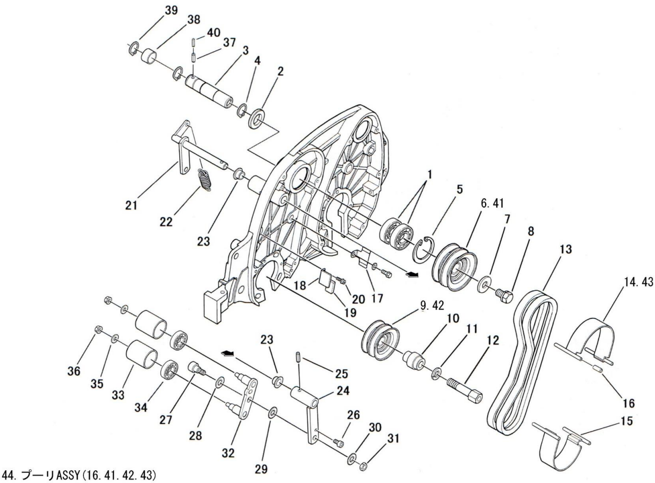
FIG. 204 テンション関係 TENSION
