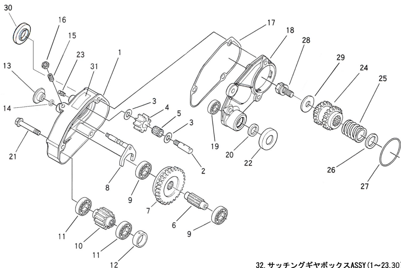
32. サッチングギヤボックスASSY(1～23.30)
