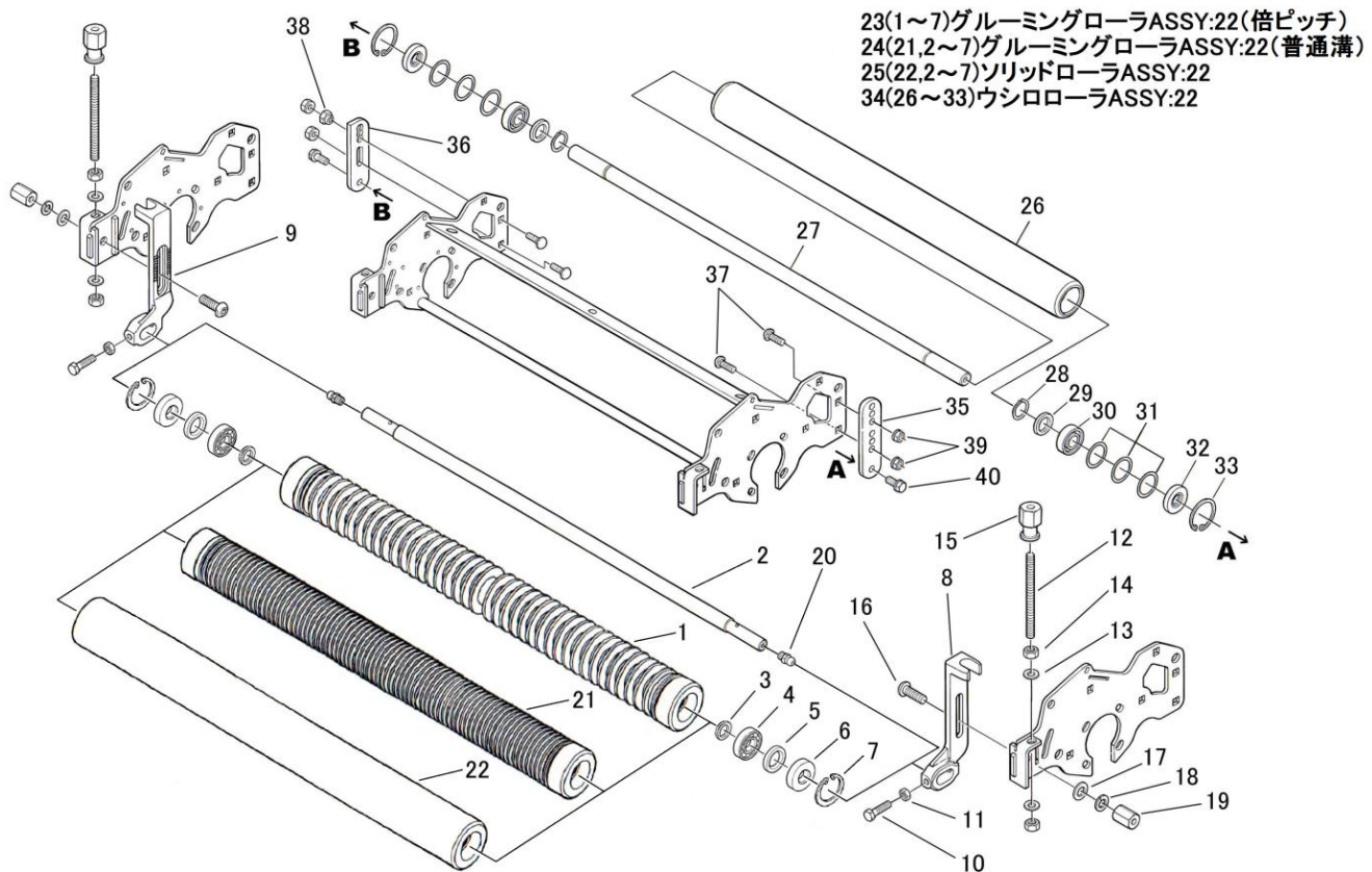
FIG. 302 前後ローラ関係 FRONT/REAR ROLLER
