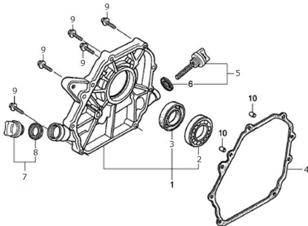
クランク ケース カバー 関係 CRANK CASE COVER
