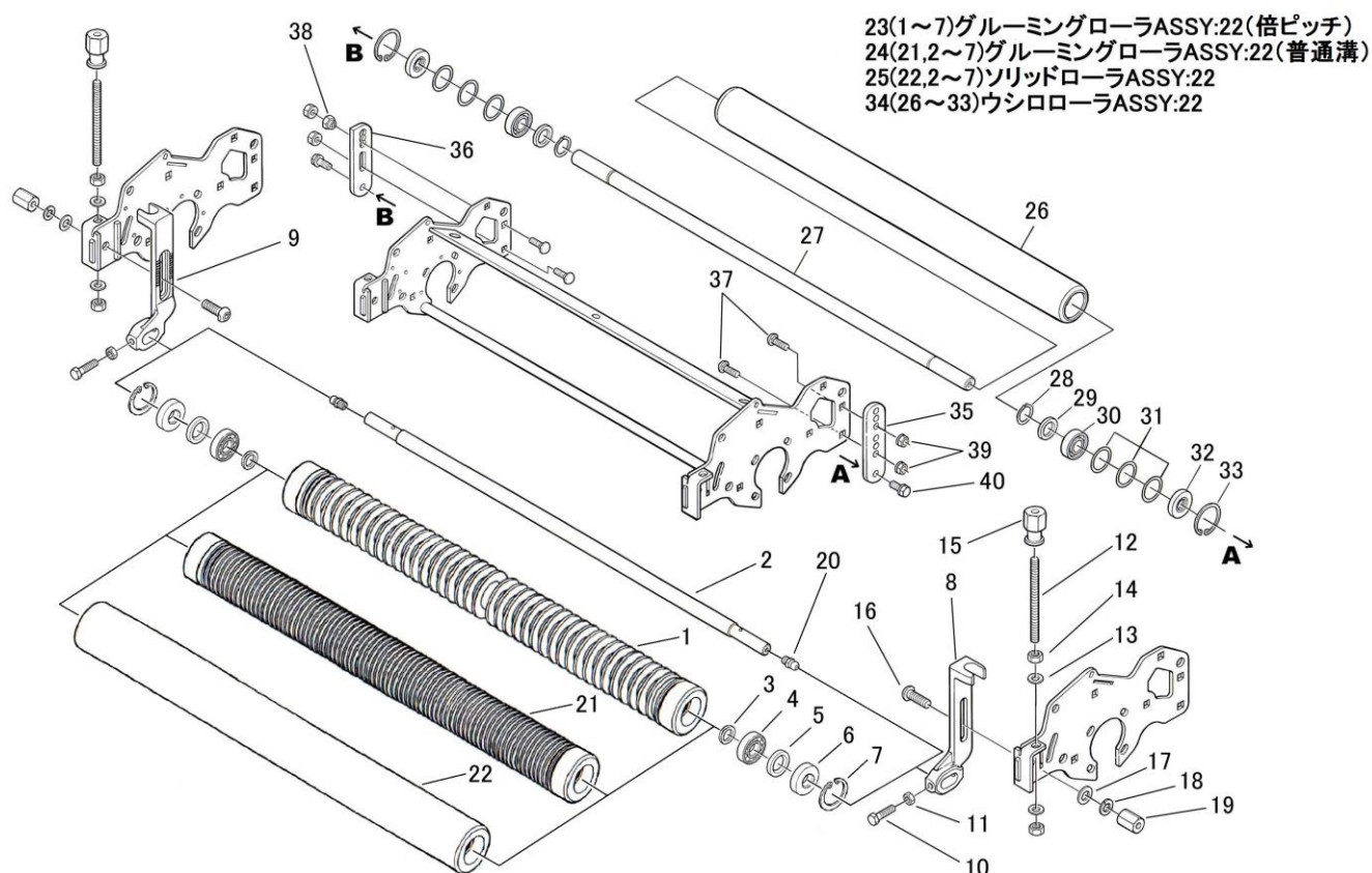
前後ローラ関係 FRONT/REAR ROLLER
