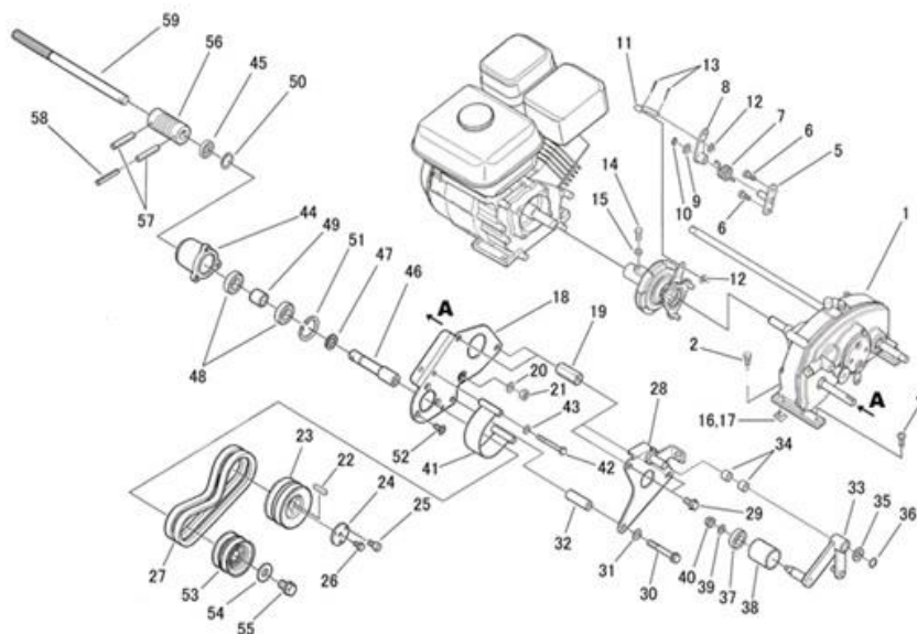
クラッチ関係 CLUTCH
