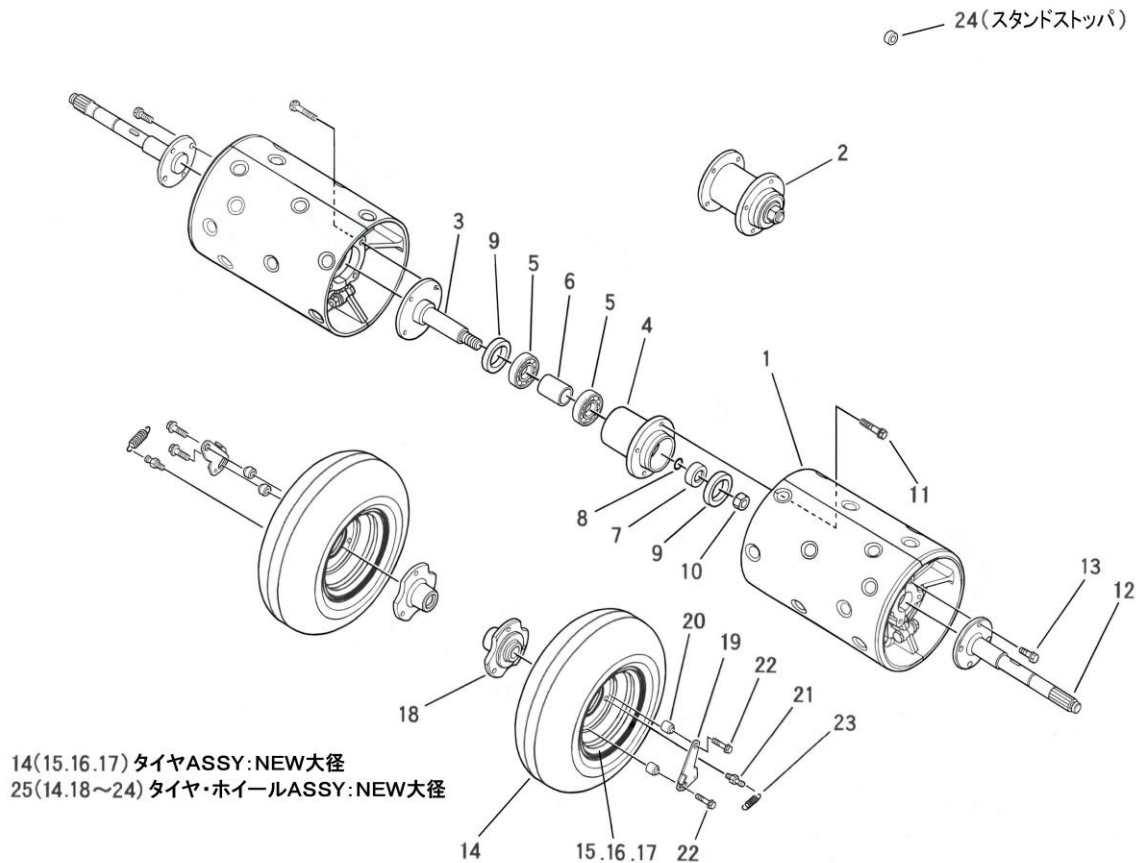
FIG. 207 後部ローラ関係 REAR ROLLER
