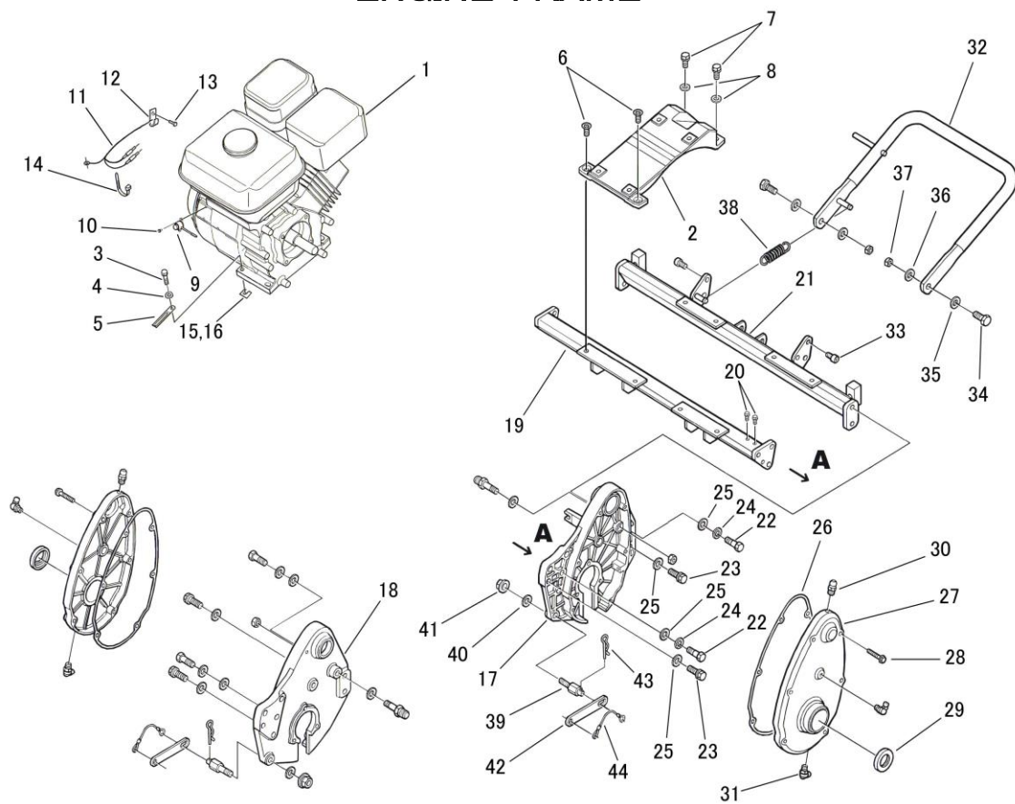
エンジン・フレーム関係 ENGINE・FRAME
