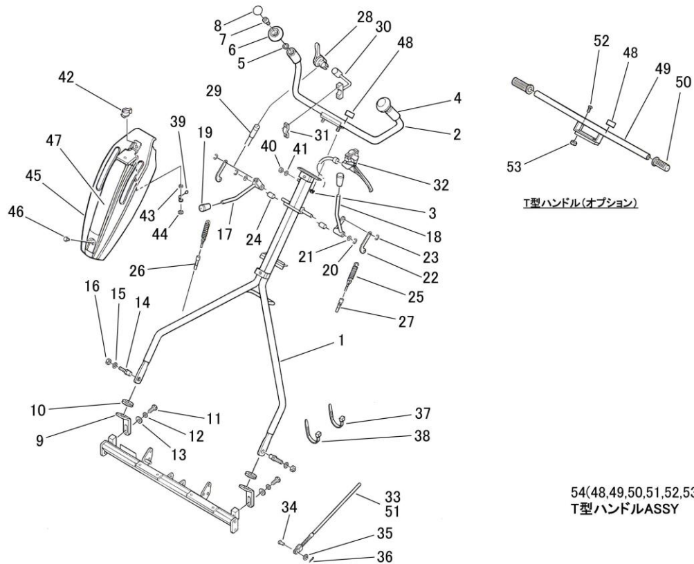
FIG. 08 ハンドル関係 HANDLE
