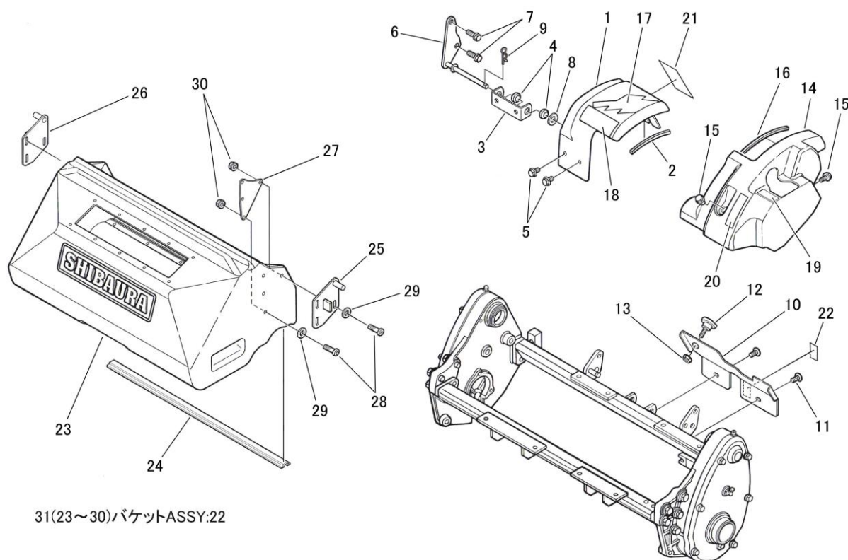
FIG. 03 カバー・バケット関係 COVER・BUCKET
