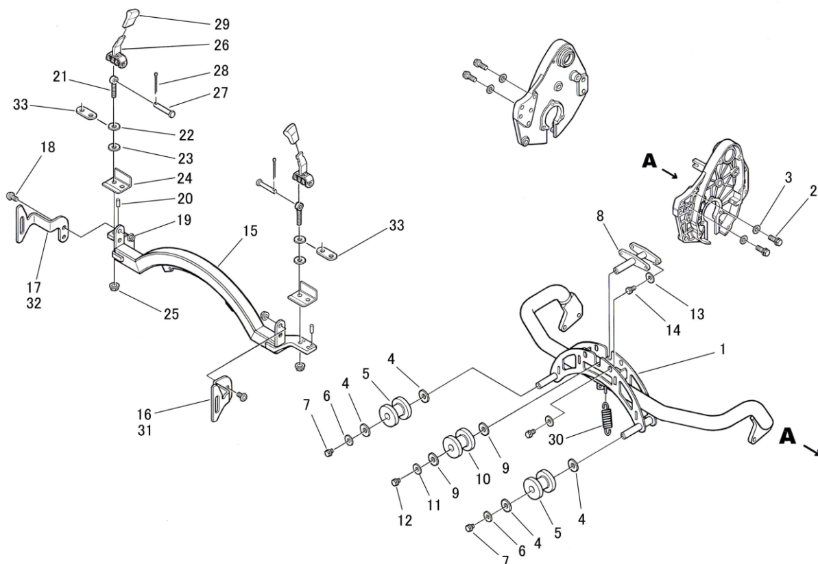
FIG. 02 アーム関係 ARM
