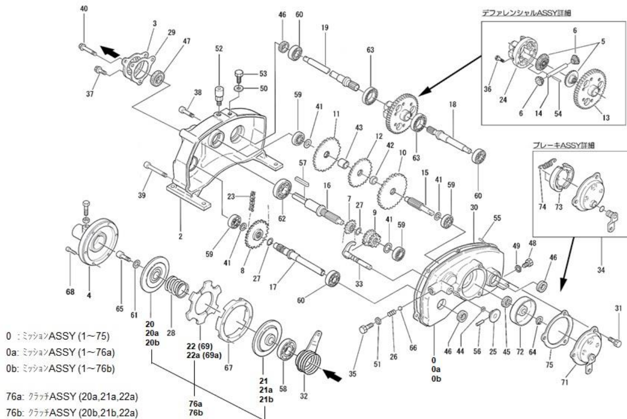
FIG. 05 ミッション関係 MISSION
