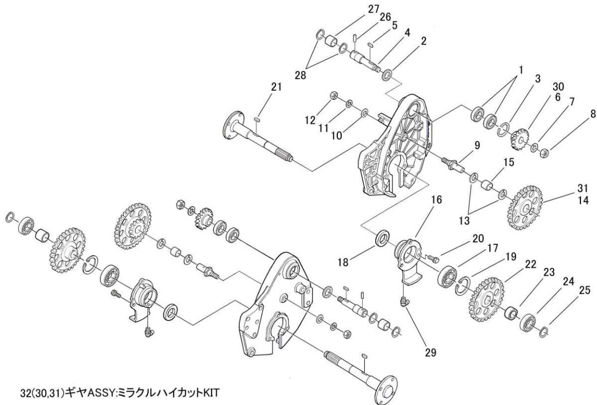
FIG. 06 ギヤ駆動関係 GEAR DRIVE
