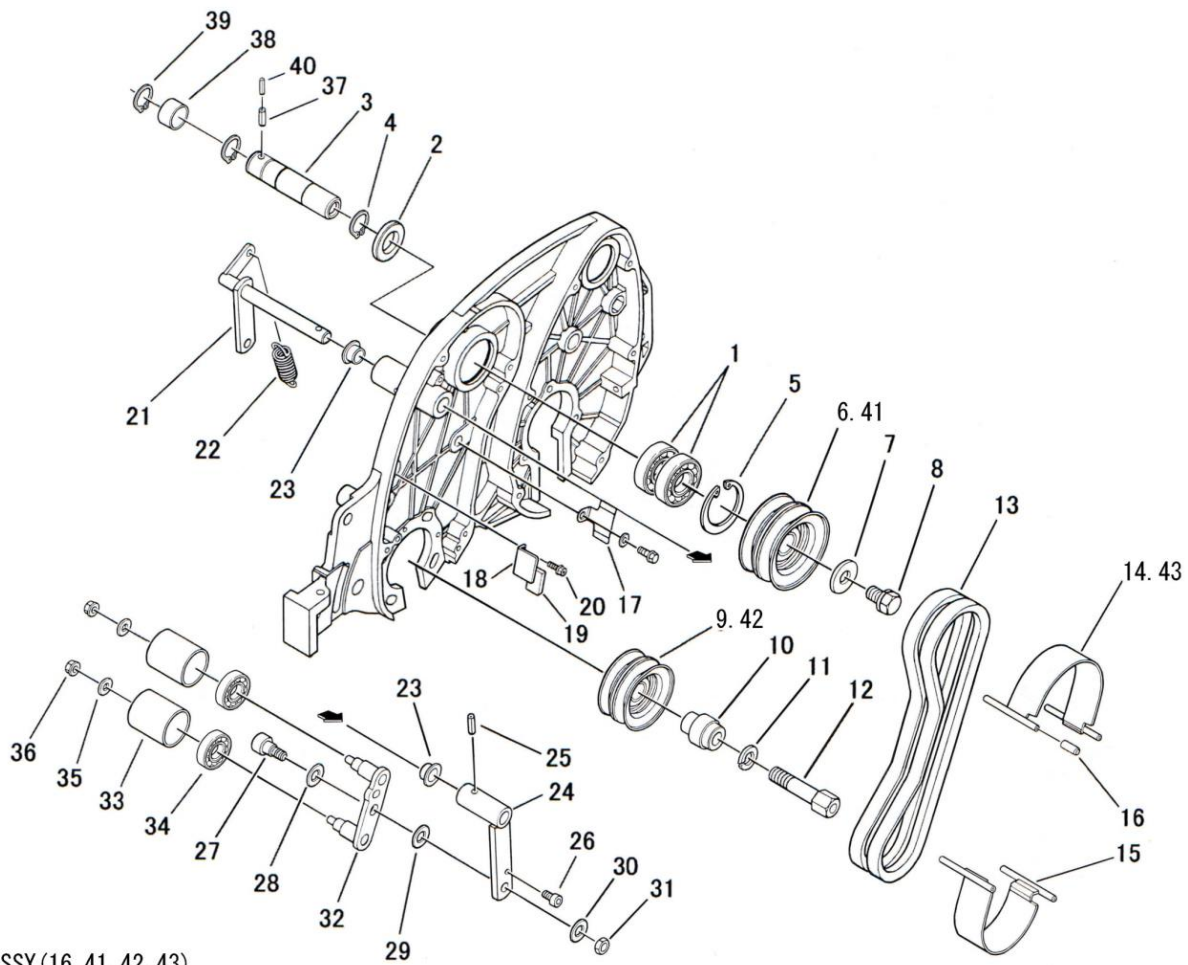
44. プーリASSY (16. 41. 42. 43)
