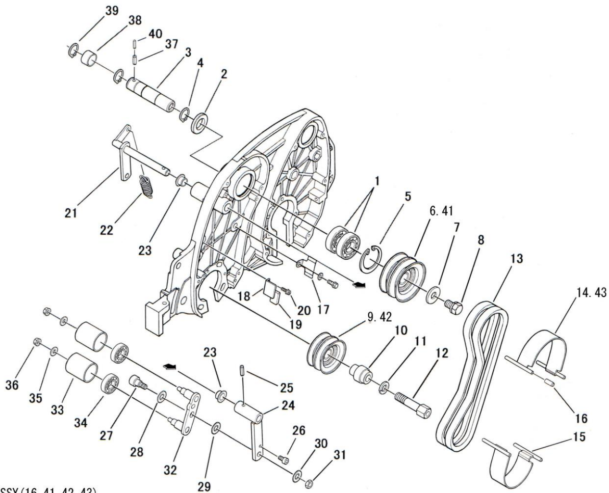
44. プーリASSY (16. 41. 42. 43)
