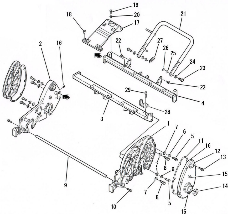
FIG. 01 フレーム関係 FRAME
