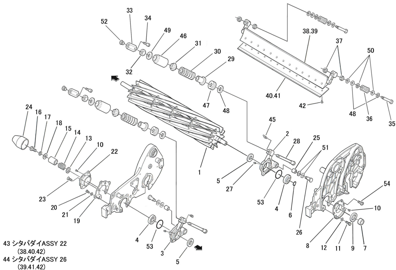
FIG. 07 刈刃関係 REEL BLADE
