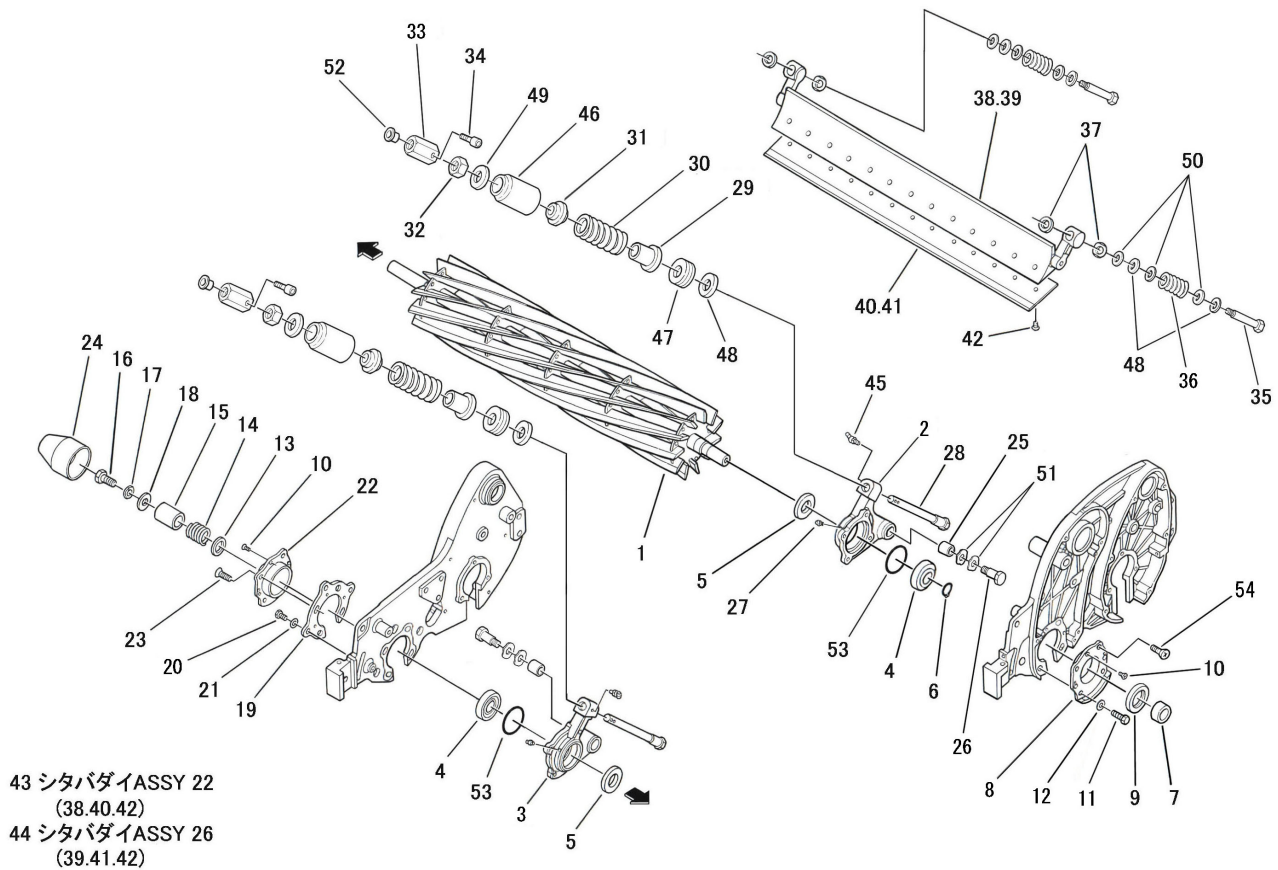
FIG. 07 刈刃関係 REAR ROLLER
