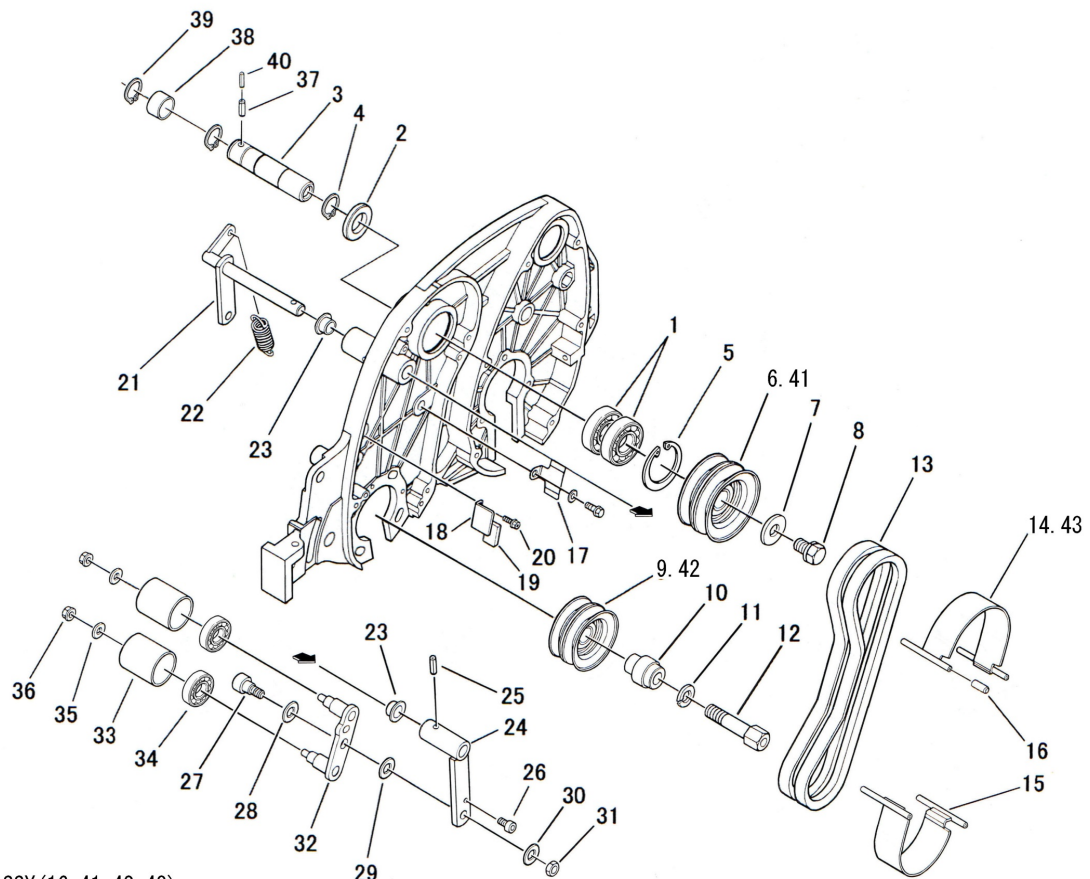
44. プーリASSY (16. 41. 42. 43)
