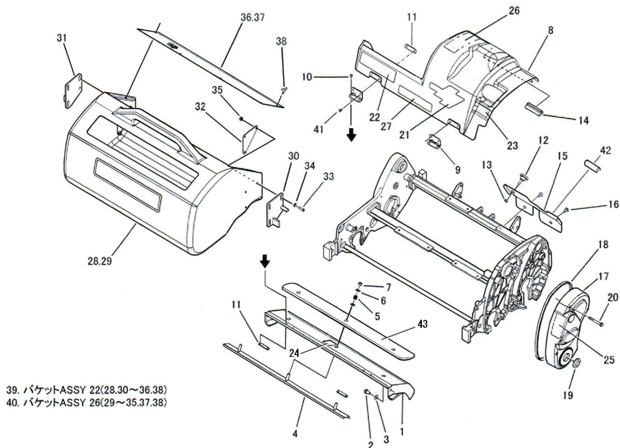
FIG. 02 カバー、バケット関係 COVER, BUCKET
