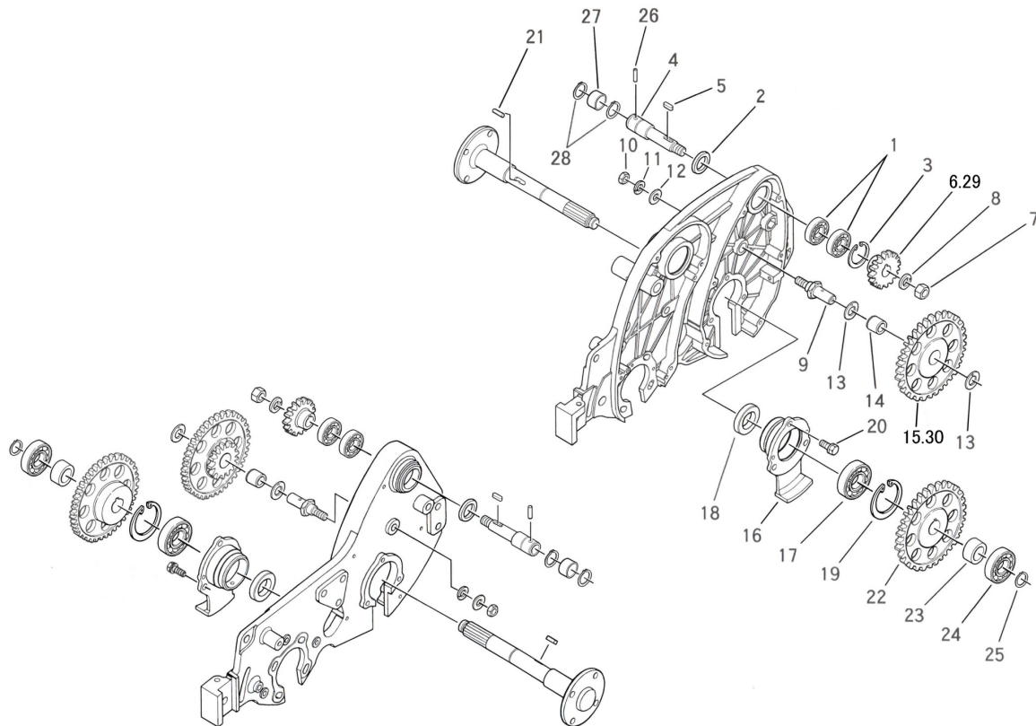
31.ギヤASSY(29.30)
