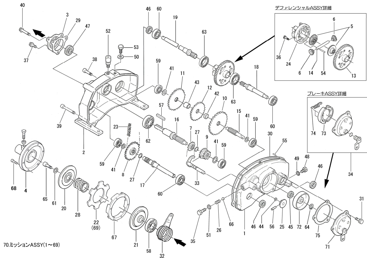
FIG. 03 ミッション関係 MISSION
