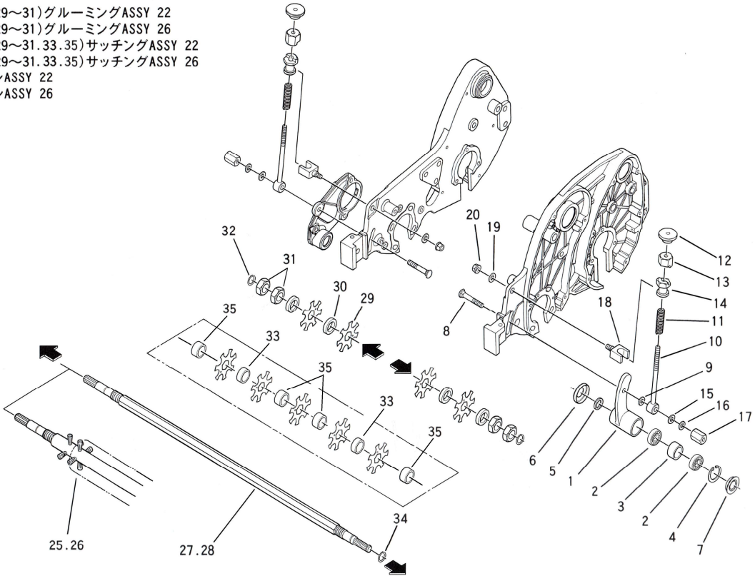
FIG. 09 グルーミングカッター関係 GROOMING CUTTER
