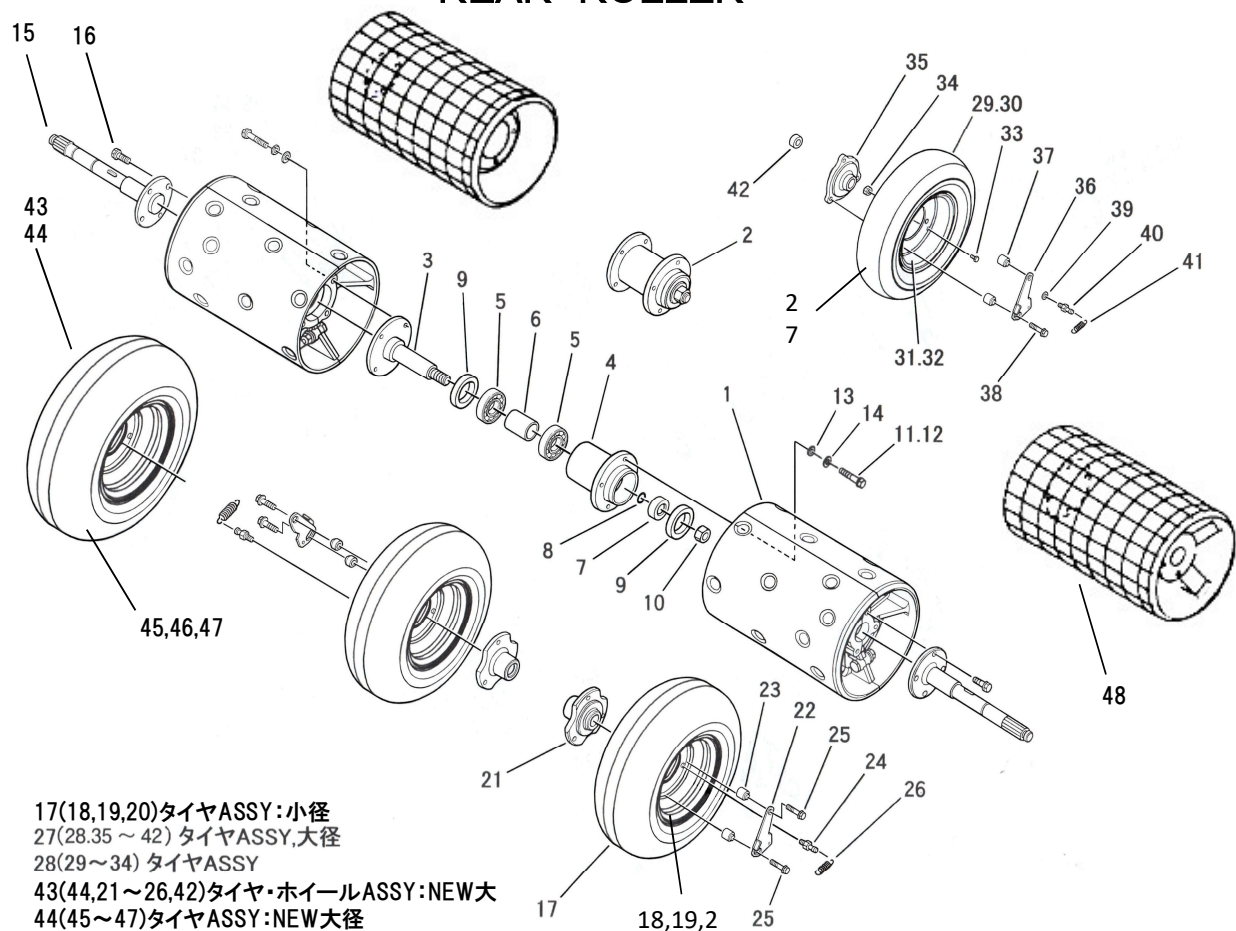
FIG. 11 後部ローラー関係 REAR ROLLER
