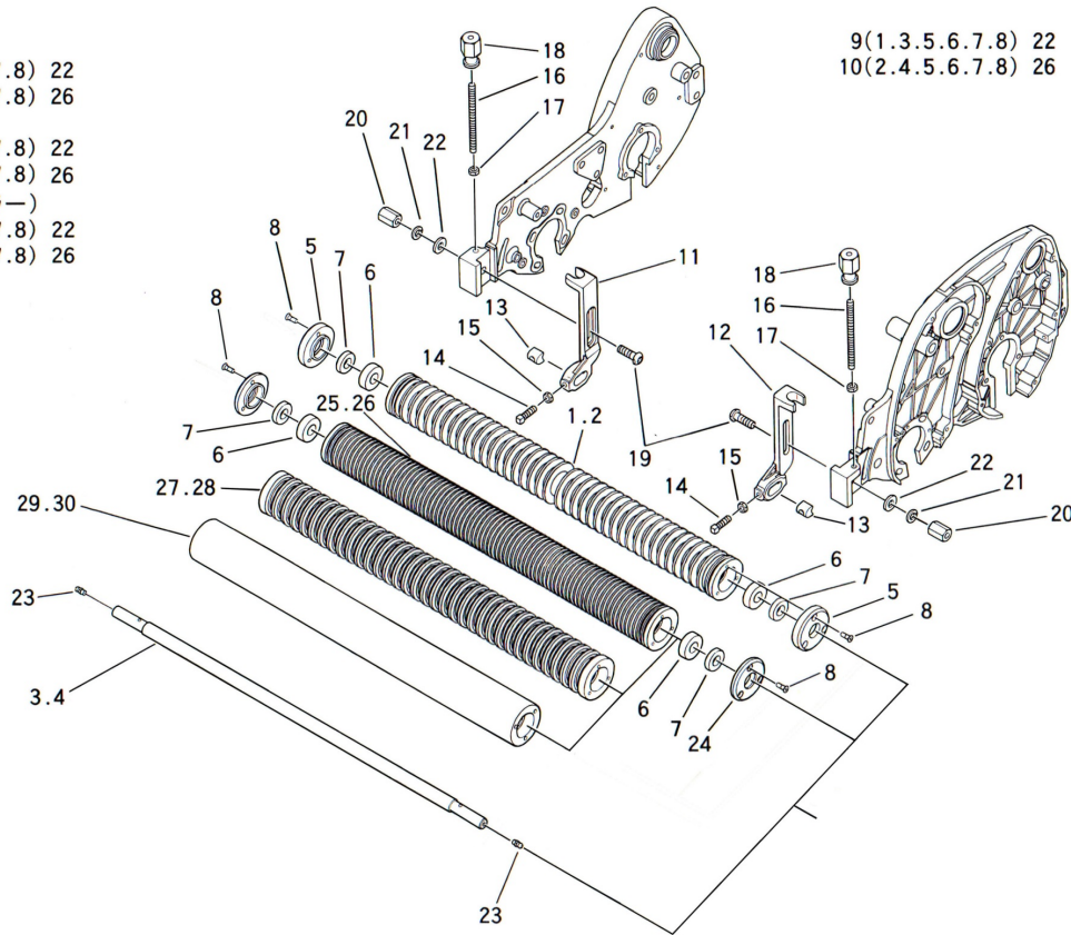
FIG. 10 前ローラー関係 FRONT ROLLER
