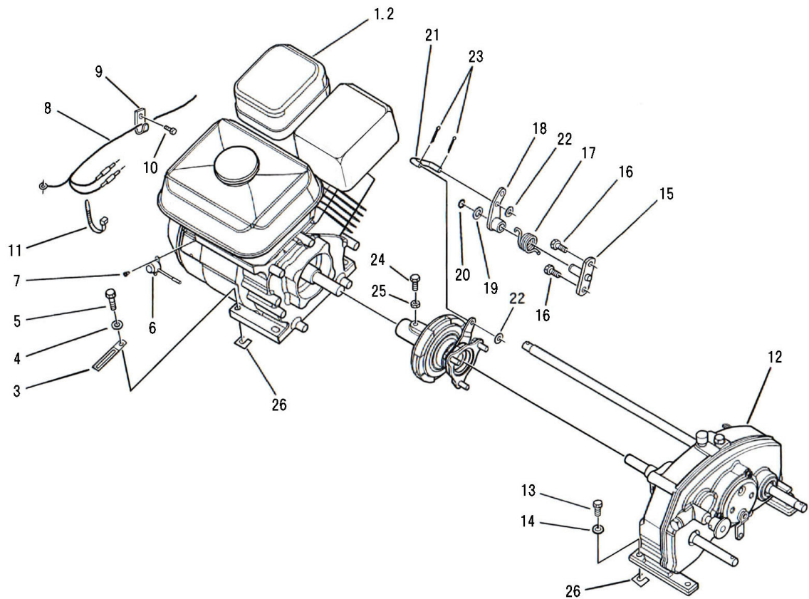
FIG. 08 クラッチ関係 CLUTCH
