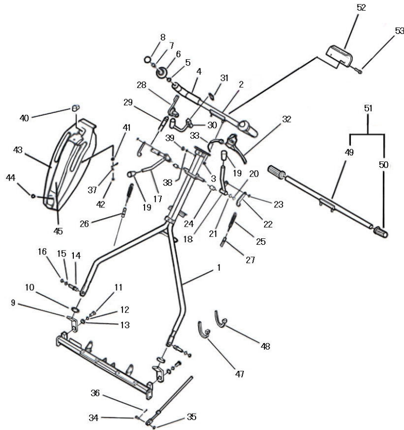
FIG. 12 ハンドル関係 HANDEL
