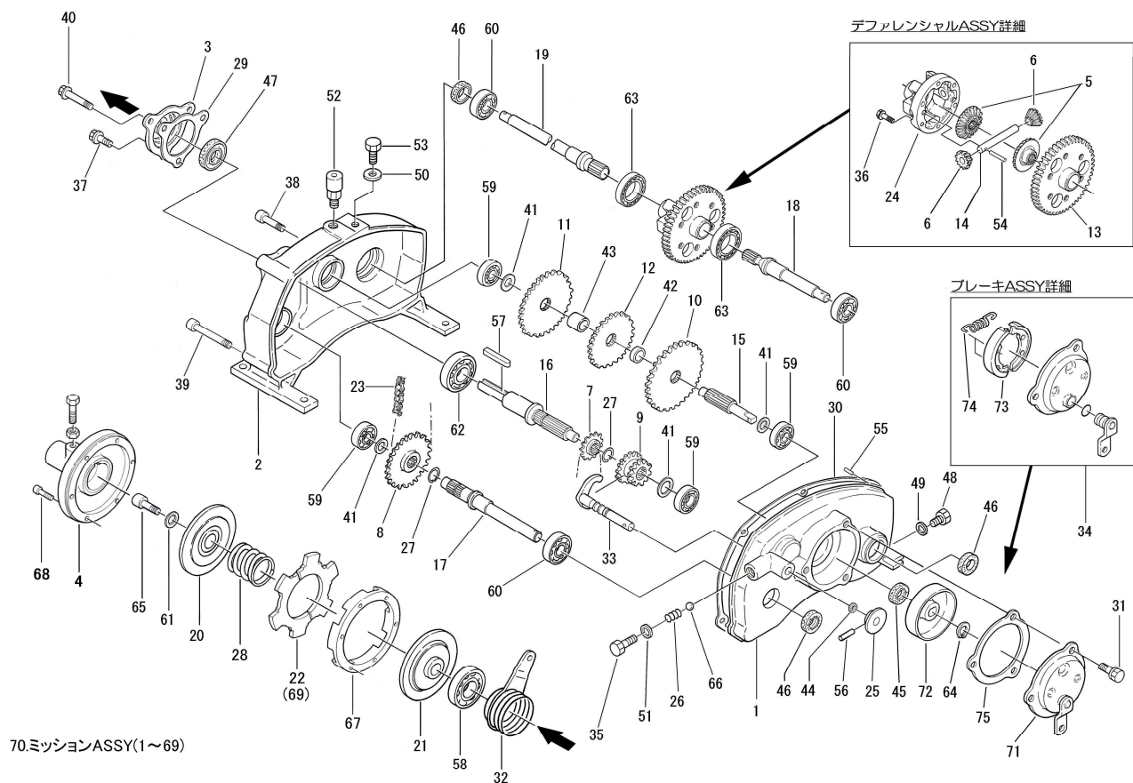
FIG. 05 ミッション関係 MISSION
