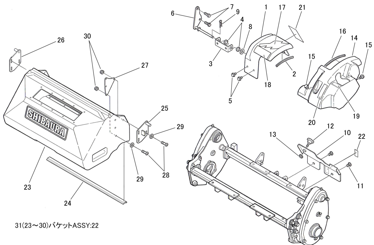
FIG. 03 カバー・バケット関係 COVER・BUCKET
