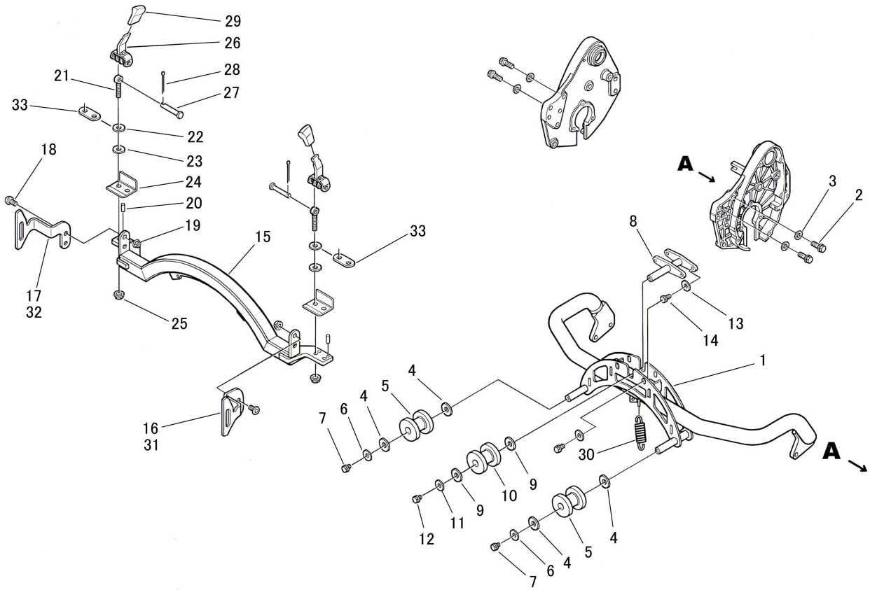
アーム関係 ARM
