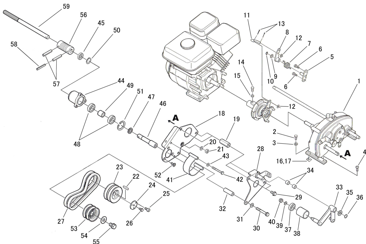
FIG. 04 クラッチ関係 CLUTCH
