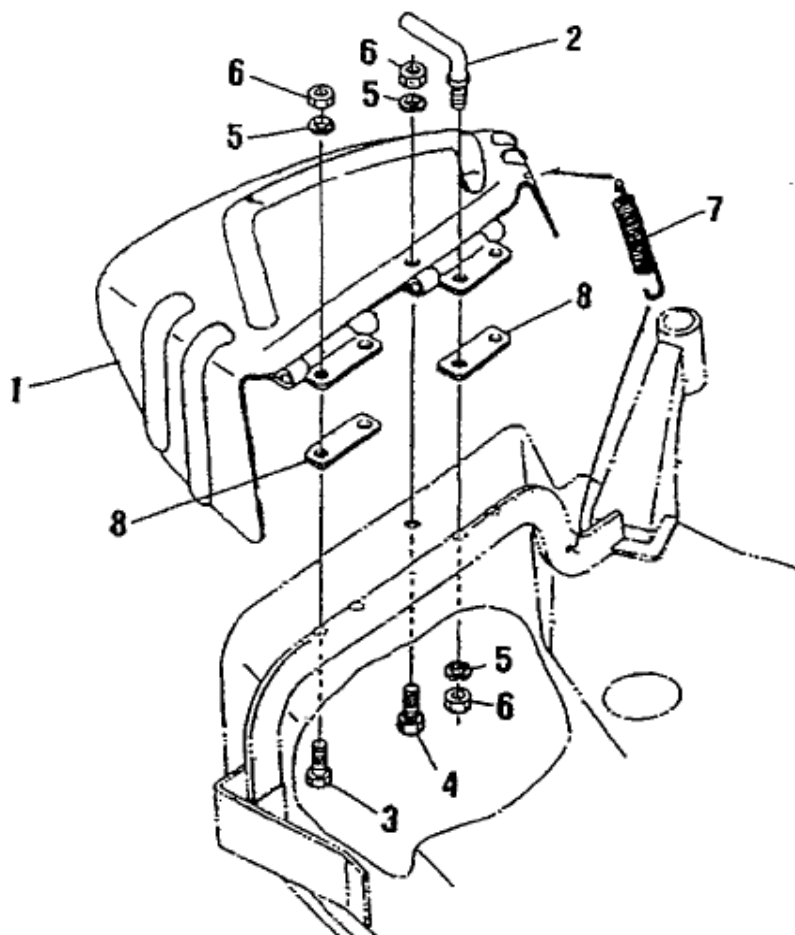
デイスチャージカバー DISCHARGE COVER
