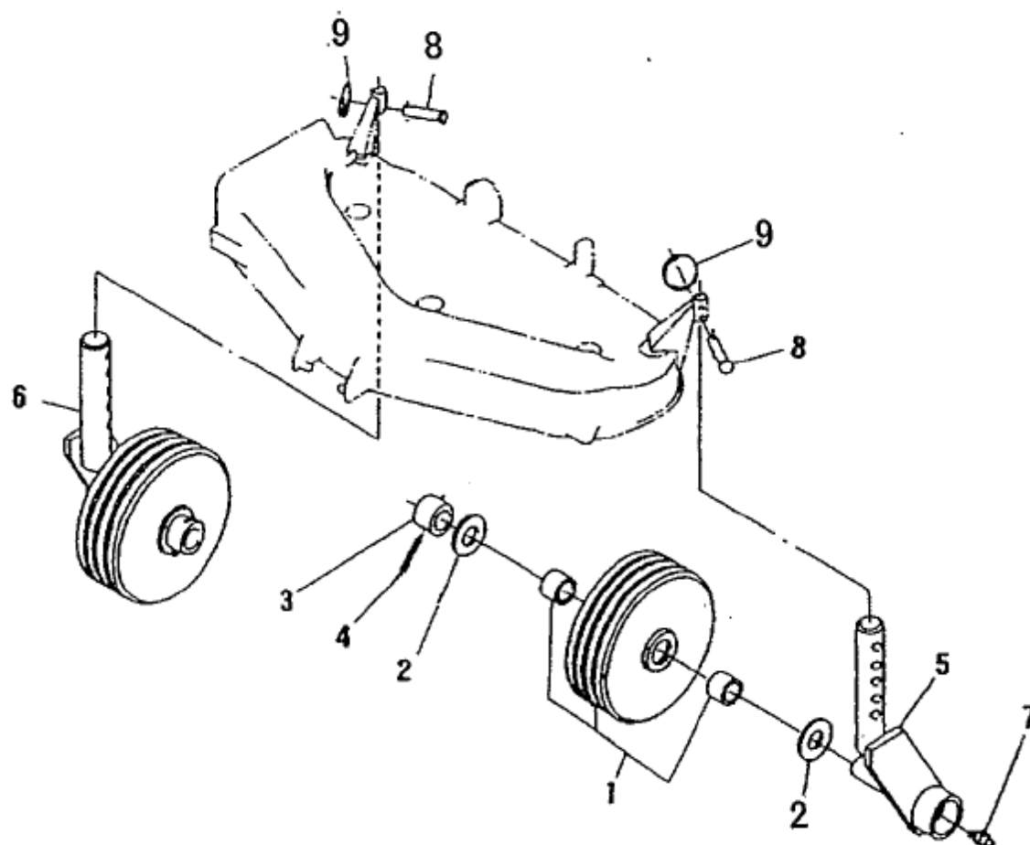
ローラ ; サイド ROLLER ; SIDE
