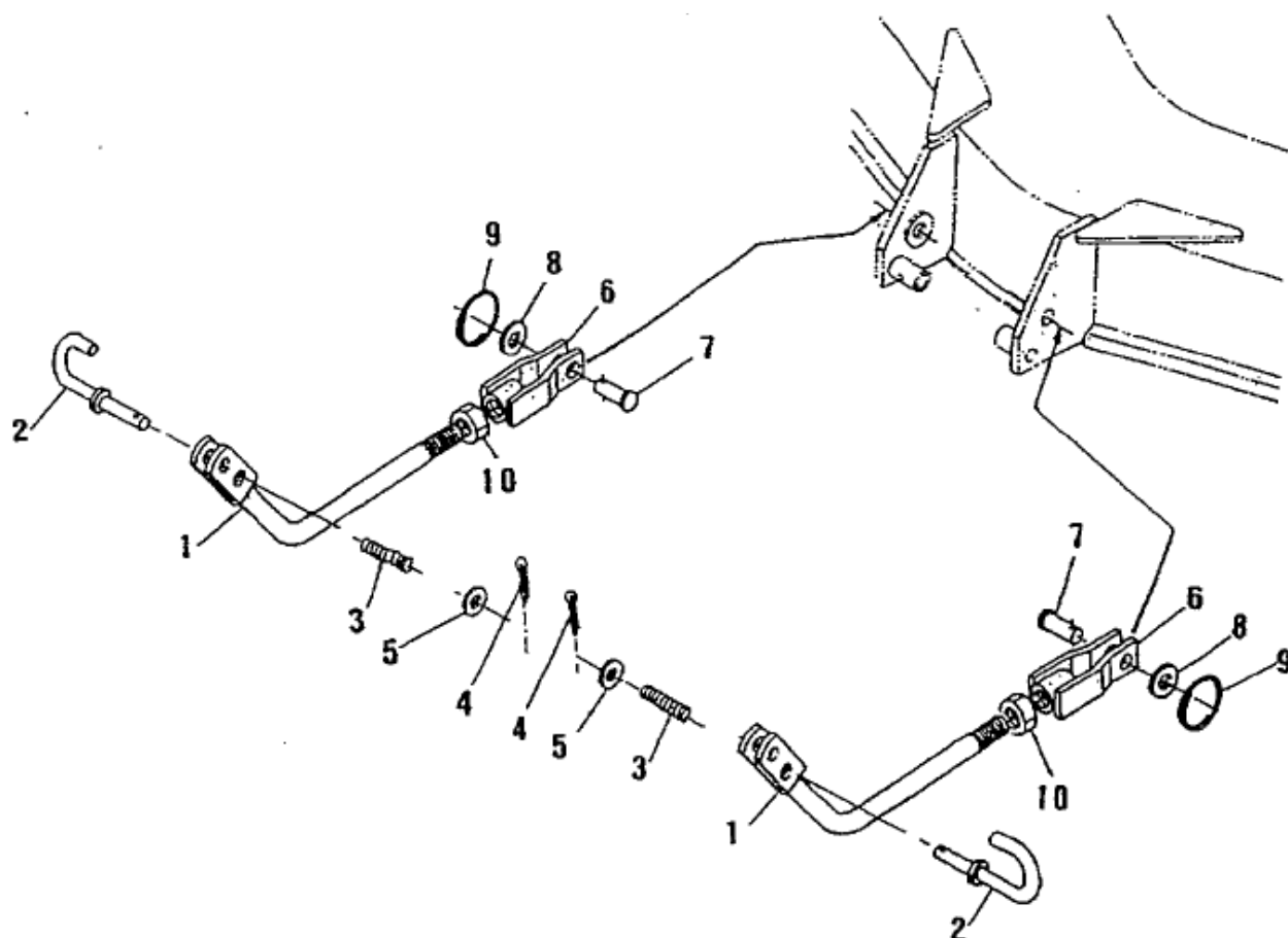
リフトリンク ; フロント LIFT LINK ; FRONT
