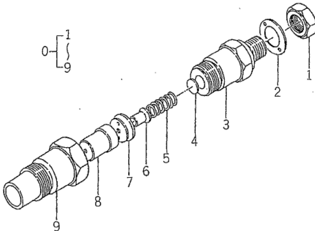
ノズル、ホルダー NOZZLE, HOLDER
