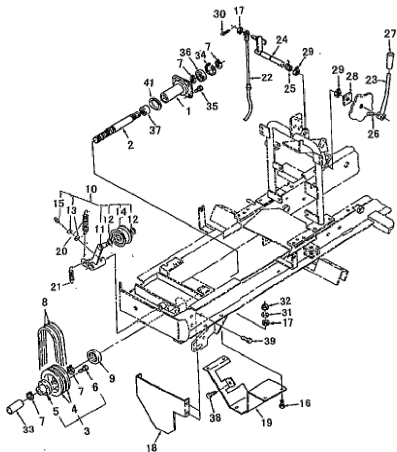
フロントPTO FRONT P.T.O
