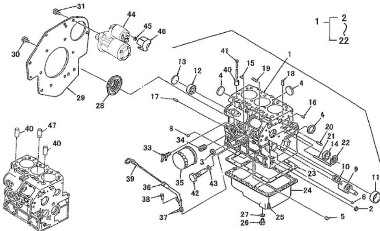
タペット組付け位置
