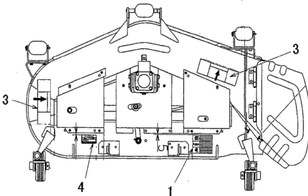
デカル :48 モア DECALS ; 48" MOWER
