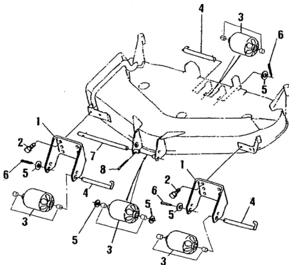
ローラ :フロント & リア ROLLER ;FRONTT & REAR
