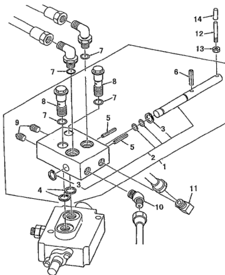
ハイドロリック デバータバルブ (オプション) HYDRAULIC DIVERTER VALVE (OPTION)
