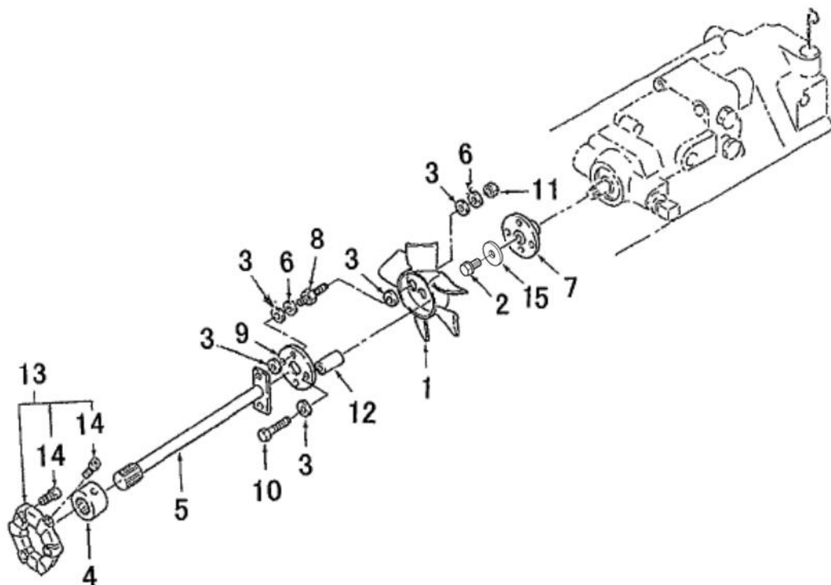
プロペラシャフト PROPELLER SHAFT
