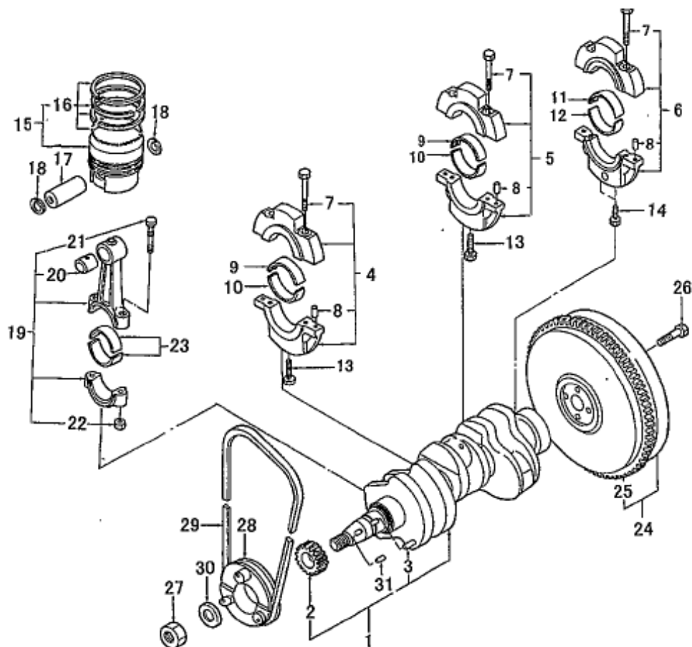
クランクシャフト、ピストン CRANK SHAFT, PISTON
