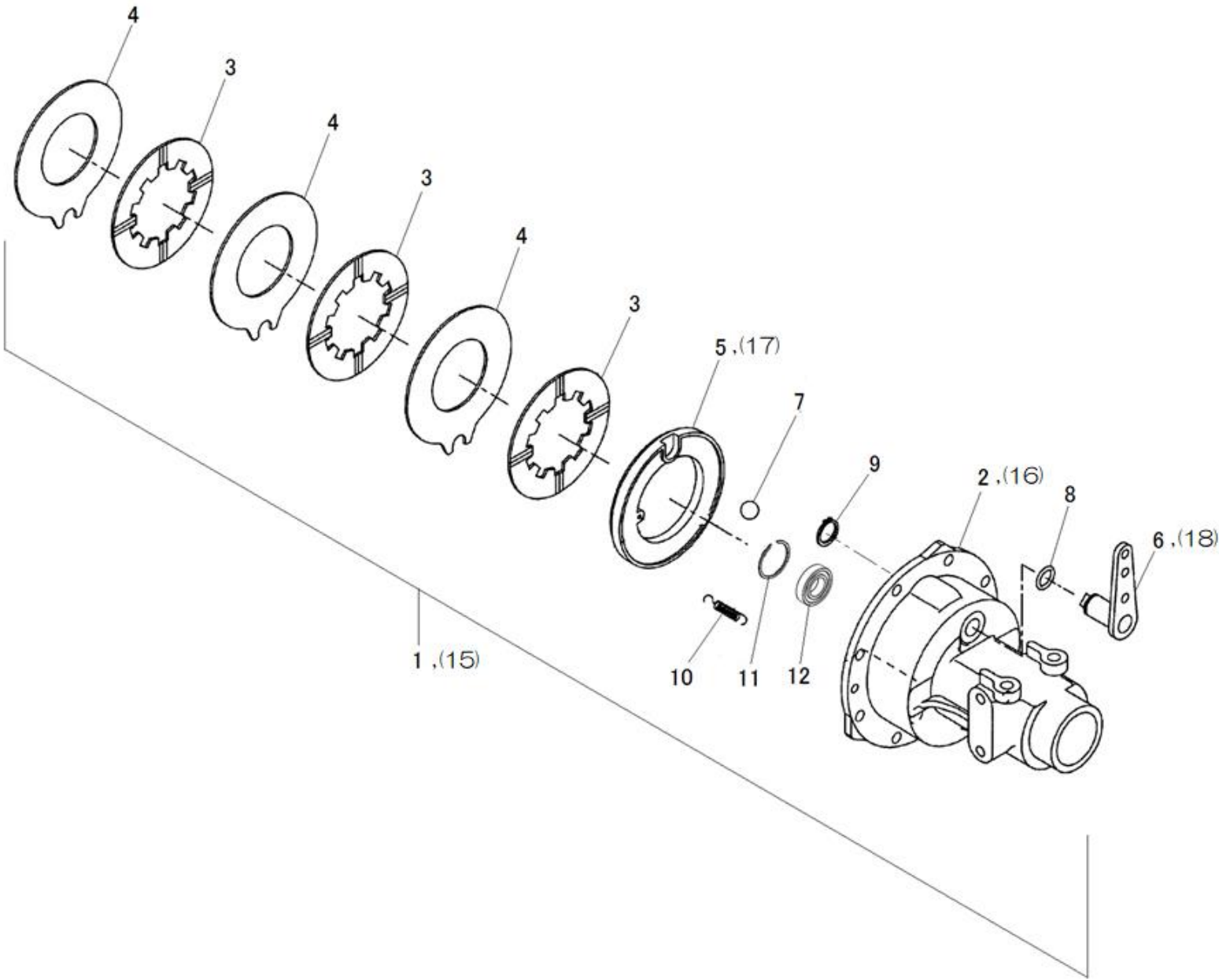
FIG.228 BRAKE ASSEMBLY ブレーキASSY
