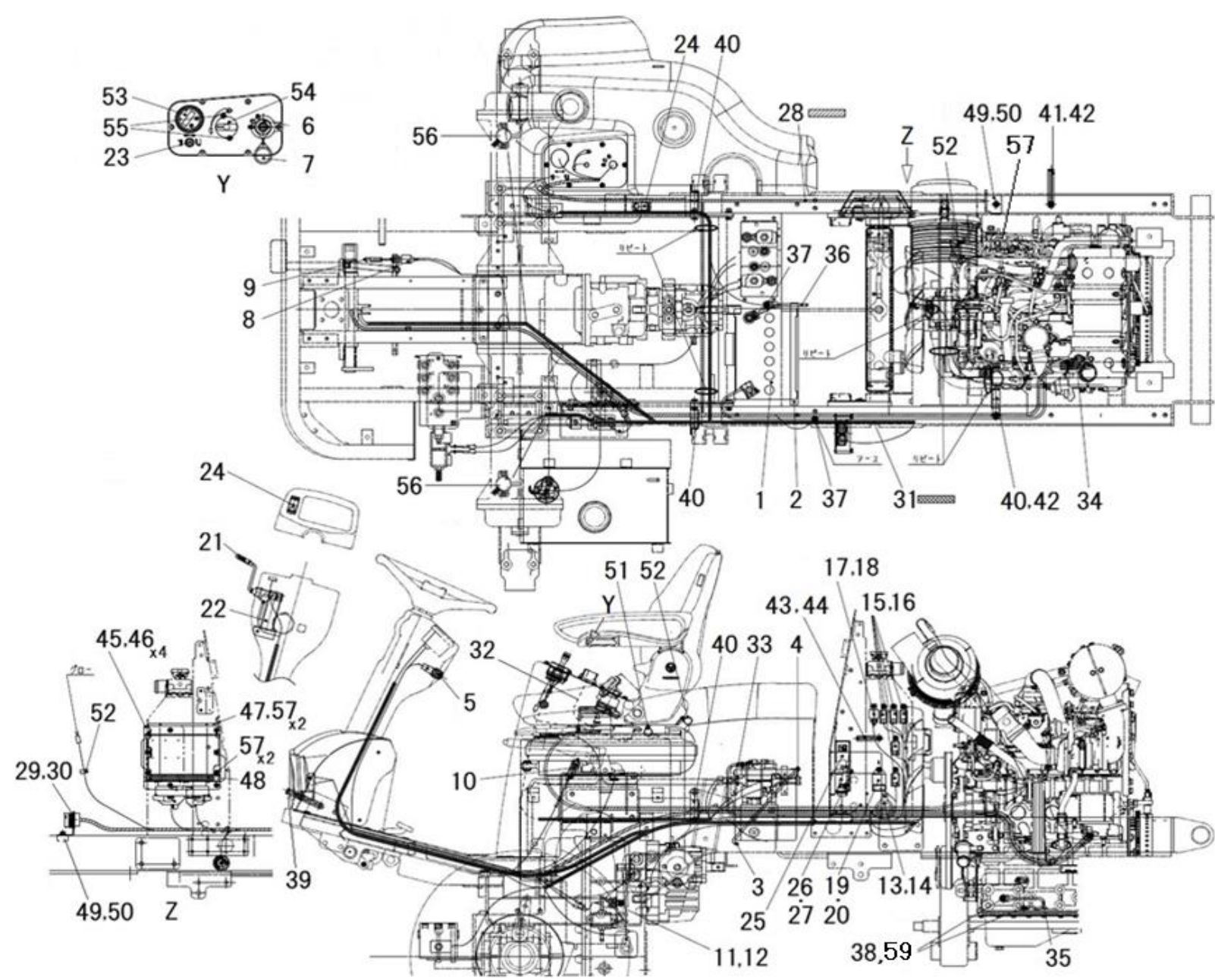
FIG.236-2 HARNESS ハイセン
