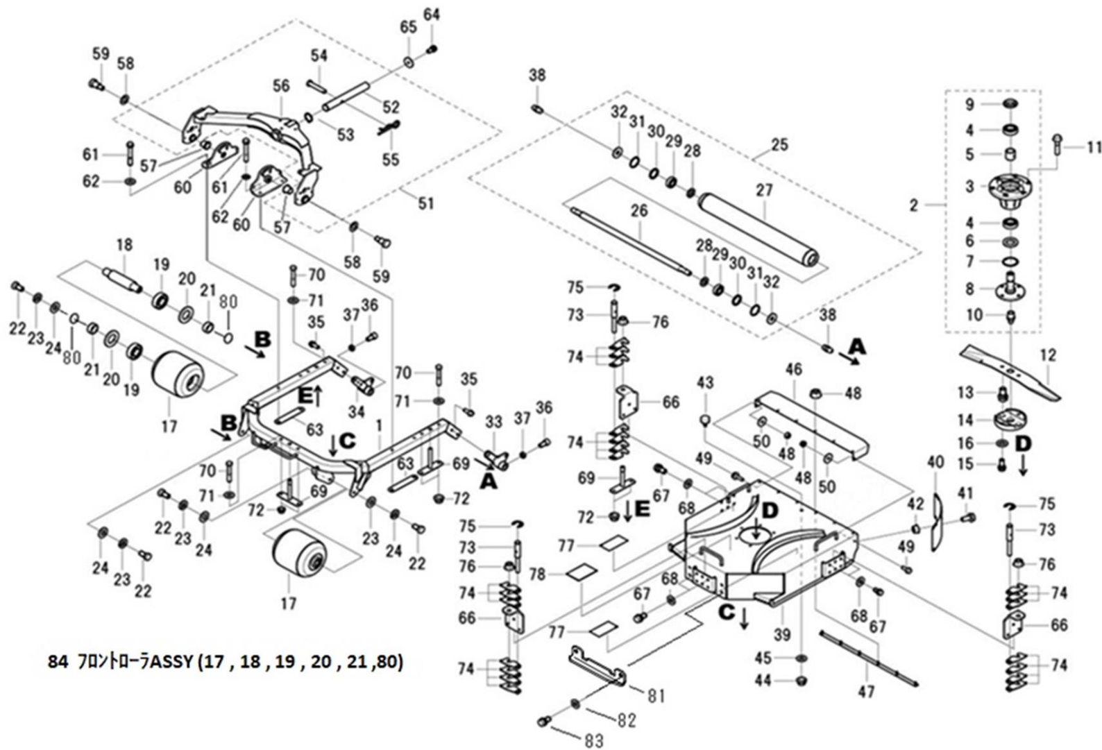
FIG.301 ROTARY UNIT ロータリーユニット
