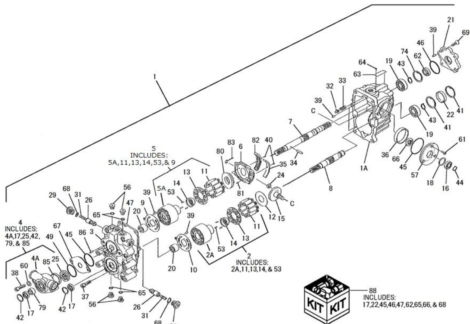
FIG.223 HYDRAU STATIC TRANSMISSION ユアツトランスミッション
