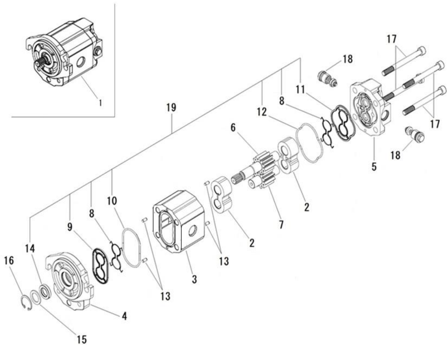
FIG.232 OIL MOTOR オイルモータ
