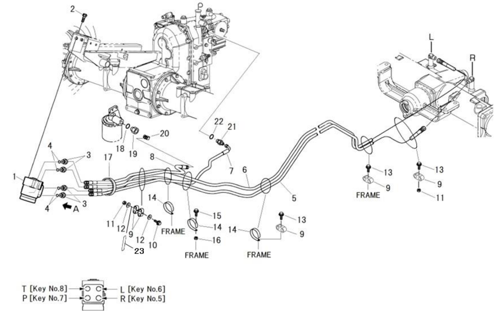
FIG.220 STEERING CASE, HYDRAULICS ステアリングケース
