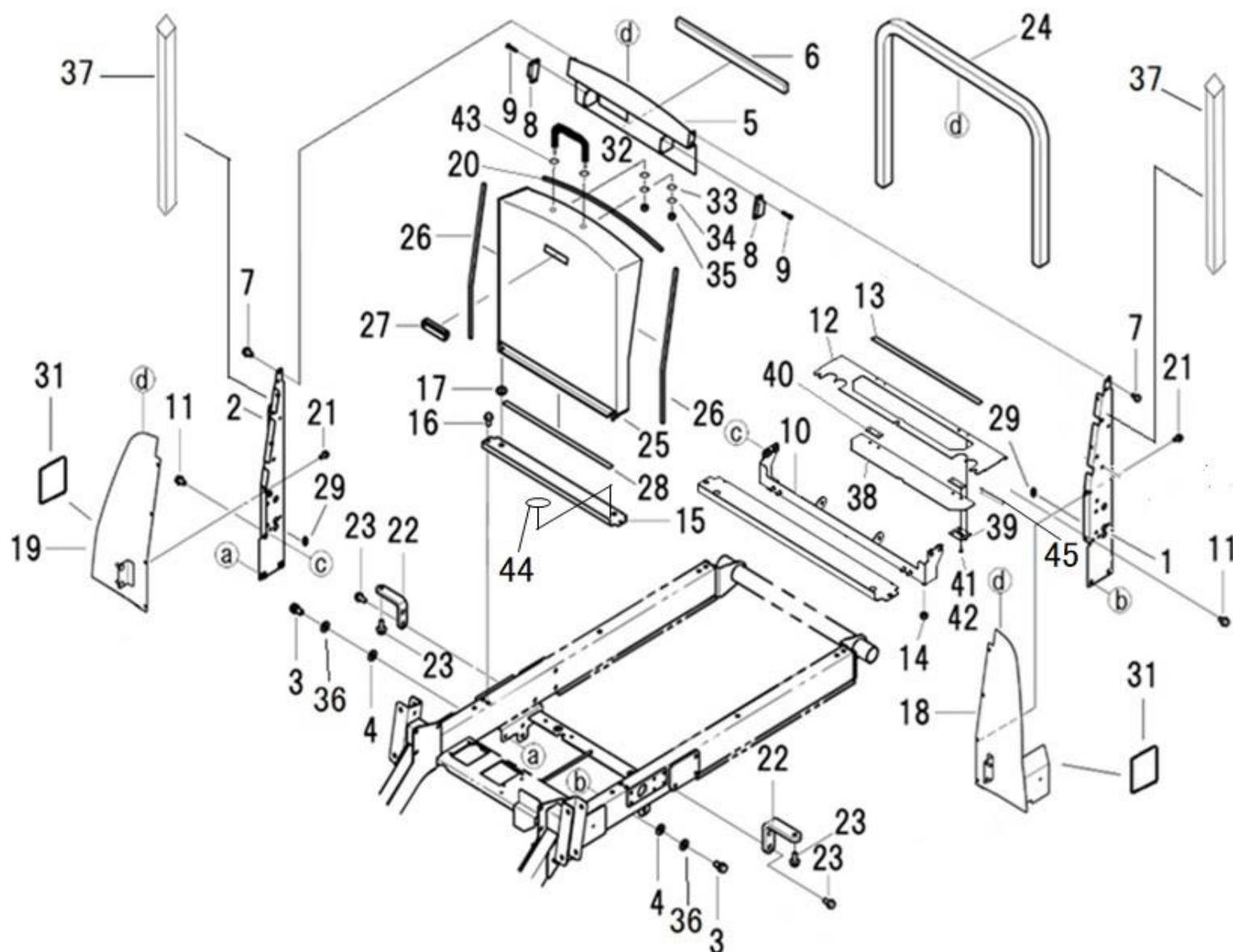
FIG.226 ENGINE SCREEN エンジンスクリーン
