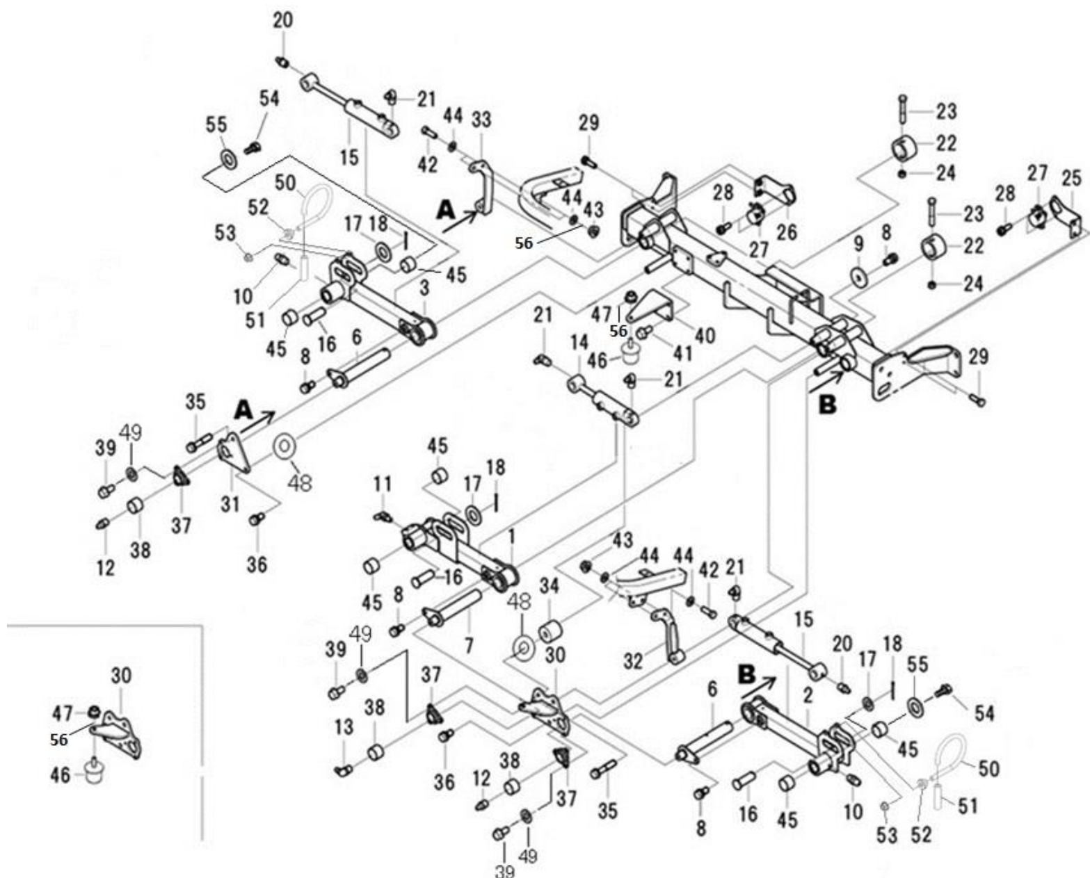
FIG.217 LIFT FRONT フロントリフト
