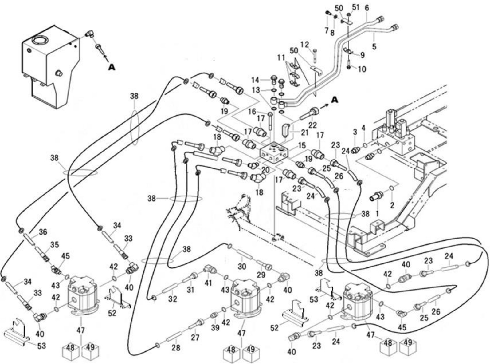
FIG.233 HYDRAULIC PIPING(FRONT) ユアツハイカン(フロント)
