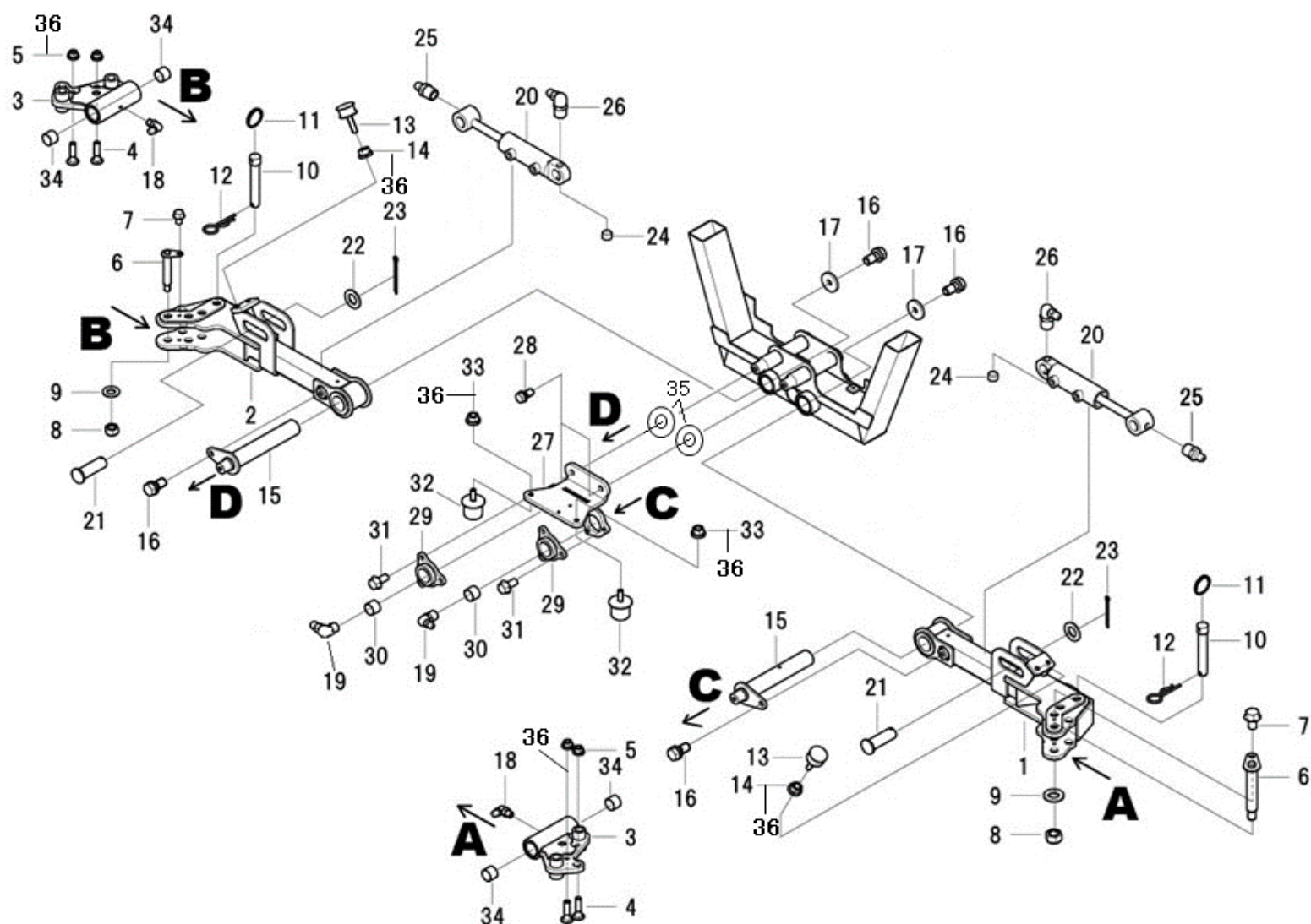
FIG.218 LIFT REAR リアリフト
