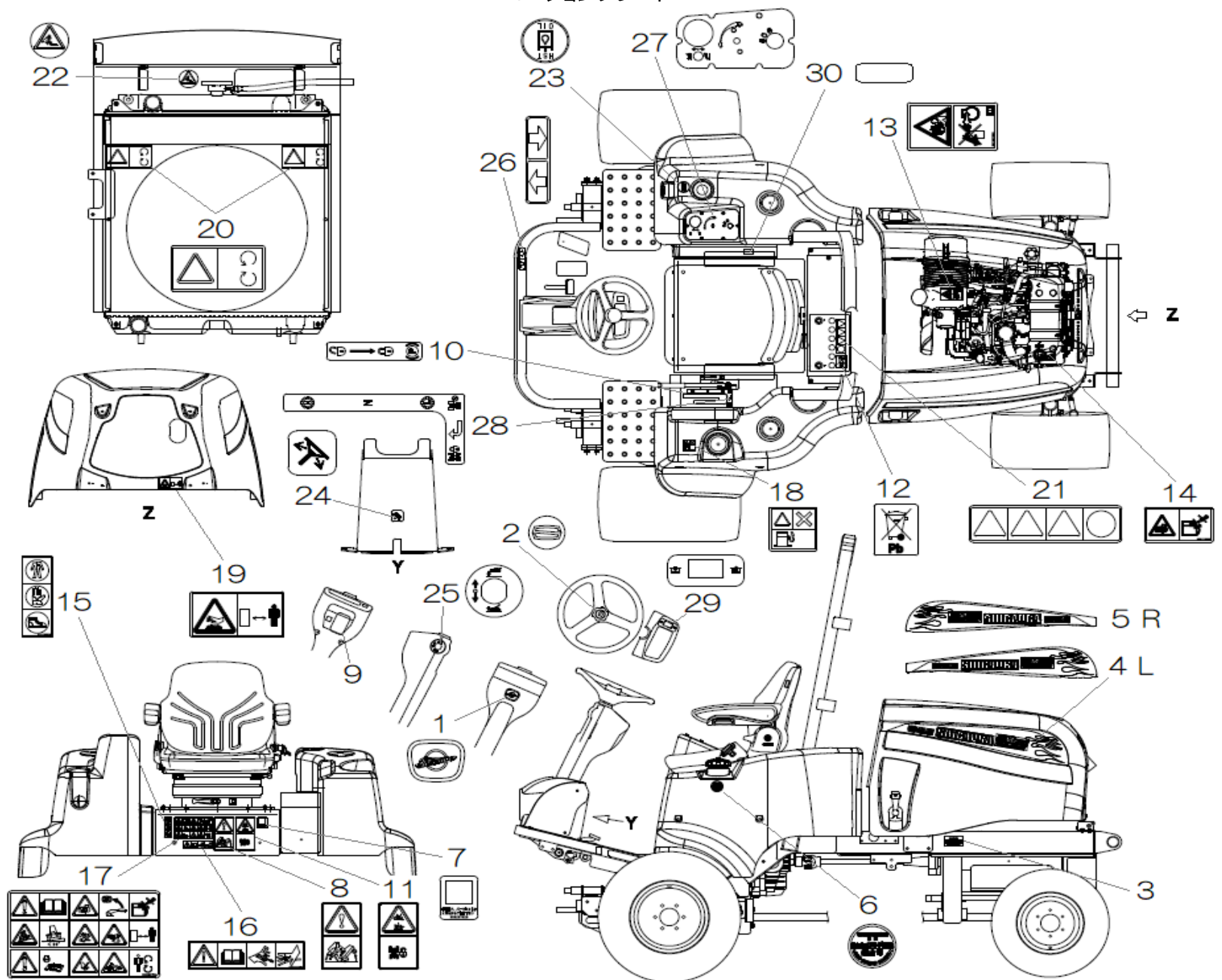
FIG237 CAUTION PLATE コーションプレート
