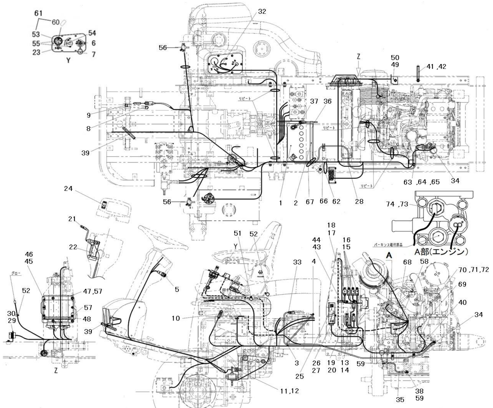
ハーネス
