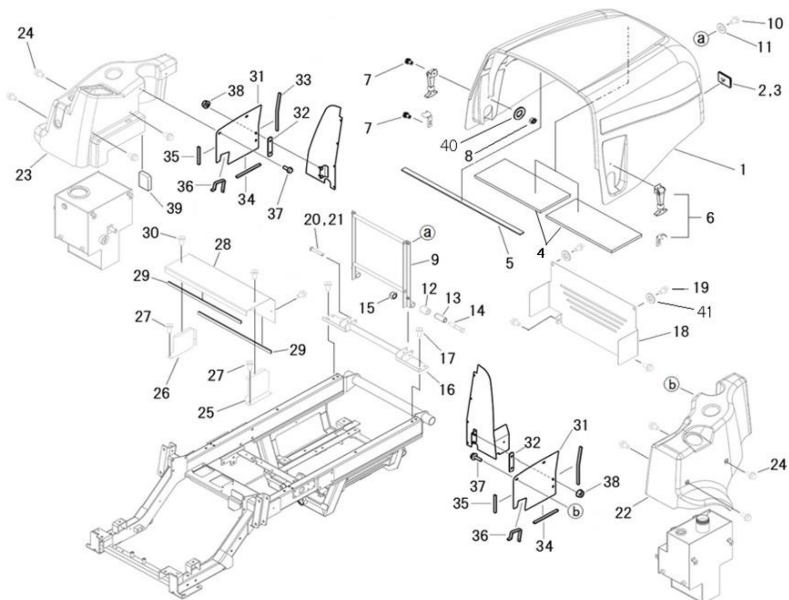
ボンネット、フエンダ
