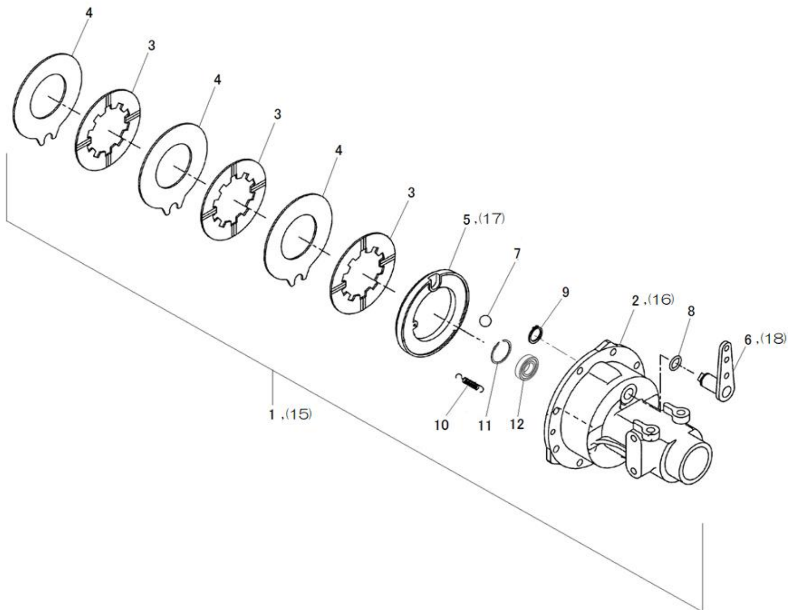
FIG.228 BRAKE ASSEMBLY ブレーキASSY
