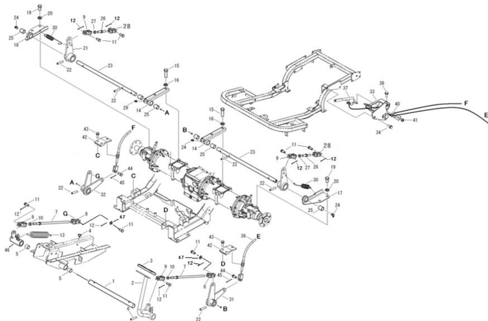
FIG.227 ブレーキペダル BRAKE PEDAL
