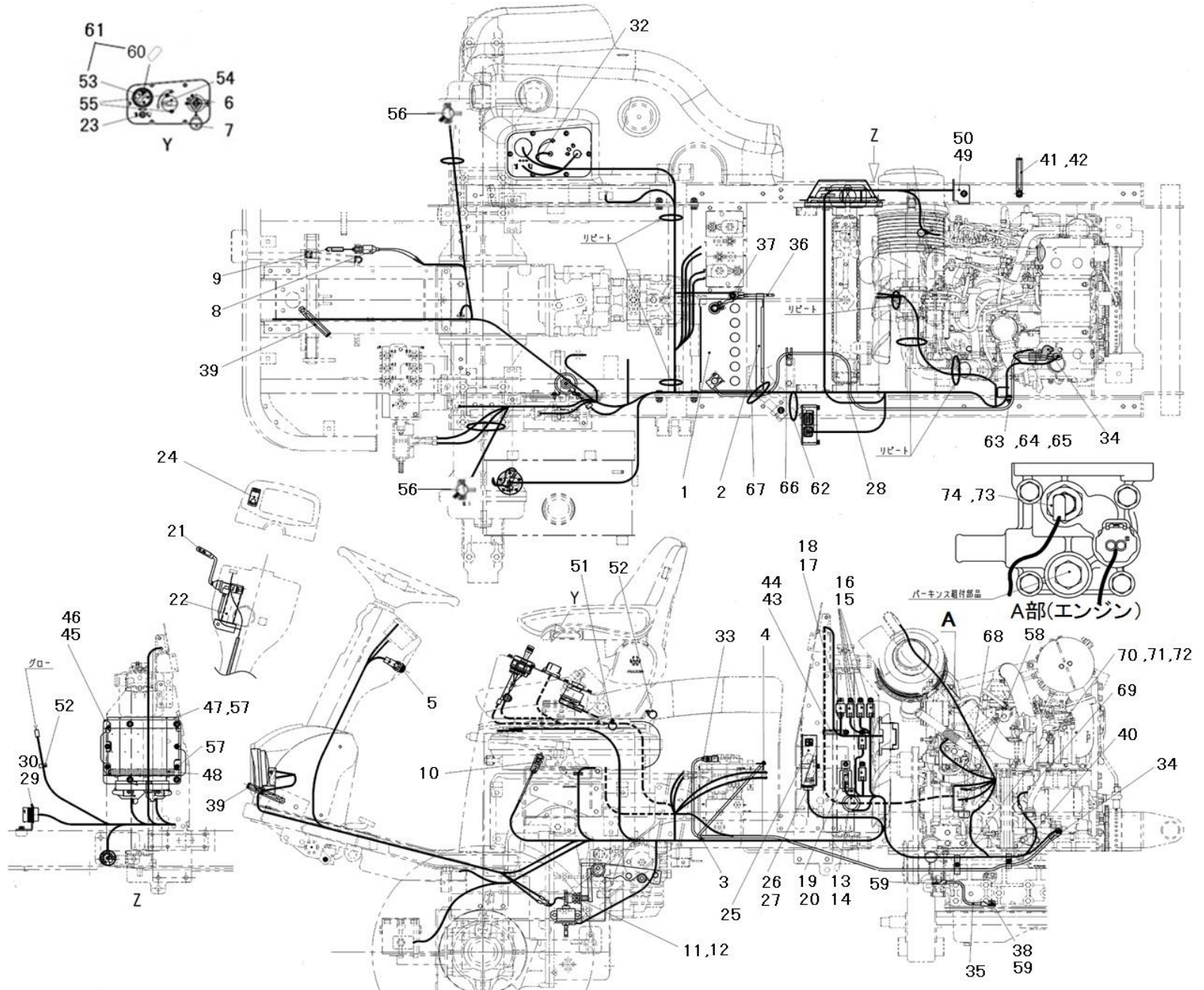
FIG.236 HARNESS ハーネス
