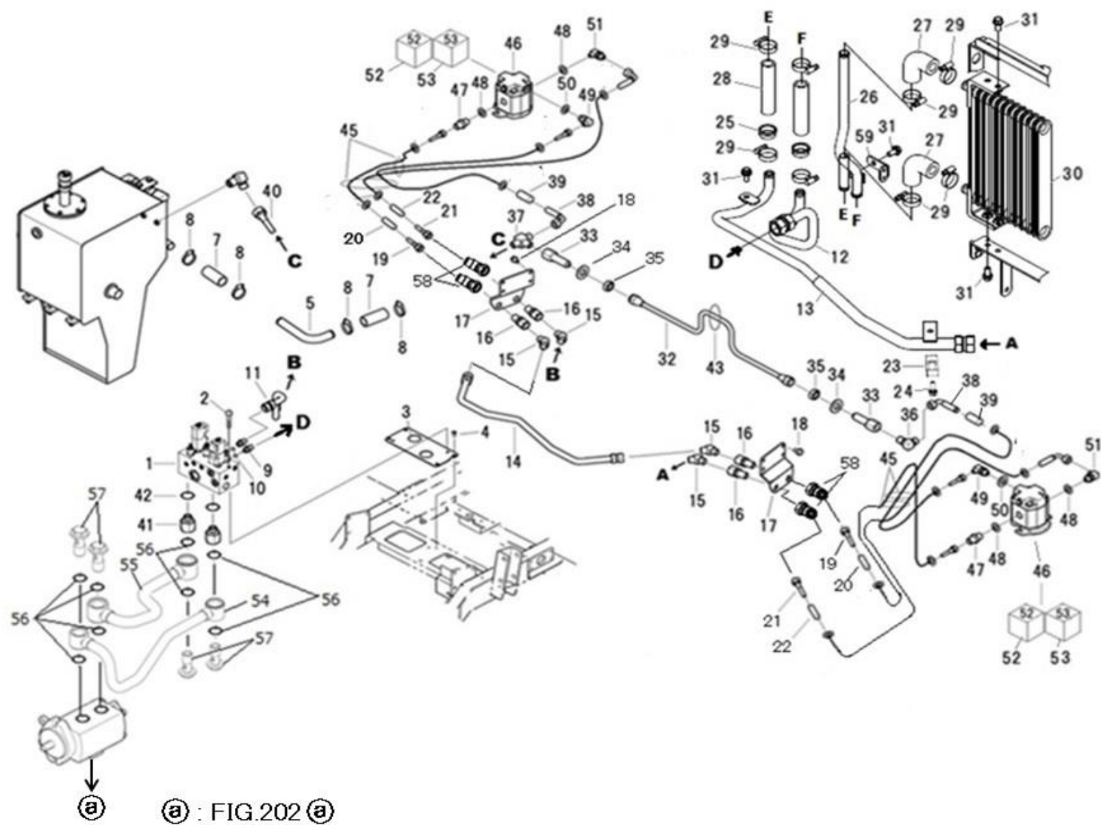
FIG.234 HYDRAULIC PIPING (REAR) エアツハイカン(リヤ)
