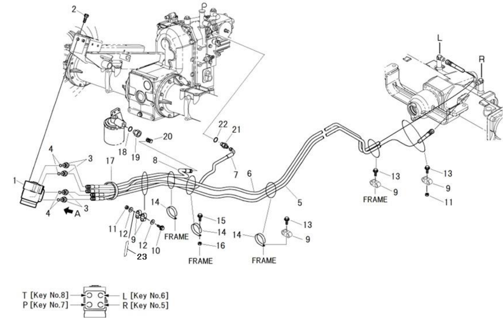
FIG.220 STEERING CASE, HYDRAULICS ステアリングケース
