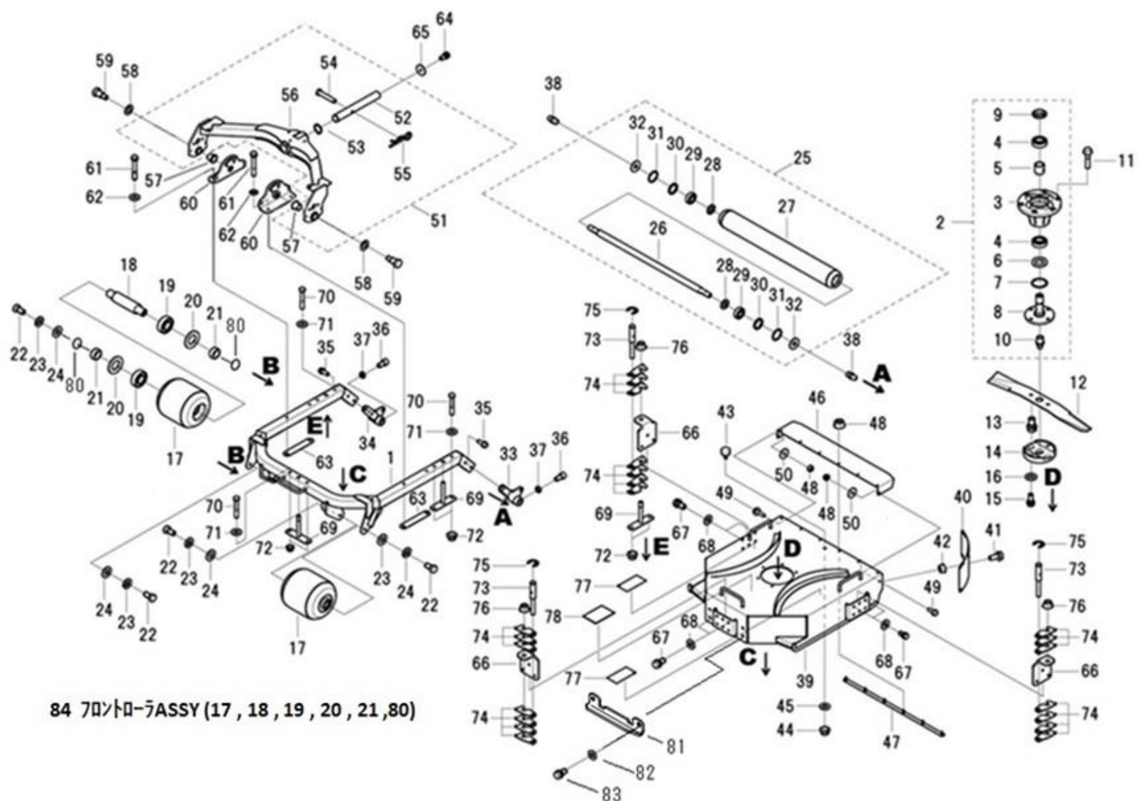
FIG.301 ROTARY UNIT ロータリーユニット
