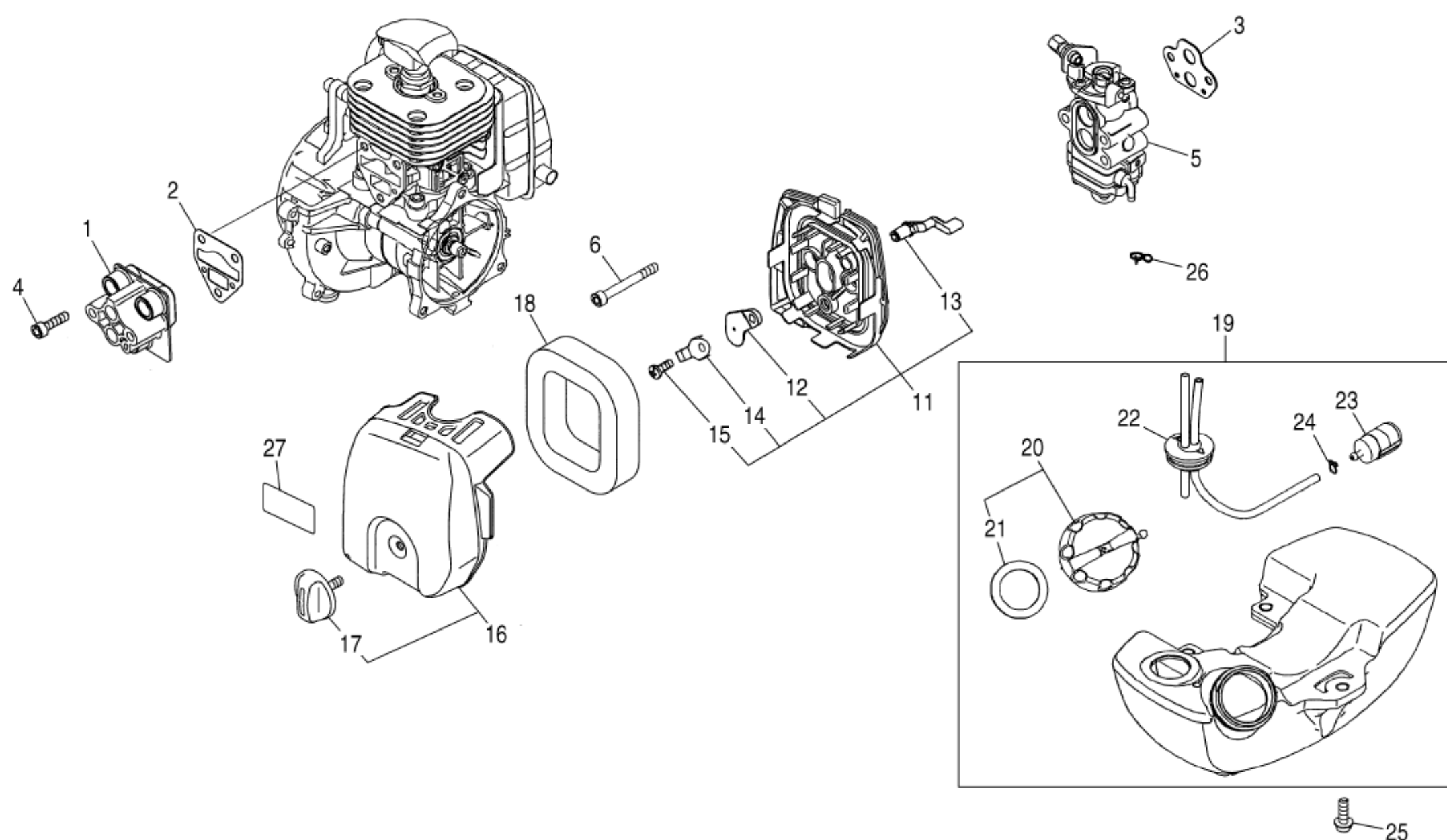
FIG 202. 燃料供給系
