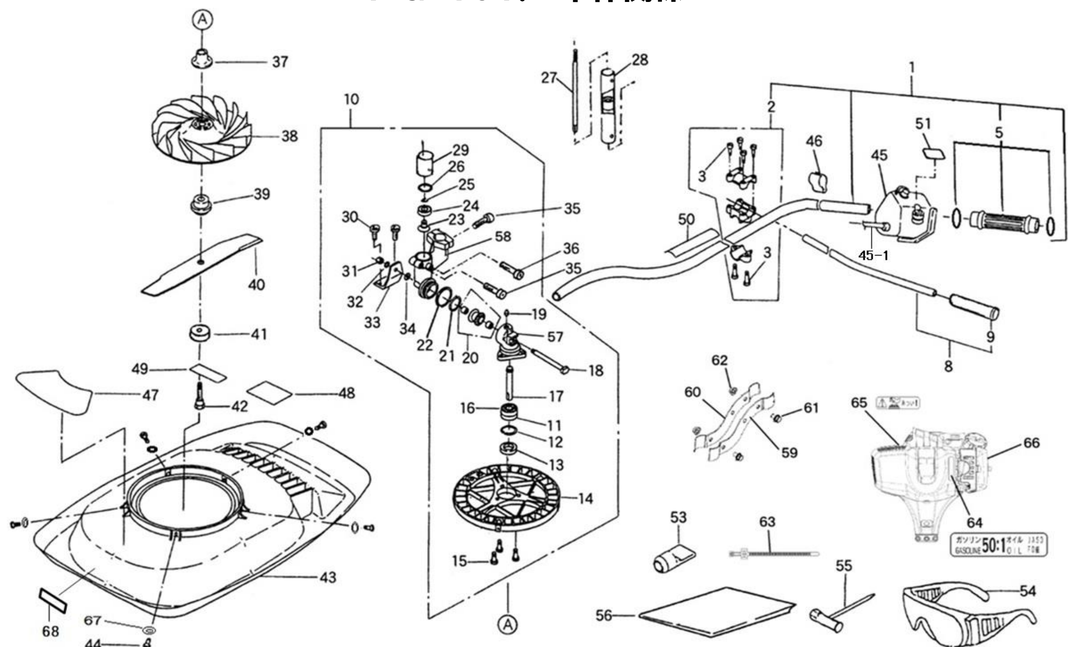
FIG 101. 本体関係
