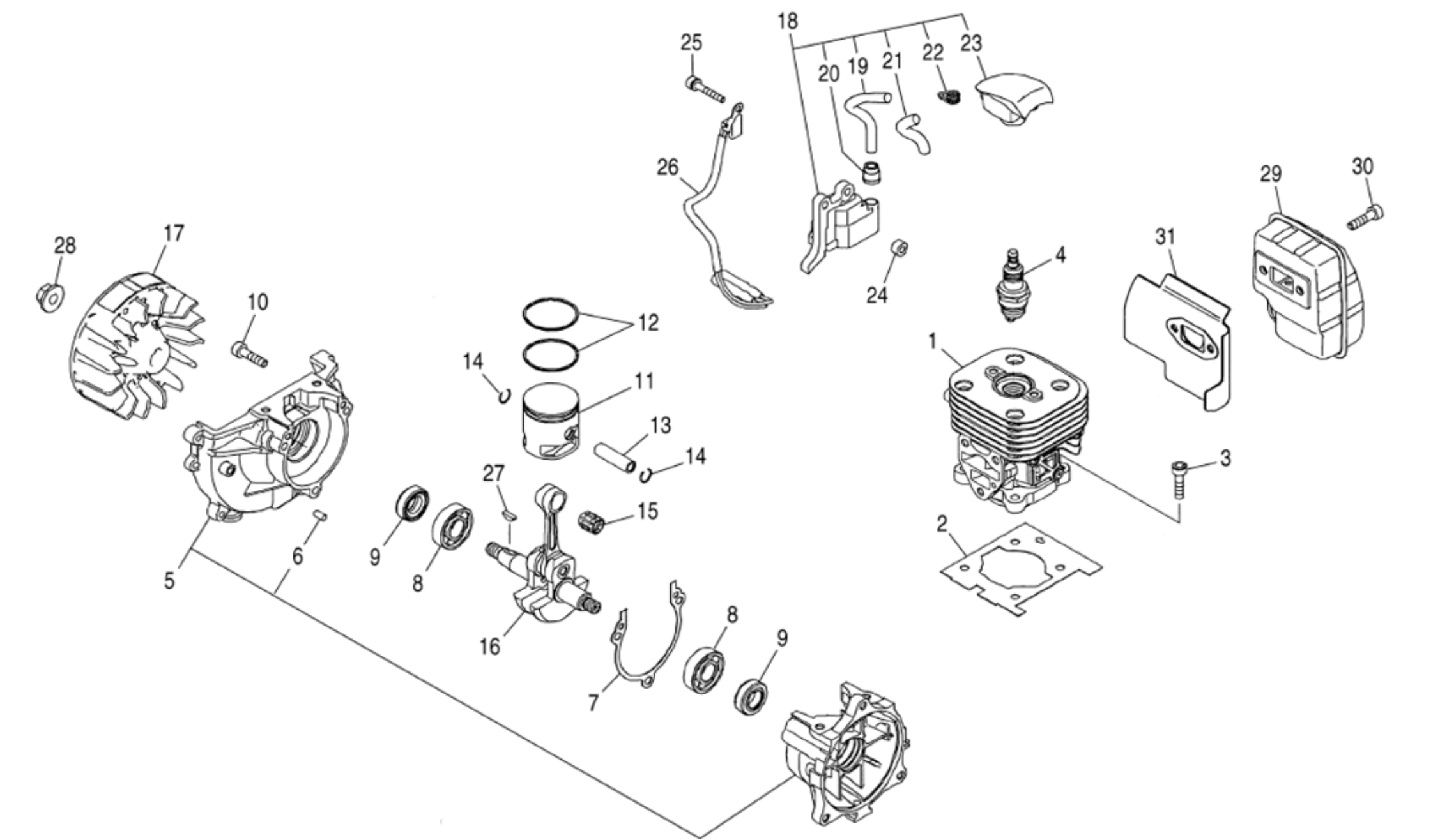
FIG 201. エンジンブロック・電装・マフラ
