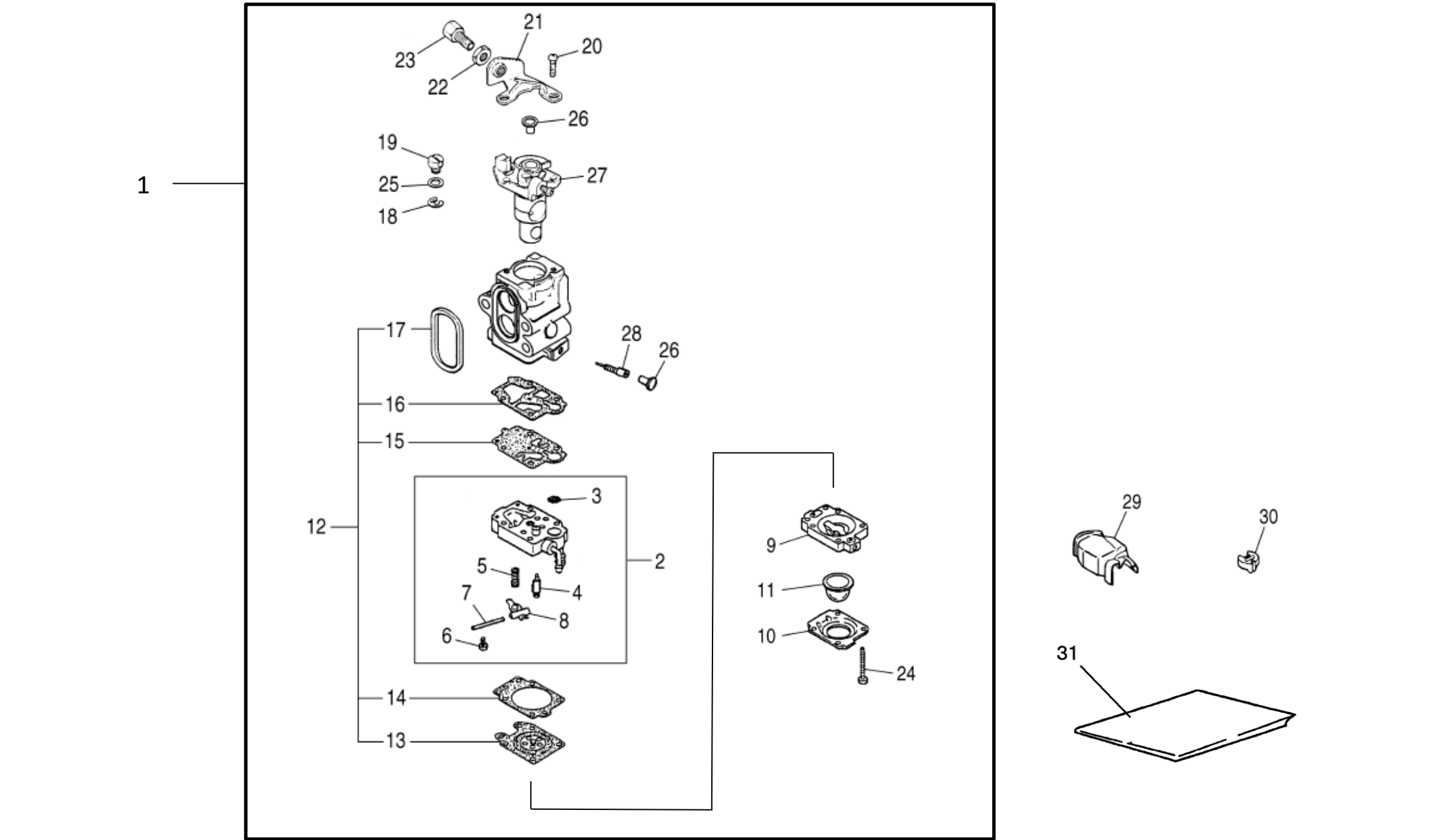
FIG 204. キャブレタ・付属品
