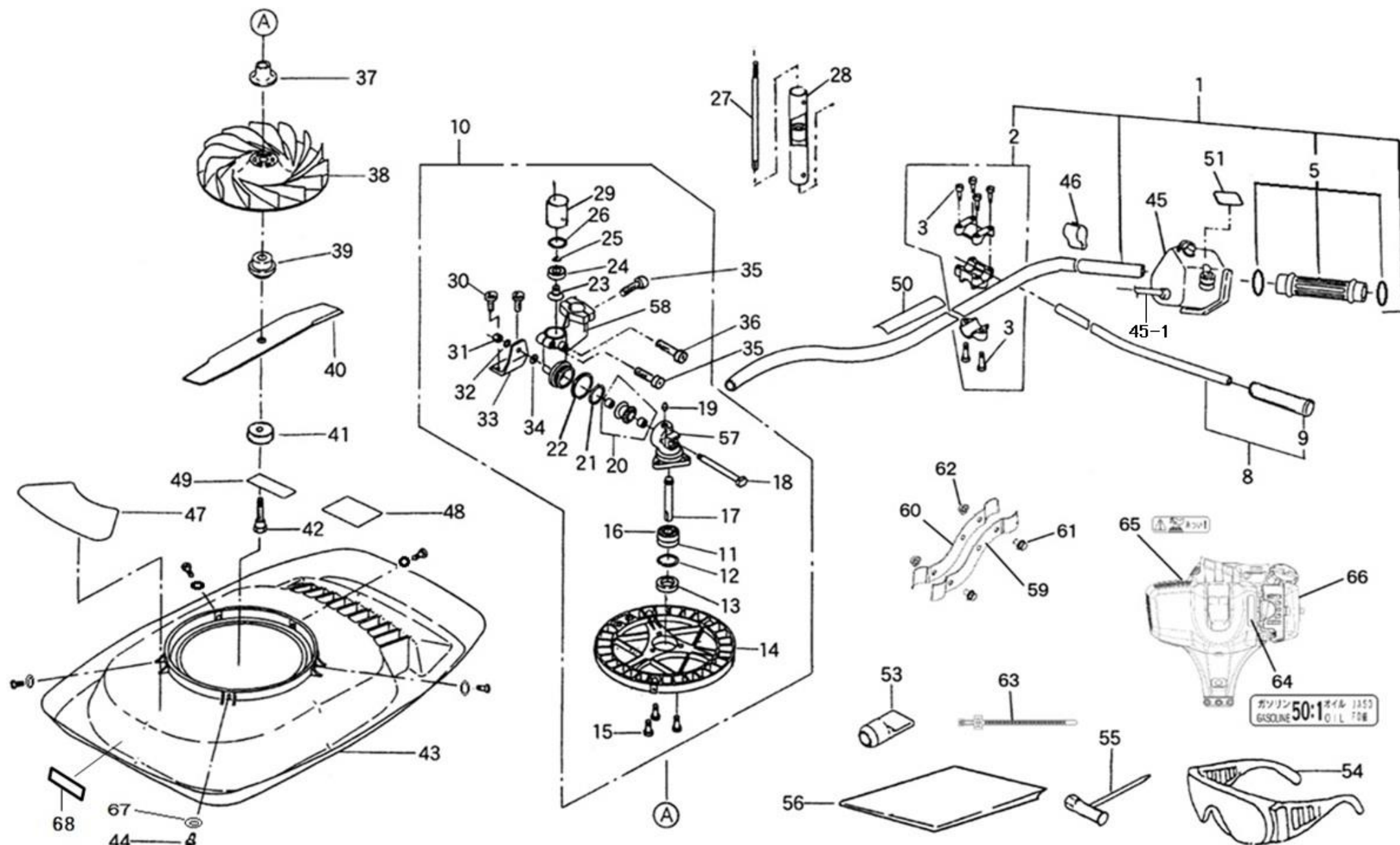
FIG 101. 本体関係
