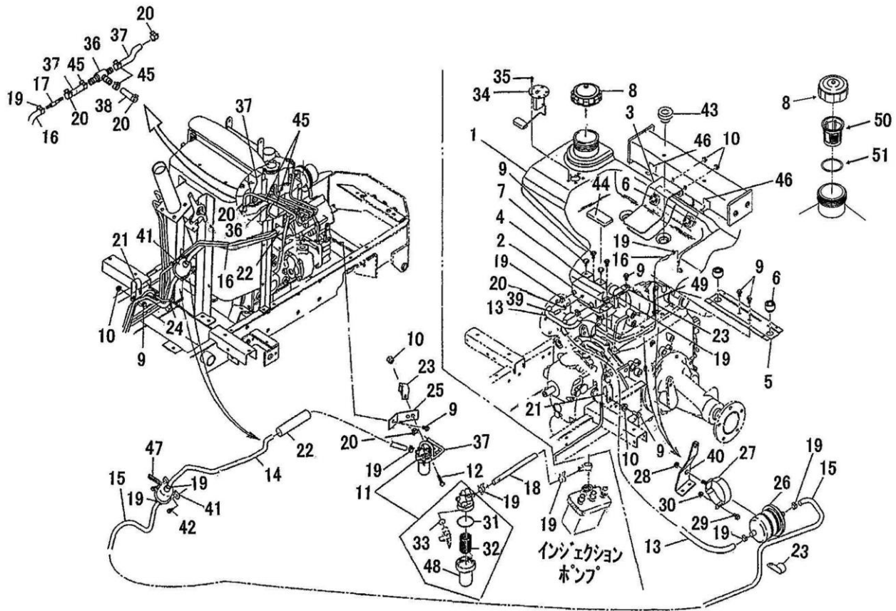
燃料タンク FUEL TANK
