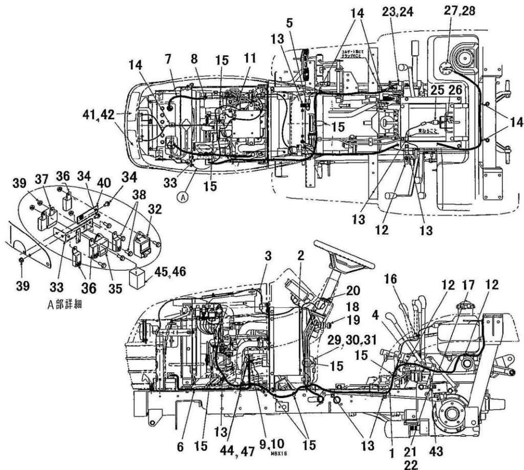
FIG.232 配線、電装品 WIRING, ELECTRICAL PARTS
