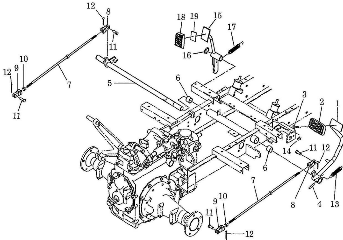
FIG.216 ペダル、ブレーキ PEDALS ; BRAKE
