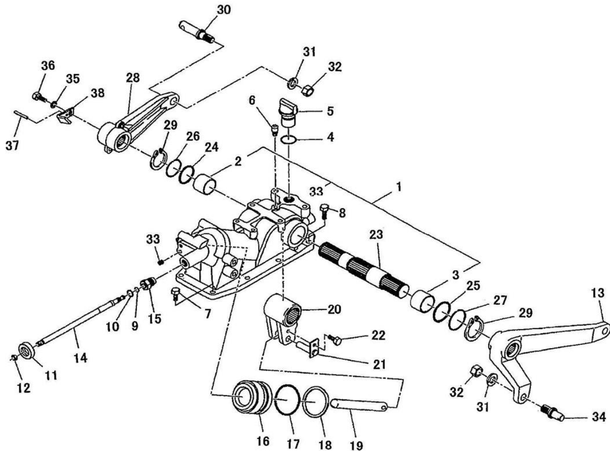
FIG.228 油圧シリンダケース HYDRAULIC CYLINDER CASE
