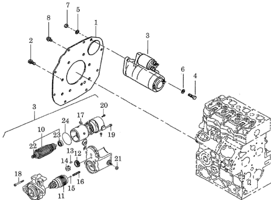
FIG.114 リヤプレート、スタータ REAR PLATE, STARTER
