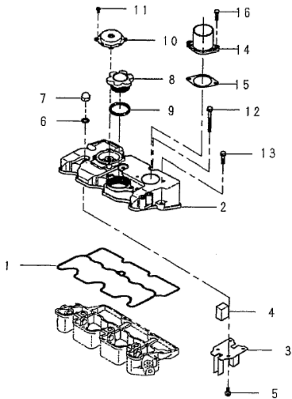
FIG.105 ヘッドカバー HEAD COVER
