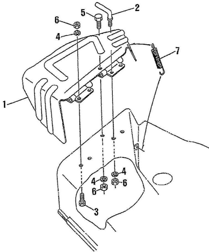
ディスチャージカバー DISCHARGE COVER
