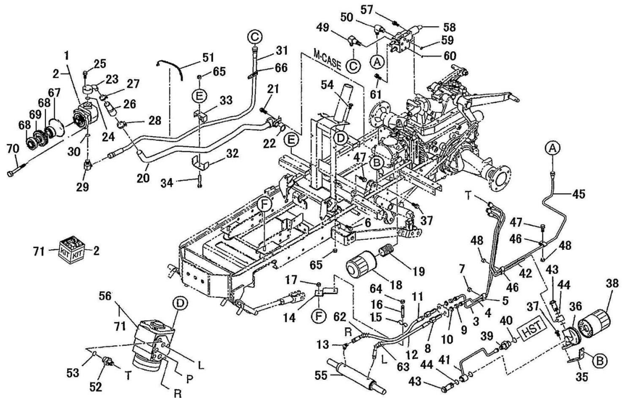
FIG.226 油圧配管 HYDRAULIC PIPNG
