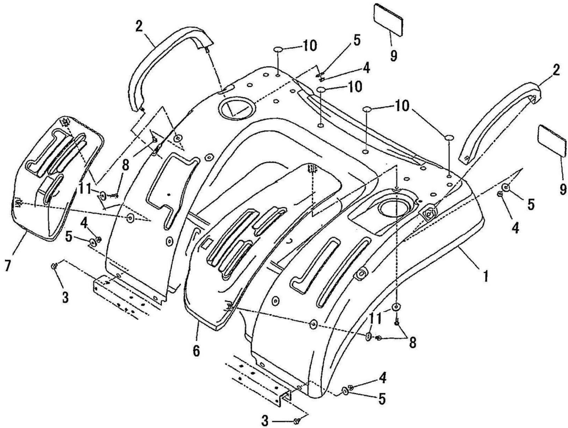
フェンダ FENDER
