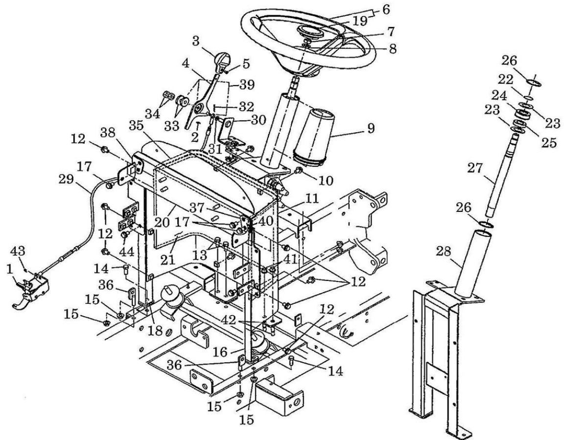
FIG.215 ステアリング STEERING
