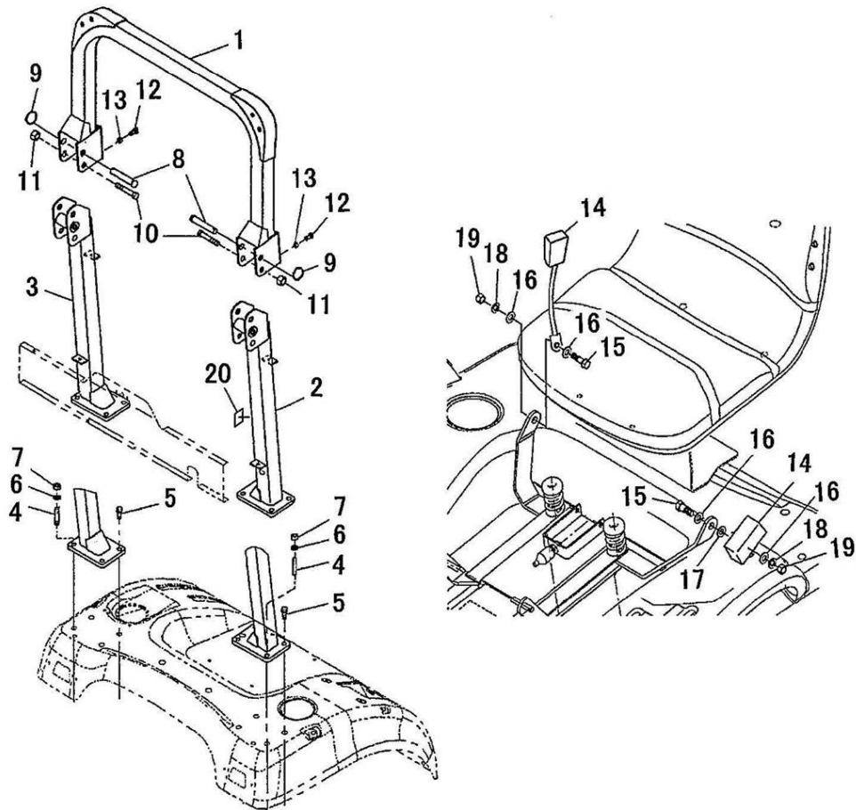
ヒョケフレーム(オプション) ROOF FRAME KIT (OPTION)
