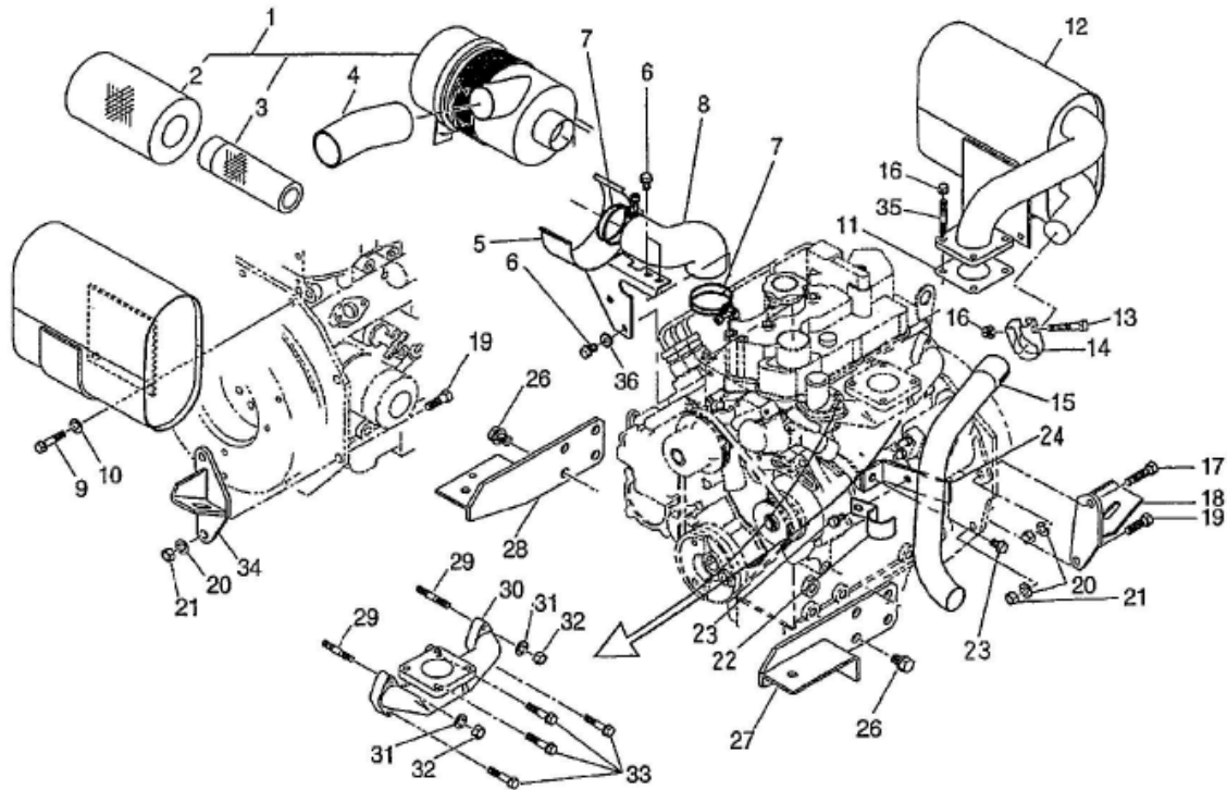
FIG.116 マフラ、エアクリーナ MUFFLER, AIR CLEANER
