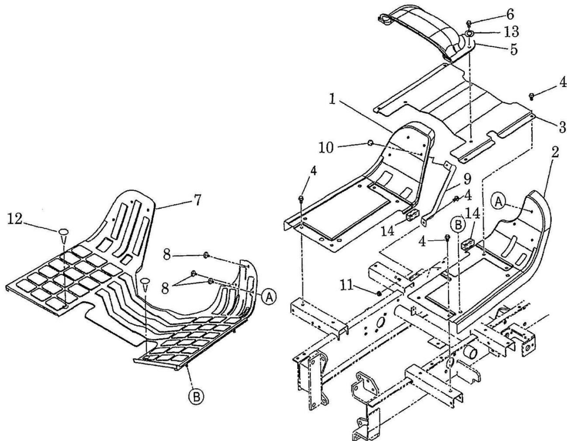
FIG.218 ステップ STEP
