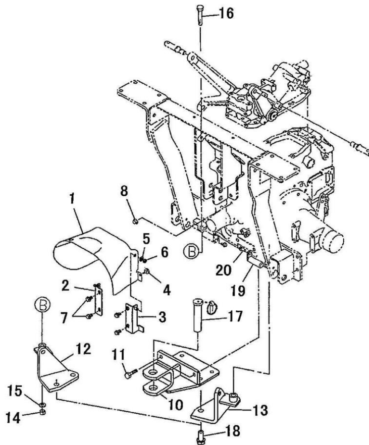
FIG.231 PTOガード&トレーラヒッチ PTO GUARD & TRAILER HITCH
