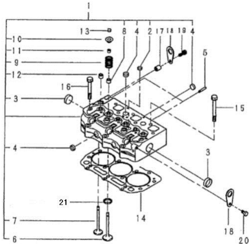
FIG.103 シリンダヘッド CYLINDER HEAD
