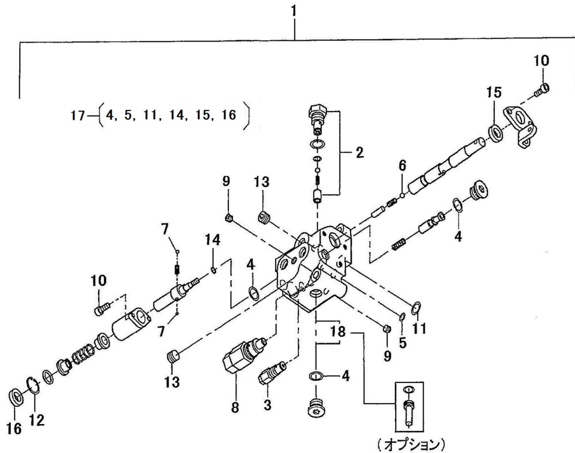
FIG.227 コントロールバルブ CONTROL VALVE
