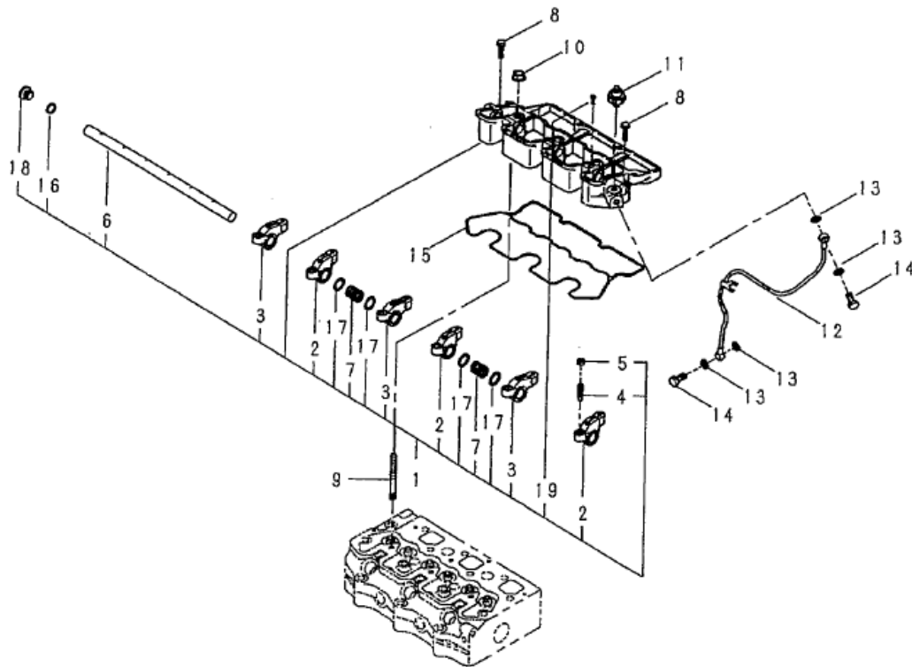
FIG.104 ロッカーアームASSY ROCKER ARM ASSY
