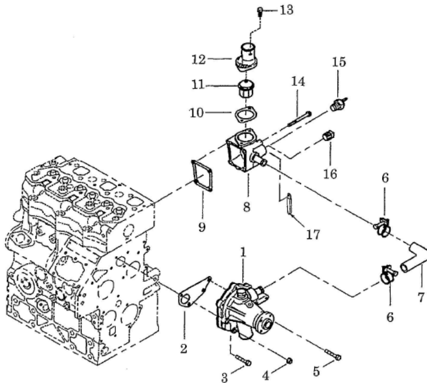
FIG.111 ウォータポンプ WATER PUMP
