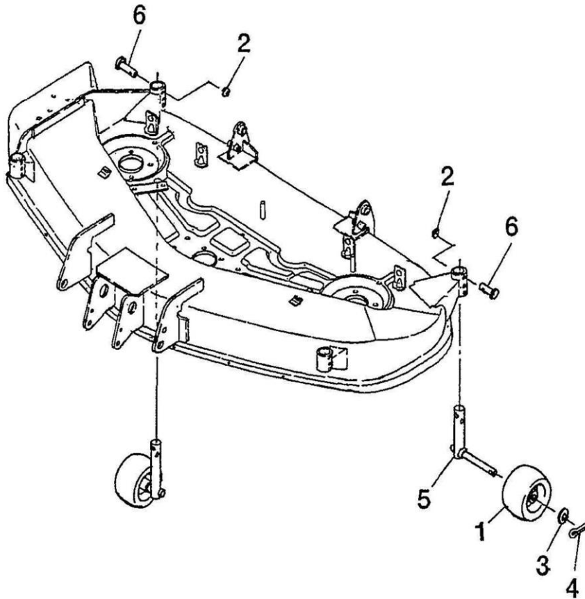
ローラ : サイド ROLLER : SIDE
