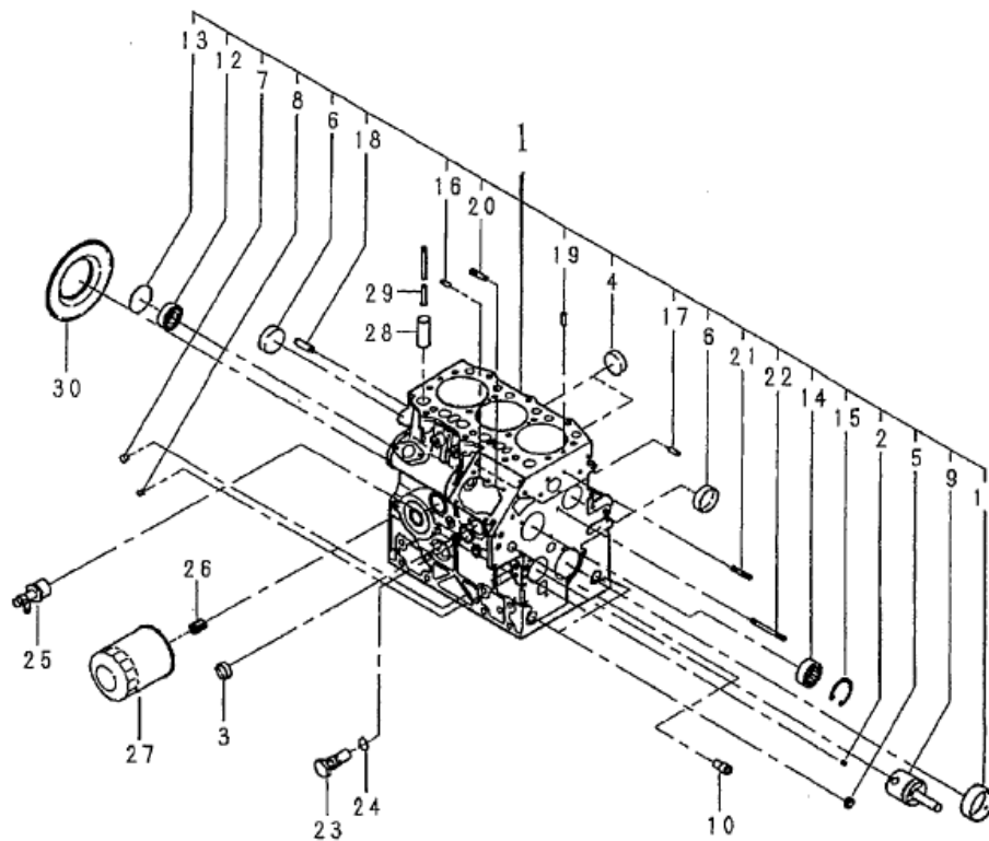
FIG.102 シリンダブロック CYLINDER BLOCK
