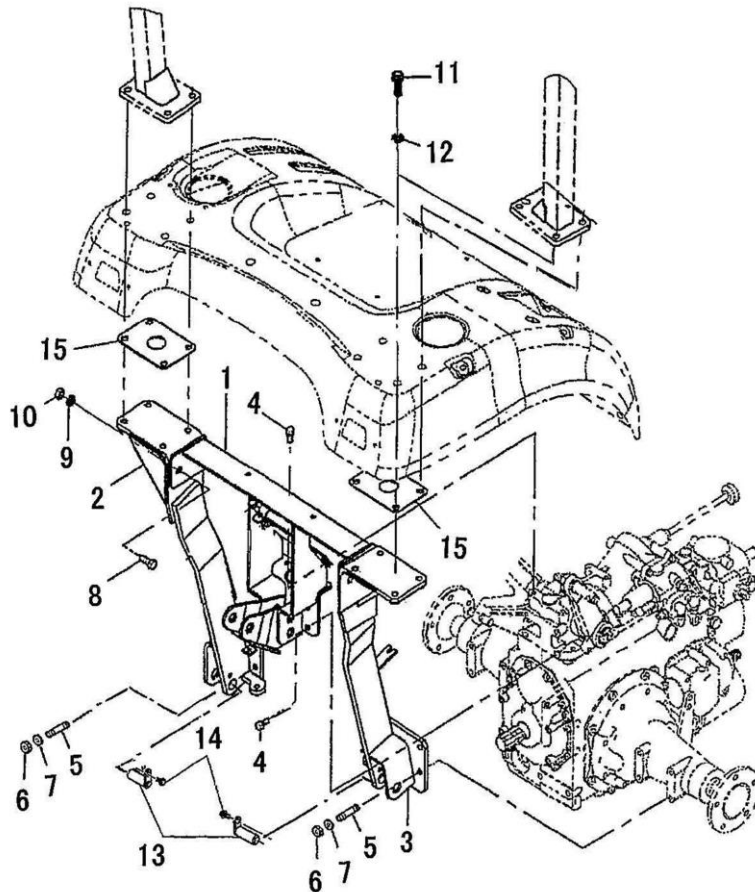
FIG.223 安全フレーム SAFETY FRAME(ROPS)
