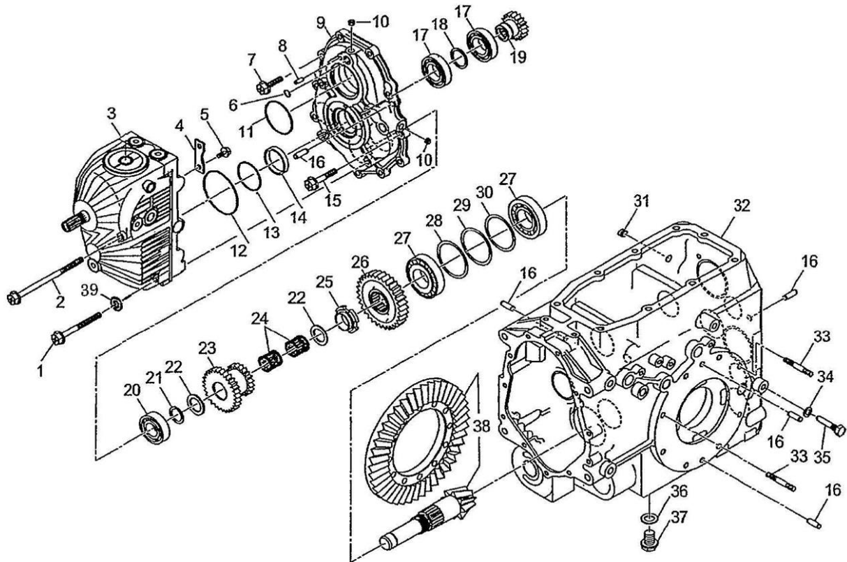
トランスミッション ; 走行 TRANSMISSION ; DRIVE
