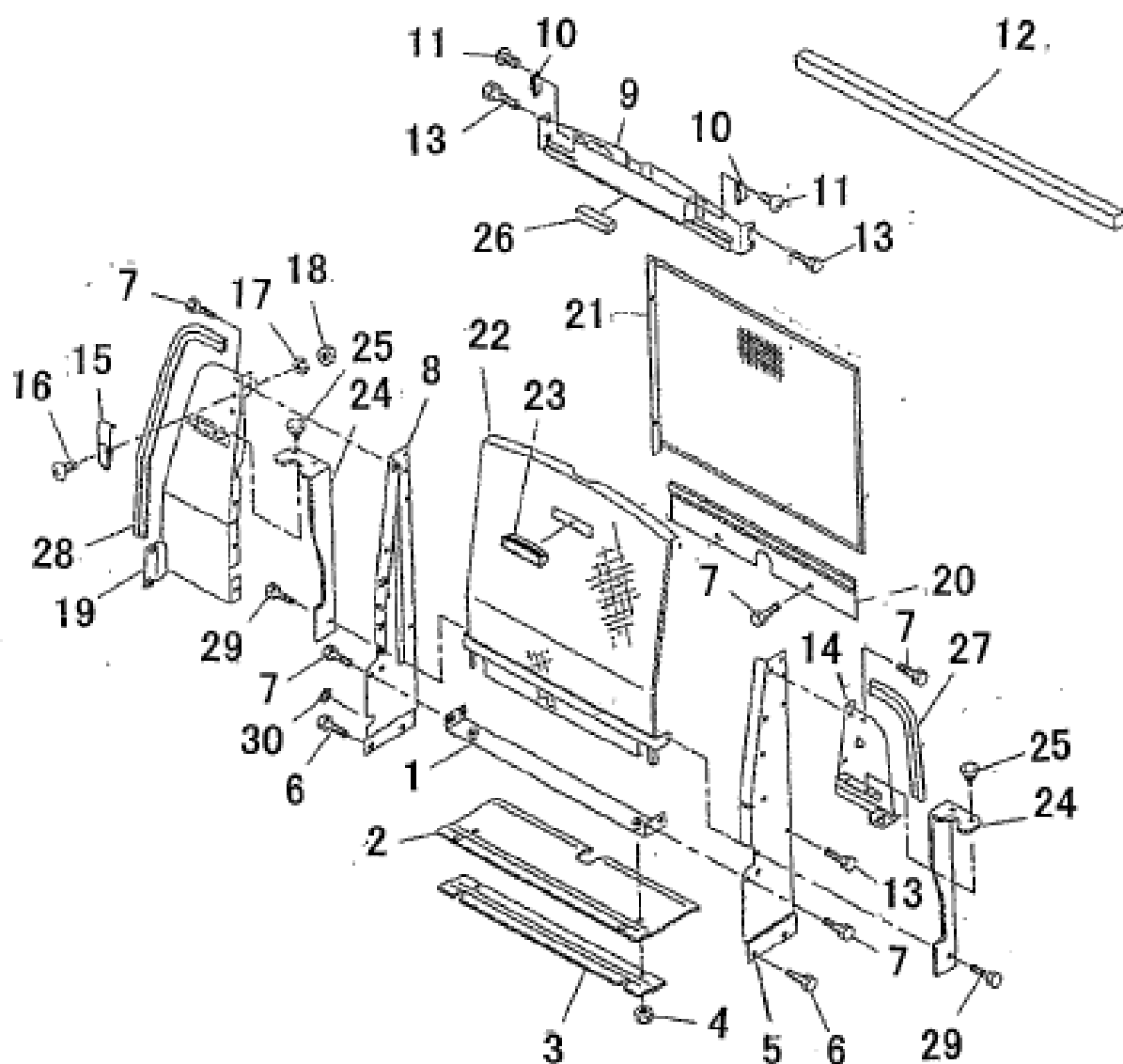
エンジンサポ o ート, シヤフウバン FIG.229 ENGINE SUPPORT、PLATE
