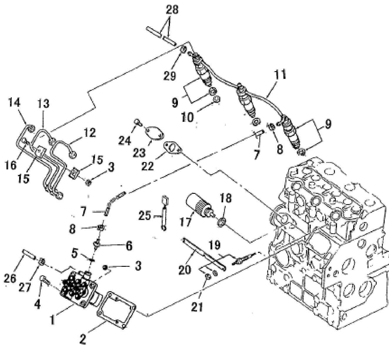
インジェクションポンプ、ライン : MC234 ティア 2 FIG.127 INJECTION PUMP, LINES : TIRE 2 MC234
