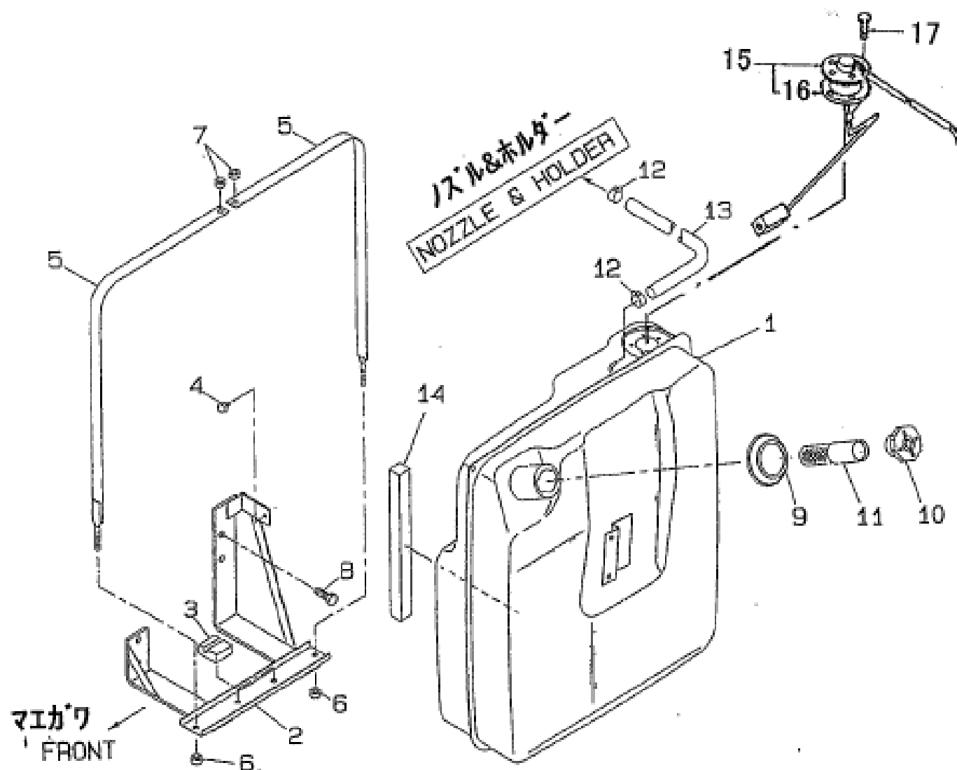
フュエルタンク FIG201 FUEL TANK
