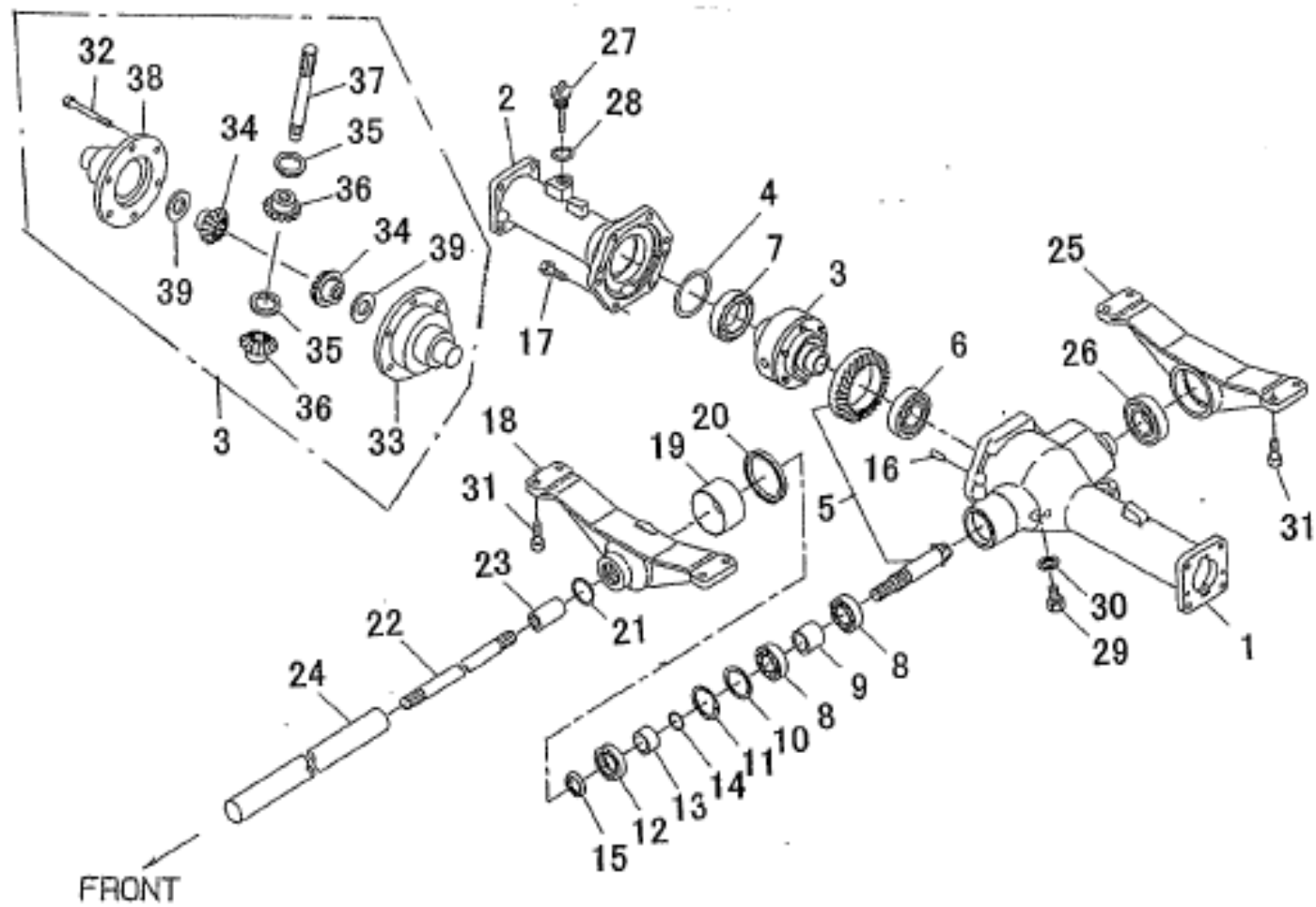
リヤアクセル ;デフ :旧部品 FIG.212 REAR AXLE , DIFFERENTIAL :CURRENT TYPE
