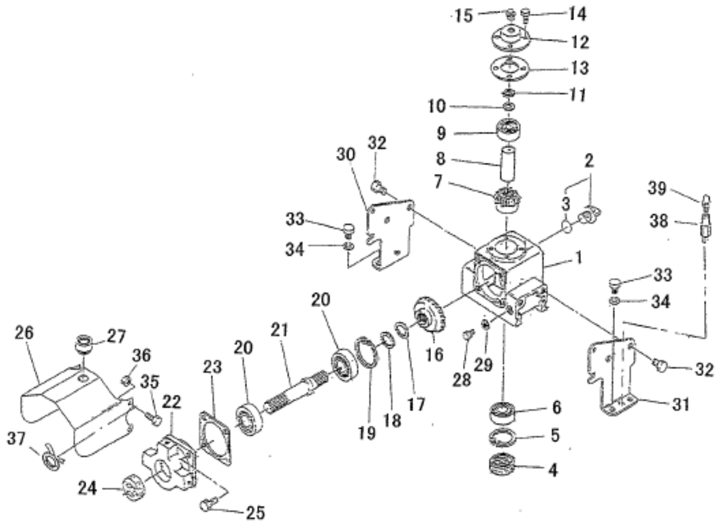
FIG. 302 GEAR BOX
