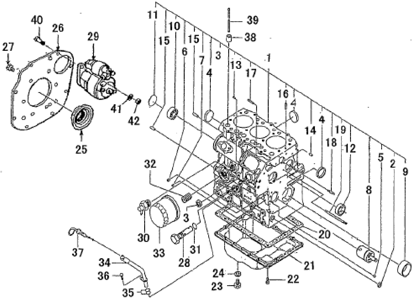
シリンダブロック :MC354 FIG.102 CYLINDER BLOCK
