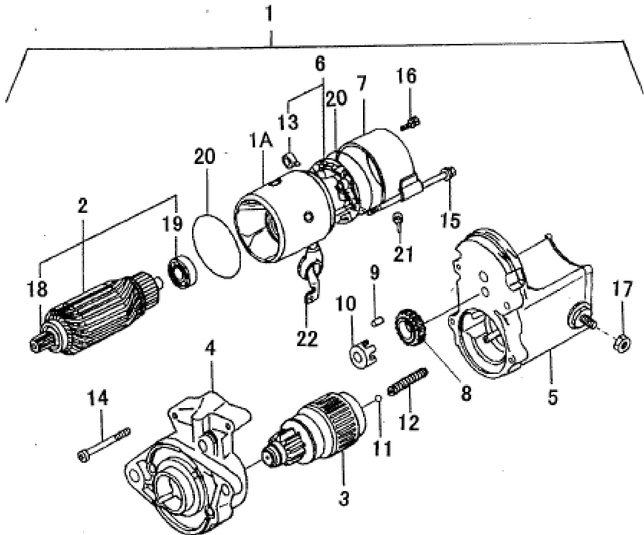
スターテイングモーター ;MC234 ティア 2 FIG.136 STARTING MOTOR ;TIRE 2 MC234
