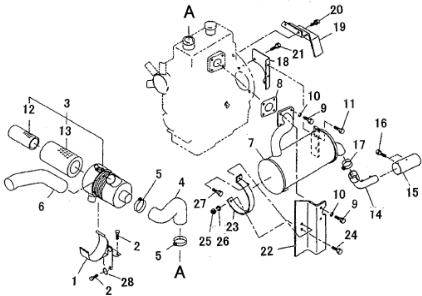
エアクリーナ、マフラ :MC234 FIG202 AIR CLEANER , MUFFER :MC234
