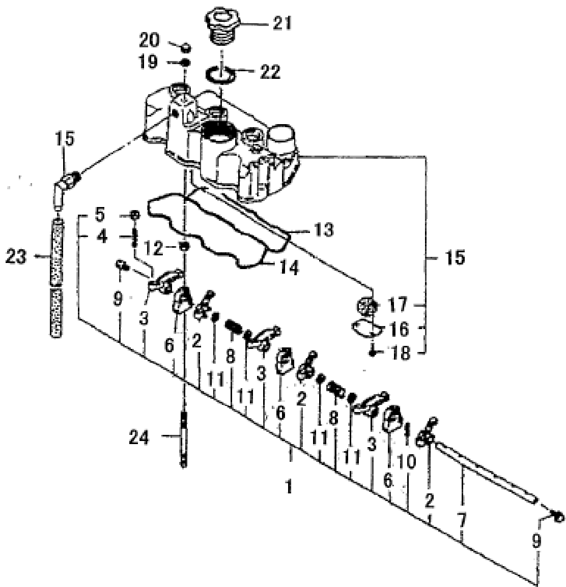
ロツカーム、ヘッドカバー MC234 :テイア 1 FIG.106 ROCKER ARM, HEAD COVER :TIRE 1
