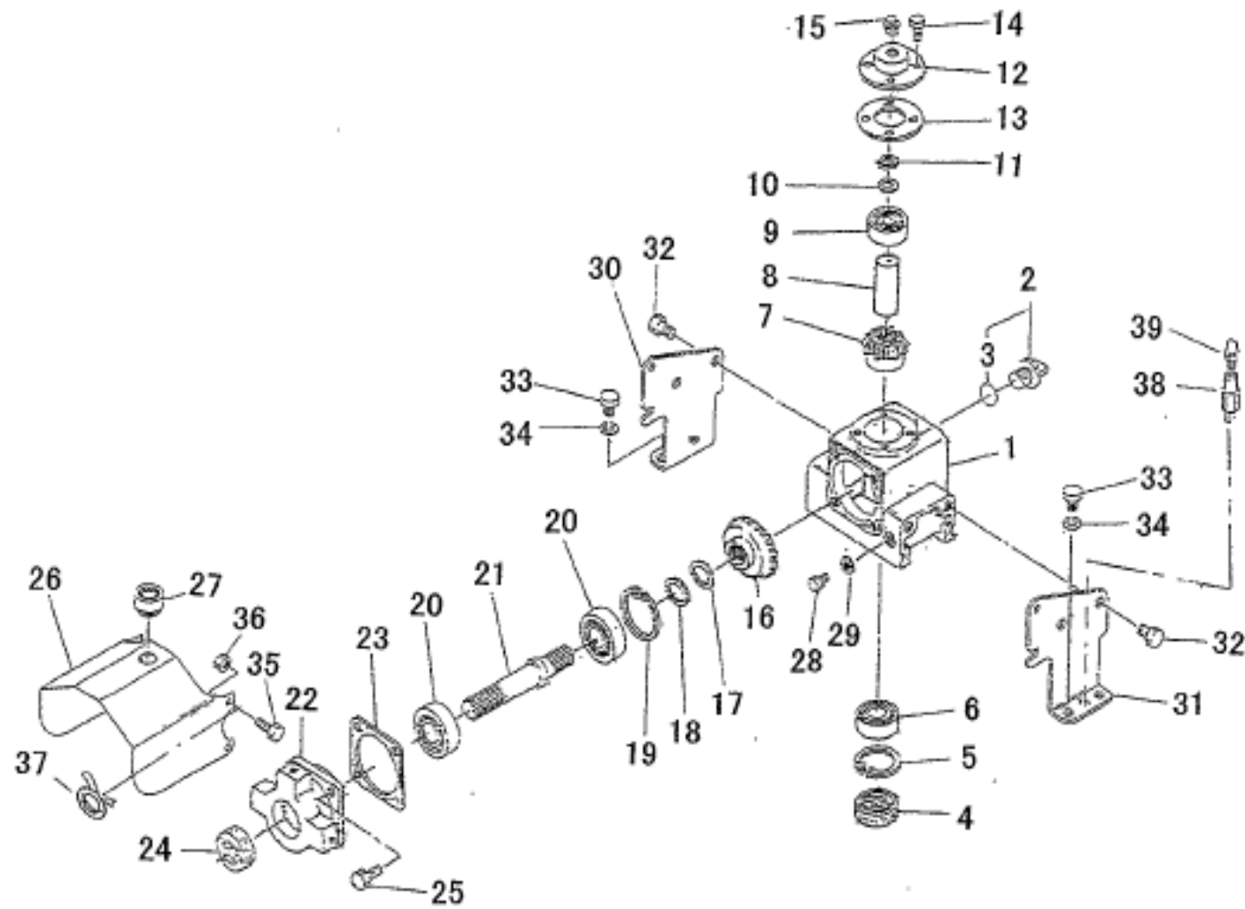
ギヤボックス FIG. 302 GEAR BOX
