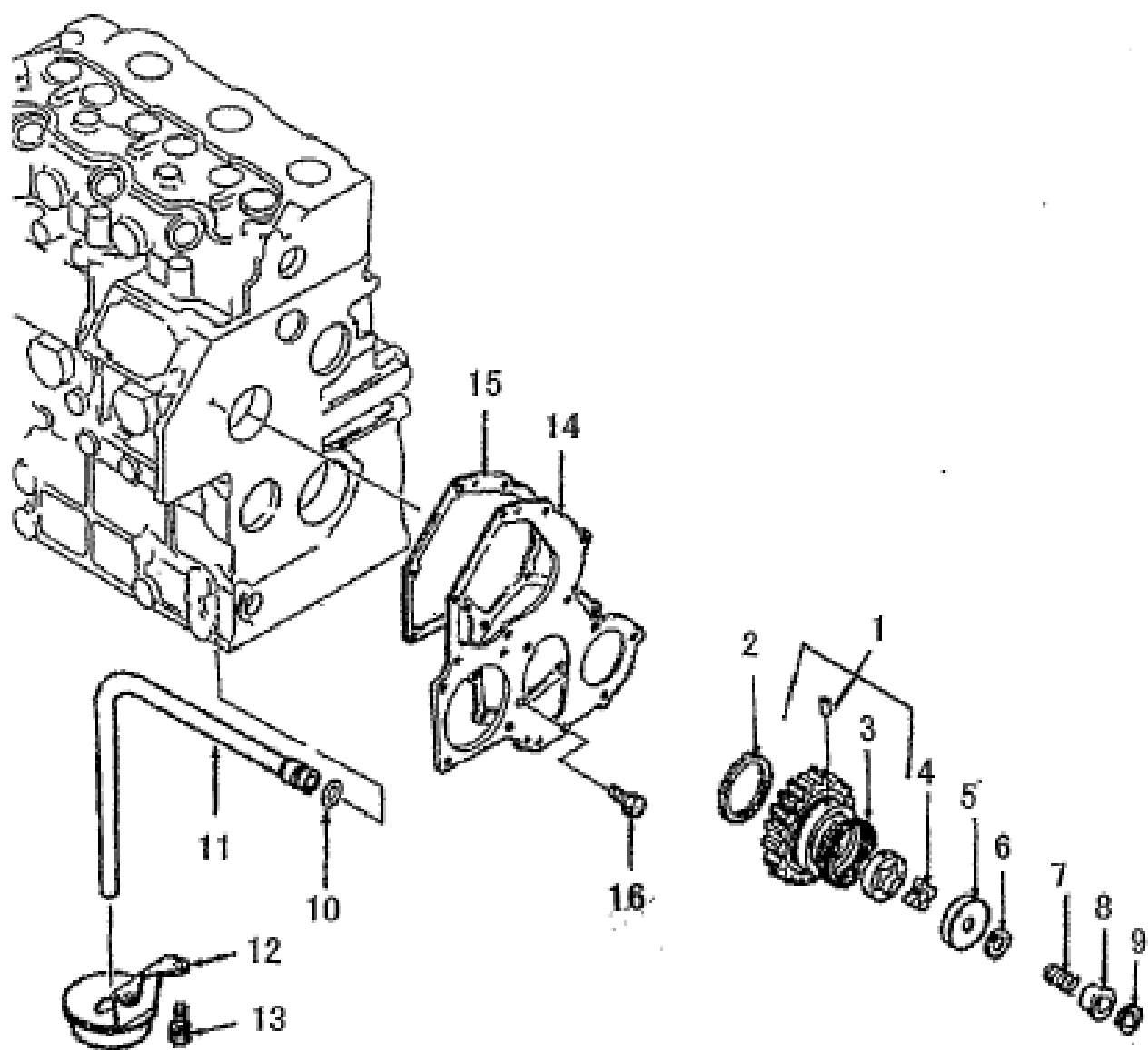
オイルポンプ FIG.118 OIL PUMP
