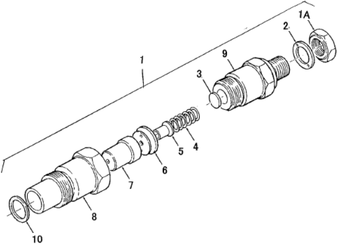
ノズル & ホルダ :MC234 FIG.130 NOZZLE, HOLDER :MC234
