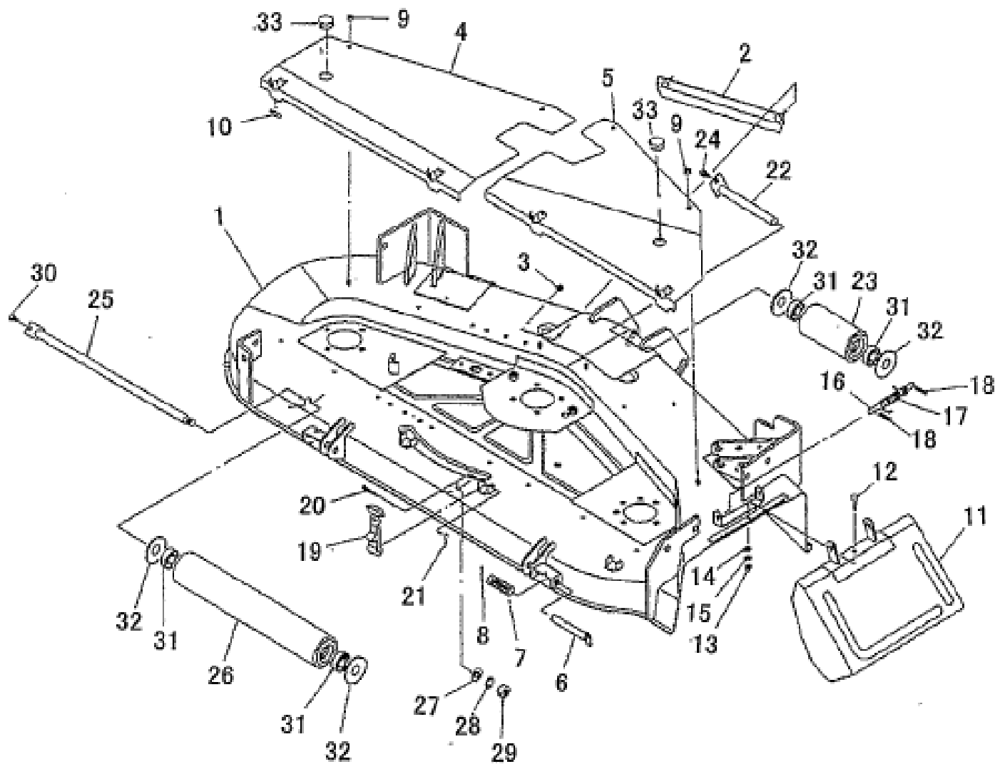
モアデツキ、カバー FIG. 304 MOWER DECK , COVER
