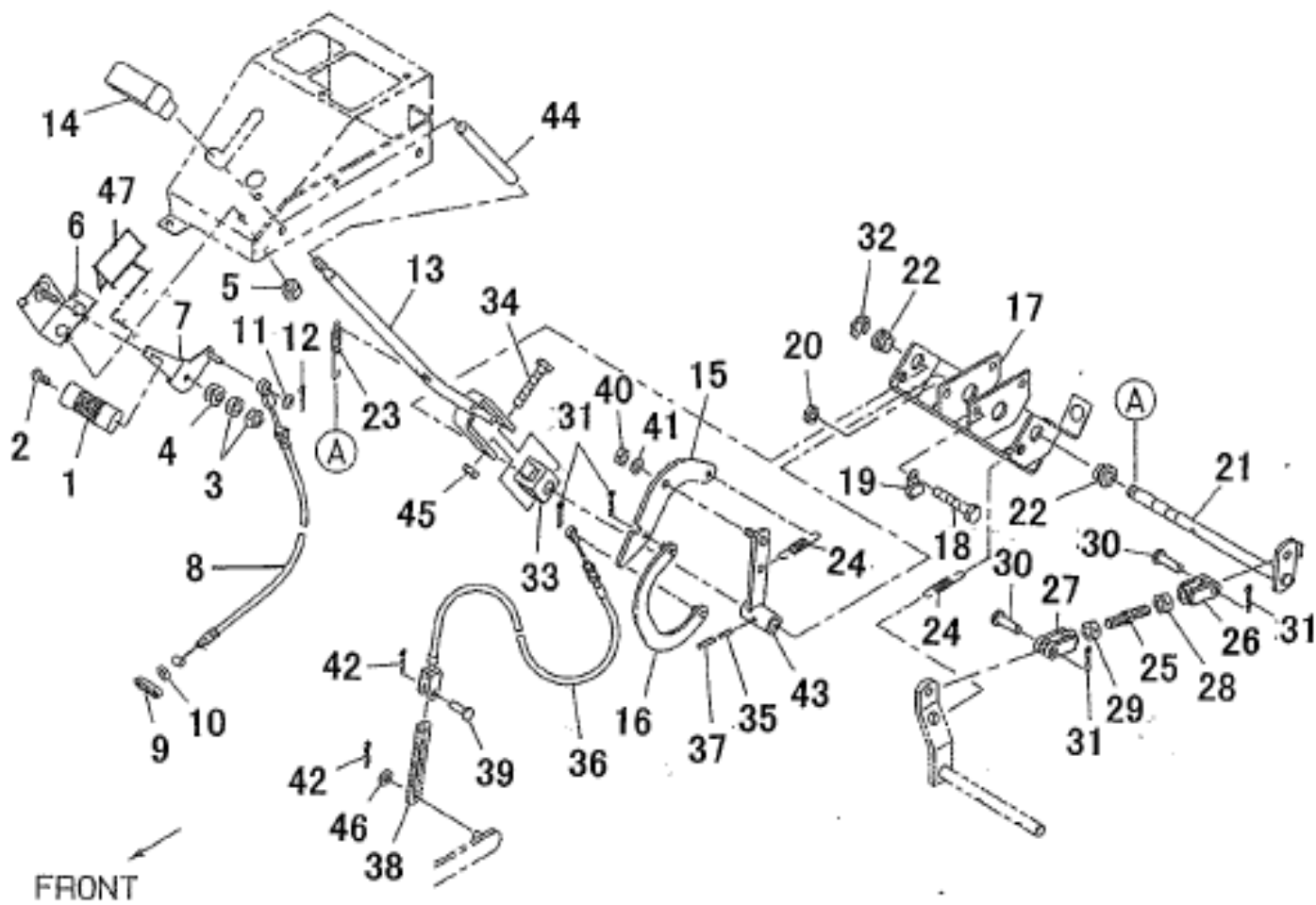
アクセルコントロール & チェンジレバー FIG.216 ACCELERATOR CONTROLS & CHANGE LEVER
