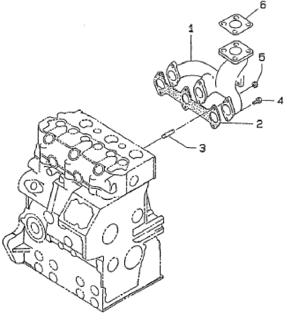
エキゾーストマニフォールド FIG.134 EXHAUST MANIFOLD
