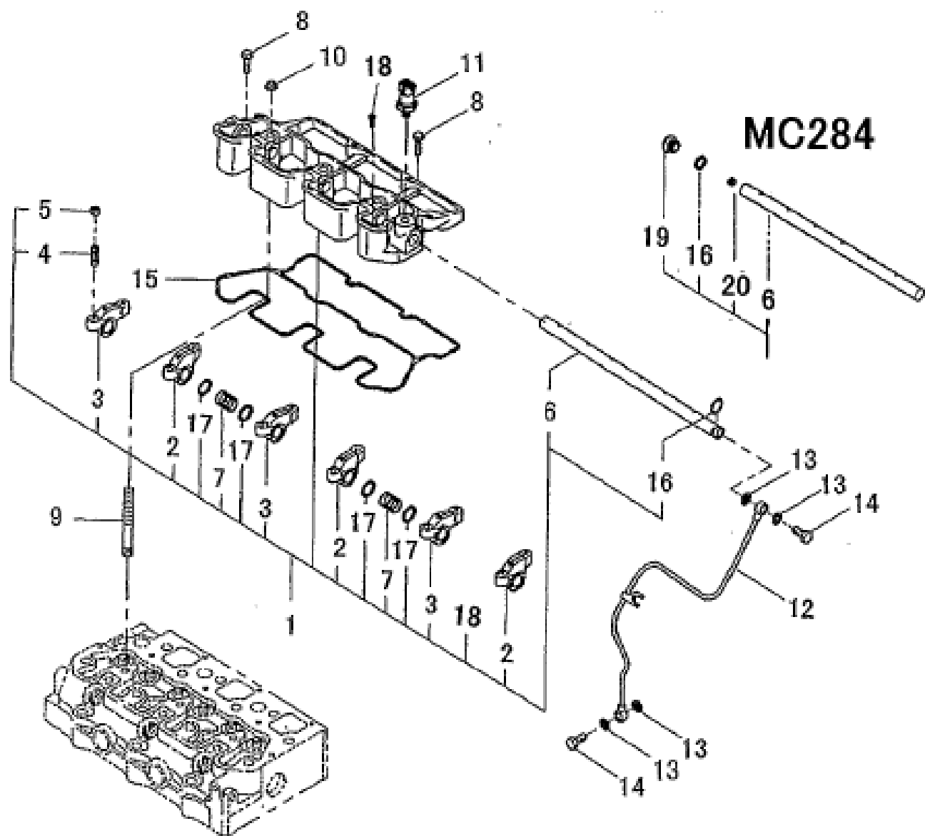
ロツカーアーム MC284/MC354 :ティア 2 FIG.109 ROCKER ARM MC284/MC354 :TIRE 2
