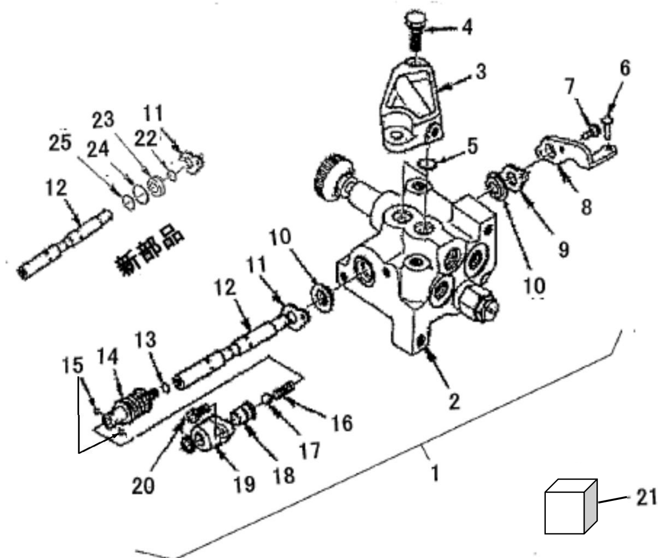
コントロールバルブ ASSY FIG.222 CONTROL VALVE ASSY
