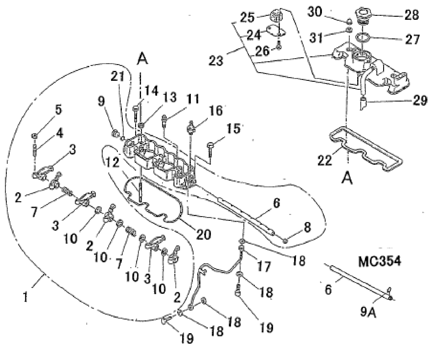
ロツカーム、ヘッドカバー MC284/MC354 :ティア 1 FIG.107 ROCKER ARM, HEAD COVER :TIRE 1
