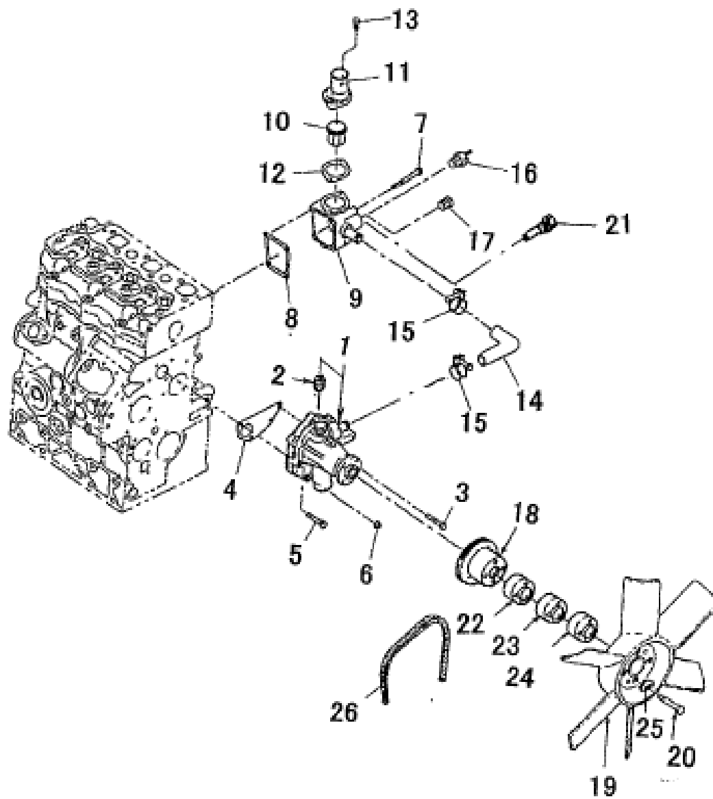
ウオータポンプ : MC234 ティア 2 FIG.123 WATER PUMP : MC234 TIRE 2
