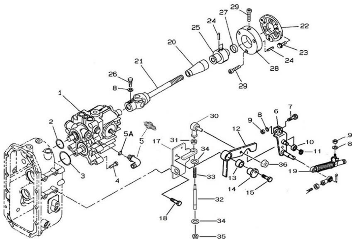
FIG.221 H.S.T DRIVE HSTドライブ
