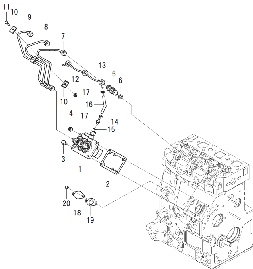
インジェクションポンプ、インジェクター、インジェクションパイプ
