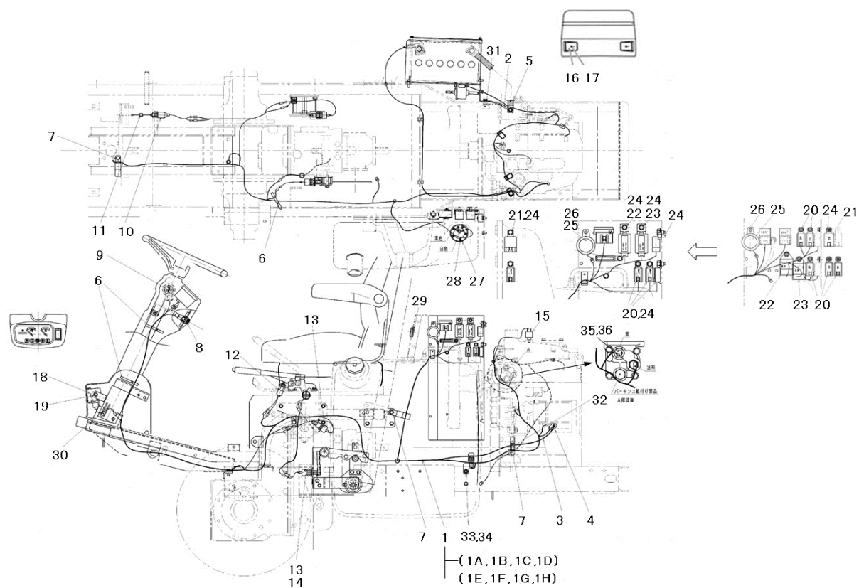
FIG.230 WIRE HARNESS ワイヤハーネス
