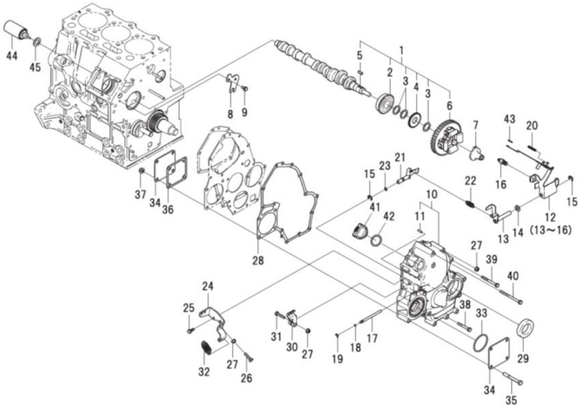
カムシャフト, タイミングギアケース
