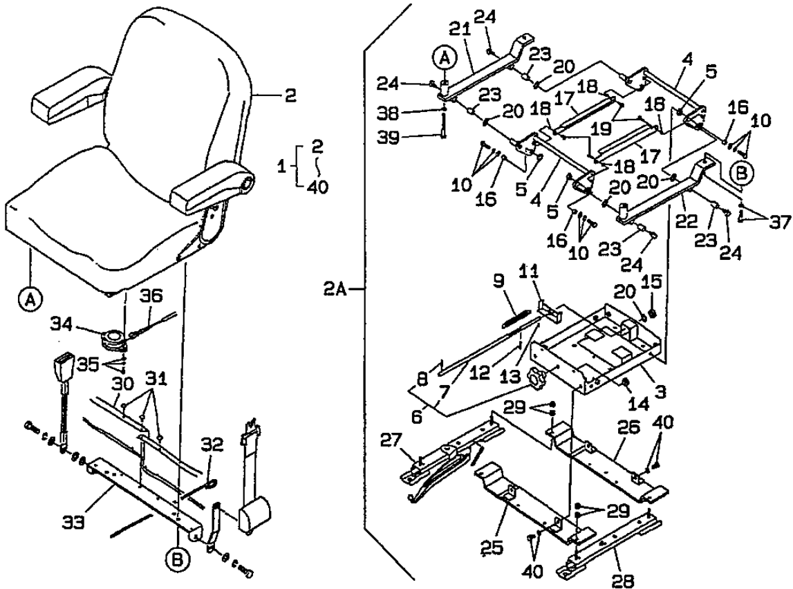
FIG.223A SEAT シート
