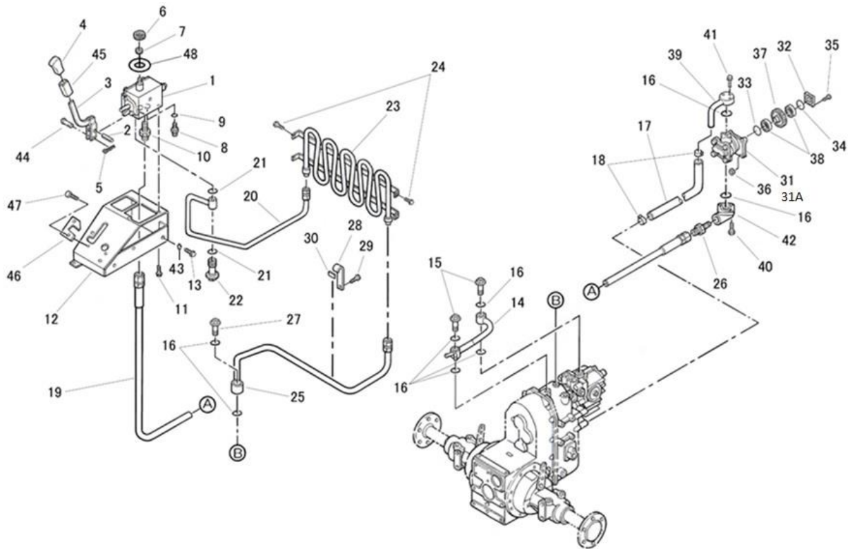
FIG.219 CONTROL VALVE コントロールバルブ
