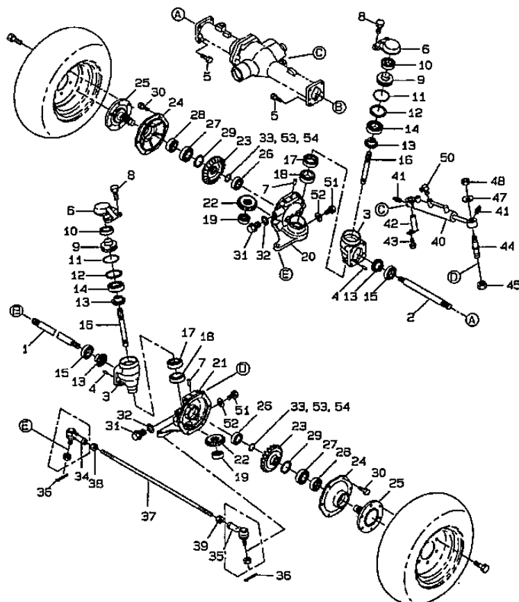
リアアクスル、ホイールシャフト
