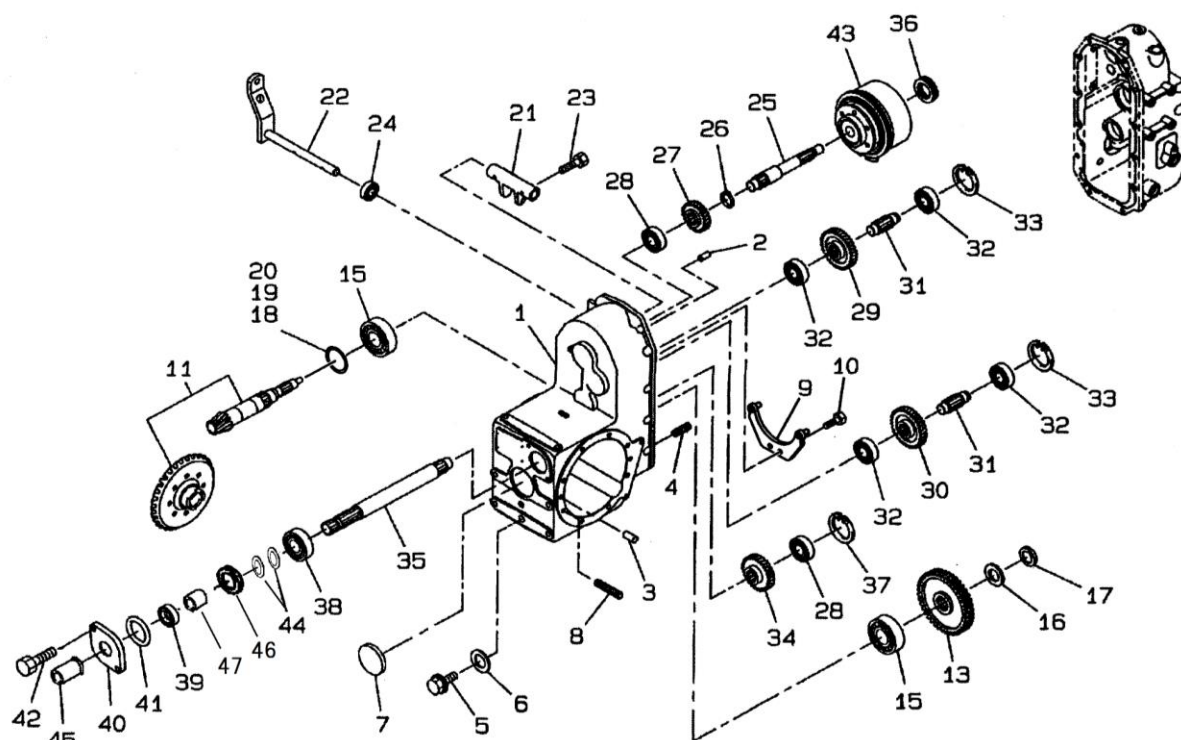
FIG.207 TRANSMISSION , DRIVE PINION トランスミッション, ドライブピニオン
