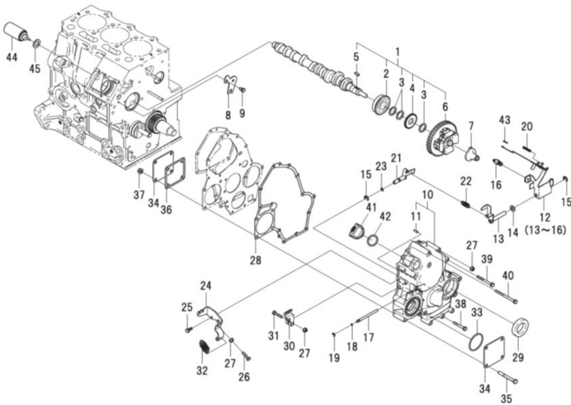
FIG.108 CAMSHAFT, TIMING GEAR CASE カムシャフト, タイミングギアケース
