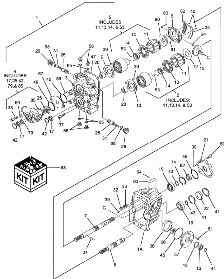
FIG.221A HST ASSEMBLY HSTアッセンブリ
