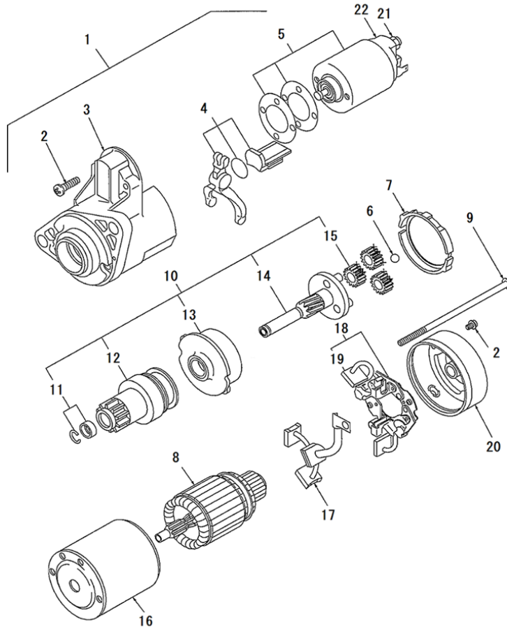
スターティングモーター
