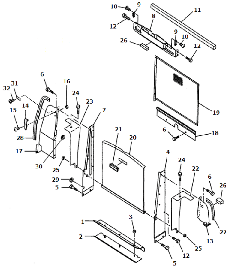
FIG.224 ENGINE SUPPORT エンジンサポート
