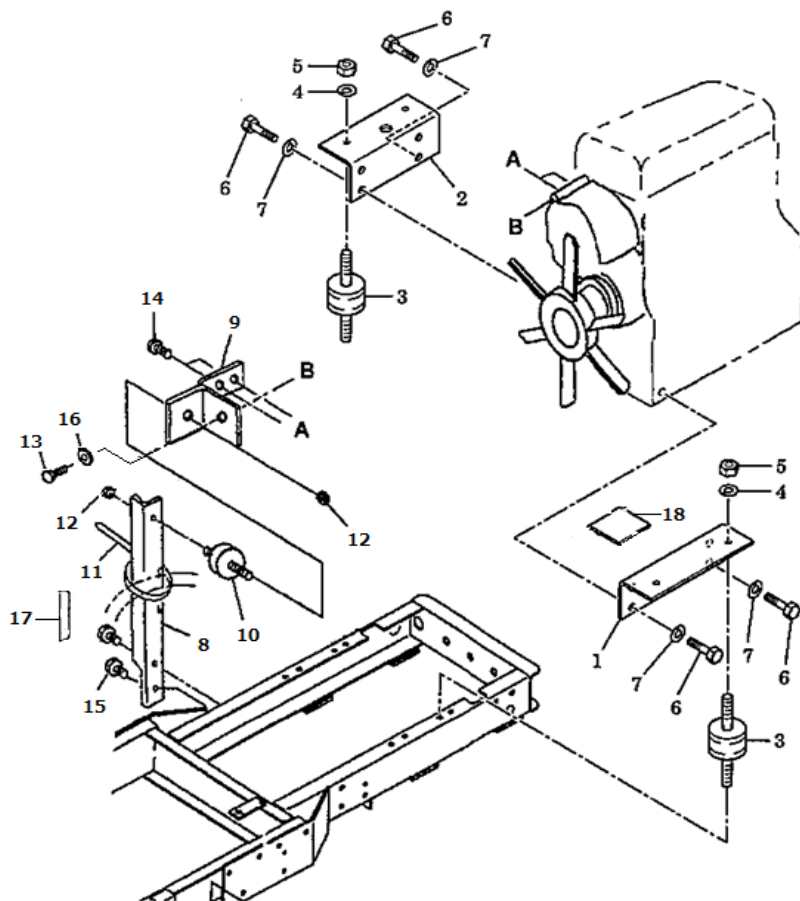
エンジンサポート
