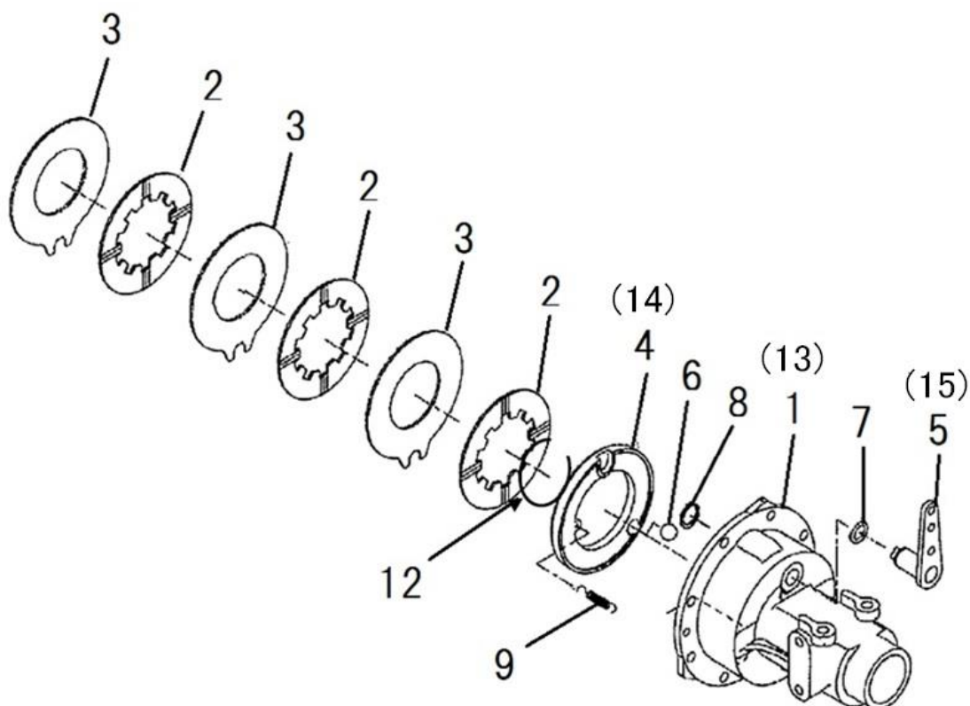
227 BRAKE ASSEMBLY ブレーキアッセンブリ
