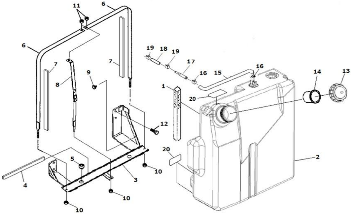
フュエルタンク
