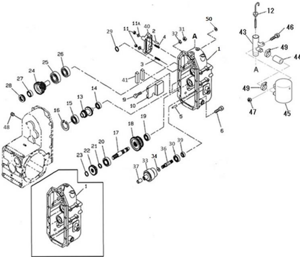
FIG.205 TRANSMISSION, GEARS トランスミッション, ギヤ
