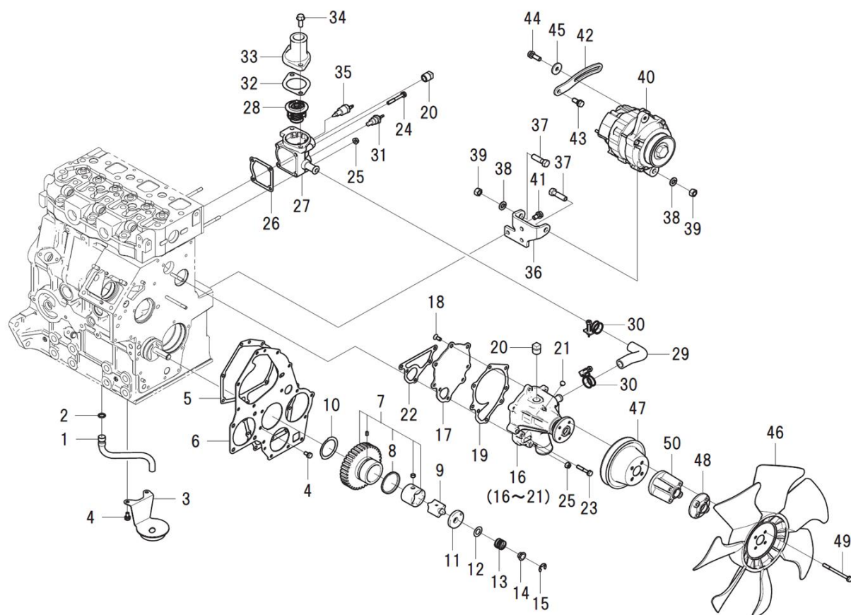
FIG.107 WATER PUMP, THERMOSTAT CASE, ALTERNATOR ウォーターポンプ, サーモスタットケース, オルターネーター
