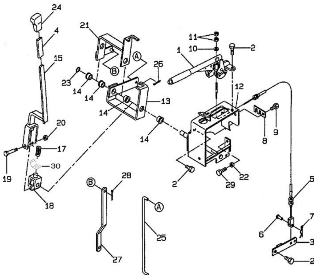
220 PARKING BRAKE, RANGE LE パーキングブレーキ レンジレバー
