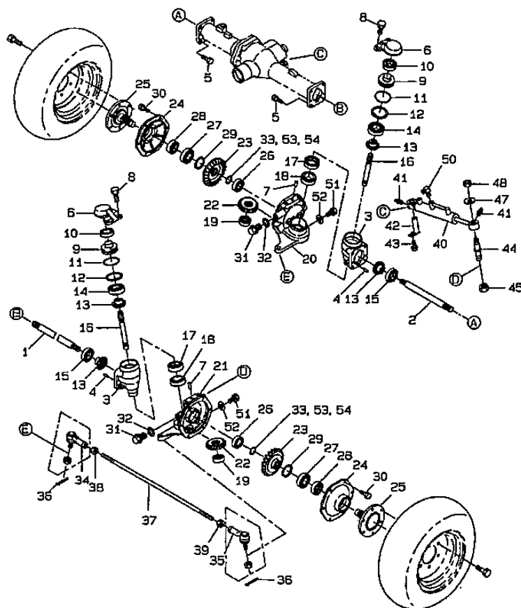
FIG.212 REAR AXLE , WHEEL SHAFT リヤアクスル, ホイルシャフト
