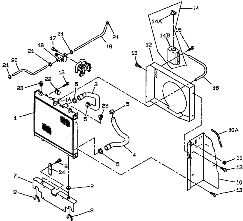
FIG.222 RADIATOR ラジエータ
