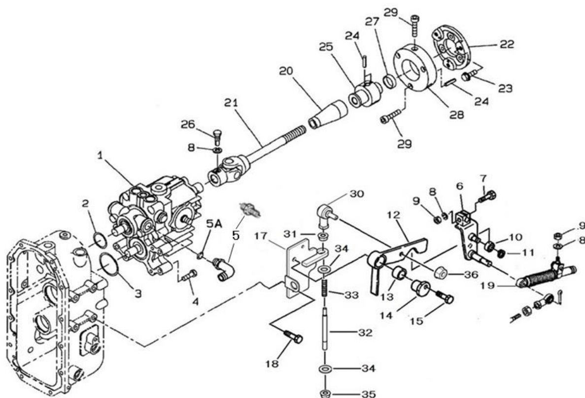
FIG.221 H.S.T DRIVE HSTドライブ
