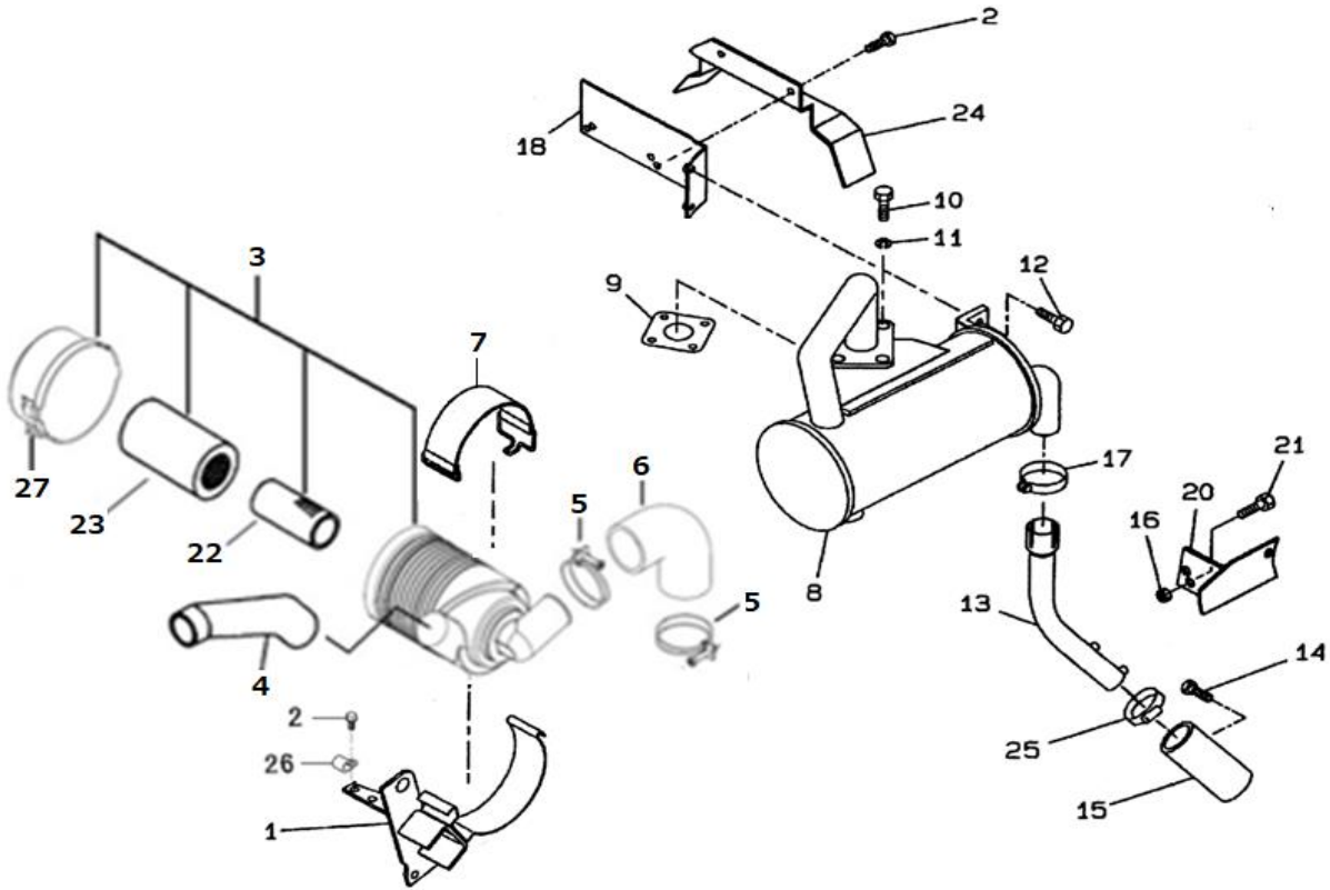
FIG.204 AIR CLEANER , MUFFLER エアクリーナ, マフラ
