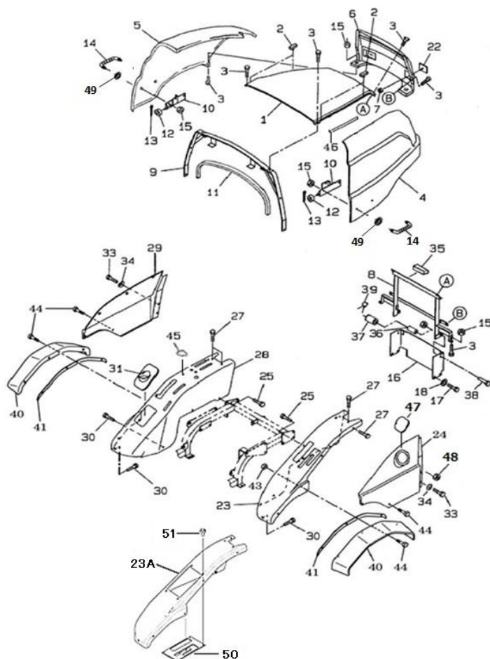
FIG.217 BONNET, FENDER ボンネット, フェンダ
