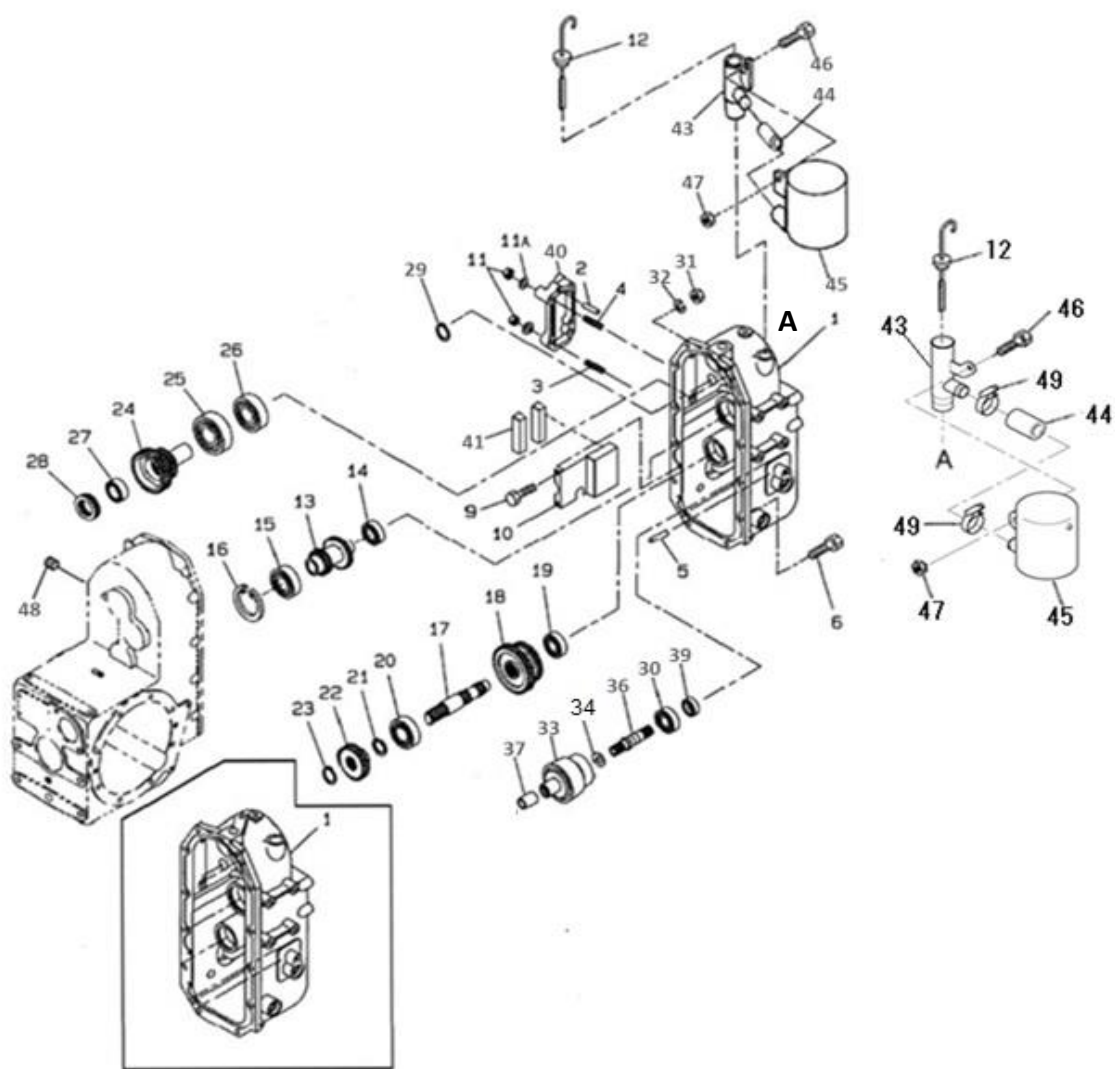
FIG.204 トランсмッション・ギヤ TRANSMISSION・GEARS
