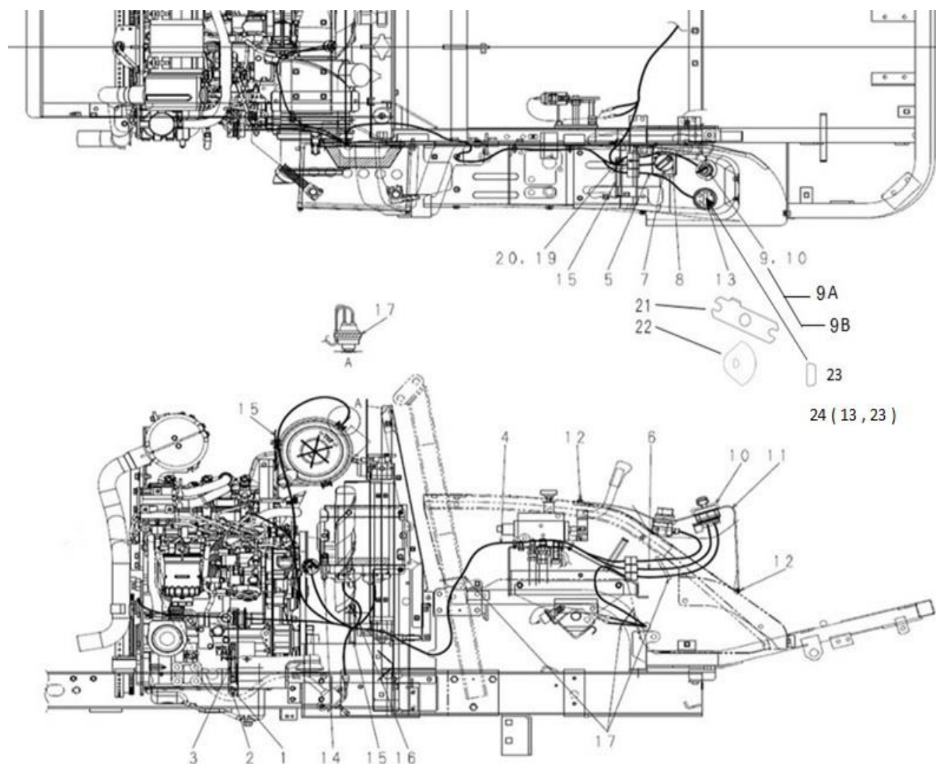
FIG.231 ワイヤハーネス WIRE HARNESS
