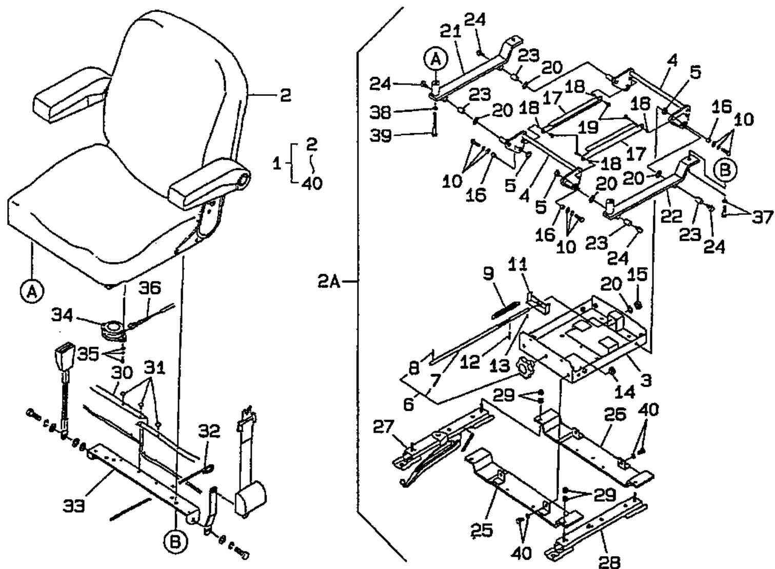
シート SEAT FIG.223A
