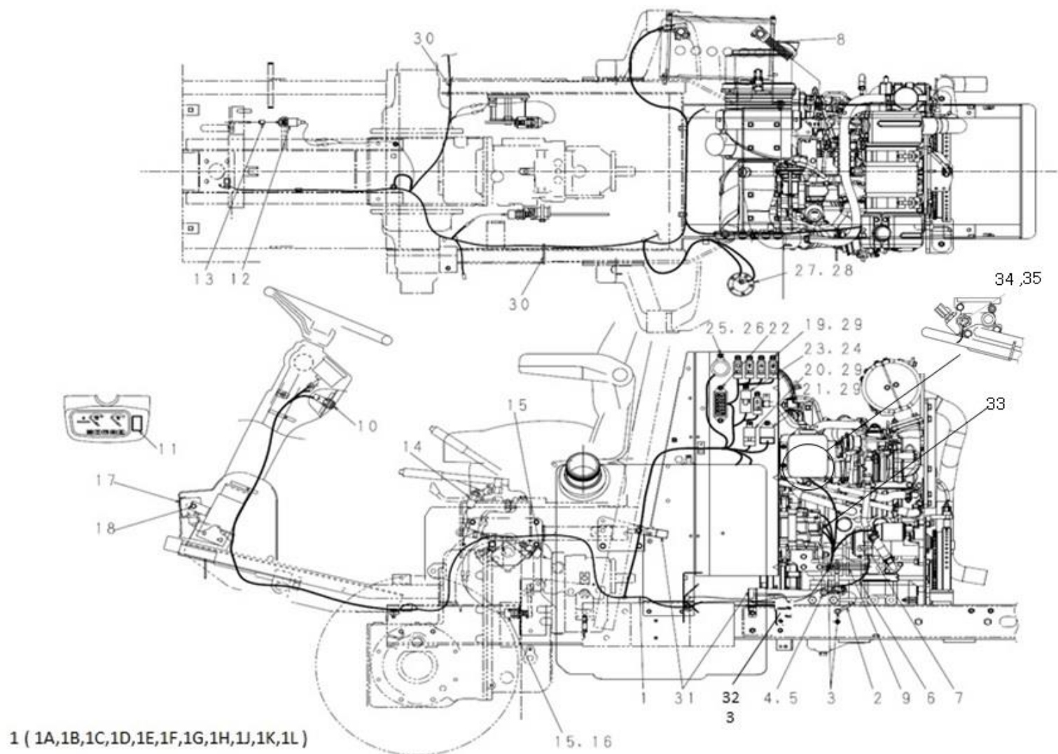
FIG.230 ワイヤハーネス WIRE HARNESS
