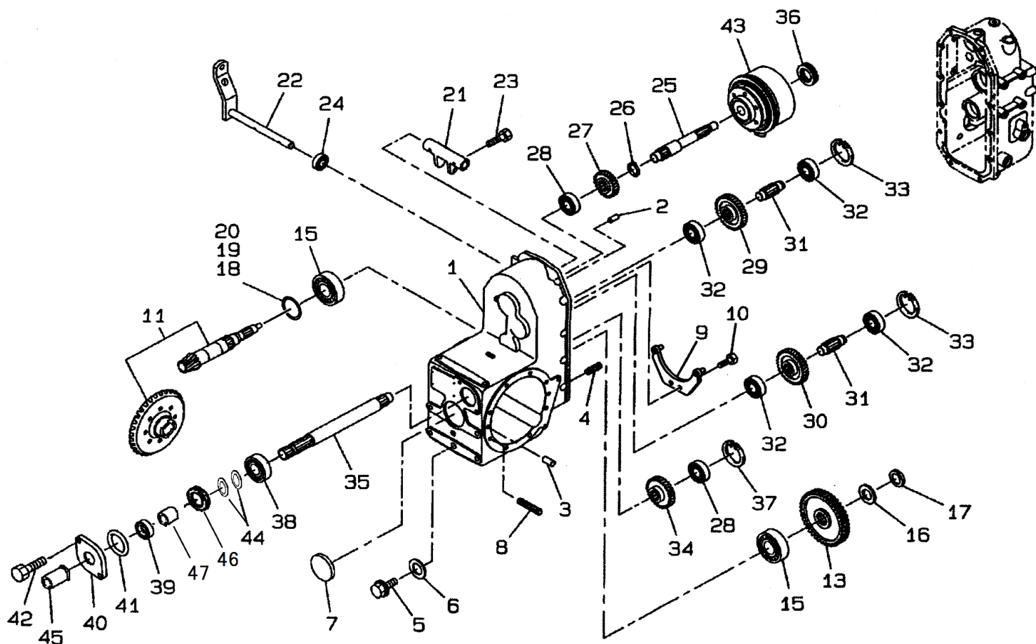
FIG.207 トランсмッション、ドライブピニオン TRANSMISSION, DRIVE PINION
