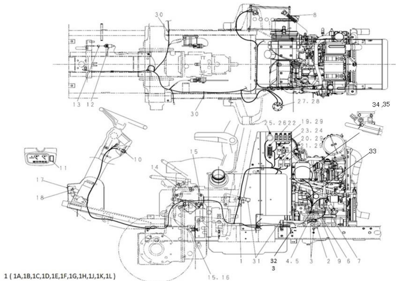
FIG.230 ワイヤハーネス WIRE HARNESS
