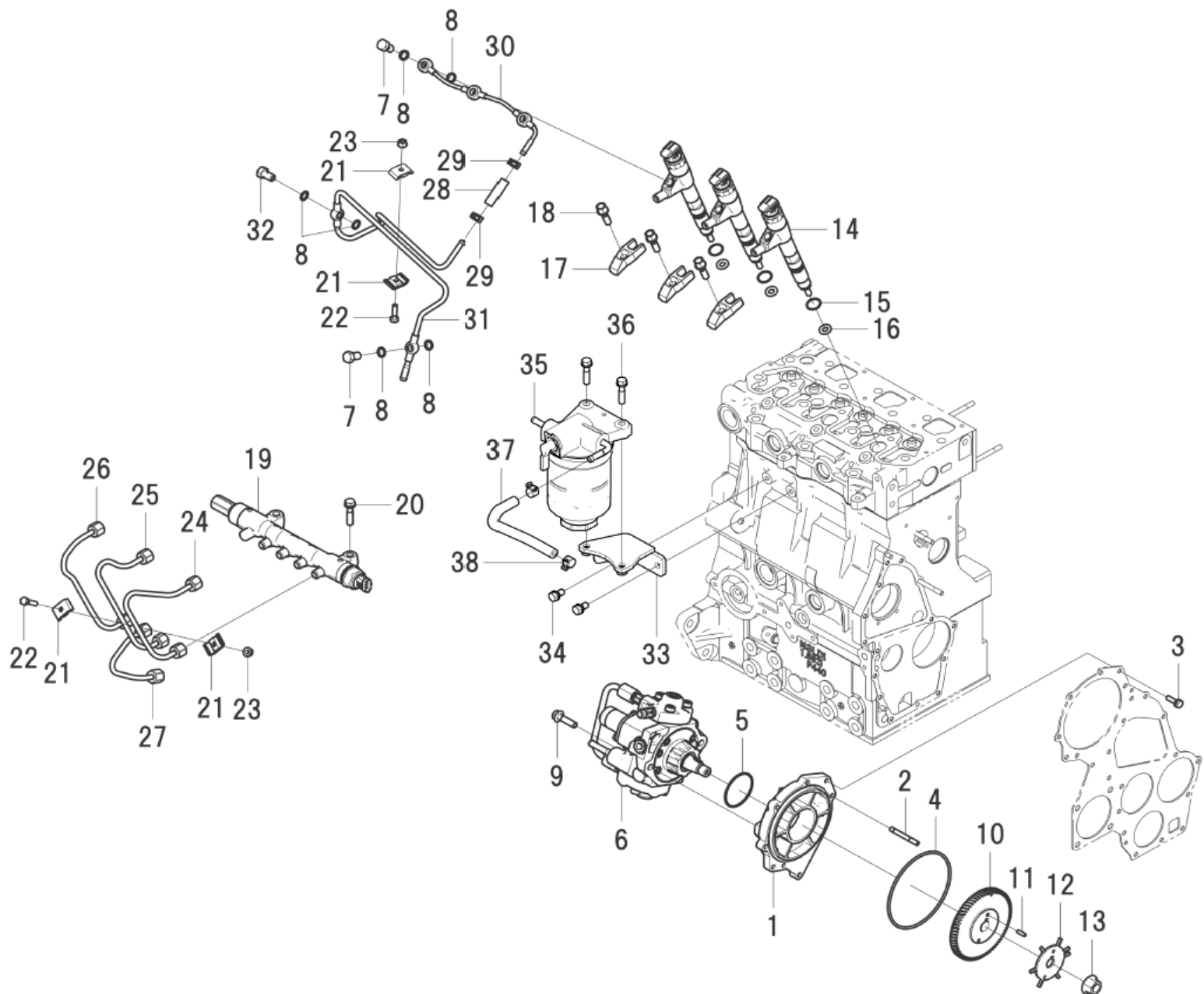
インジェクションポンプ、インジェクター、インジェクションパイプ
