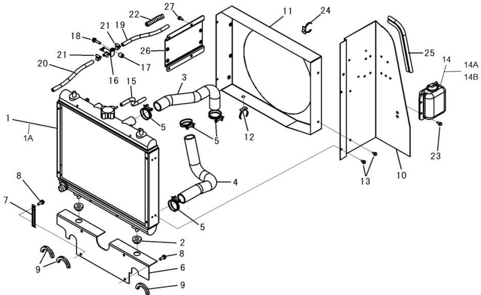
ラジエータ FIG.222 RADIATOR
