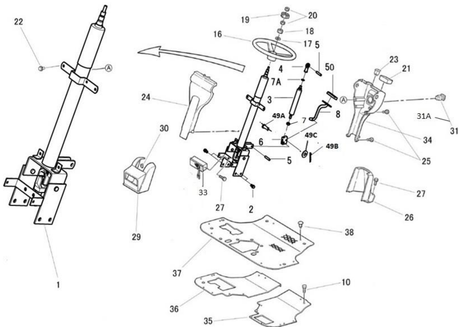
ステアリング FIG.209 STEERING COLUMN & OPERATOR'S DECK
