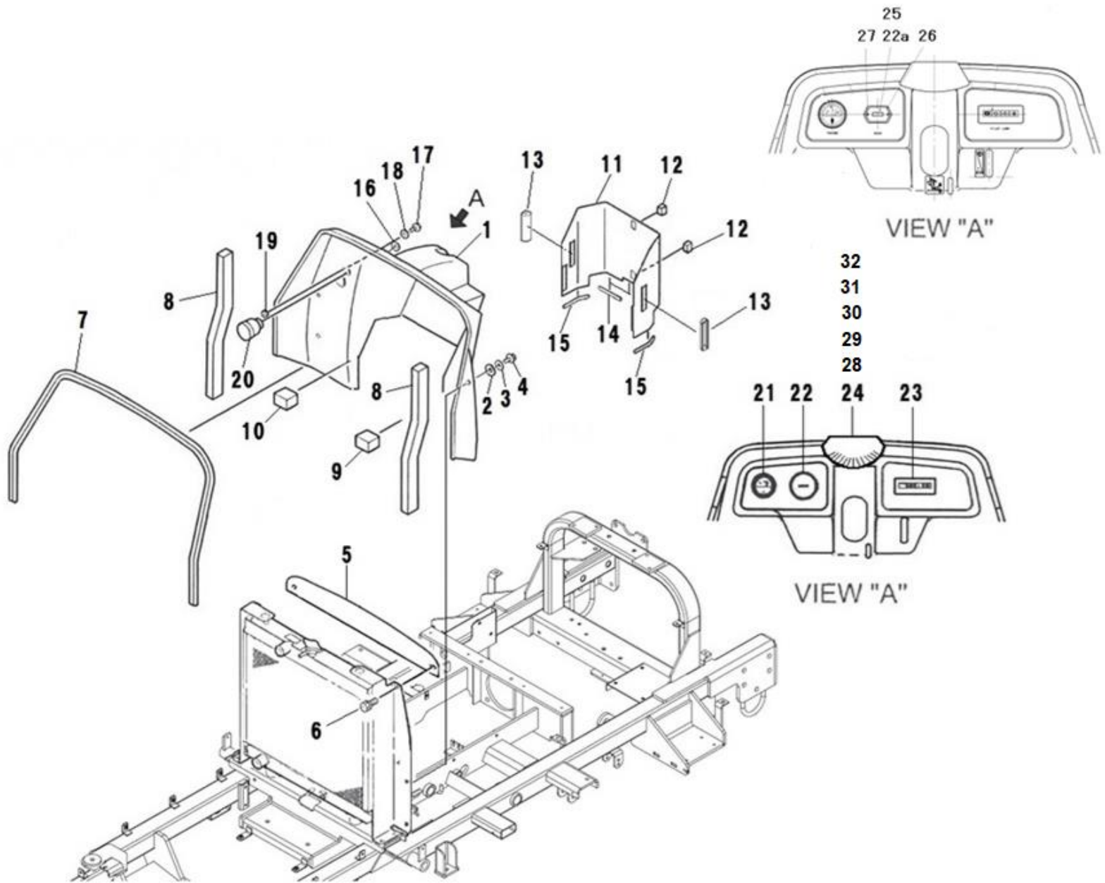
FIG.212 DASHBOARD ダッシュボード
