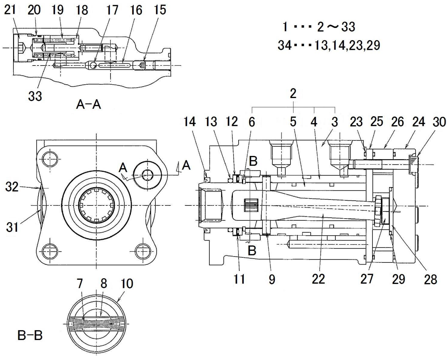
FIG.256 STEERING CASE ASSY ステアリングASSY
