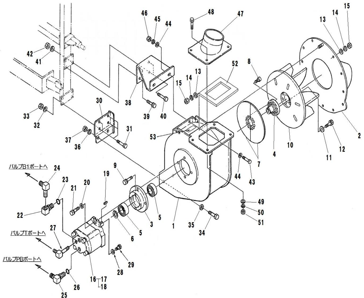
FIG.245 BLOWER HD ブロワ HD
