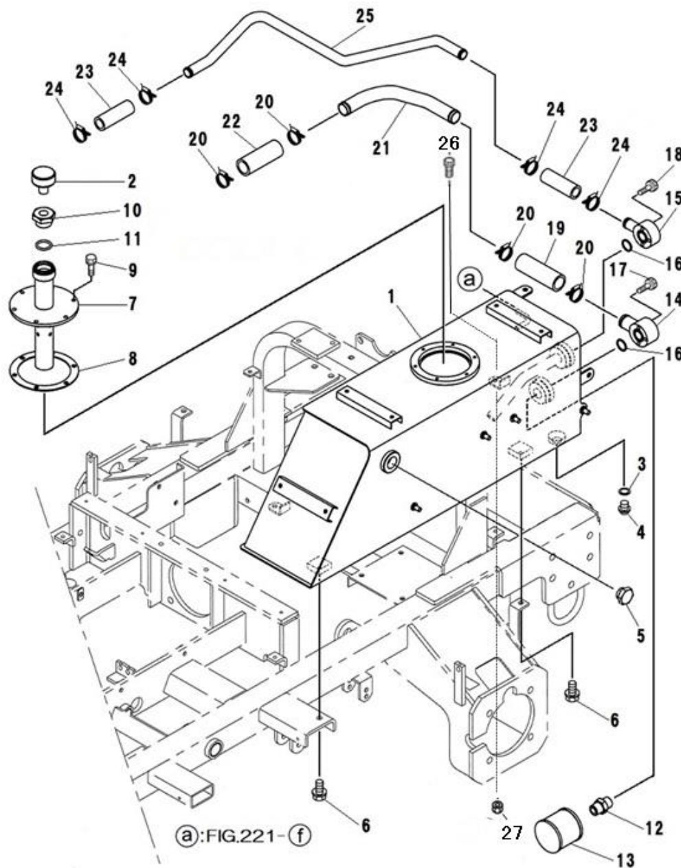
FIG.224 OIL TANK オイルタンク、サクシヨンライン
