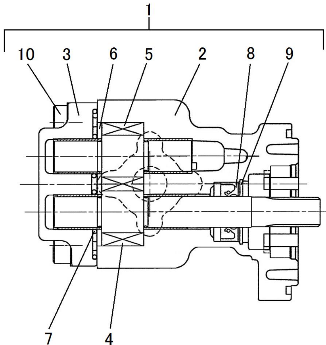
FIG.254 OIL PUMP オイルポンプ
