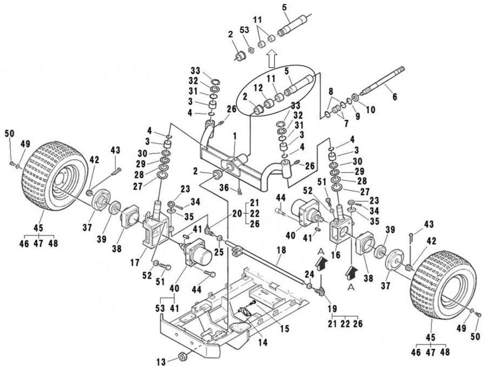
FIG.206 FRONT AXLE フロントアクスル
