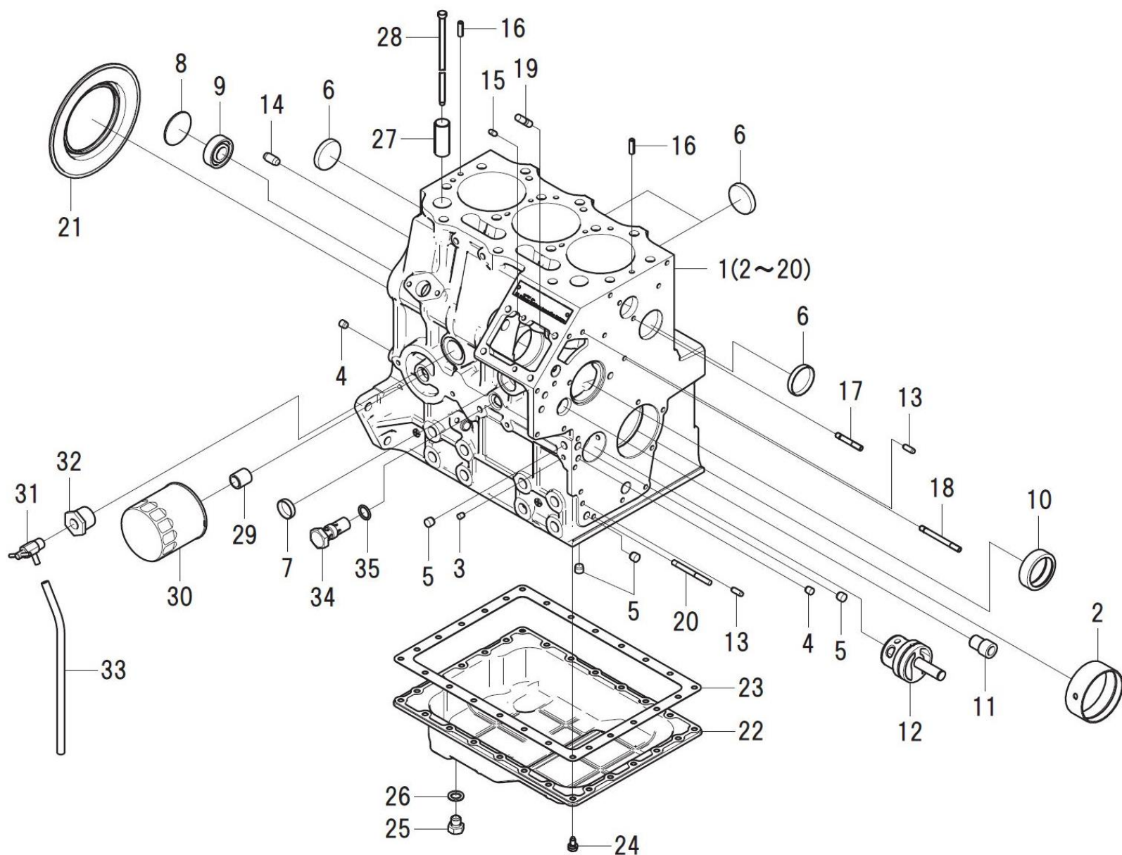
FIG.101 CYLINDER BLOCK/OIL PAN シリンダブロック/オイルパン
