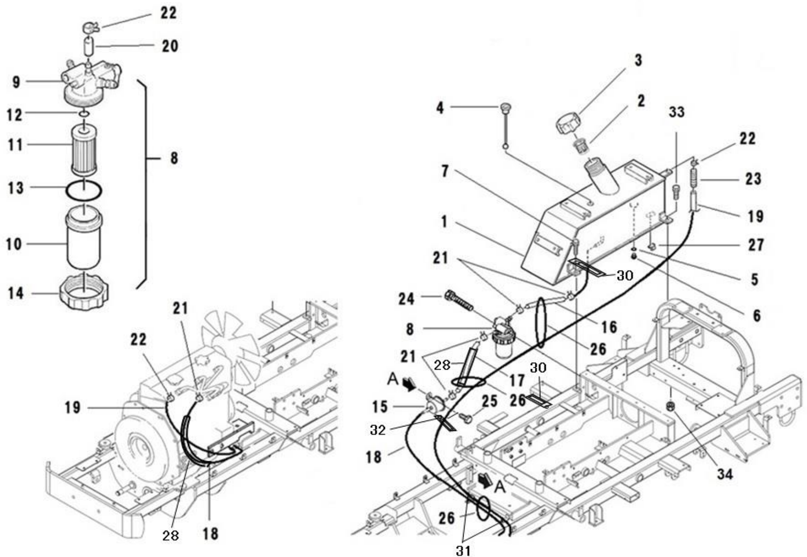
FIG.225 FUEL TANK ネンリョウタンク
