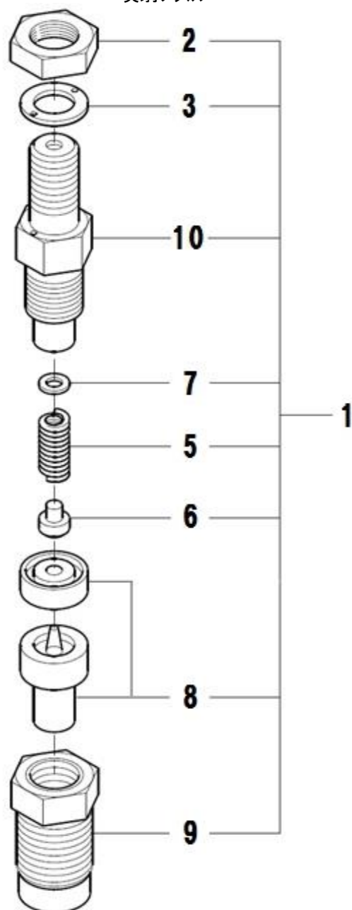
FIG.111 INJECTOR ASSY 噴射ノズル
