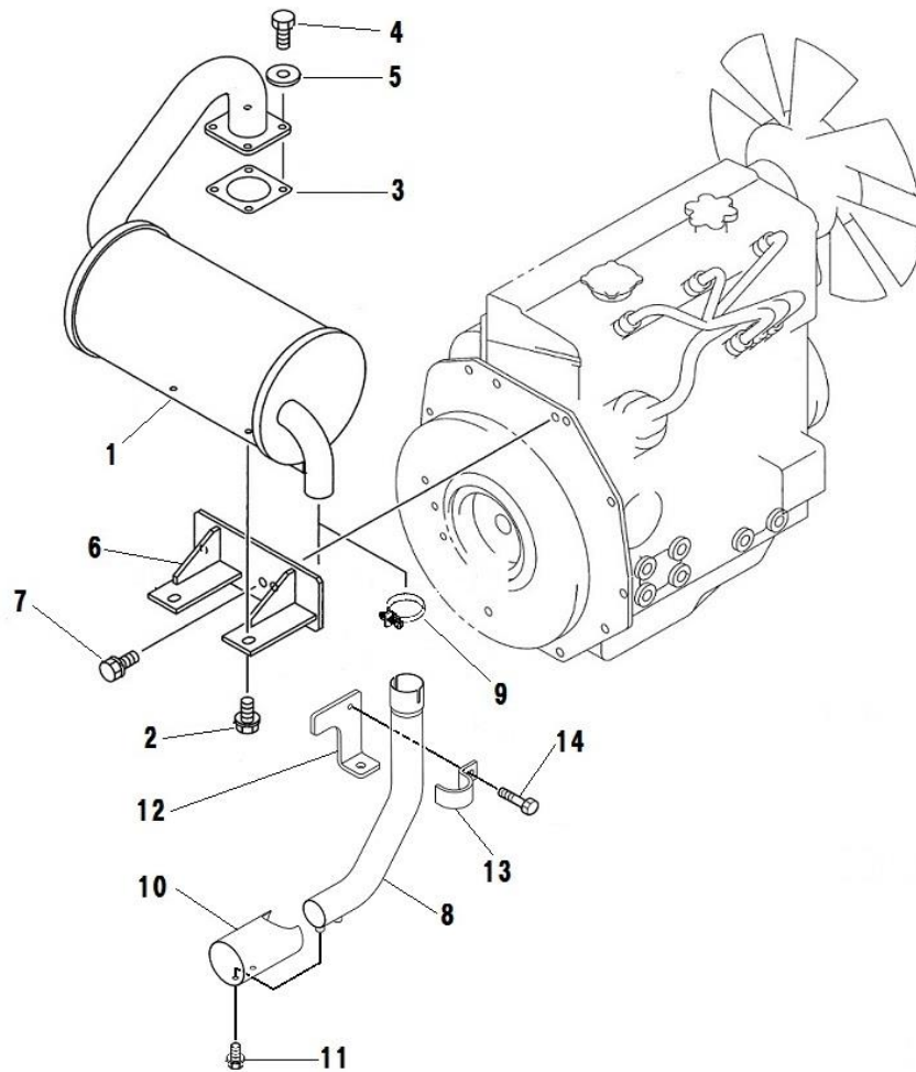
FIG.201 MUFFLER マフラー
