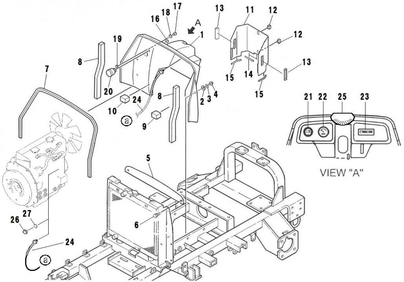
FIG.212 DASHBOARD ダッシュボード
