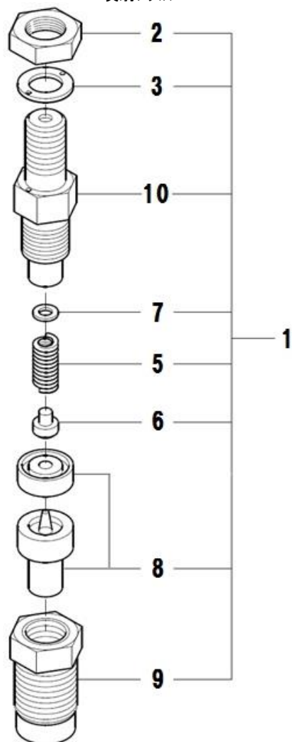
FIG.111 INJECTOR ASSY 噴射ノズル
