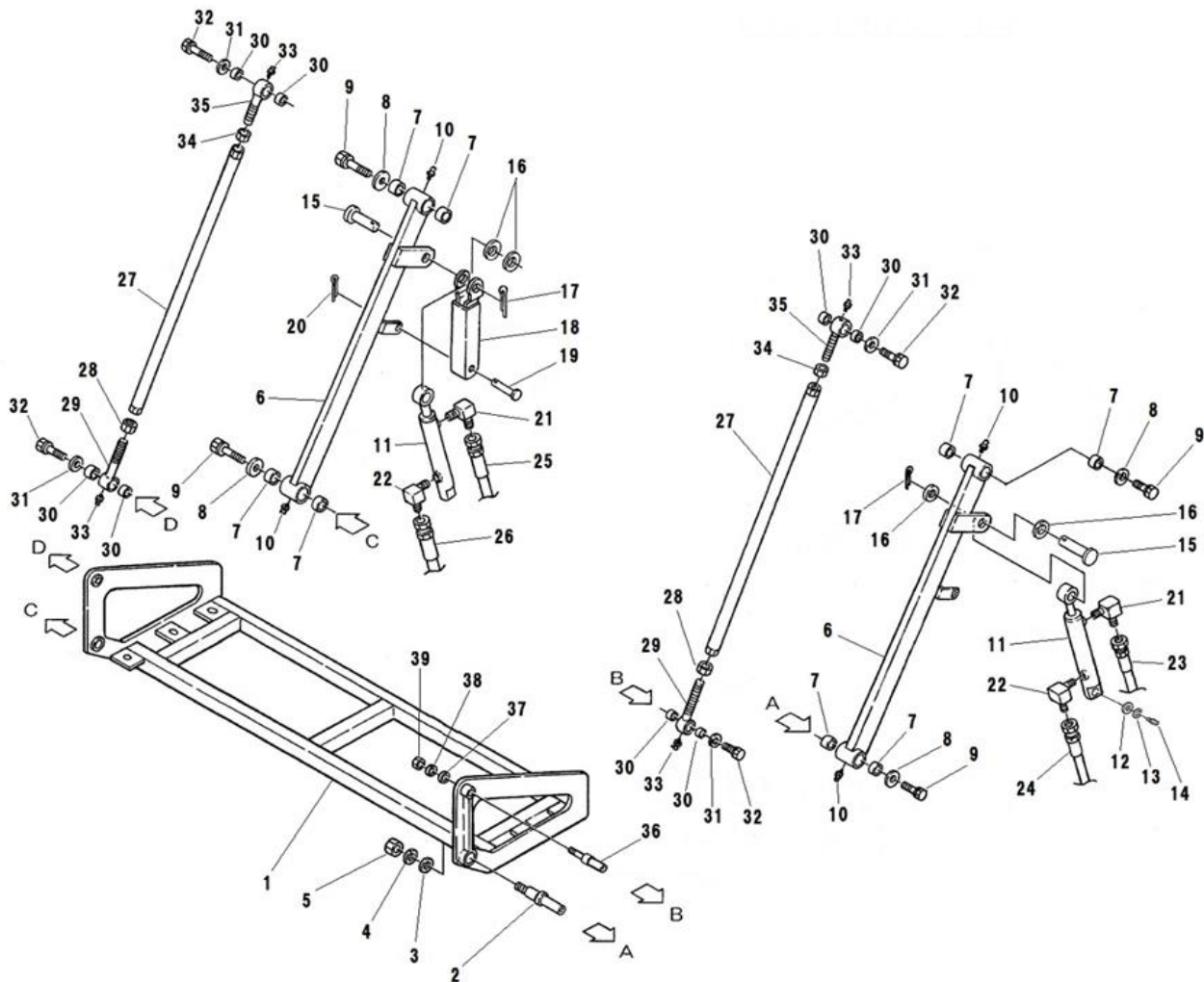
FIG.239 RINK HD リンク HD
