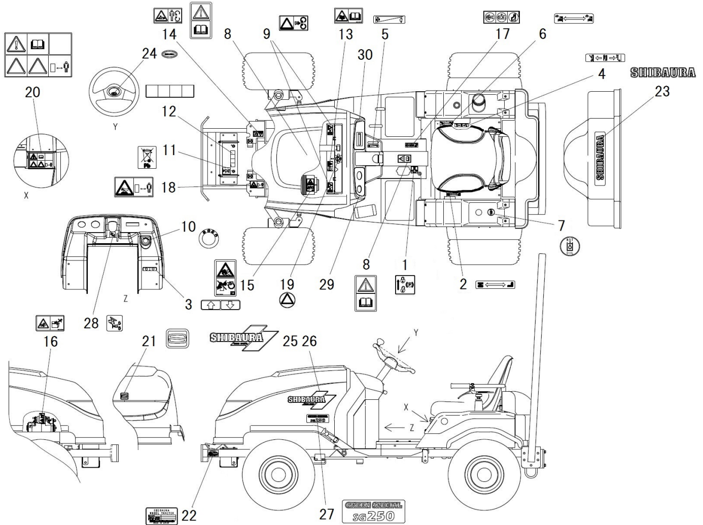
FIG.227 MARK メイバン
