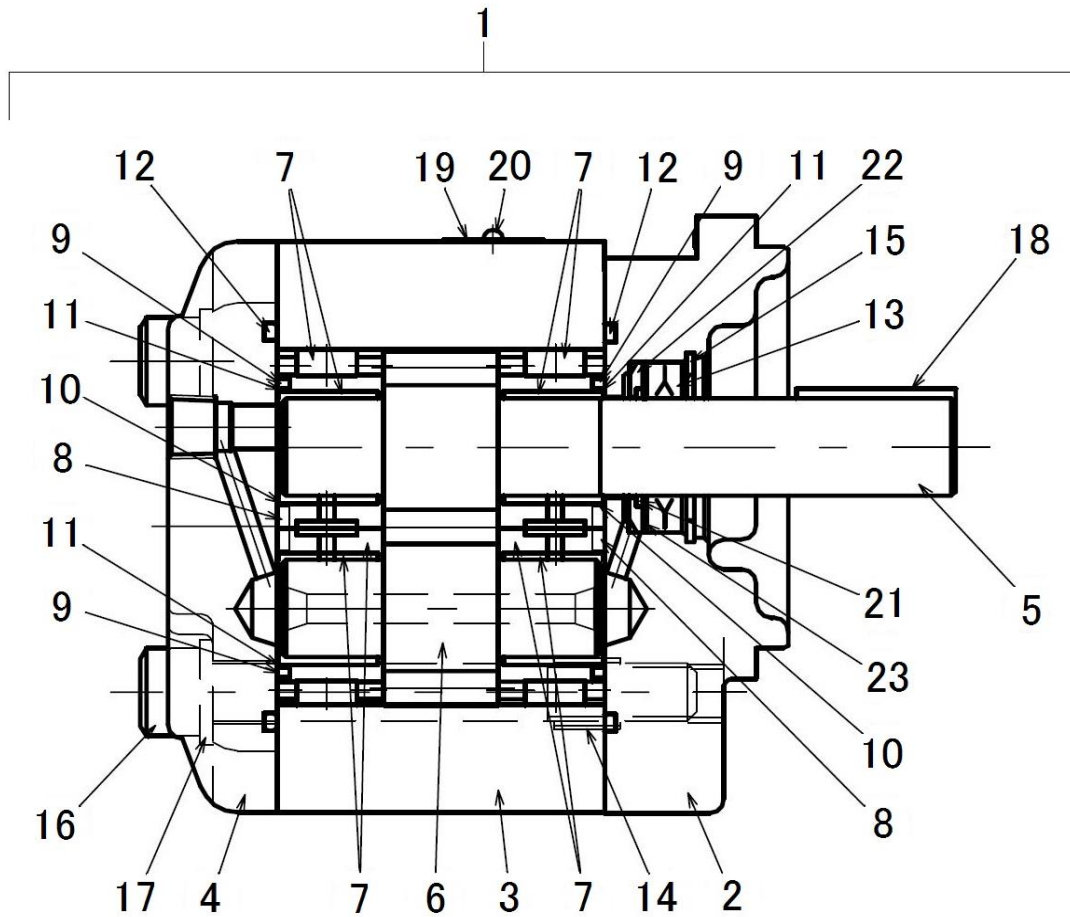
FIG.254 OIL MOTOR ASSY オイルモータASSY
