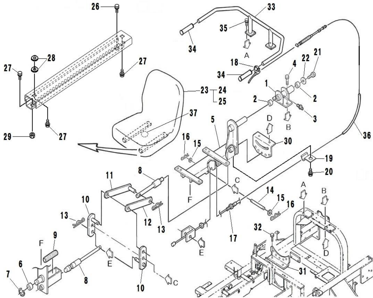
FIG.210 SEAT シート
