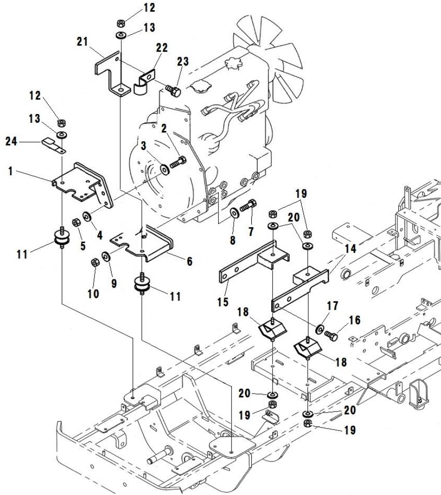
FIG.204 ENGINE MOUNT エンジンマウント
