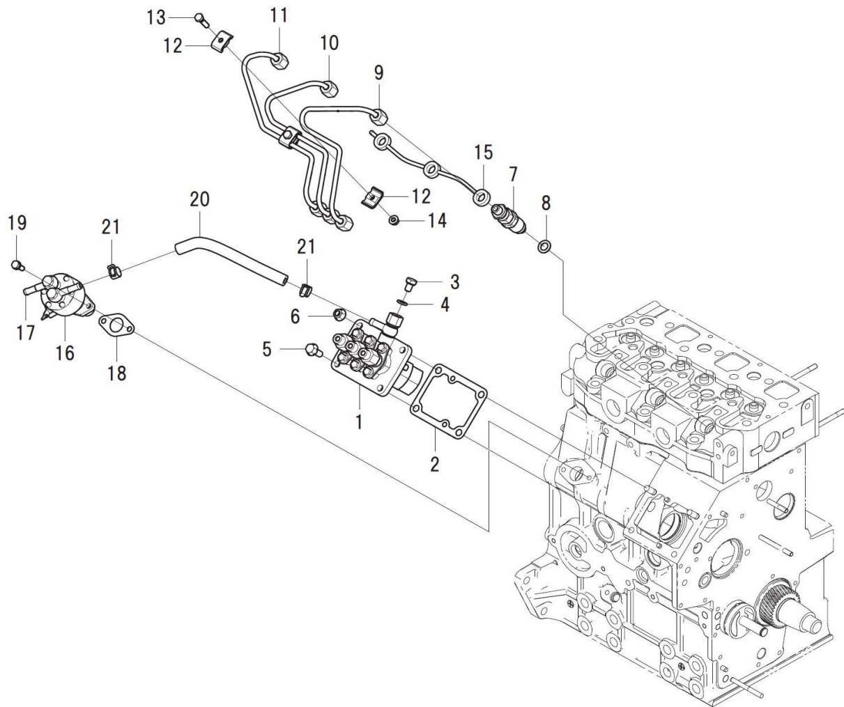
FIG.109 INJ PUMP/INJECTOR/INJ PIPE インジェクションポンプ/インジェクター/インジェクションパイプ
