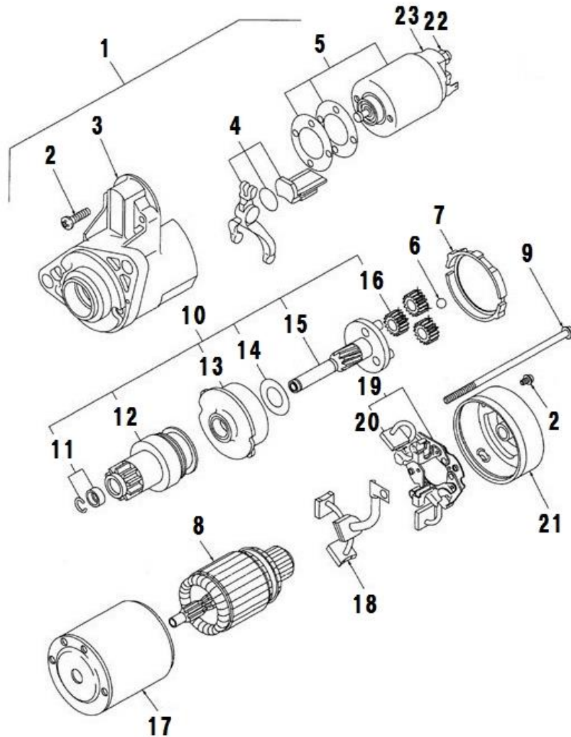
FIG.112 STARTING MOTOR スターティングモーター
