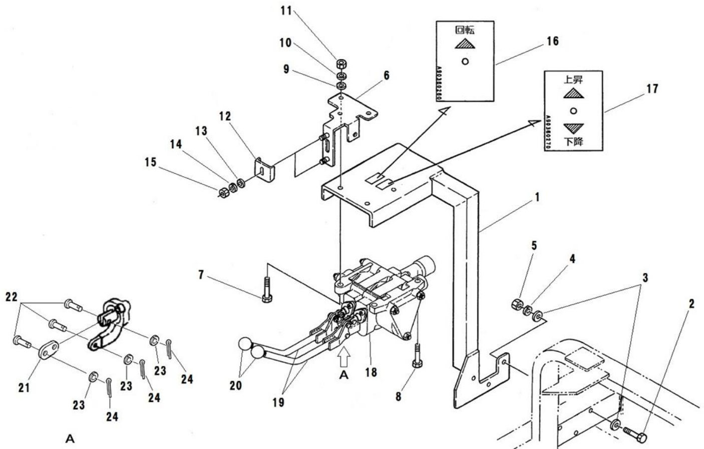
FIG.233 VALVE STAY T バルブステイ T
