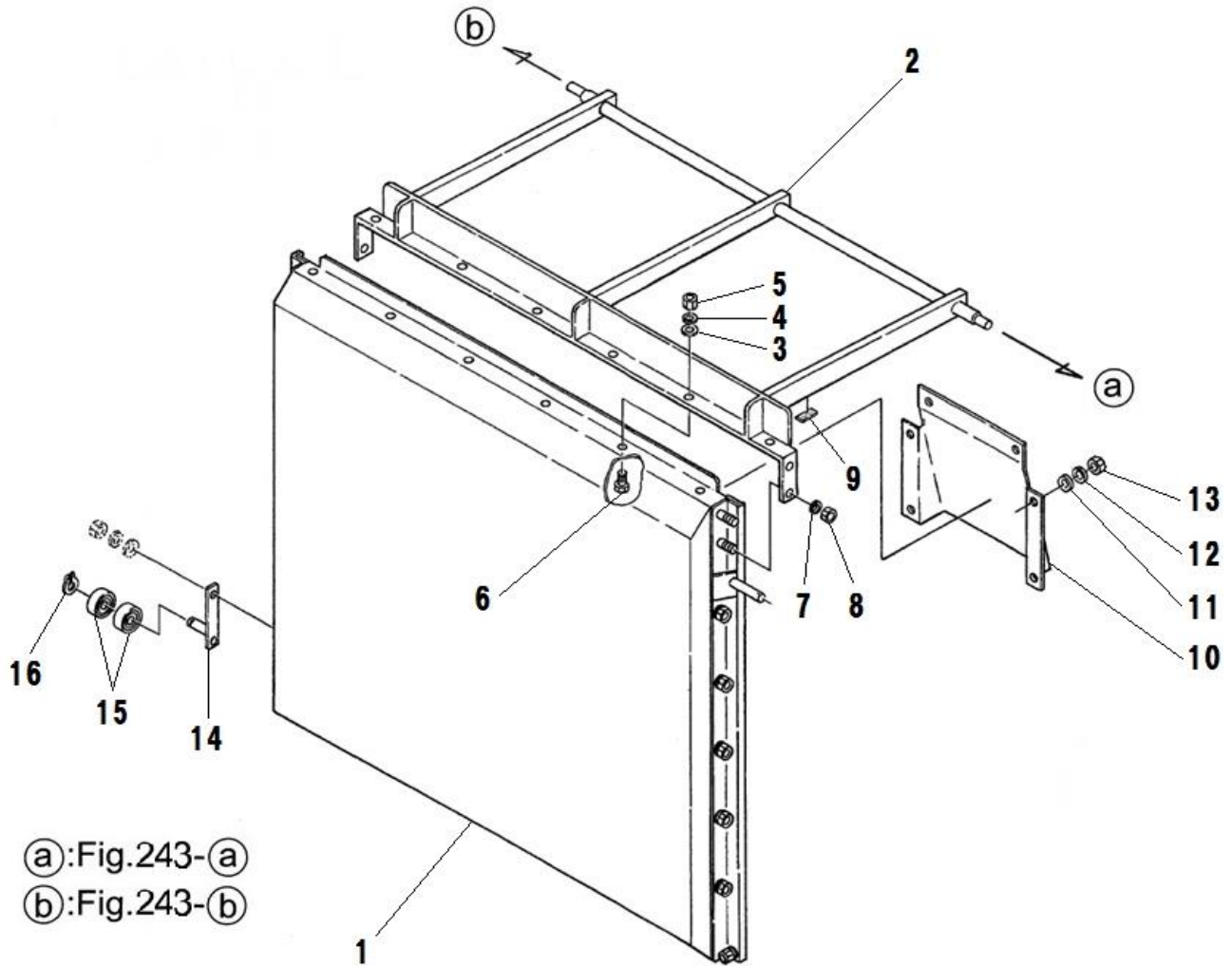
FIG.242 DOOR PARTS HD ドアパーツ HD
