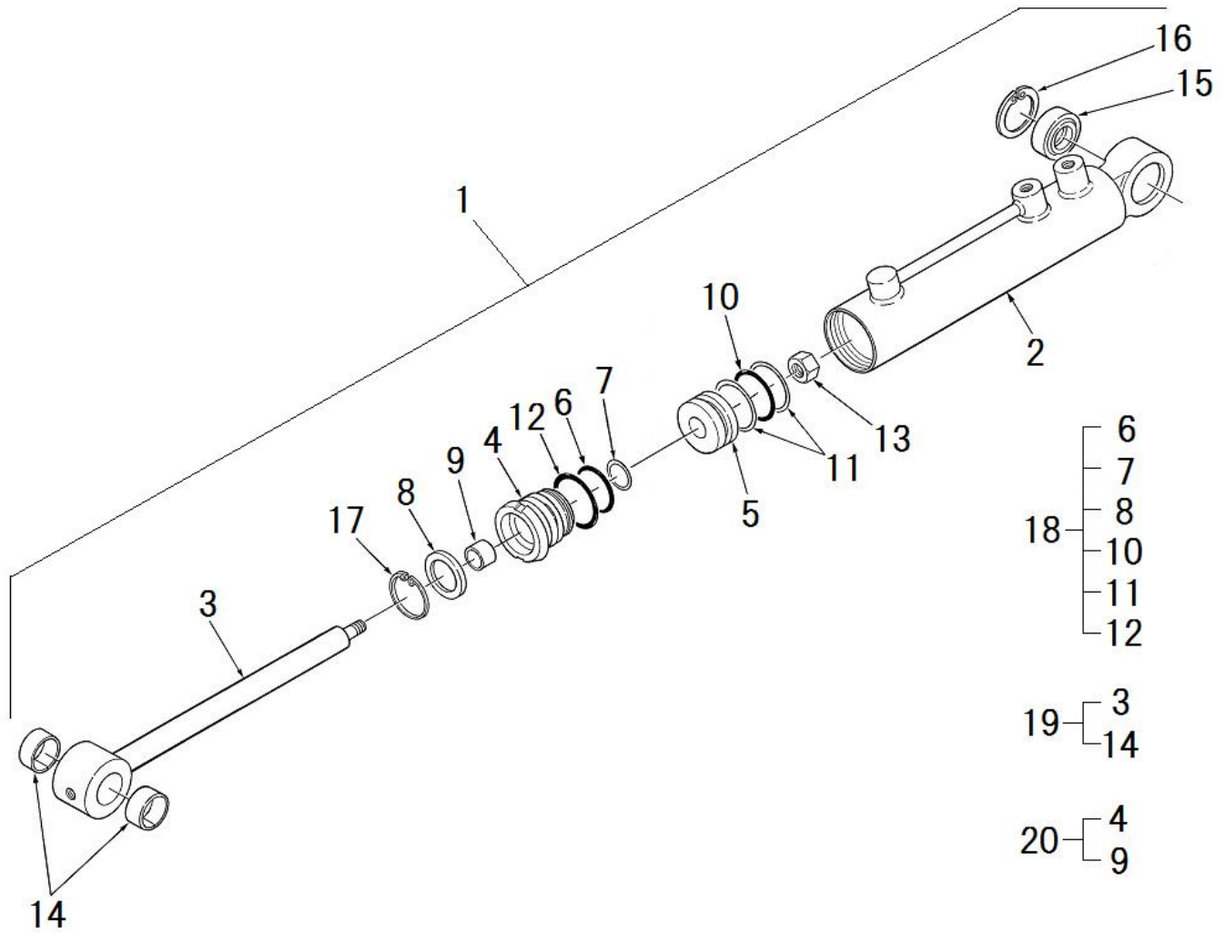
FIG.249 CYLINDER ASSY :STEERING シリンダーASSY パワーステ
