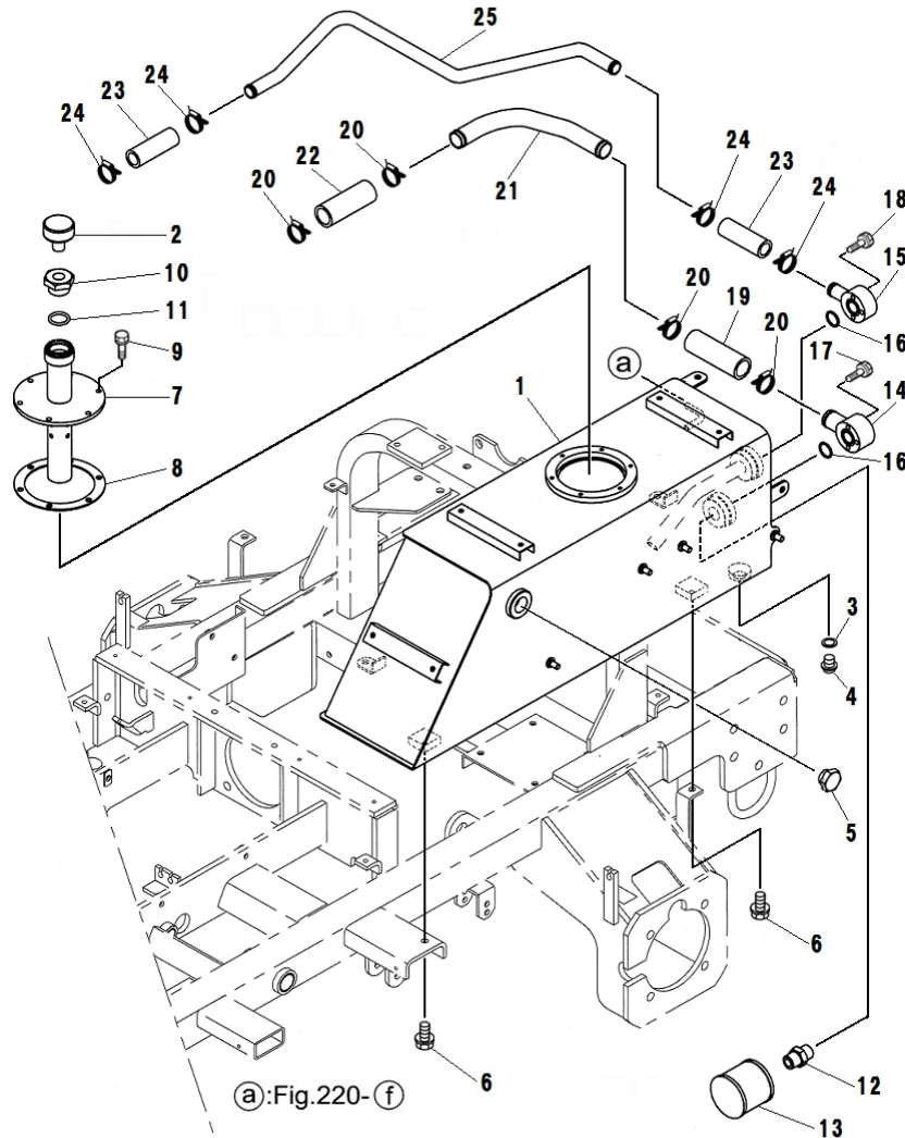
FIG.223 OIL TANK オイルタンク、サククションライン
