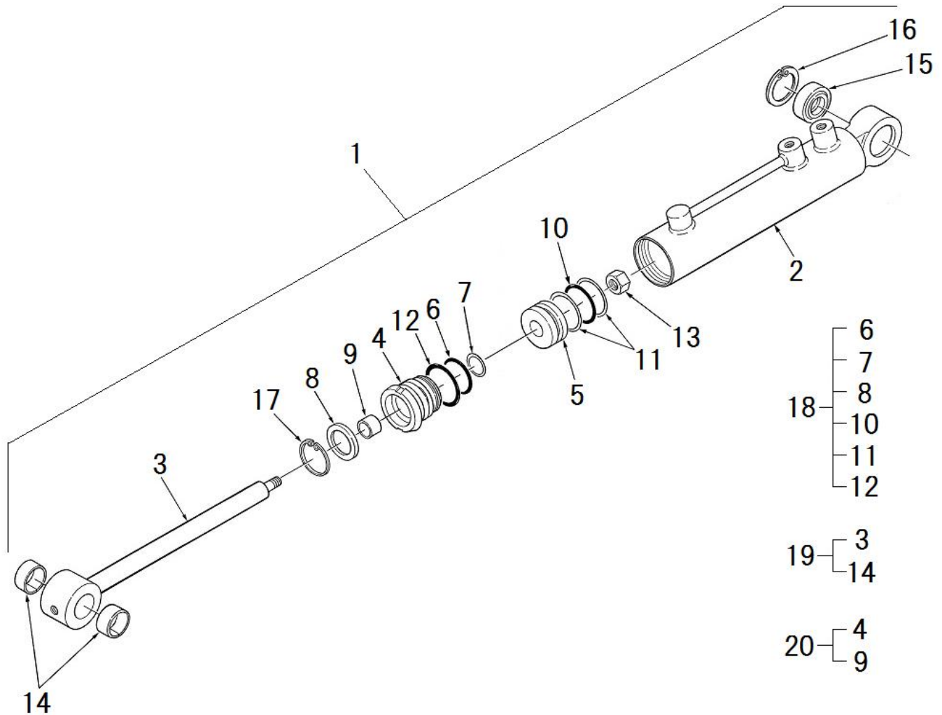
FIG.250 CYLINDER ASSY :LIFT シリンダーASSY モアリフト
