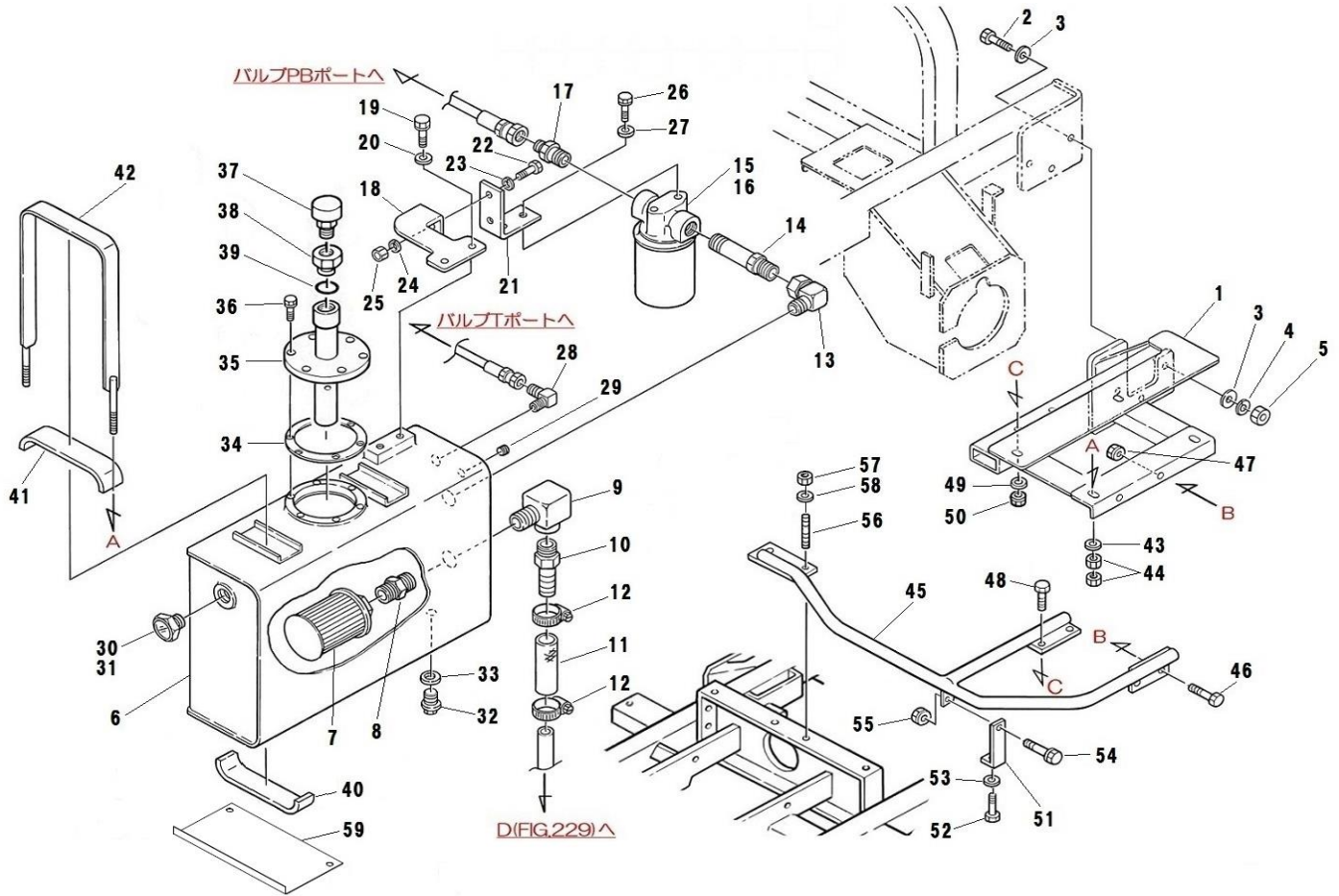
FIG.229 OIL TANK (M.T.HD) オイルタンク (M.T.HD)
