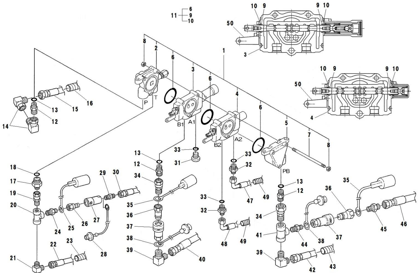
FIG.234 CONTROL VALVE T コントロールバルブ T
