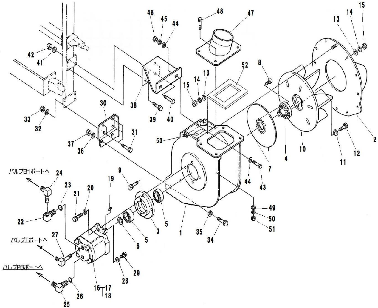
FIG.244 BLOWER HD ブロワ HD
