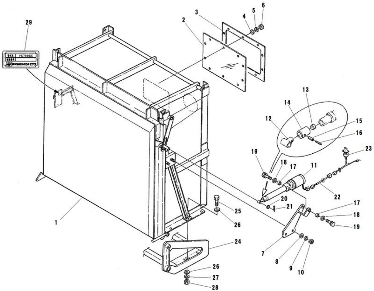
FIG.240 HOPPER HD ホッパー HD
