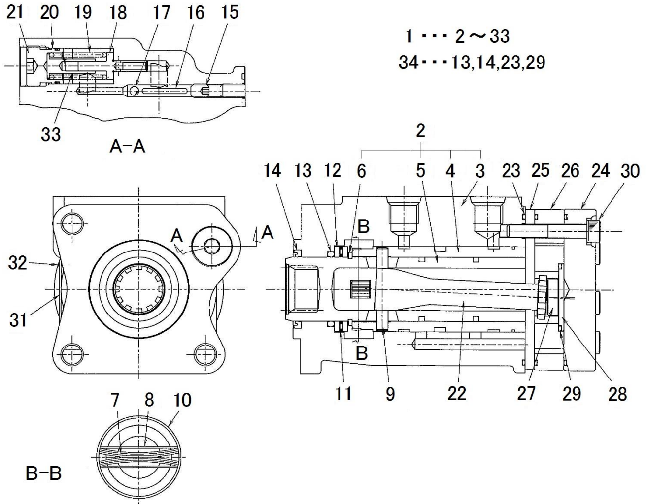
FIG.255 STEERING CASE ASSY ステアリングASSY
