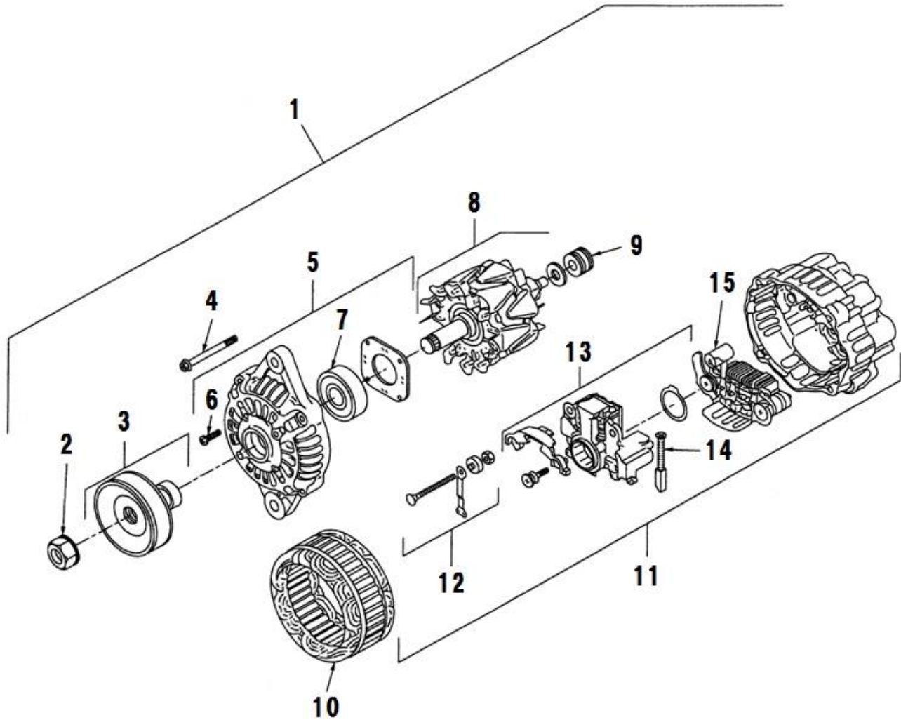
FIG.113 ALTERNATOR オルタネータ
