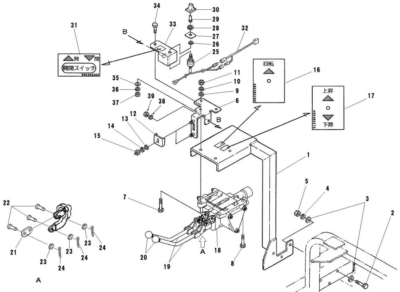
FIG.236 VALVE STAY HD バルブステイ HD
