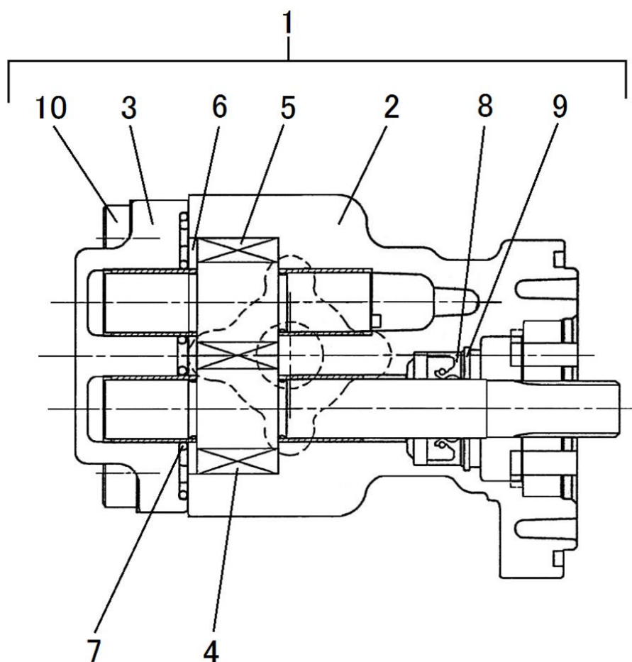
FIG.253 OIL PUMP オイルポンプ
