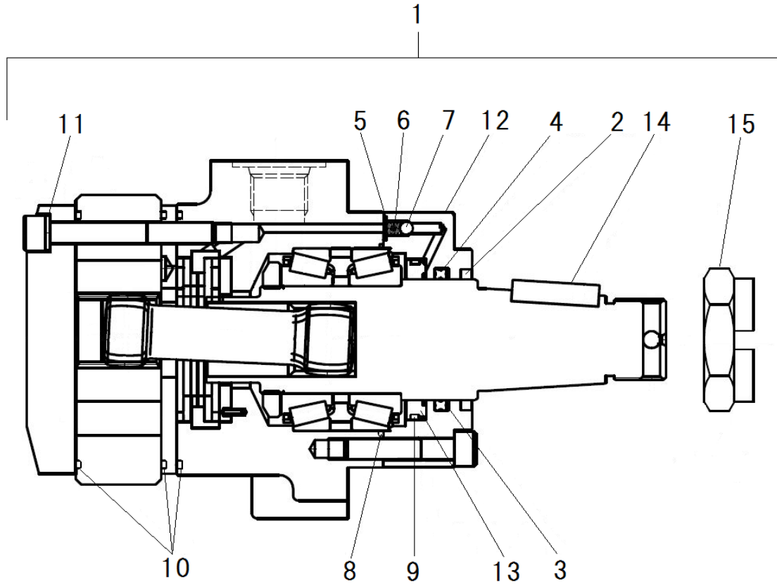
FIG.246 OIL MOTOR ASSY F オイルモータASSY F
