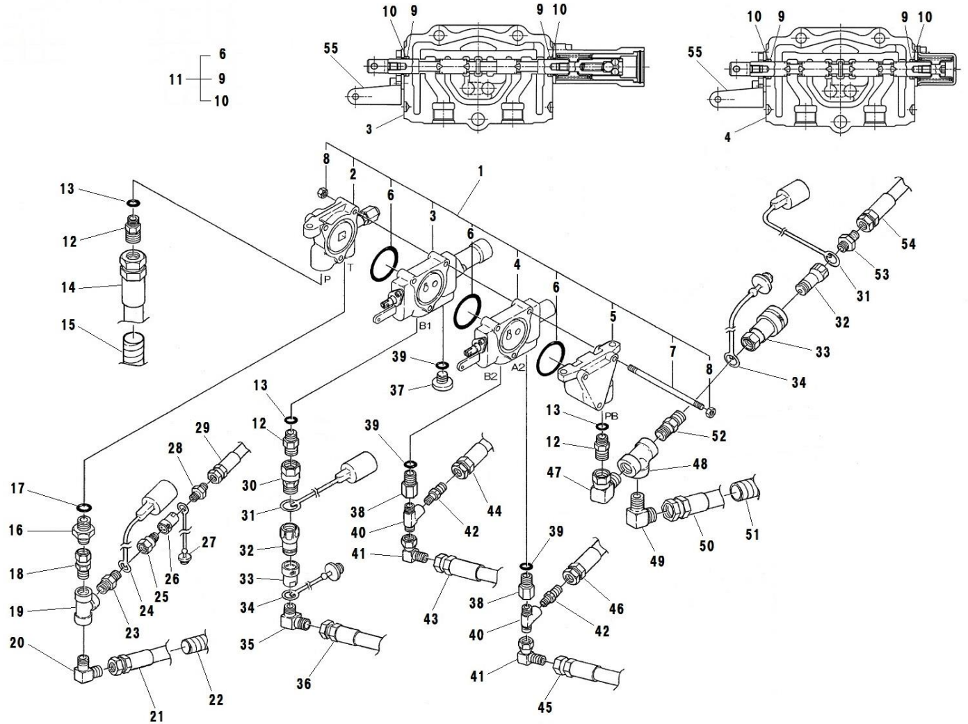
FIG.237 CONTROL VALVE HD コントロールバルブ HD
