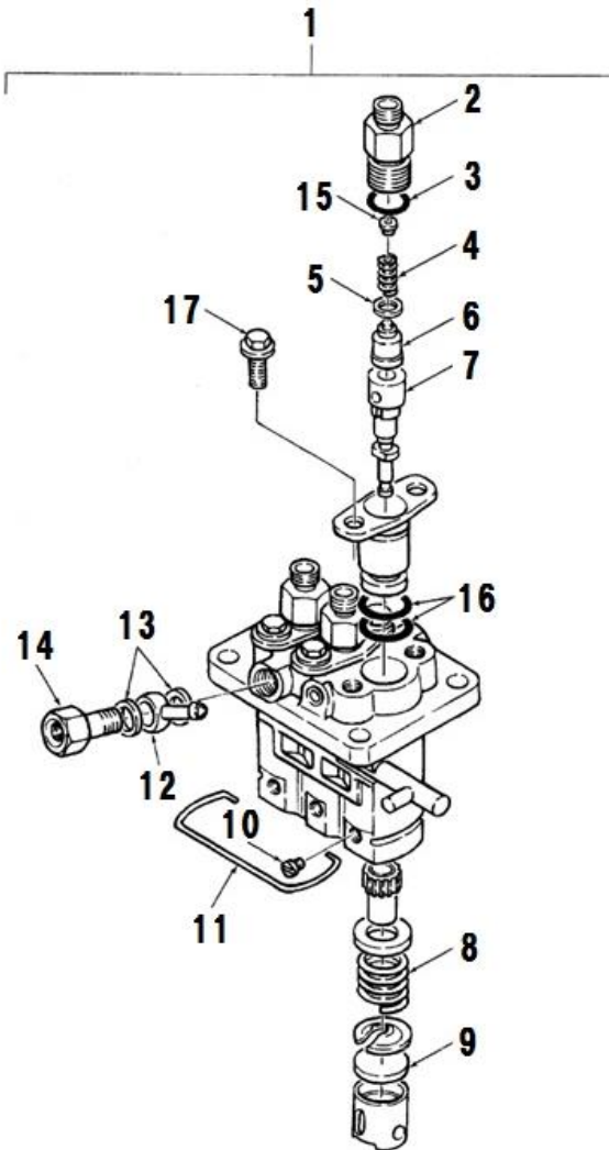
FIG.110 INJECTION PUMP インジェクションポンプ
