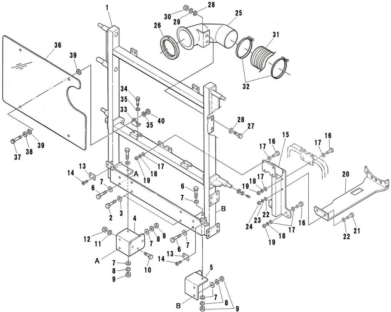
FIG.238 FRAME HD フレーム HD
