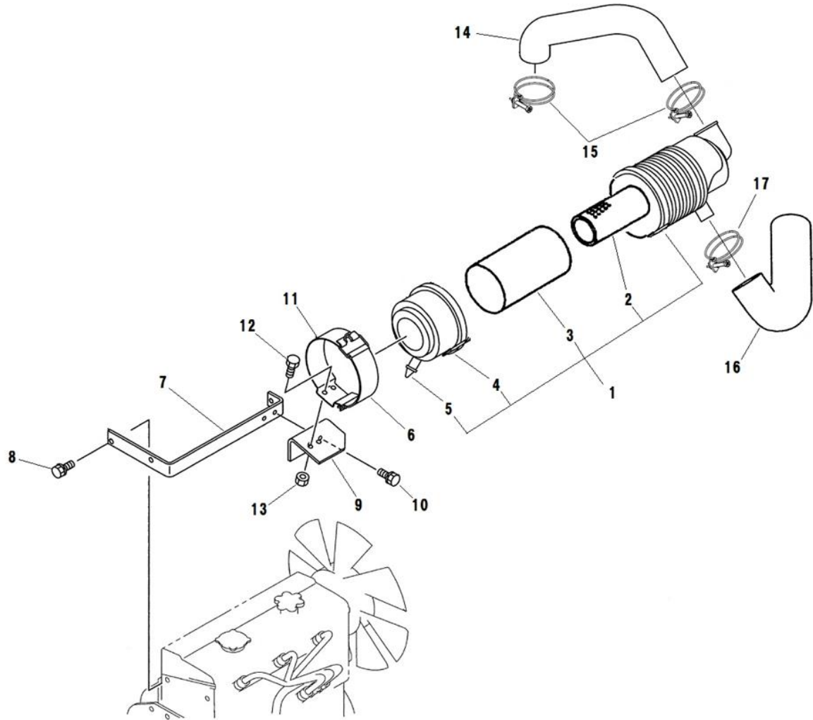
FIG.202 AIR CLEANER エアークリーナー
