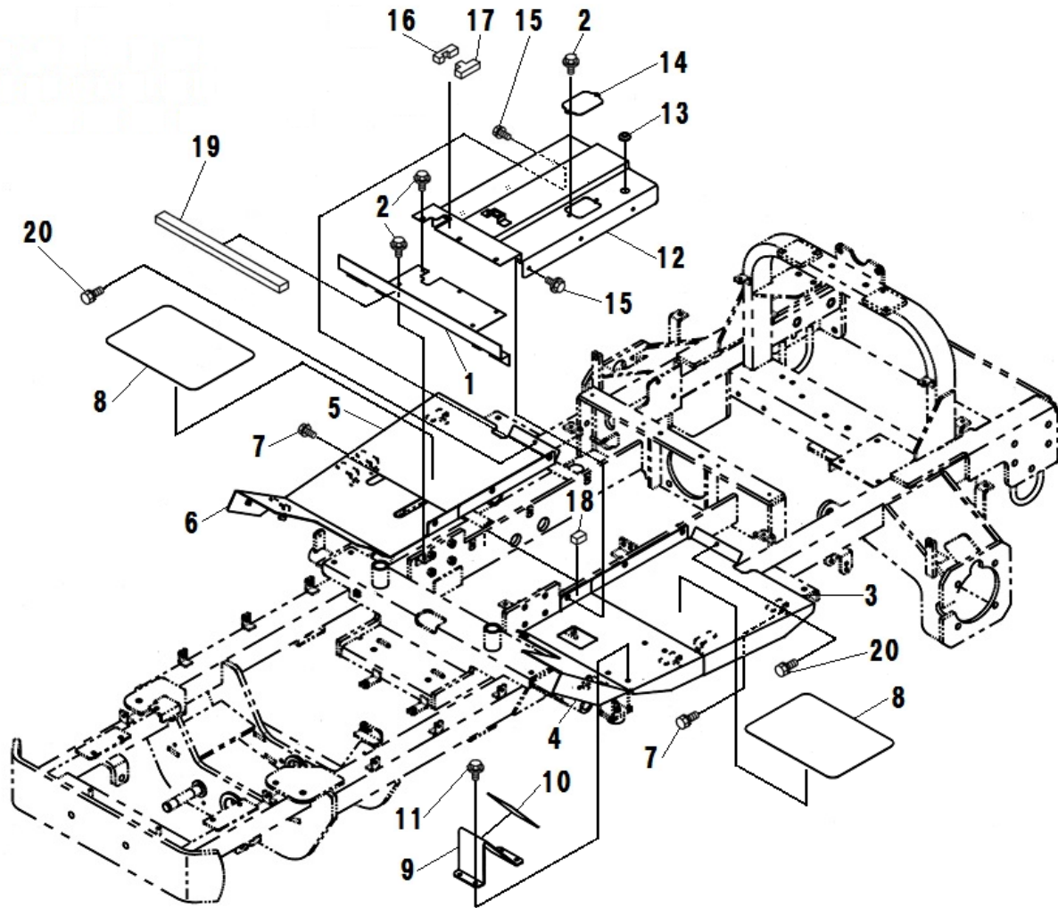
FIG.214 STEP ステップ
