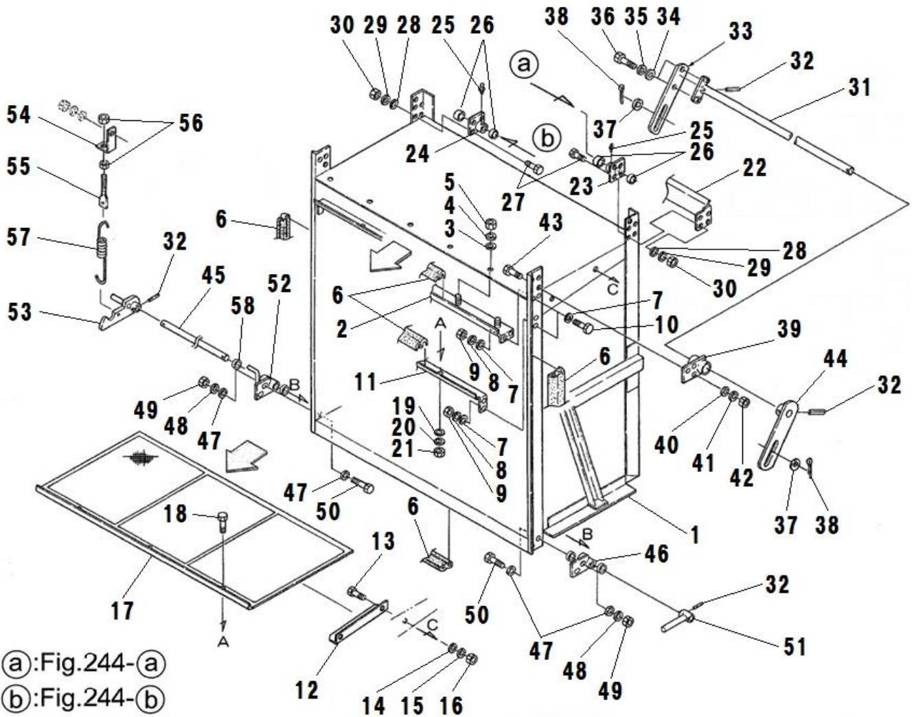
FIG.241 HOPPER PARTS HD ホッパーパーツ HD
