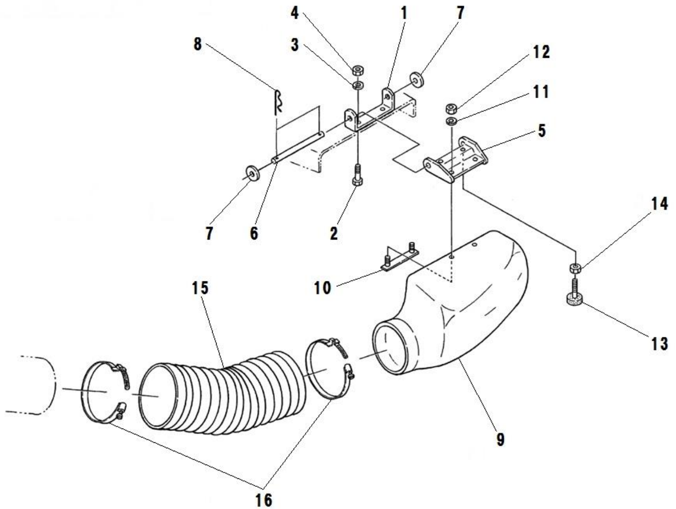
FIG.243 BOOTS HD ブーツ HD
