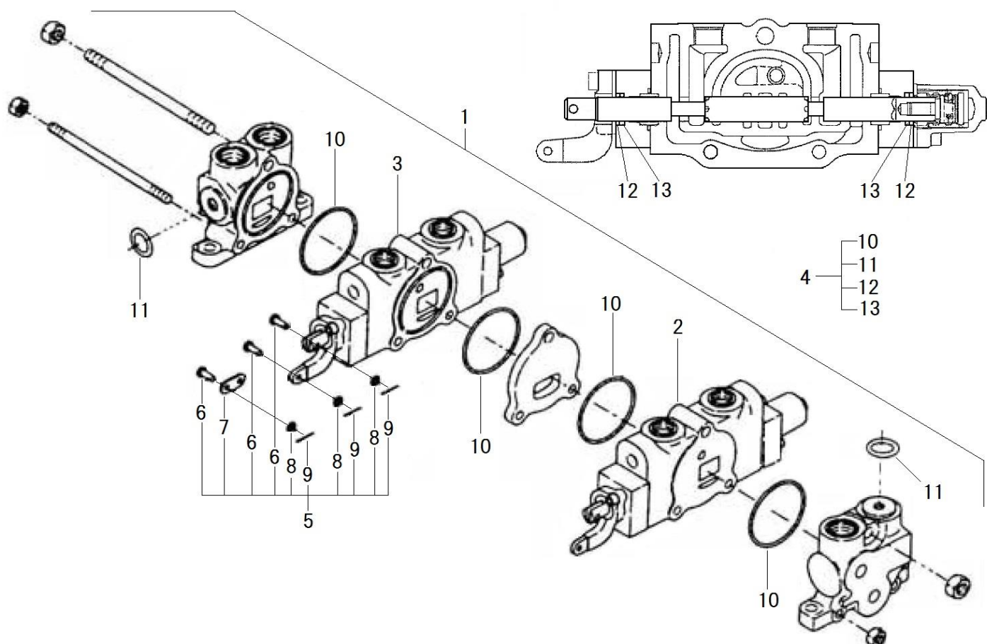
FIG.245 VALVE ASSY コントロールバルブASSY
