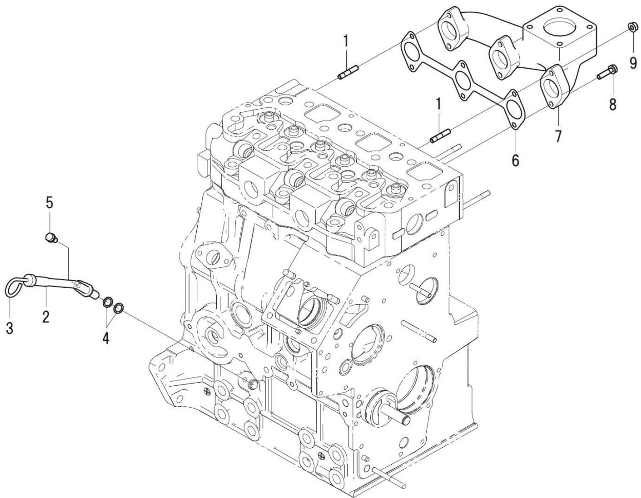
FIG.106 EXHAUST MANIFOLD/GAUGE エキゾーストマニホルド/ゲージ
