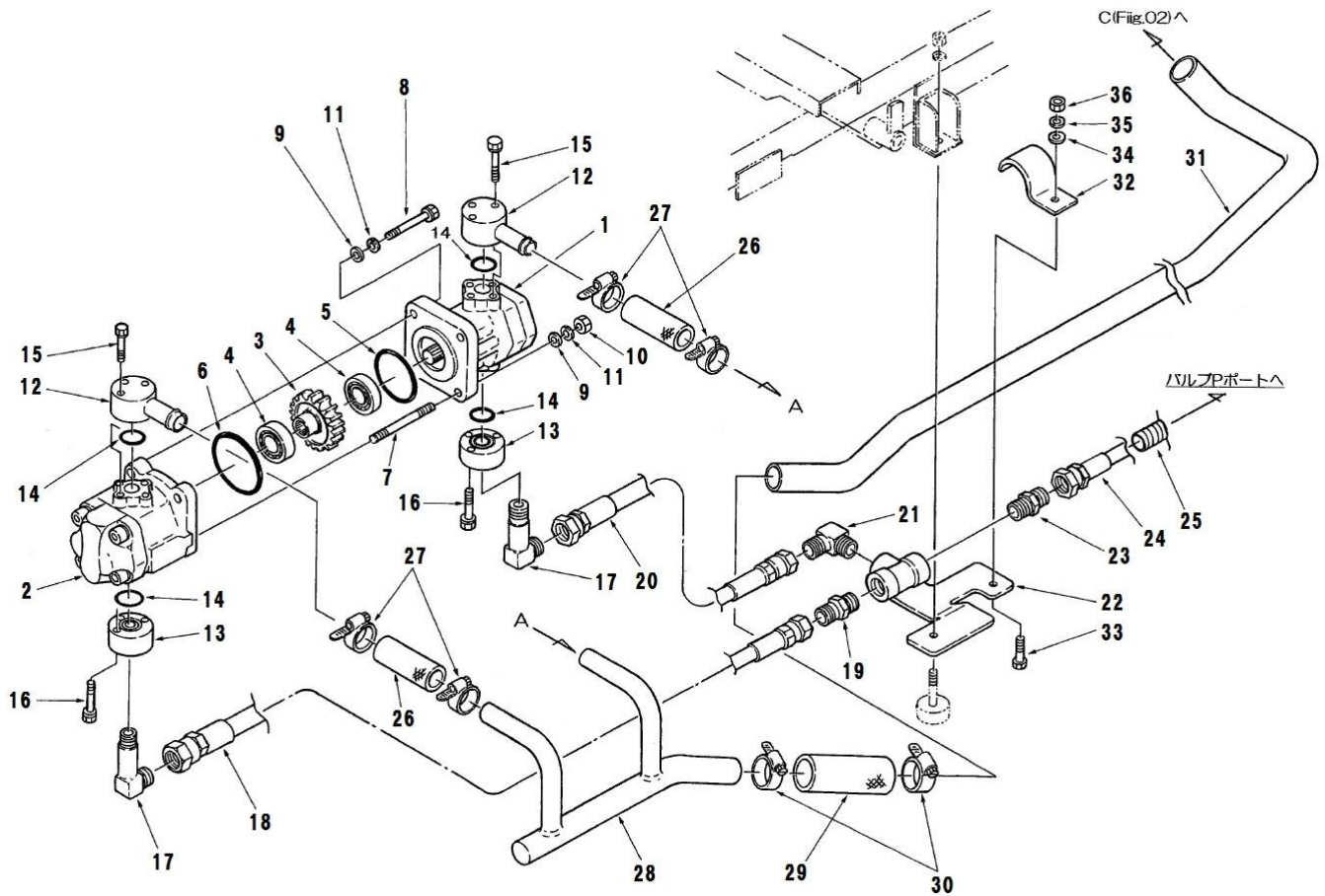
FIG.228 PUMP (M.T.HD) ポンプ (M.T.HD)
