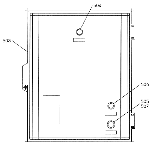
スターデルタ動力盤
