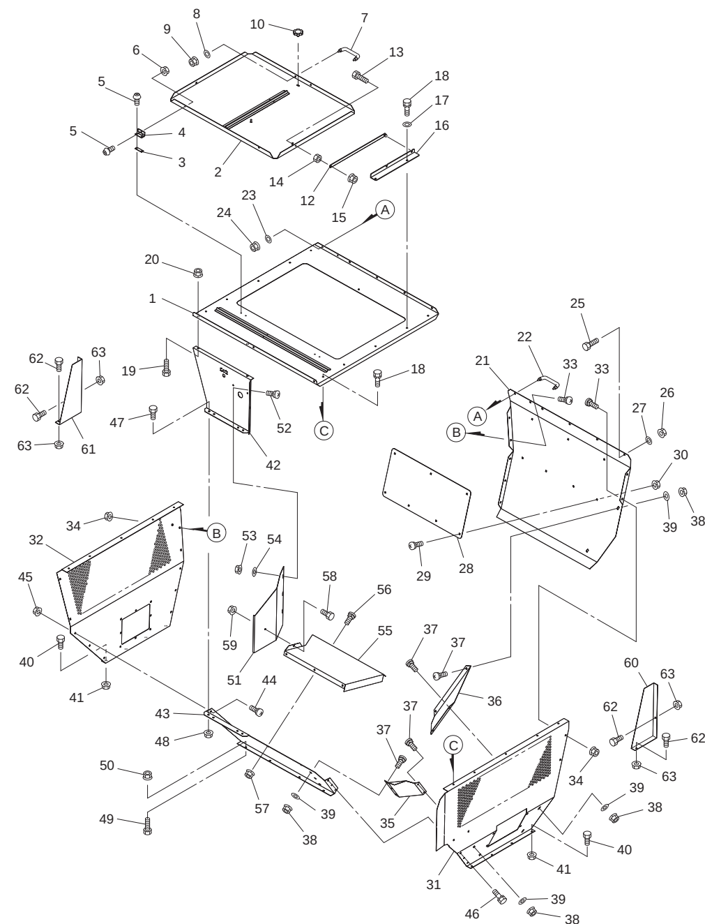
Fig.404. ホッパ
