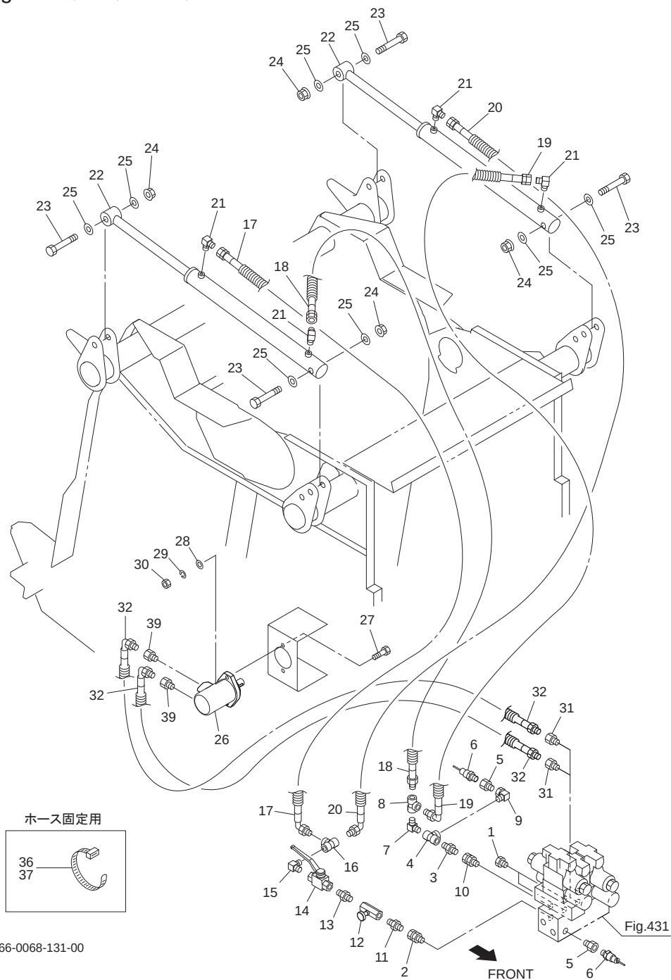
Fig.432. 油圧(ゲート)
