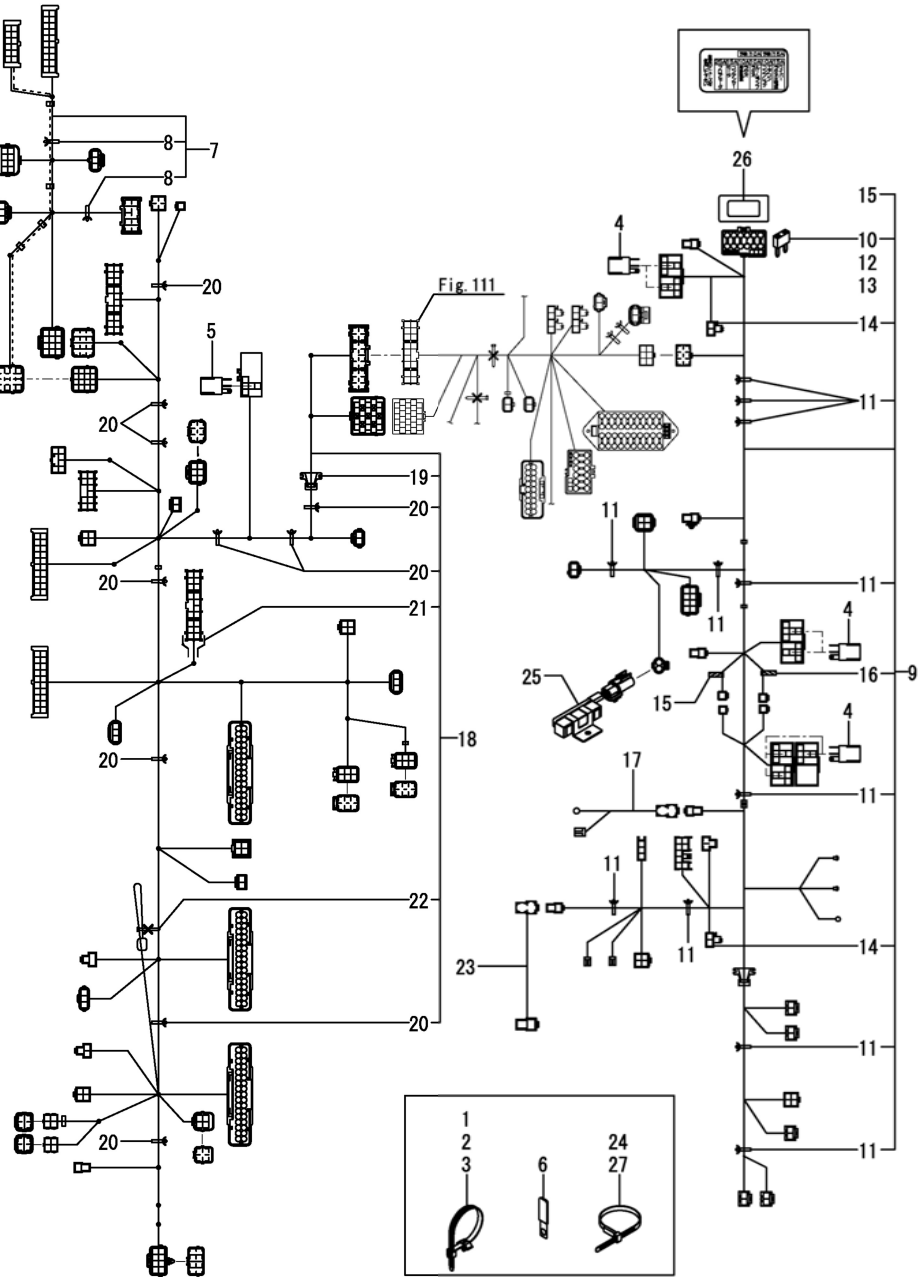
Fig.113. ワイヤハーネス(キャビン)
