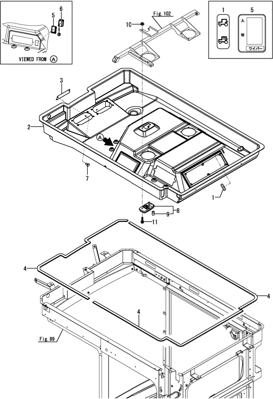
OCNP7-M01300 キャビン部 Fig.88. キャビン(天井)
