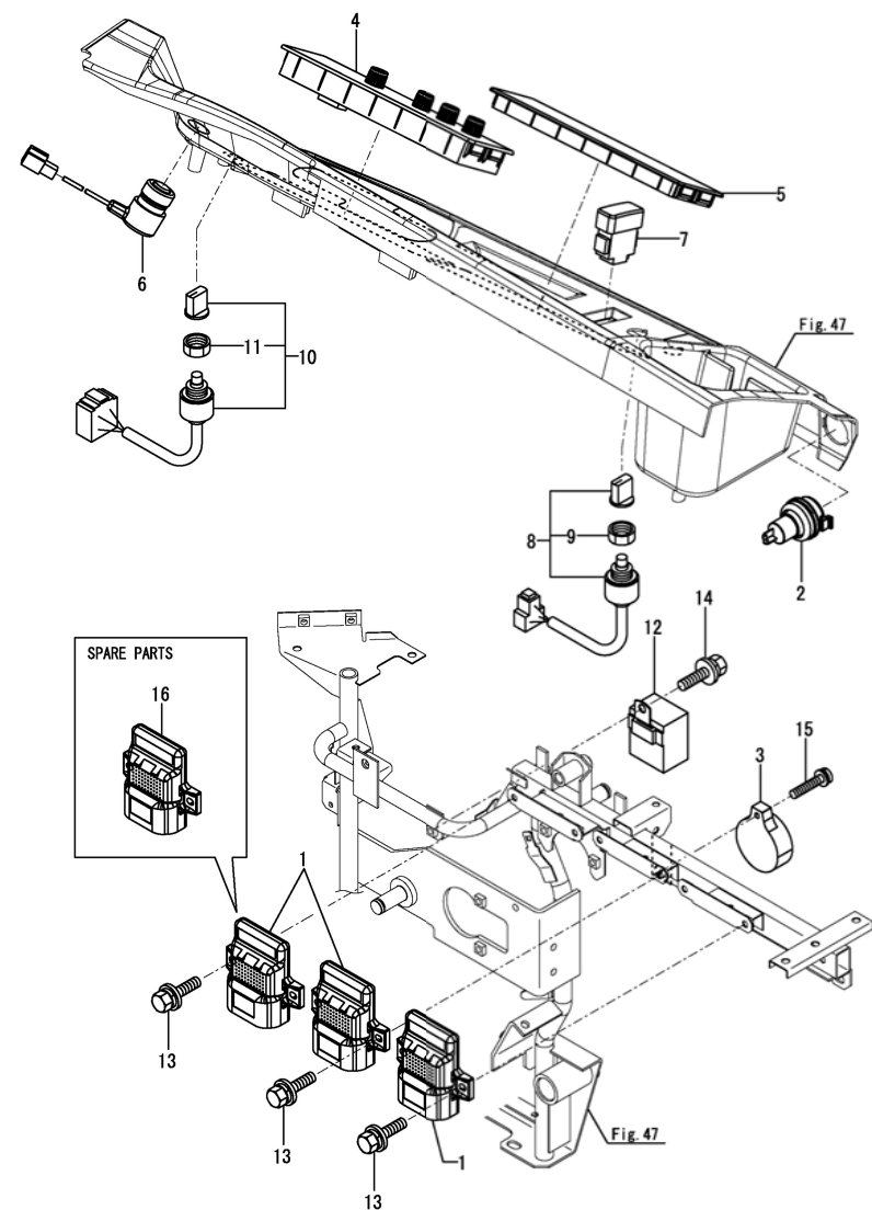
0CNP7-M01300 走行部(2) Fig.48. サイドコラム(2)
