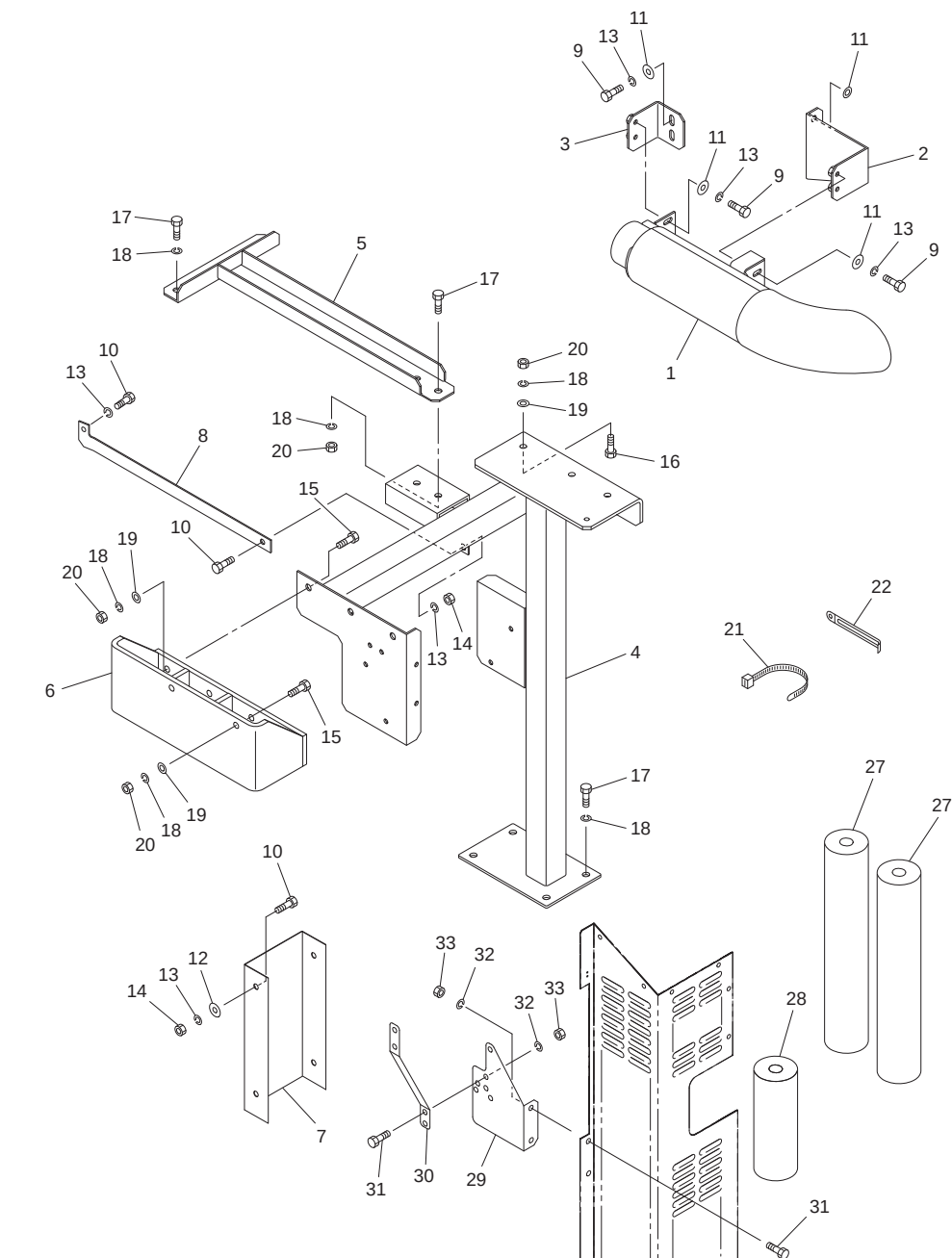
Fig.434. マフラー
