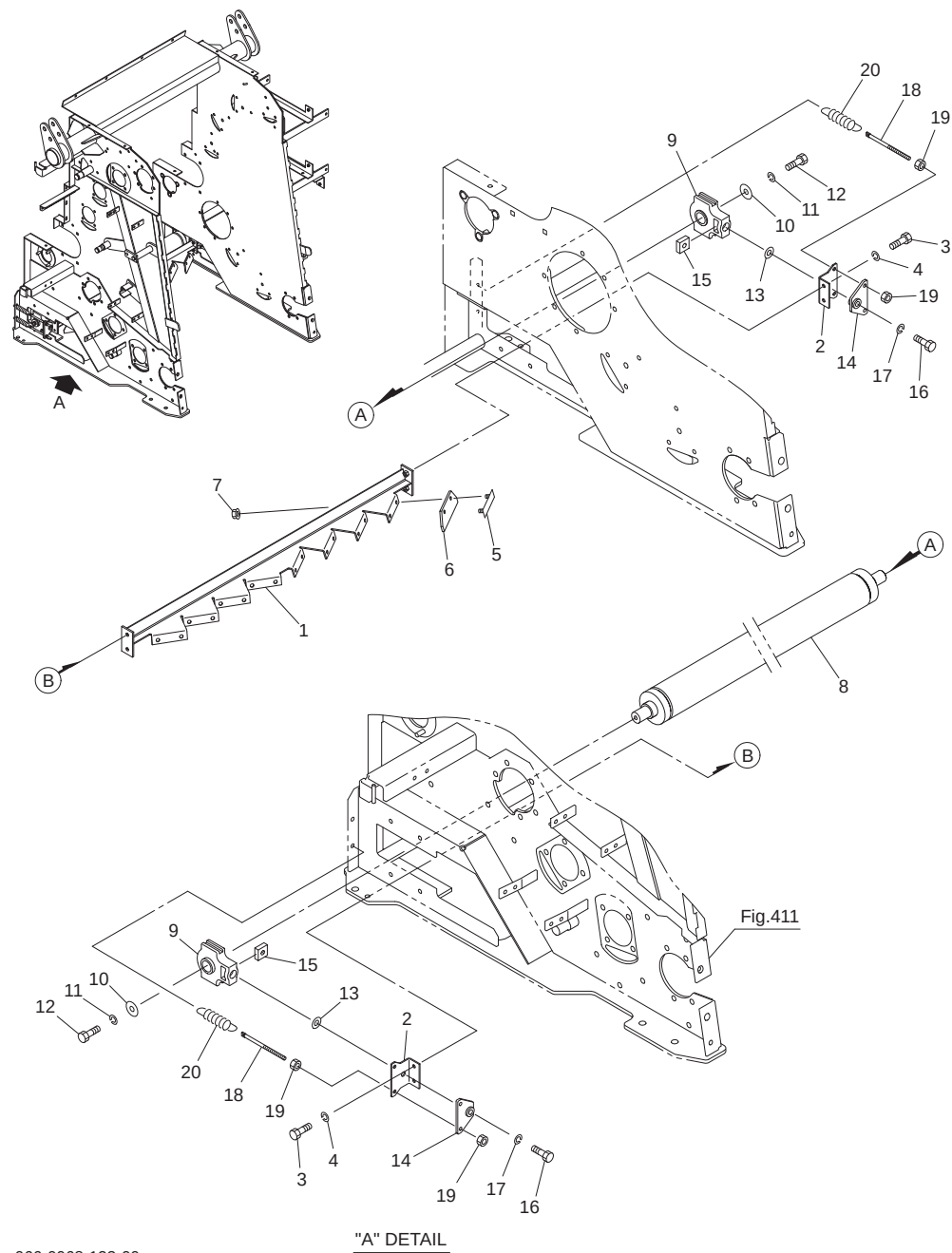
Fig.414. 成形ベルト(1)
