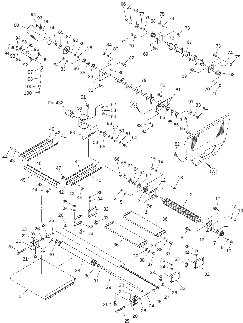
Fig.406. コンベア
