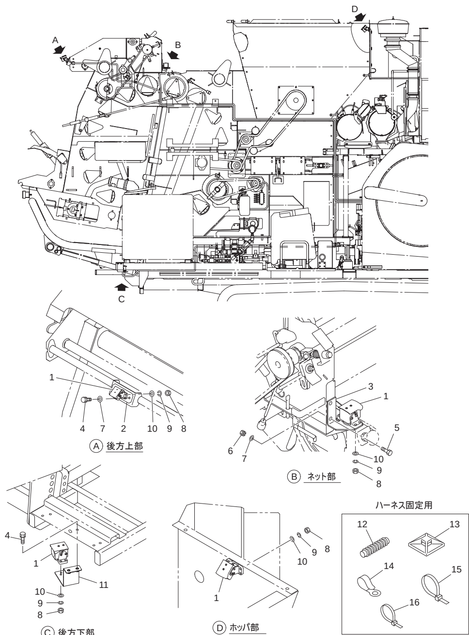
Fig.437. 電装(3)
