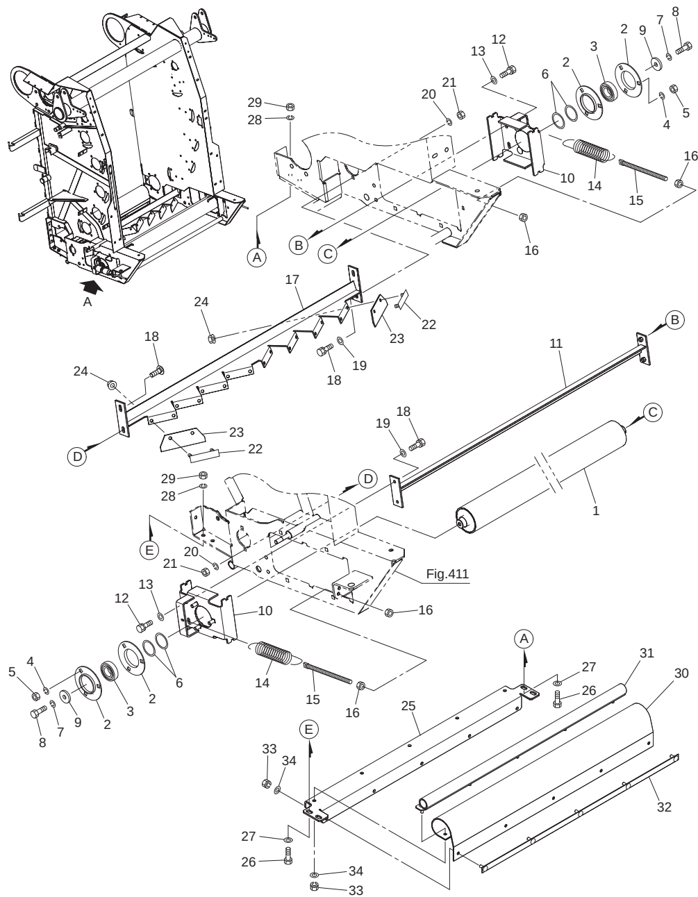
Fig.415. 成形ベルト(2)
