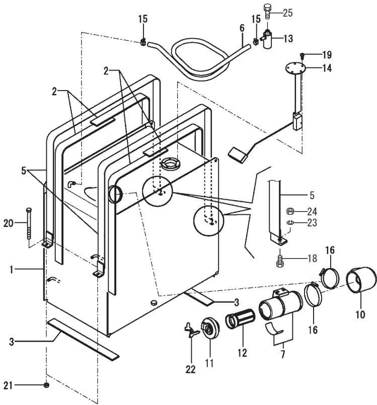
Fig.4. 燃料タンク(1)
