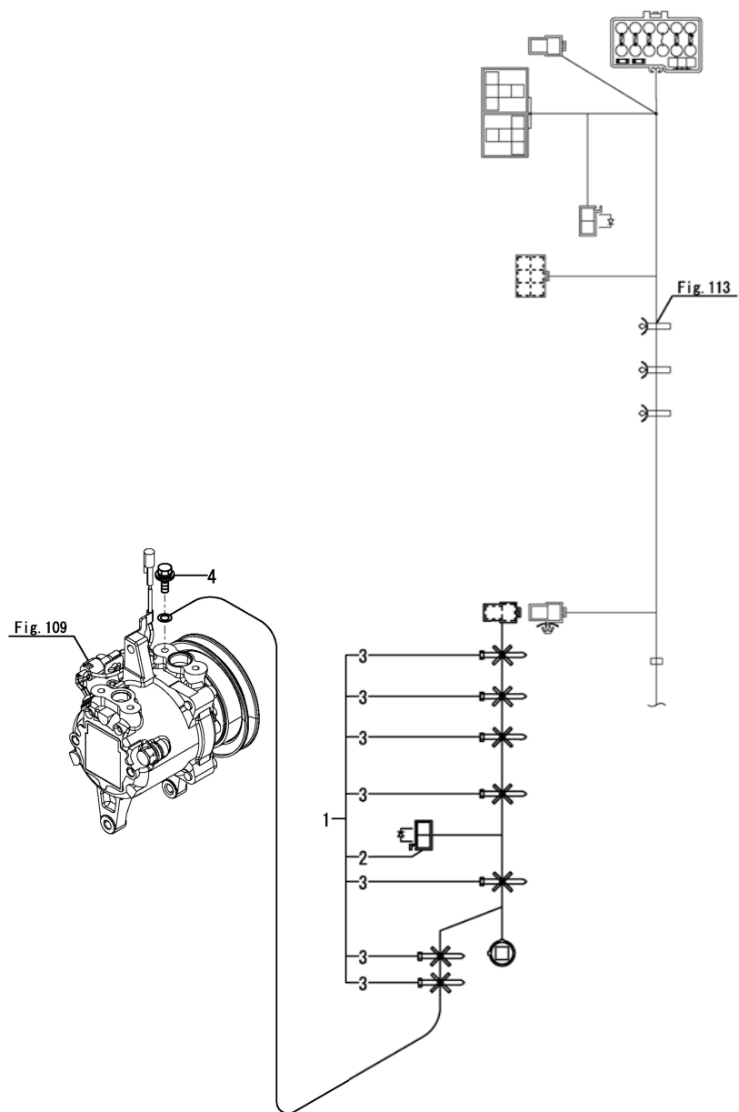
Fig.112. ワイヤーハーネス(コンプレッサー)
