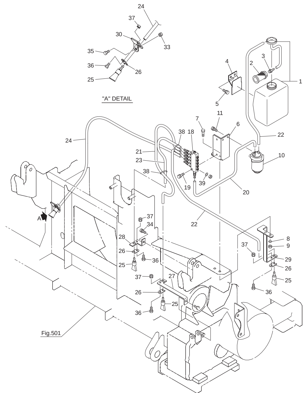
Fig.520. 給油
