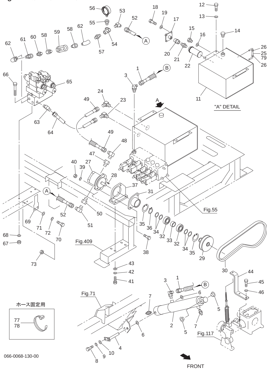
Fig.431. 油圧(メイン)
