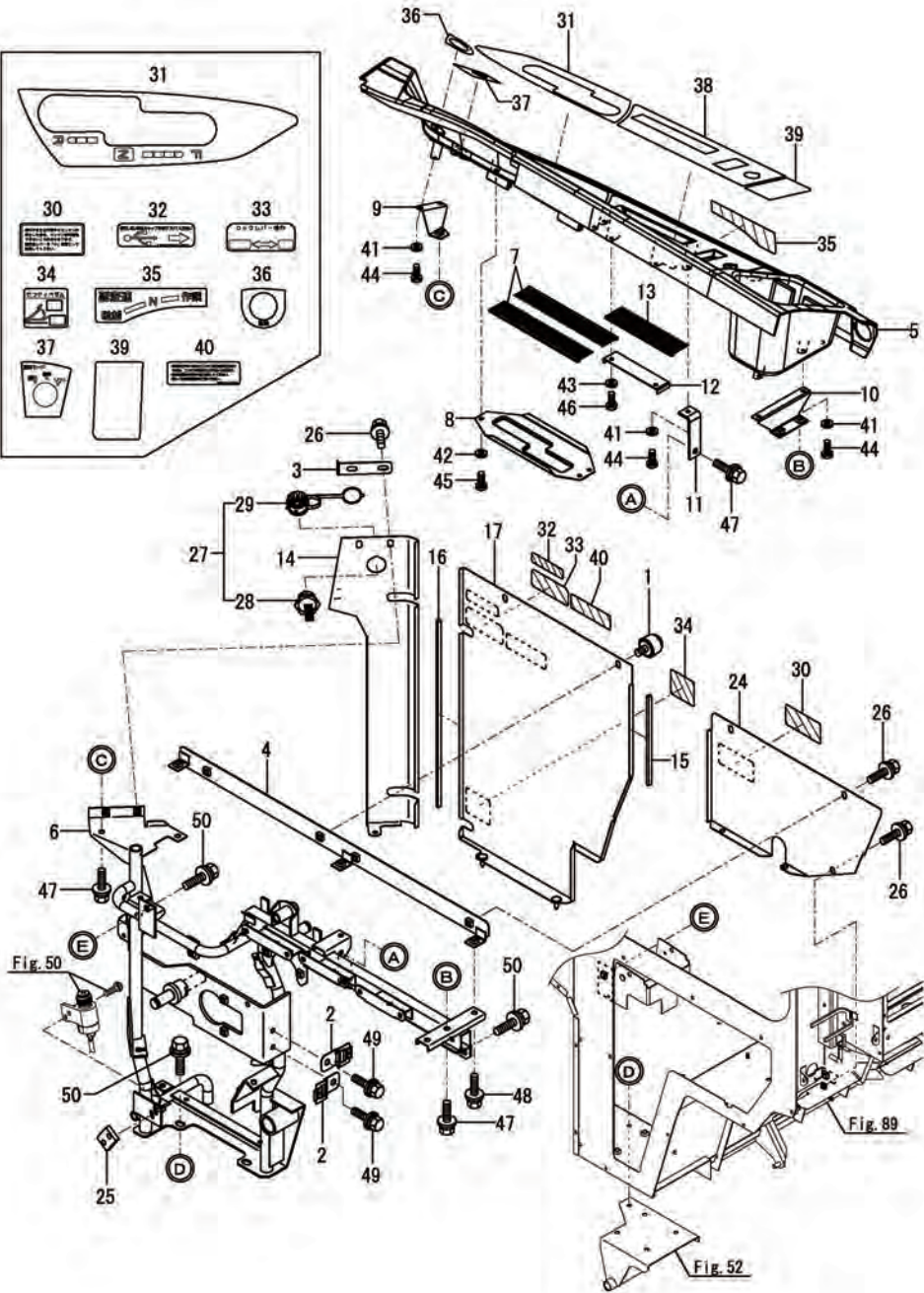
0CNP7-M01300 走行部(2) Fig.47. サイドコラム(1)
