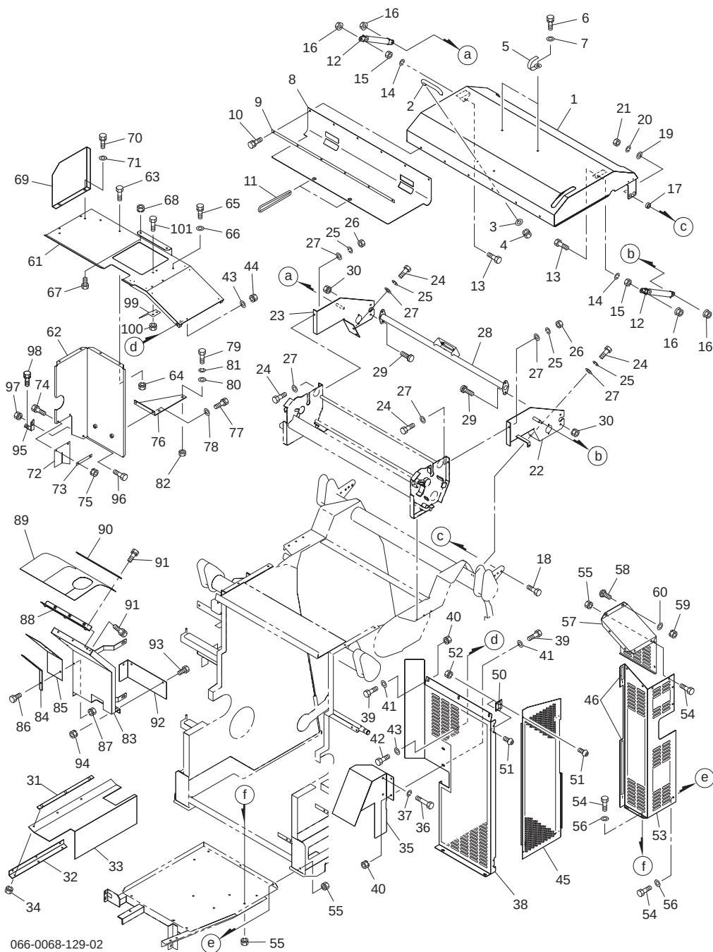
Fig.428. カバー(3)
