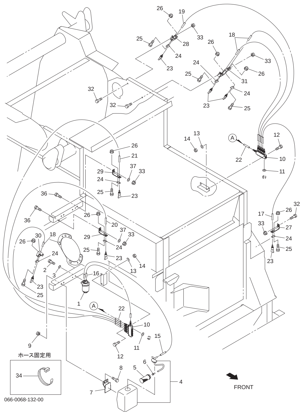
Fig.430. 給油
