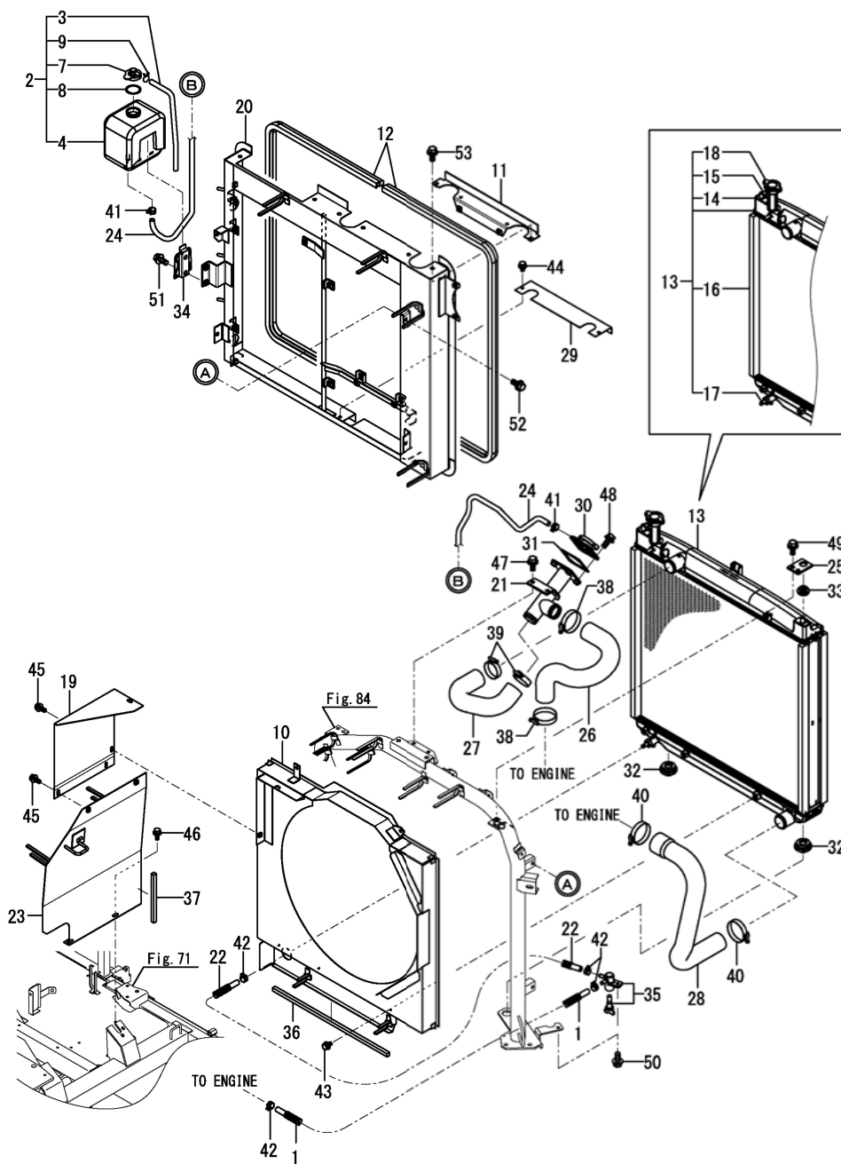
Fig.11. ラジエータ
