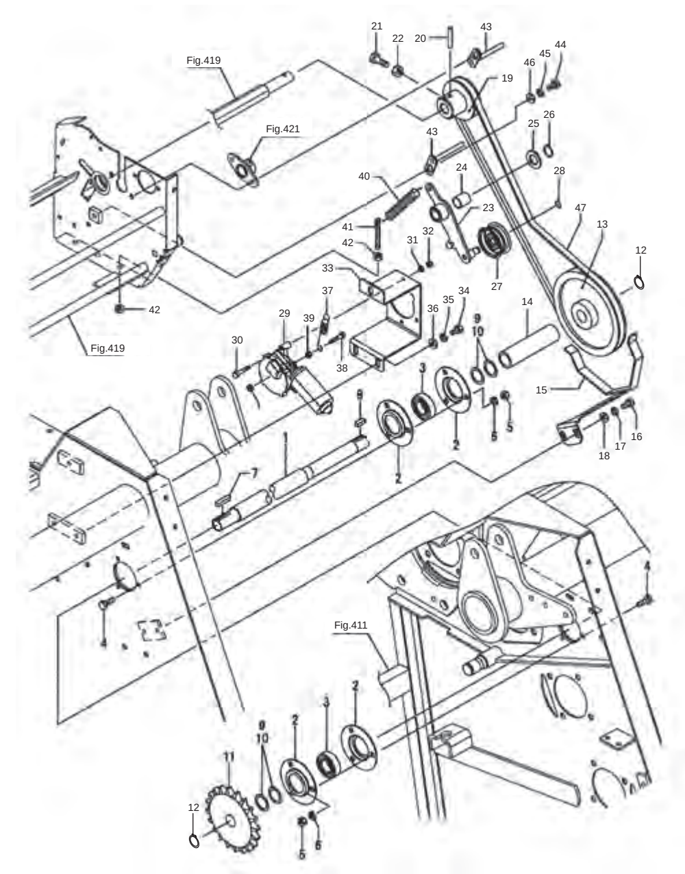
Fig.418. 駆動(ネット)
