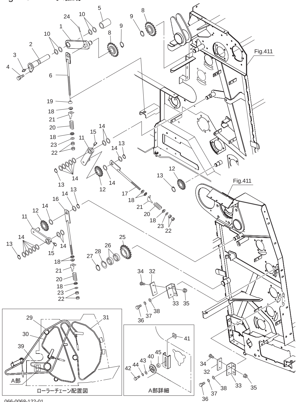
Fig.413. ローラ駆動
