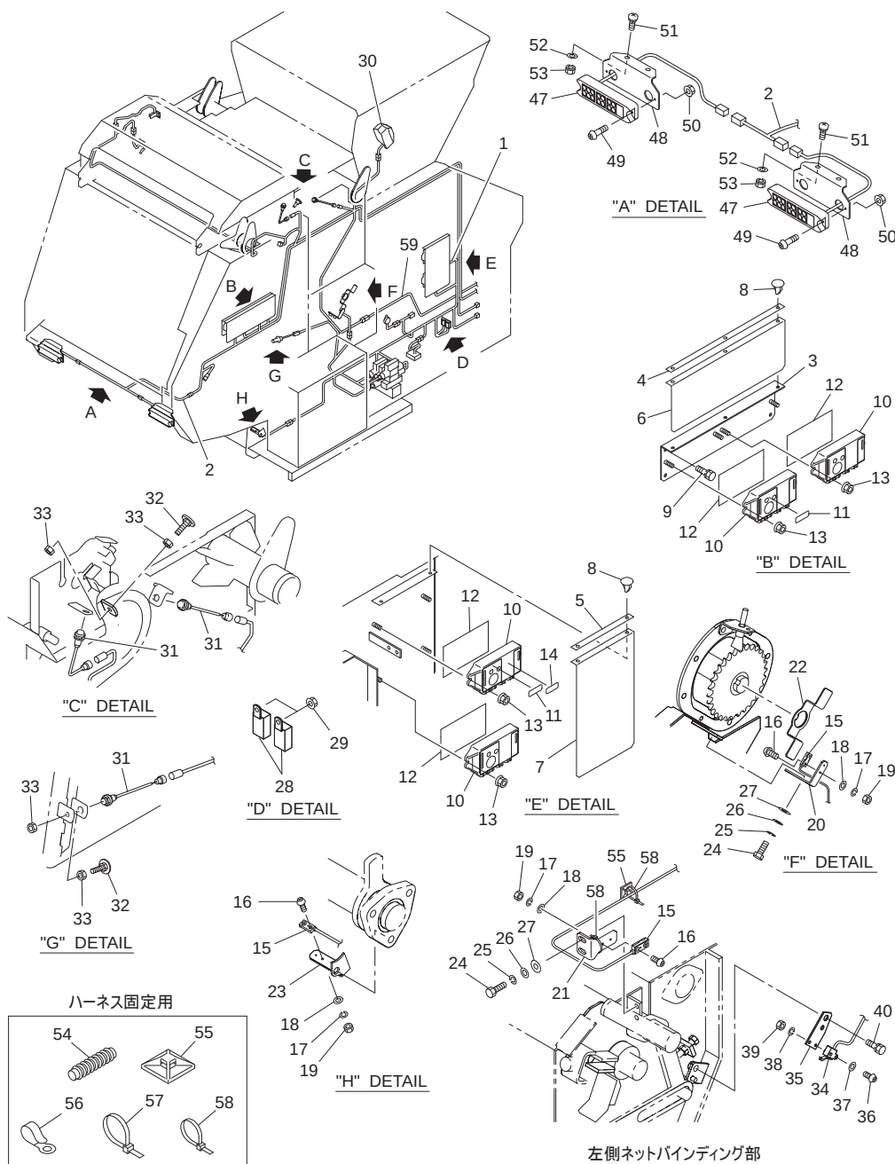
Fig.436. 電装(2)
