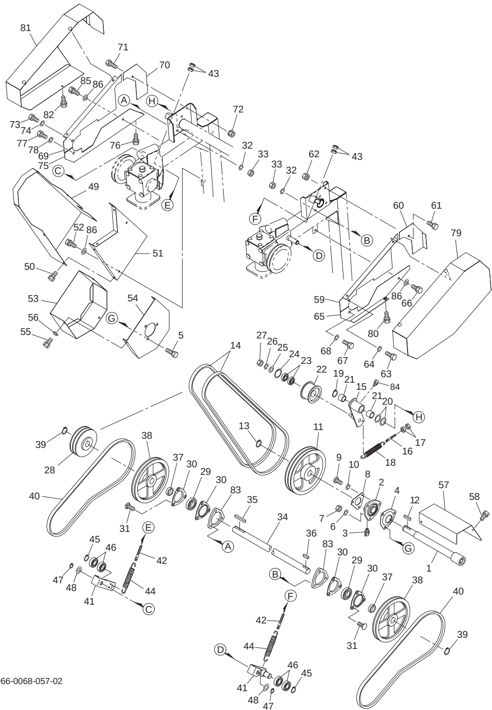
Fig.513. 駆動;ドラム
