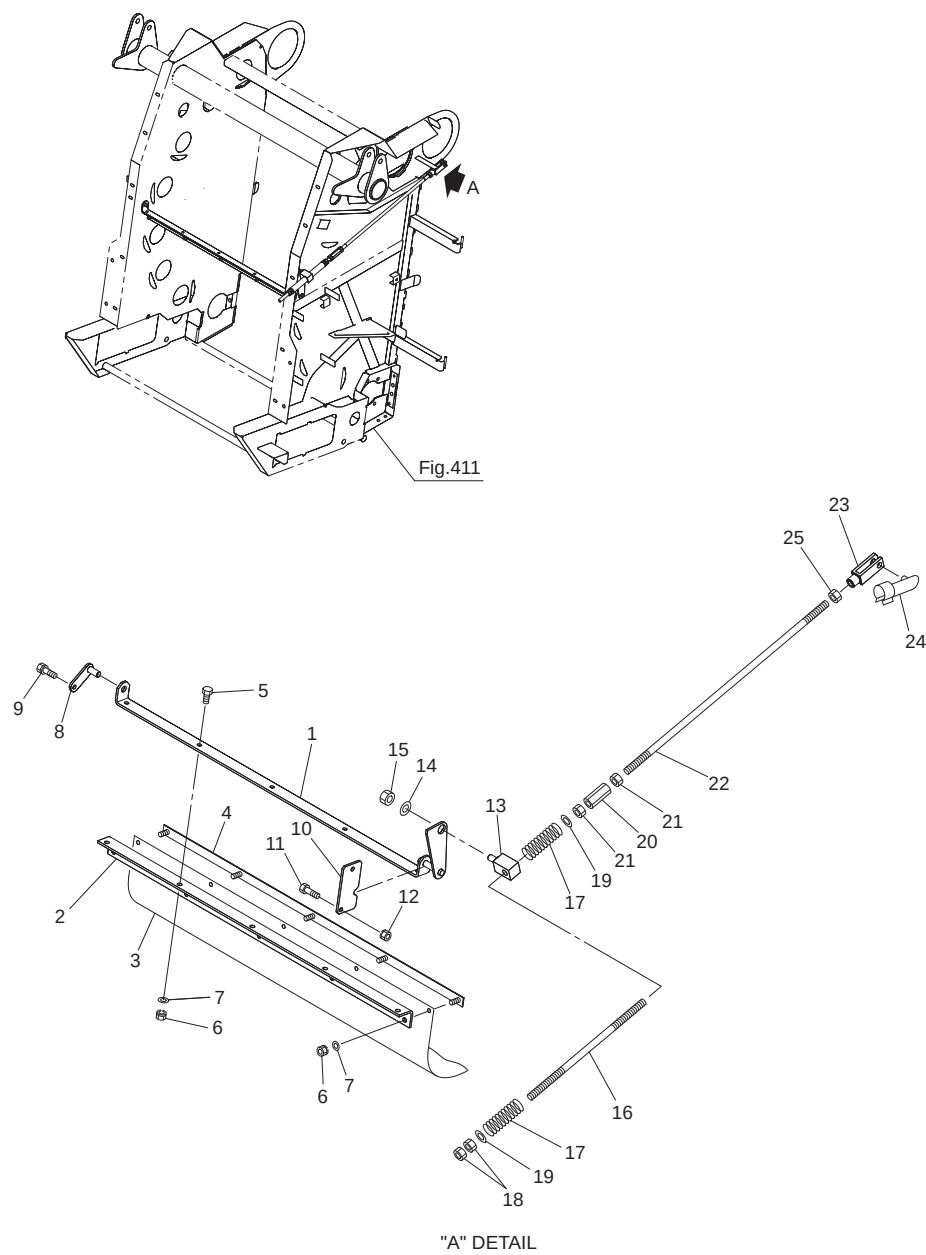
Fig.417. コボレ止め
