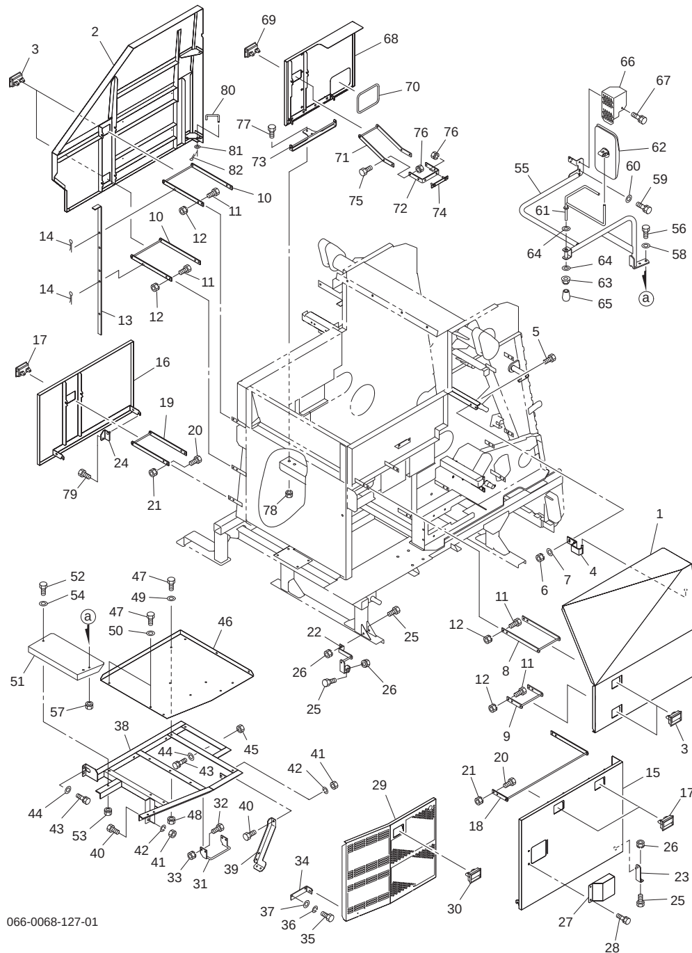
Fig.426. カバー(1)
