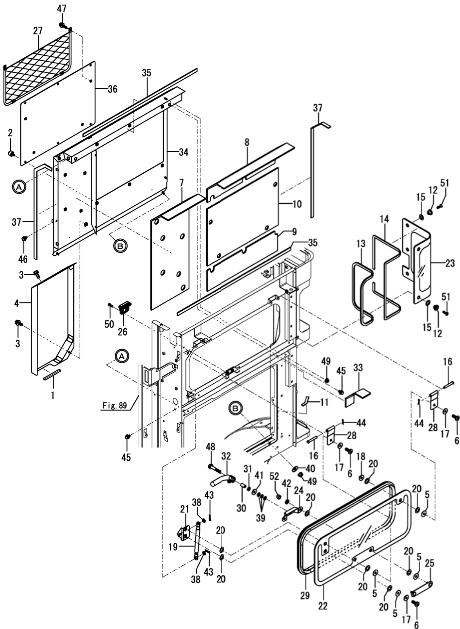
OCNP7-M01300 キャビン部 Fig.92. キャビン艀装(後)
