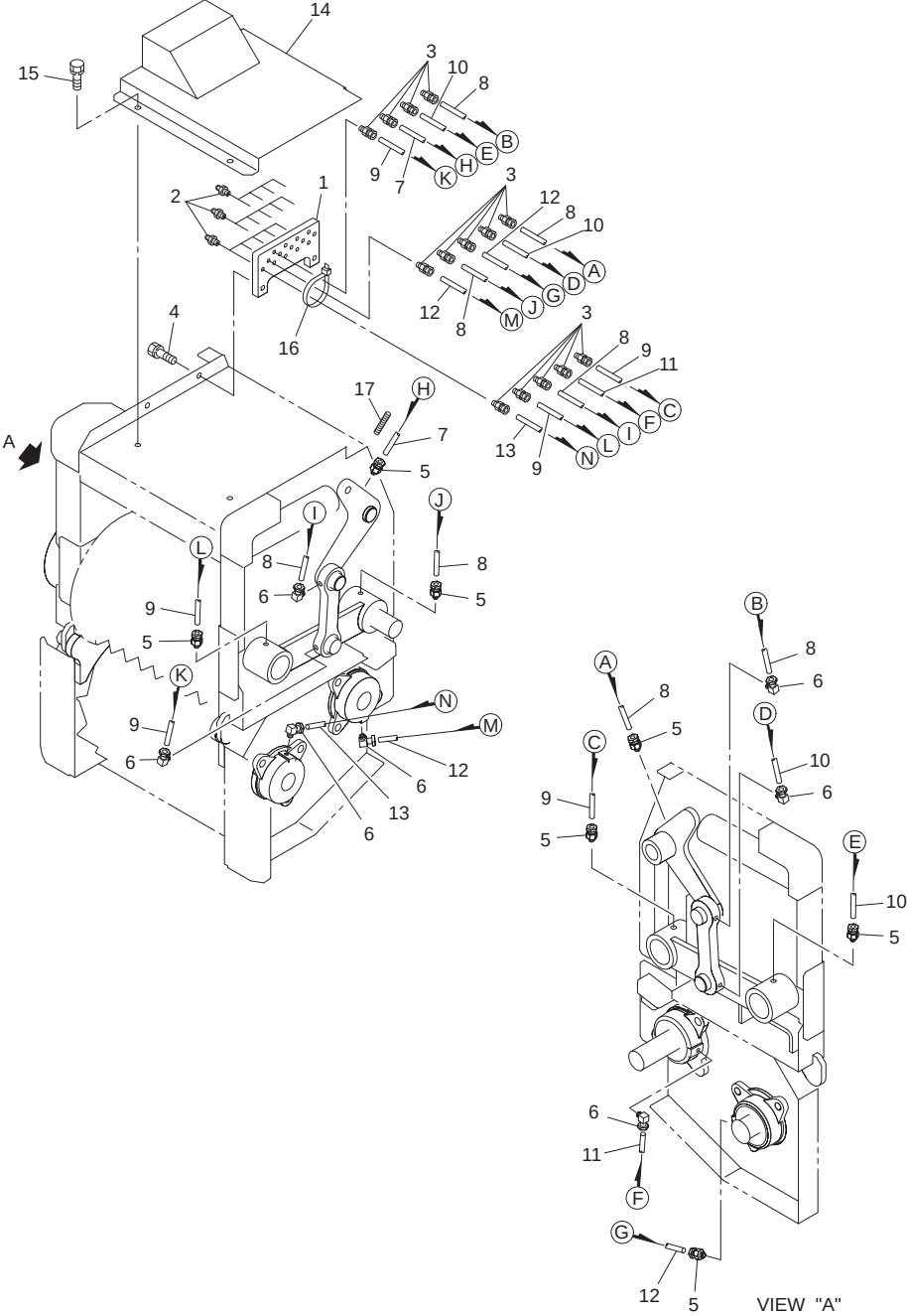
Fig.521. 給脂
