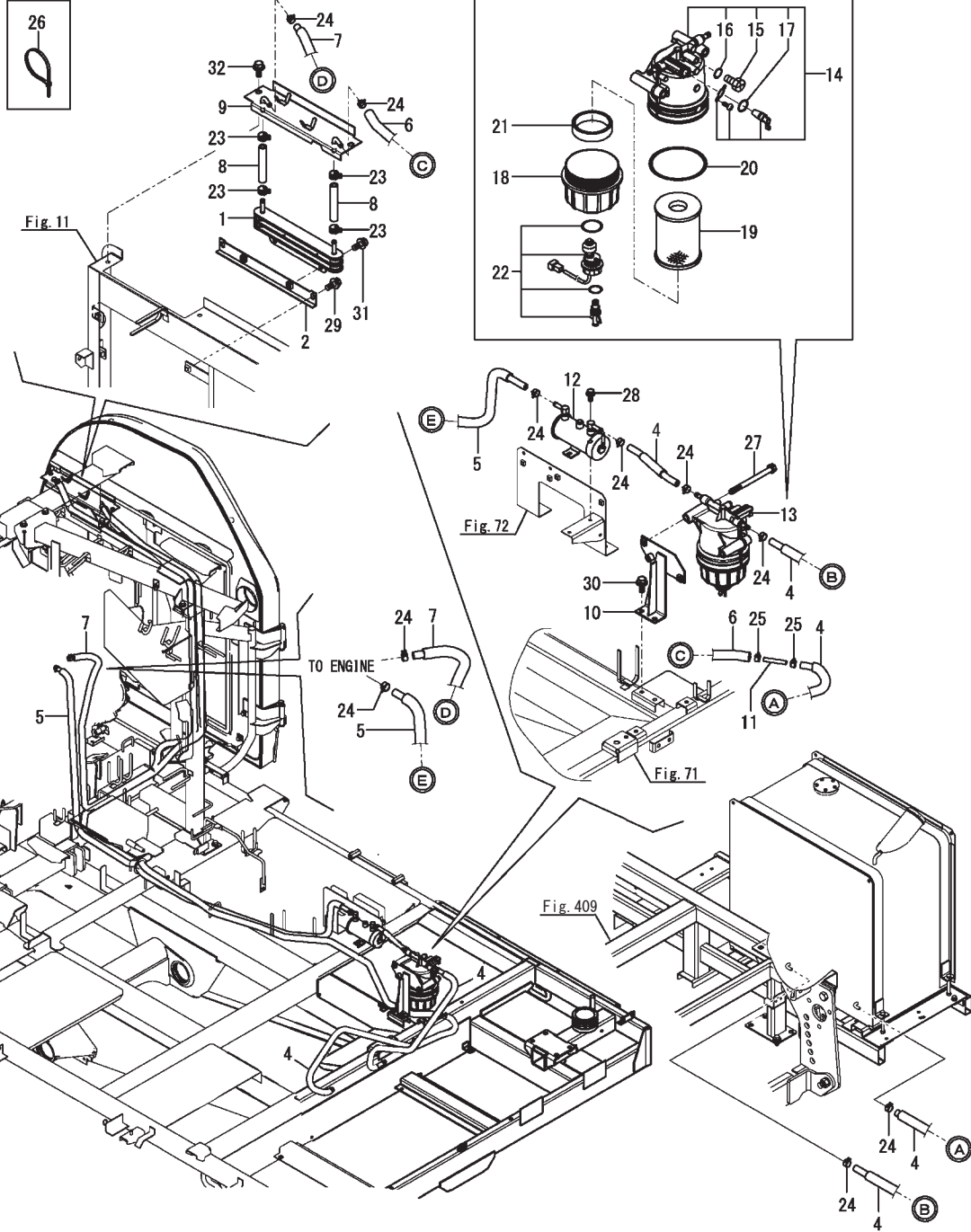
Fig.5. 燃料タンク(2)
