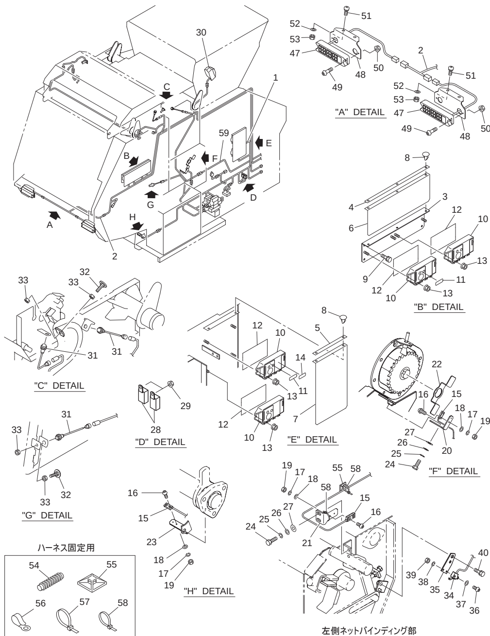
Fig.436. 電装(2)
