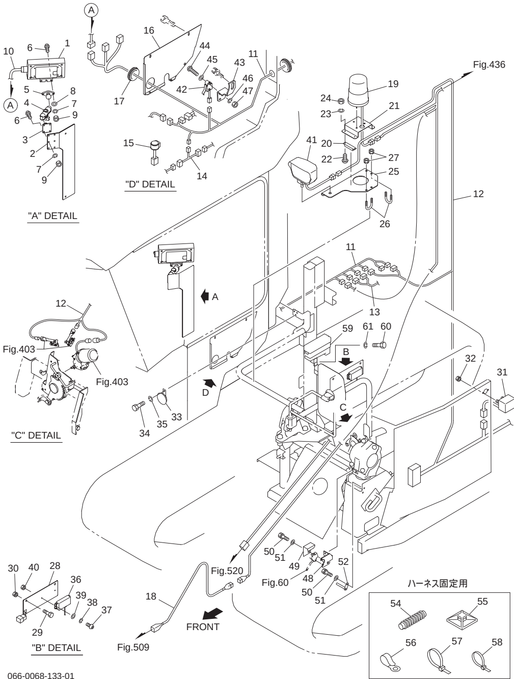
Fig.435. 電装(1)
