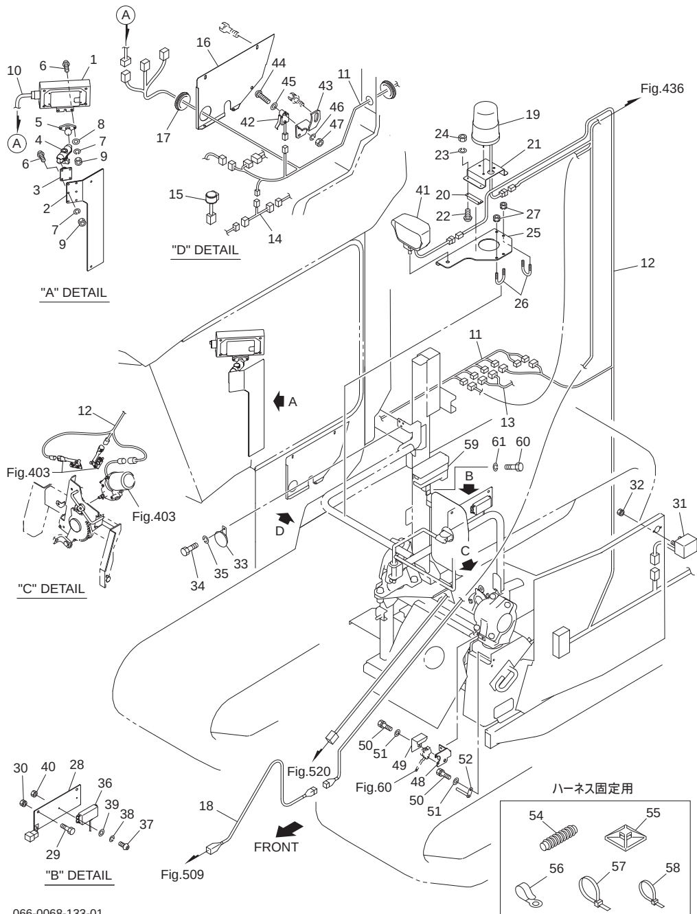
Fig.435. 電装(1)
