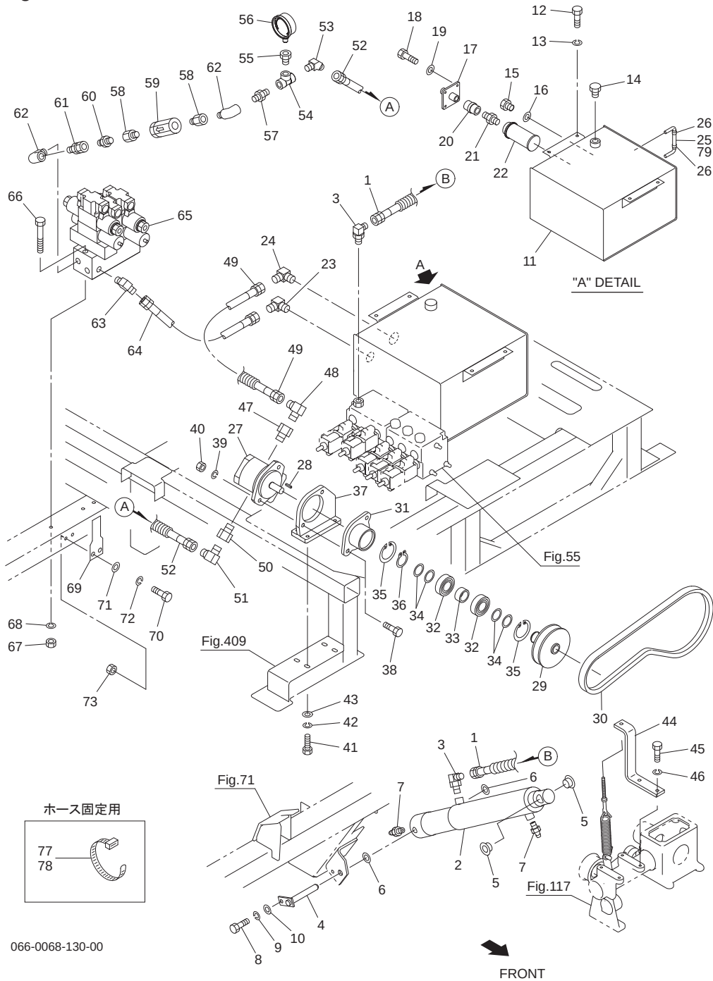
Fig.431. 油圧(メイン)
