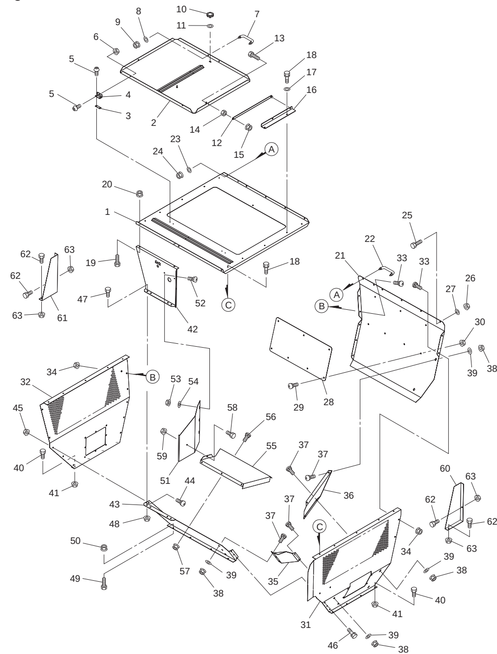
Fig.404. ホッパ
