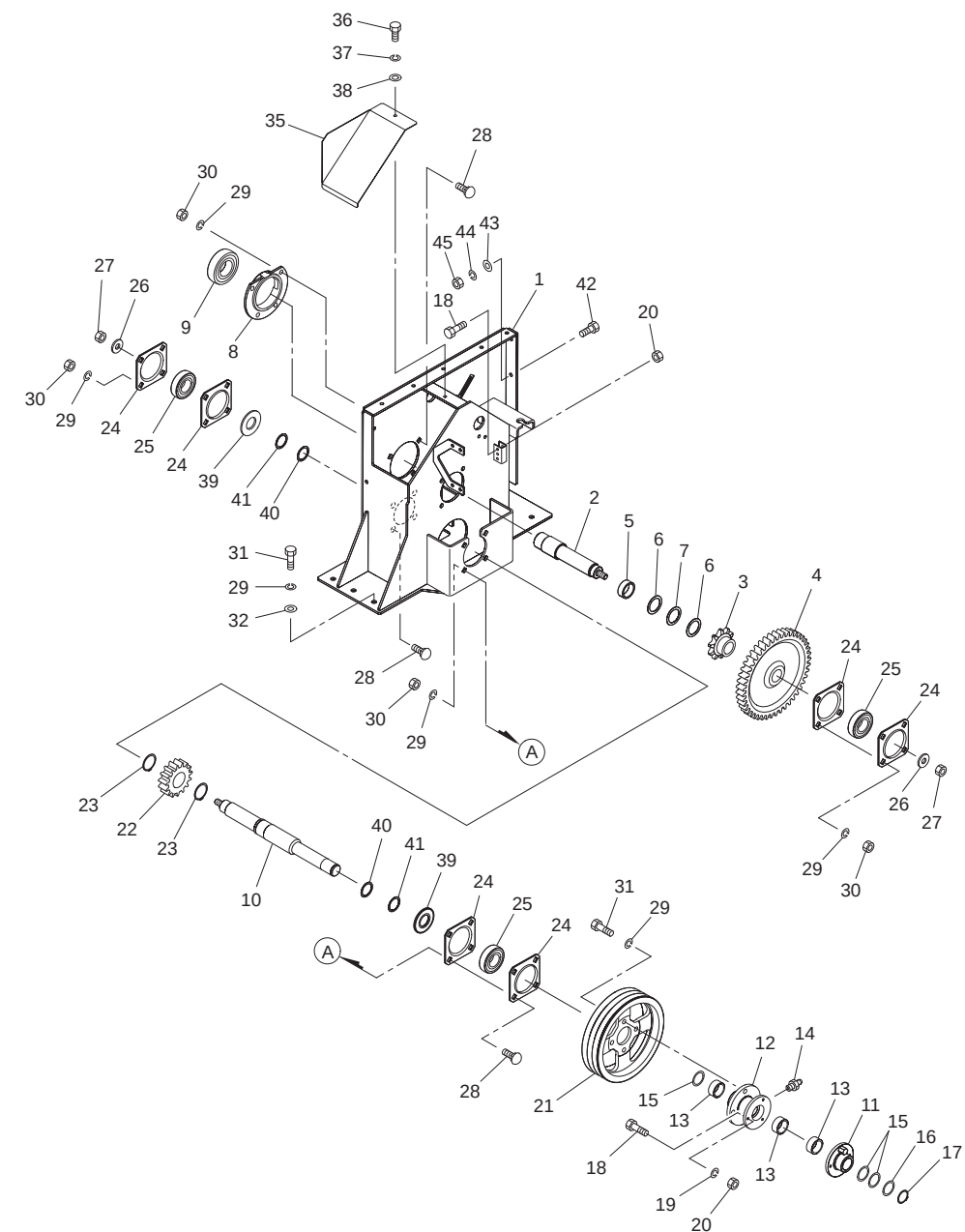
Fig.408. 駆動; 2
