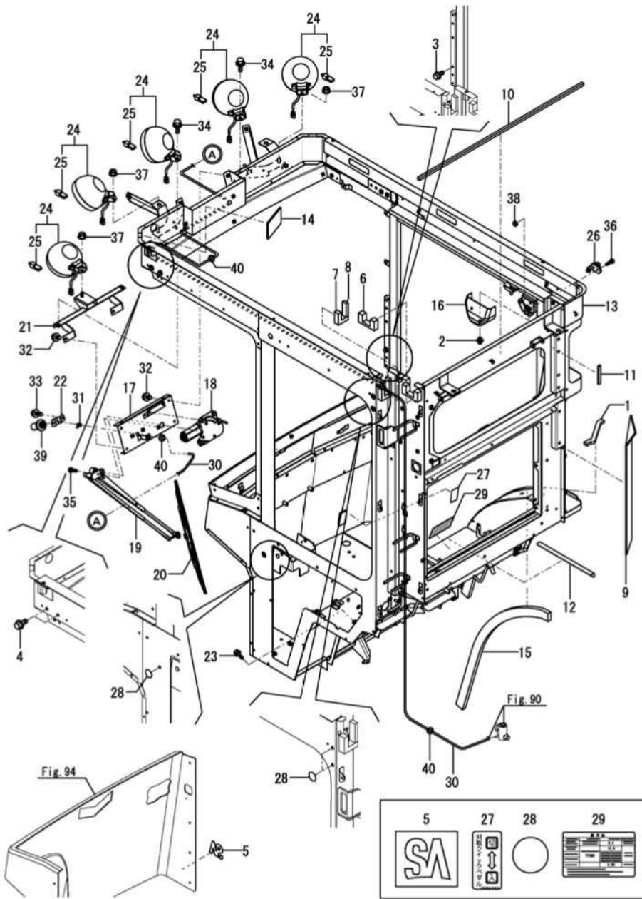
OCNP7-M01300 キャビン部 Fig.89. キャビン(本体)
