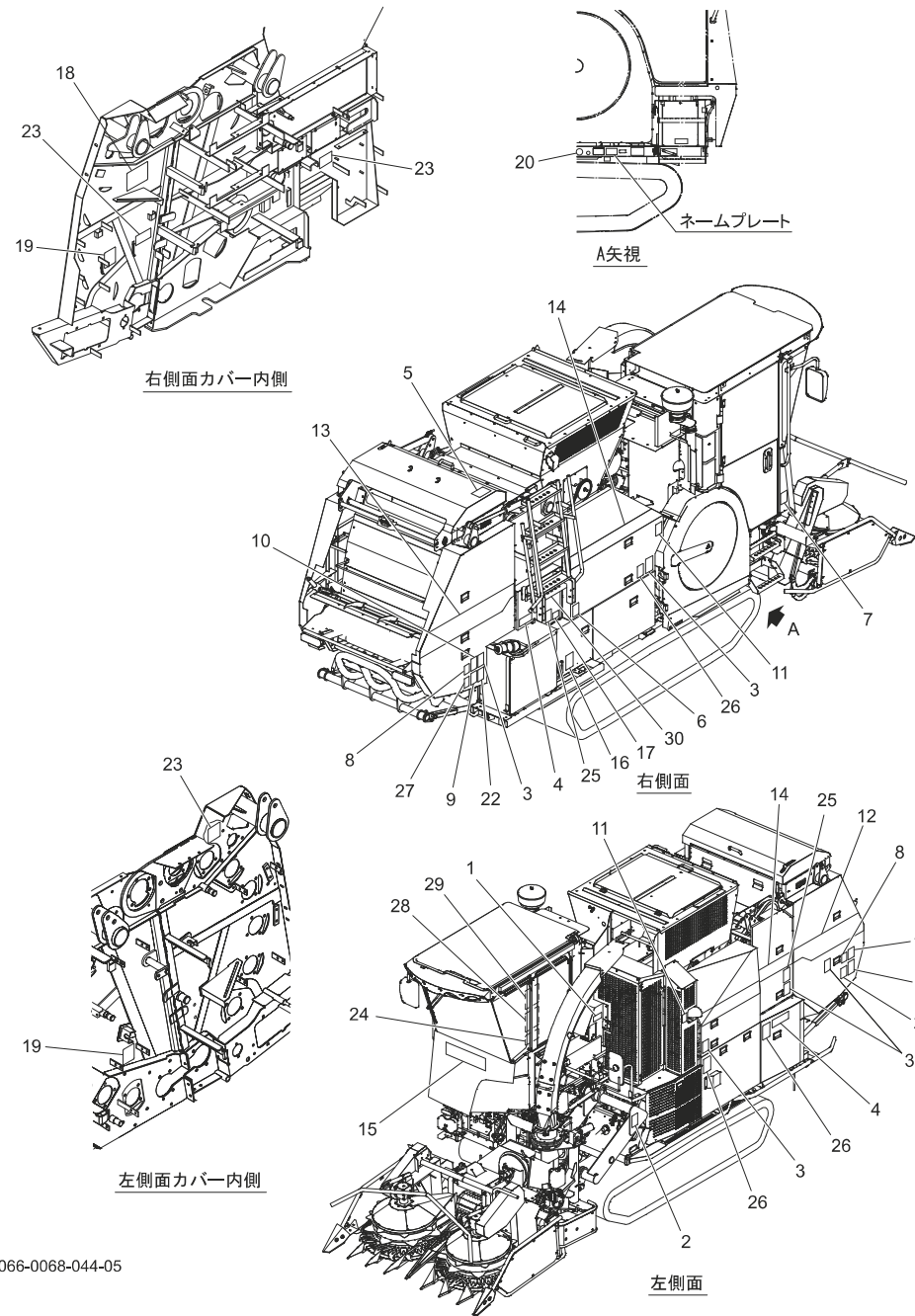
Fig.439. ラベル
