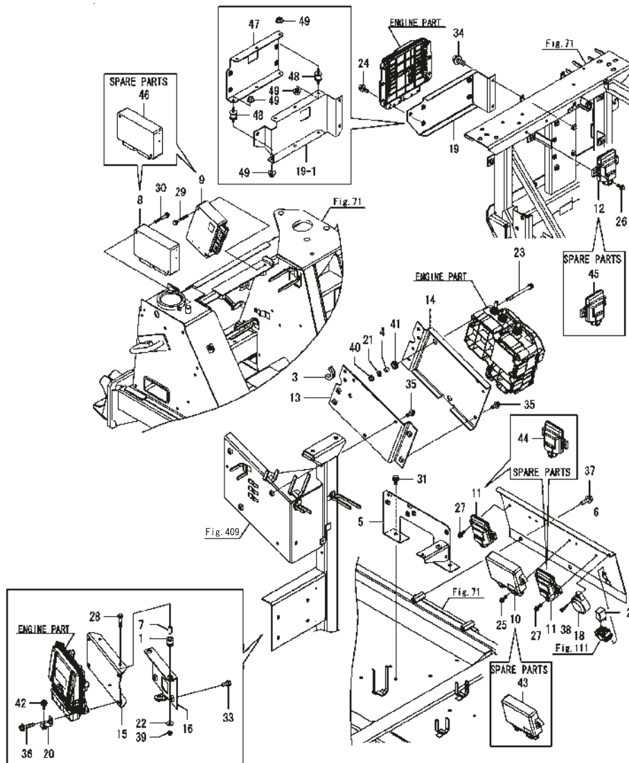
Fig.72. コントロール(シャーシ)
