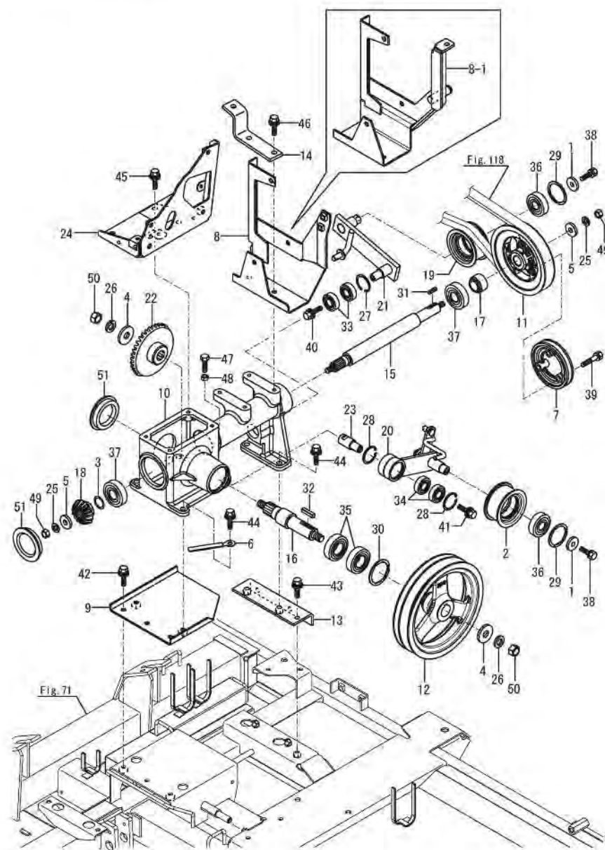
Fig.117. ポンプ入力
