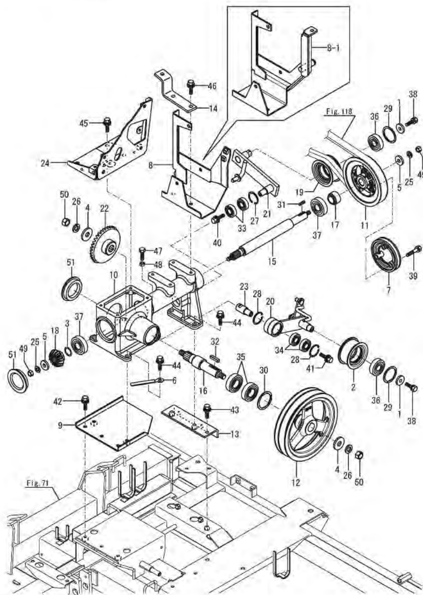
Fig.117. ポンプ入力
