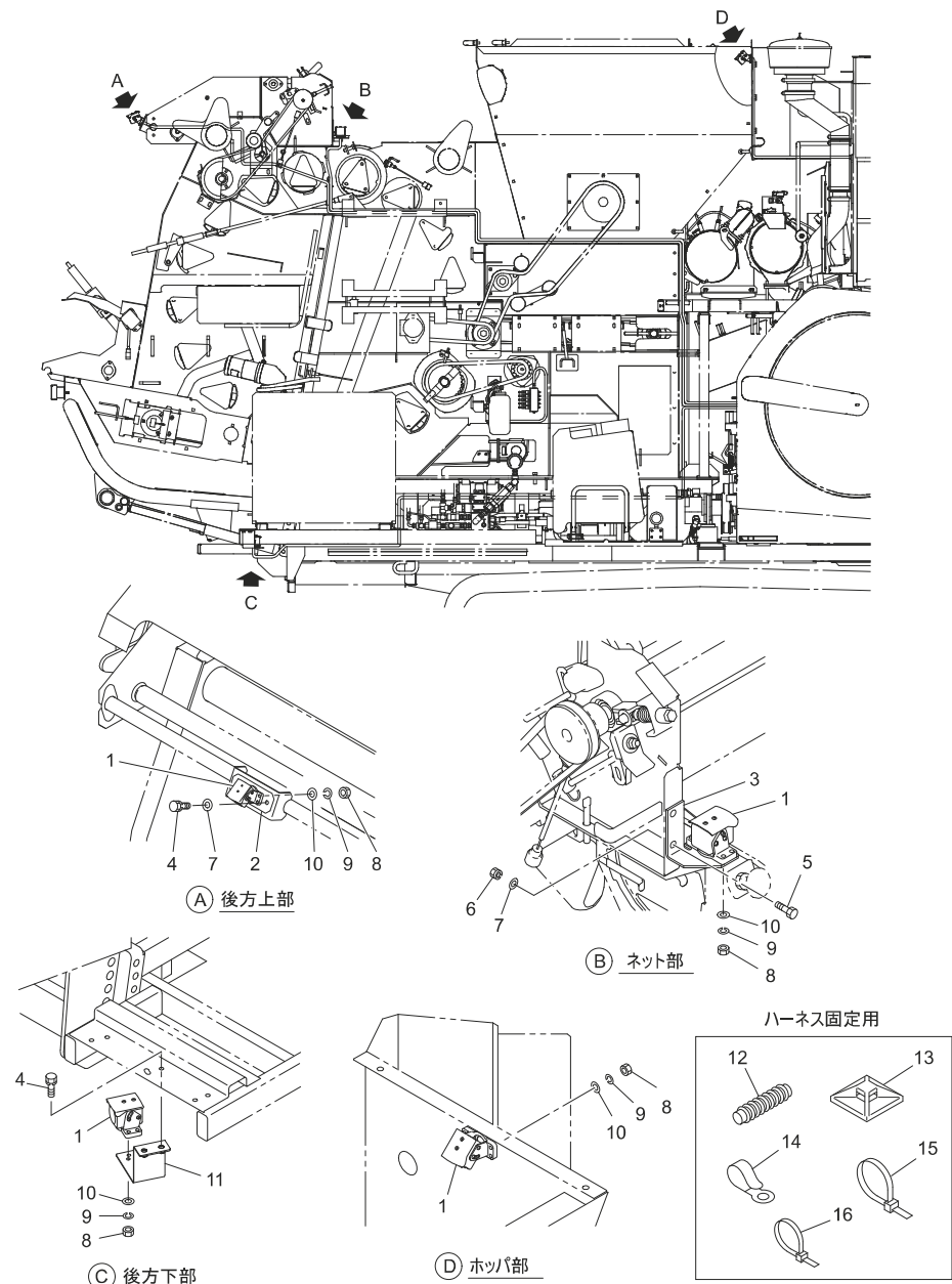
Fig.437. 電装(3)
