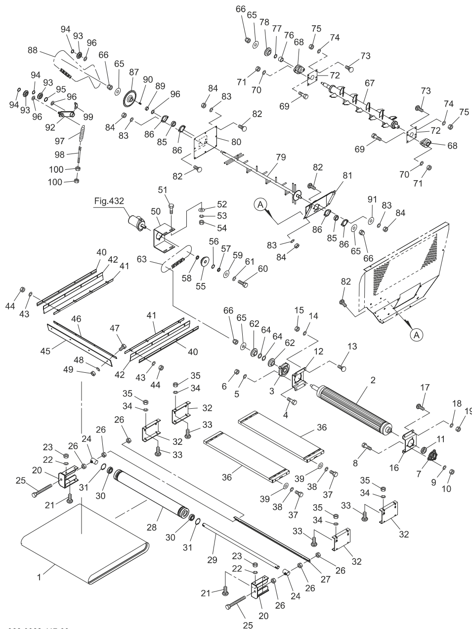
Fig.406. コンベア
