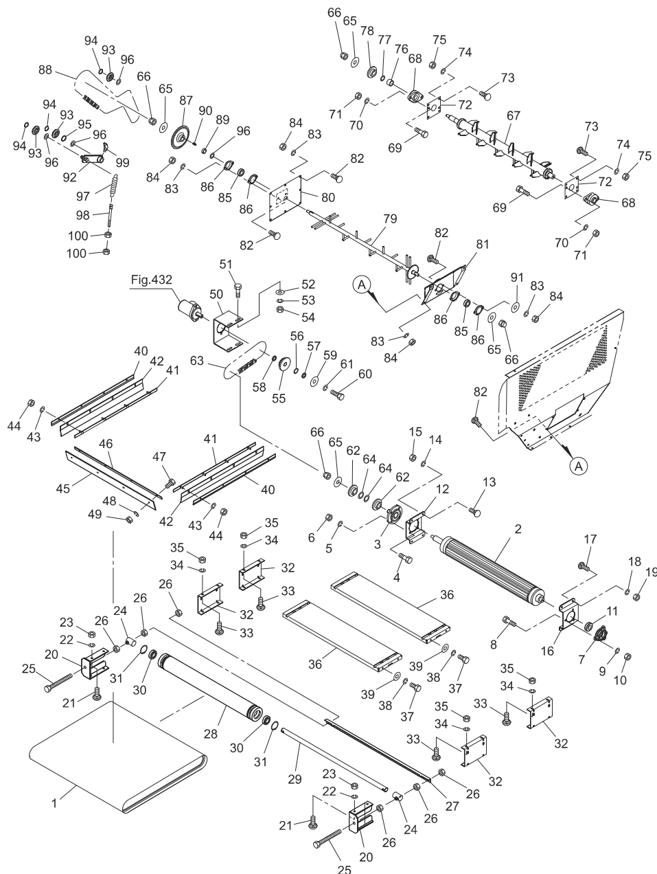
Fig.406. コンベア
