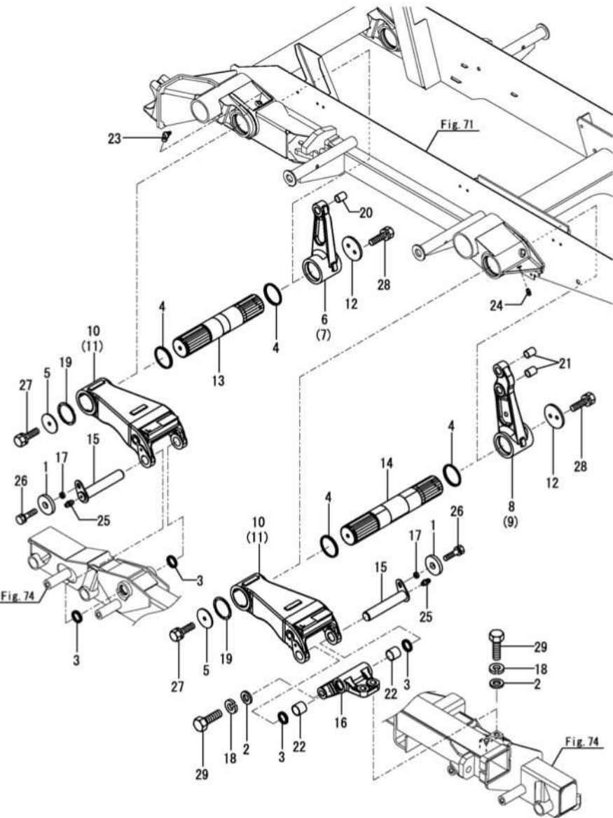
Fig.82. スイング(1)
