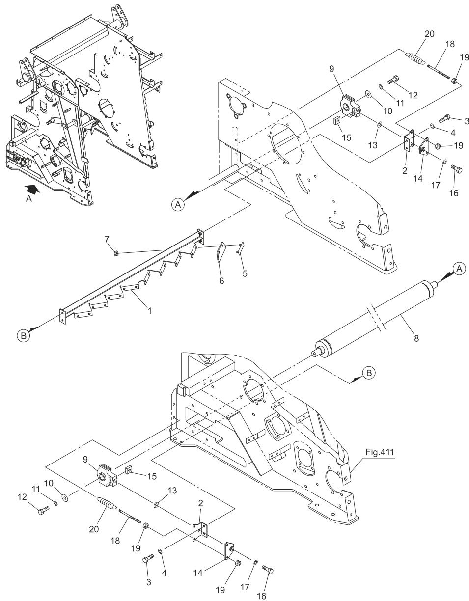
Fig.414. 成形ベルト(1)
