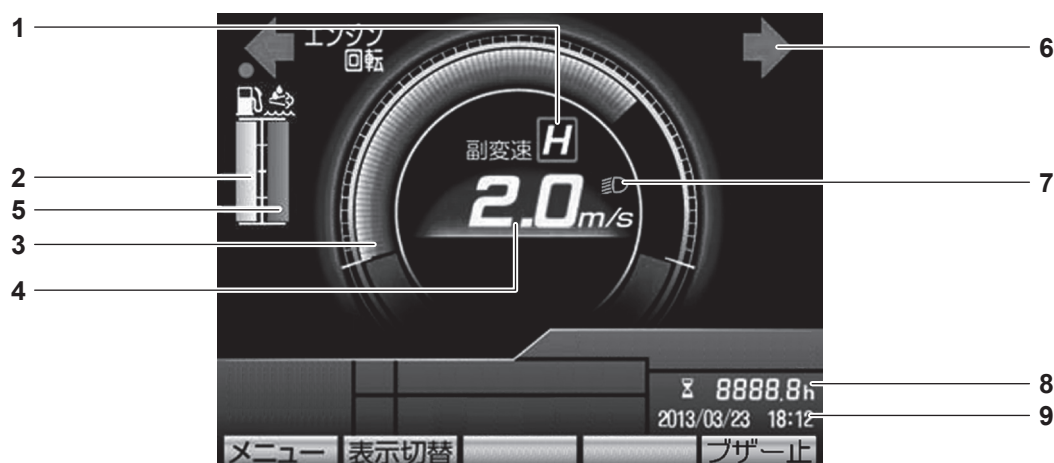
非作業時(作業クラッチレバー「OFF」)の画面
