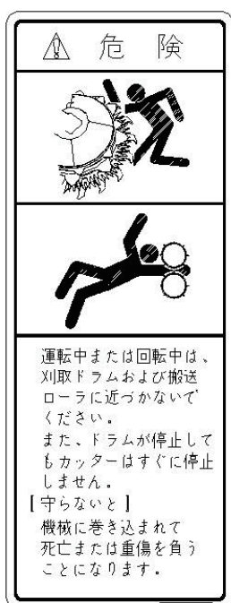
(11) 1511450000 ラベル 危険
