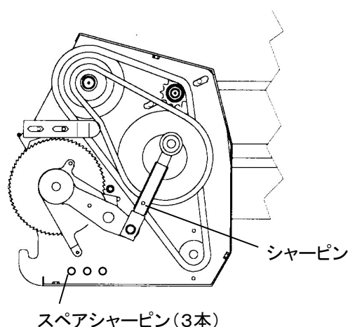
フロアコンベアギアボックス
