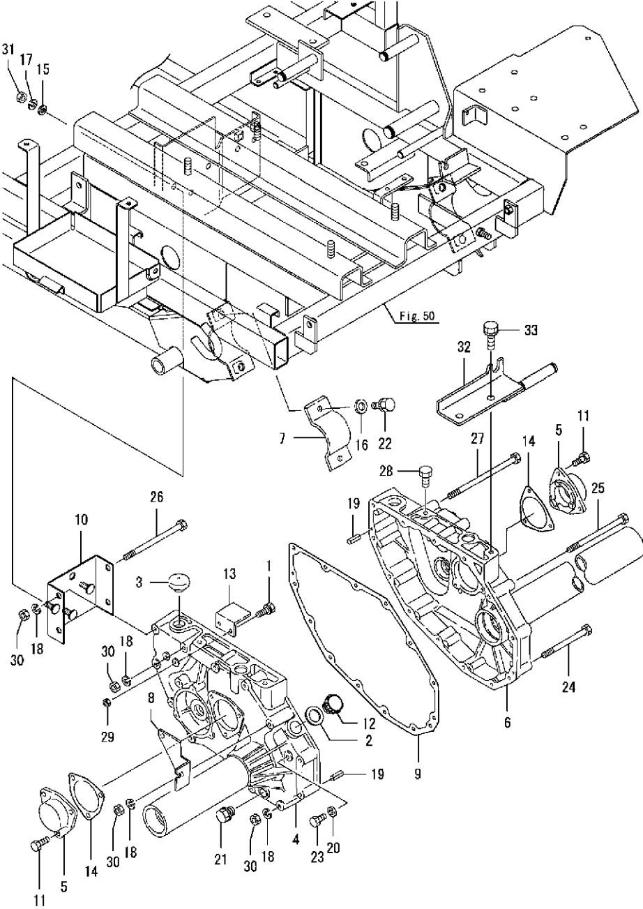
OCNP6-M02290 走行部(1) Fig.29. ミッションケース
