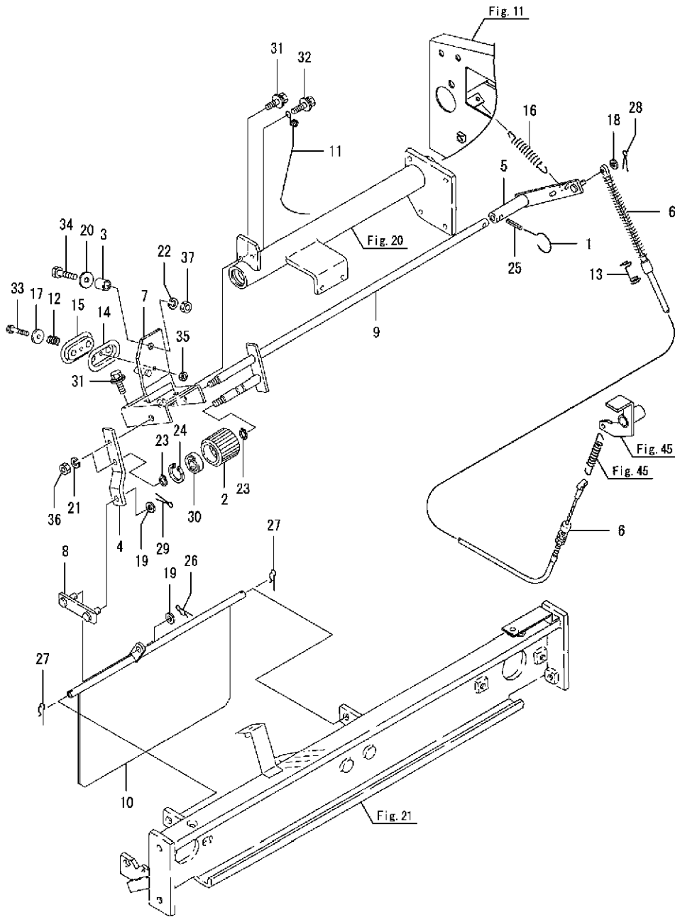
OCNP6-M02290 結束部 Fig.23. 結束操作機器
