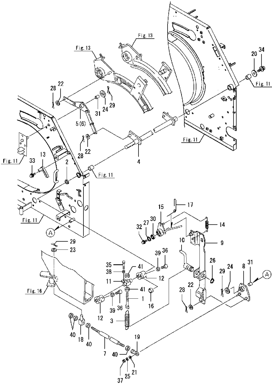
OCNP6-M02290 ベーラ部 Fig.14. 下チャンバー回転
