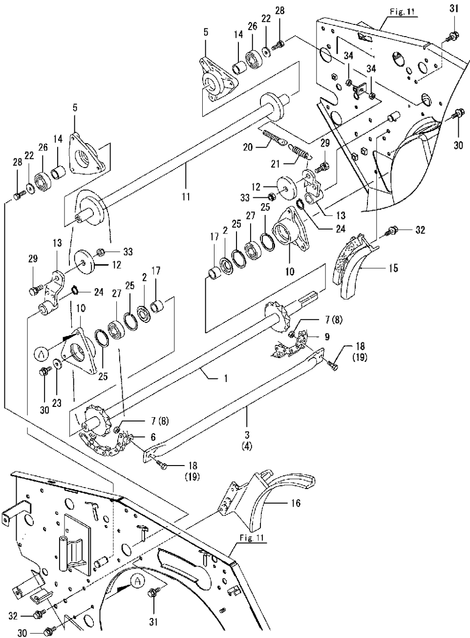
OCNP6-M02290 ベーラ部 Fig.12. 上チャンバー
