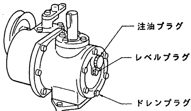
ギヤボックス
