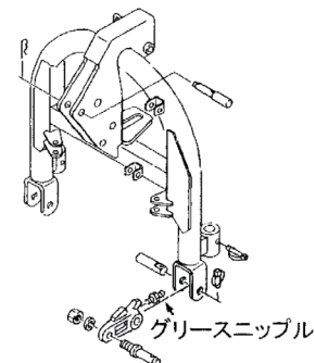
8. ローリング ブラケット
