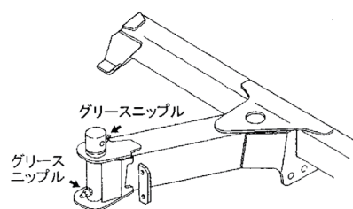
7. メインフレーム
