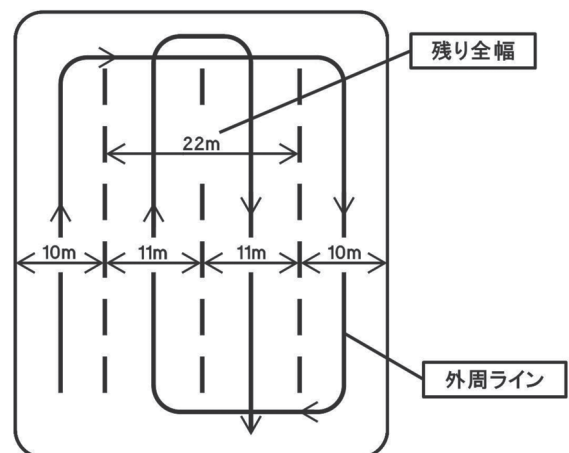
散布間隔：10m 誘導幅の下限値：80% 残り全幅22mの場合
