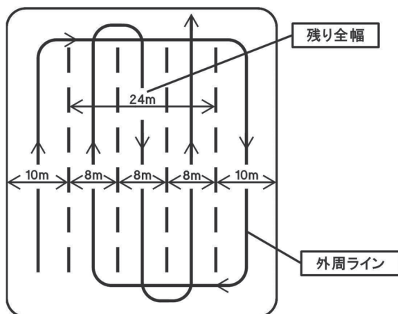
散布間隔：10m 誘導幅の下限値：80% 残り全幅24mの場合
