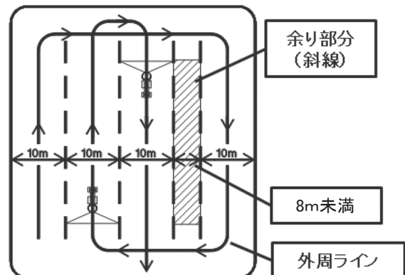
「余り部分」が生じるほ場の例 ※散布間隔：10m 誘導幅の下限値：80%
