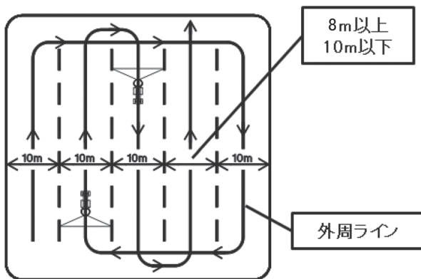
「余り部分」が生じないほ場の例 ※散布間隔：10m 誘導幅の下限値：80%
