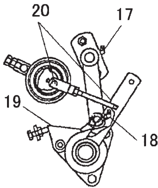
17.ハウジング 18. ラッチ 19. ストップバ 20. クランクアーム支点
