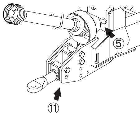
ヒッチカン (THM11010M・13010M)、PIC軸関係
