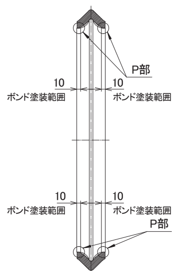
ゴムホイール断面
